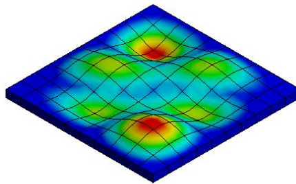
Mod 7
