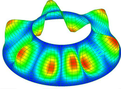
Mode 1-2. 343 Hz.
