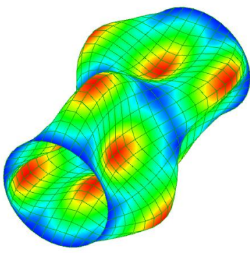
209 Hz. Mod 13-14
