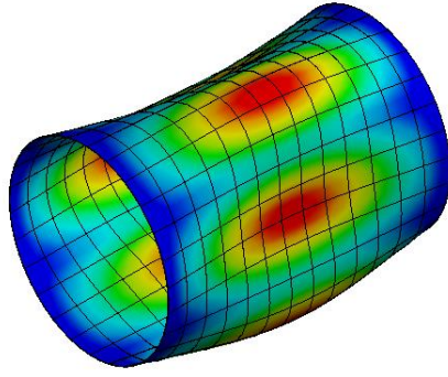
Mod 15
