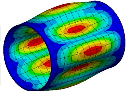
Mod 4
