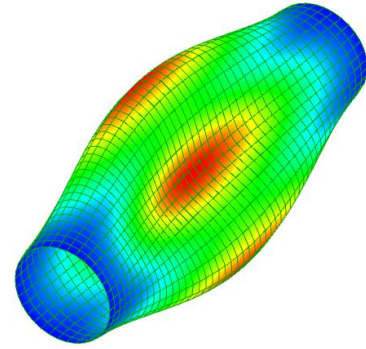
57 Hz. Mod 3-4
