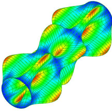
127 Hz. Mod 13-14
