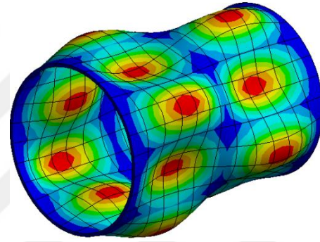
Mod 10
