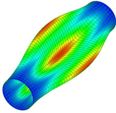
55.7 Hz. Mod 1-2
