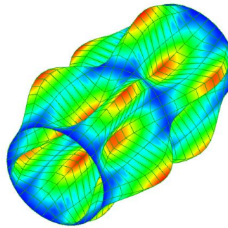
188 Hz. Mod 11-12
