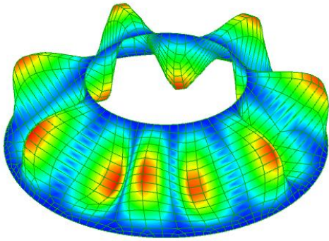
Mode 5-6. 352 Hz.
