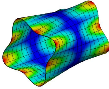
Mod 17
