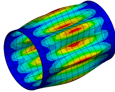
Mod 10
