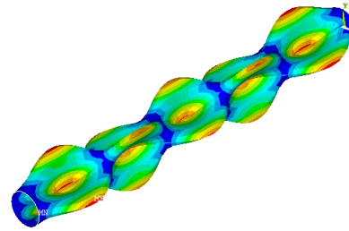
Mod 19-) 766.86 Hz.
