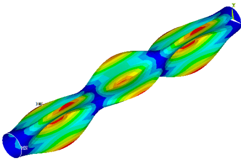
Mod 13-) 541.02 Hz.
