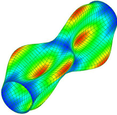
87.1 Hz. Mod 5-6
