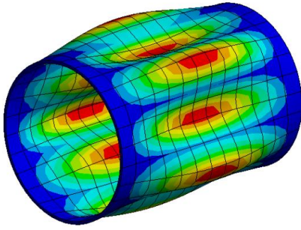
Mod 7
