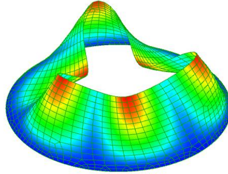
Mode 7-8. 316 Hz.
