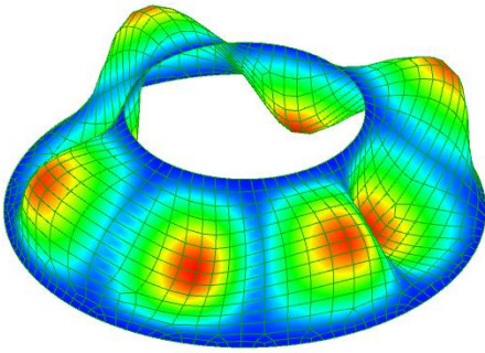
Mode 9-10. 397 Hz.
