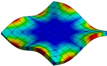
Mod 15
