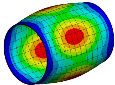
Mod 6
