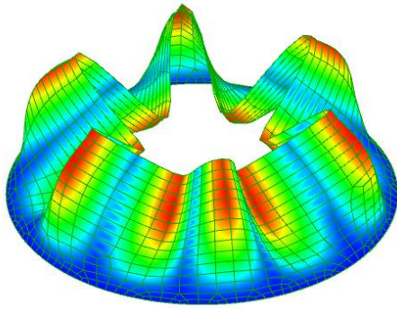
Mode 5-6 . 277 Hz.
