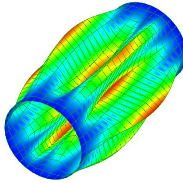
223 Hz. Mod 15-16
