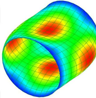
365 Hz. Mod 15-16
