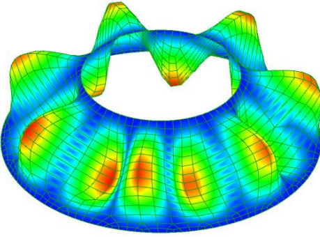
Mode 5-6. 358 Hz.
