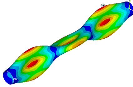
Mod 11-) 526.79 Hz.
