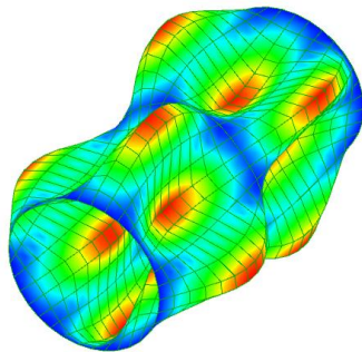
175 Hz. Mod 9-10
