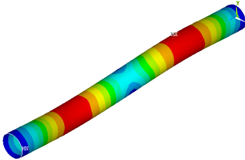
Mod 17-) 707.24 Hz.
