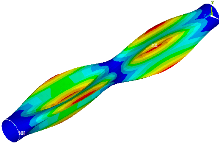
Mod 9-) 493.30 Hz.
