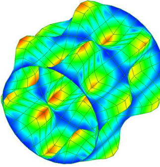
339 Hz. Mod 13-14
