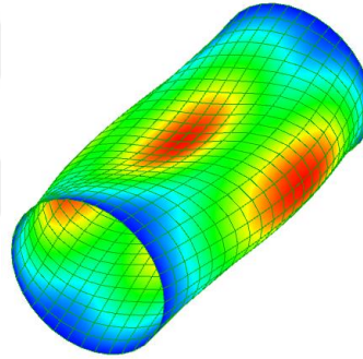
160 Hz. Mod 7-8
