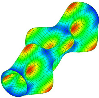
139 Hz. Mod 17-18
