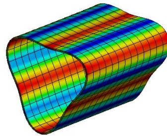
Mod 12
