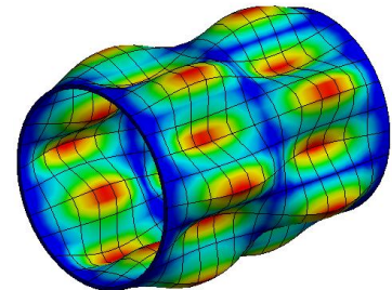
Mod 20
