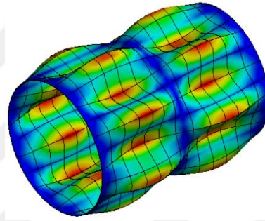
Mod 12
