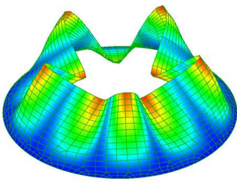
Mode 1-2. 241 Hz.
