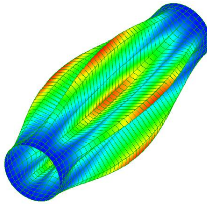
150 Hz. Mod 19-20
