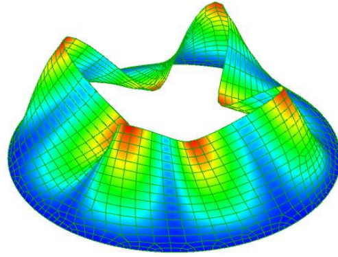
Mode 3-4. 246 Hz.
