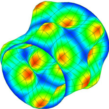
387 Hz. Mod 19-20
