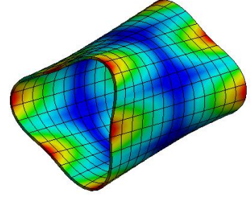
Mod 14
