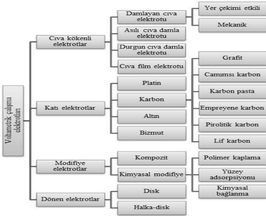
Şekil 1.6.Voltammetride kullanılan çalışma elektrotlarının genel bir sınıflandırması
