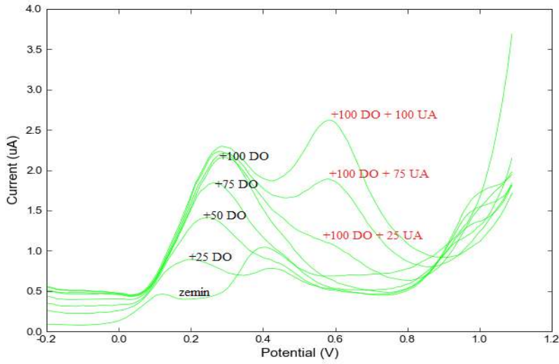
Şekil 4.19. Zencefil modifyeli elektrodun zeminde, artan DA ve UA miktarlarına göre pH=7 0,1 M PBS tamponunda DP voltamogramı
