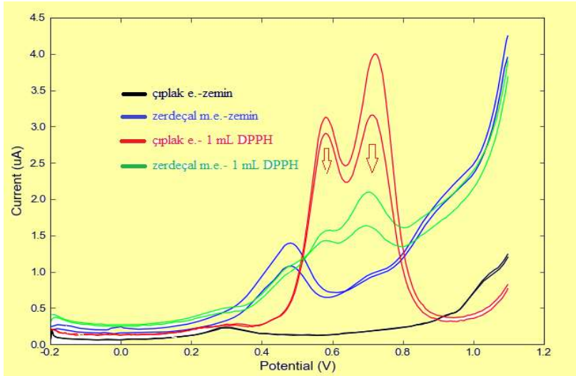
Şekil 4.24.Zeminde çıplak (siyah) ve zerdeçal (mavi) modifiyeli elektrotlarla, 10^{-3} M DPPH test çözeltisi içinde çıplak (kırmızı) ve zerdeçal (yeşil) modifiyeli elektrotlarla pH=2 0,1 M PBS tamponunda diferansiyel puls voltamogramlar
