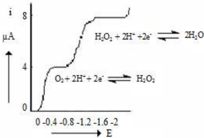
Şekil 1.5. Damlayan cıva elektrotunda, hava ile doyurulmuş 0,1 mol L -1 KCl çözeltisinde oksijenin indirgenme dalgaları
