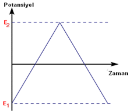
Şekil1.2. Doğrusal taramalı ve dönüşümlü voltametride potansiyel taramasının zamanla değişimi
