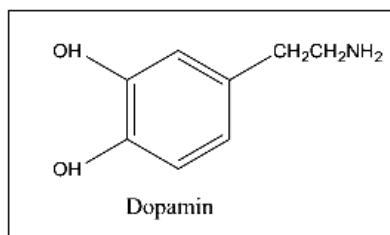
Şekil 2.6. Dopaminin molekül formülü
