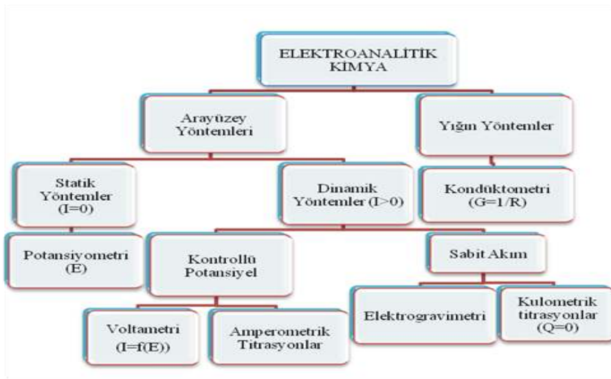
Şekil 1.1.Elektroanalitik yöntemlerin sınıflandırılması
