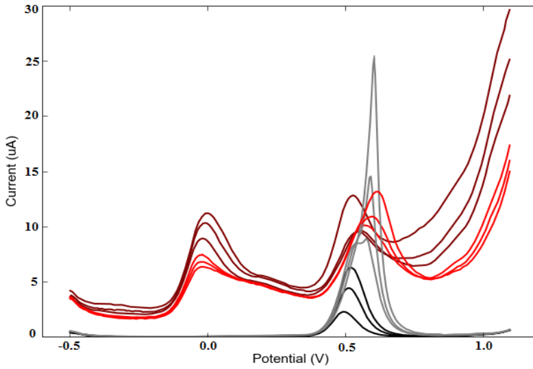
Şekil 4.15. İlk üç ölçümde 50 \mu L artan DA (kırmızı) ve sonraki üç ölçümde 50 \mu L artan UA (gri) miktarlarına bağlı çıplak (siyah) ve kına modifiyeli elektrodun (koyu kırmızı) pH=2, 0,1 M PBS tamponunda DP voltamogramları
