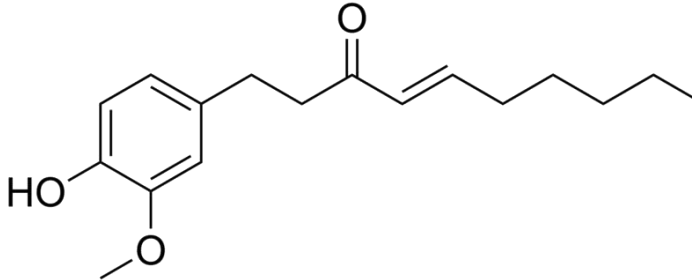
Şekil 2.3.Shogaol'ün kimyasal yapısı
