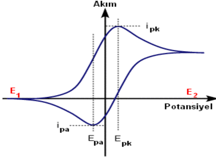
Şekil1.3. Dönüşümlü voltametrde akım potansiyel eğrisi
