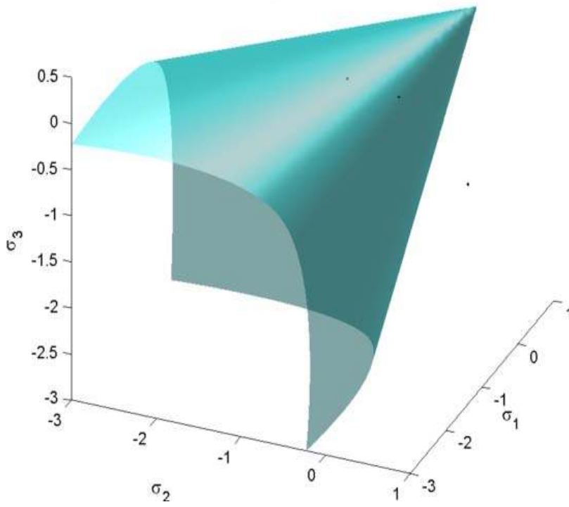
Şekil 2.2. Üç boyutlu William-Warke göçme yüzeyi
