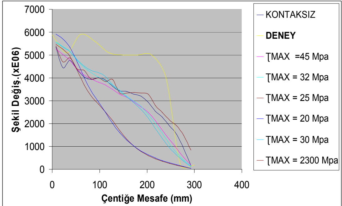
Şekil 2.11. Farklı T_{MAX} değerleri için şekil değiştirme dağılımları
