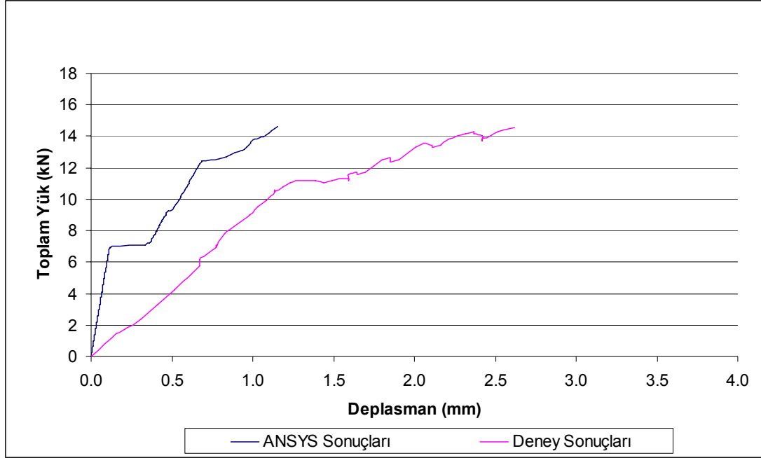
Şekil 5.4 Eleman 13 iin yk Őekil deęiřtirme iliřkisi
