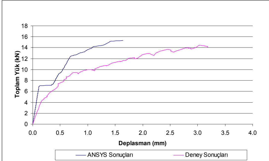
Şekil 5.5 Eleman 14 iin yk Őekil deęiřtirme iliřkisi
