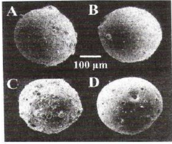
Resim 2.4. Uçucu kül taneciklerinin morfolojik yapısı [59]
