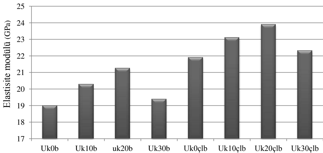
Şekil 4.9. Elastisite modülü grafiği
