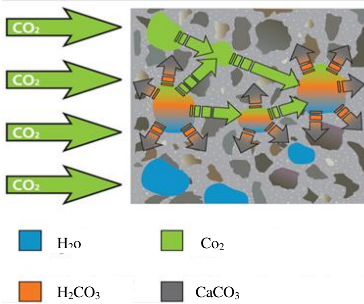
Şekil 2.4. \text{CO}_2 'in Şematik Etkisi
