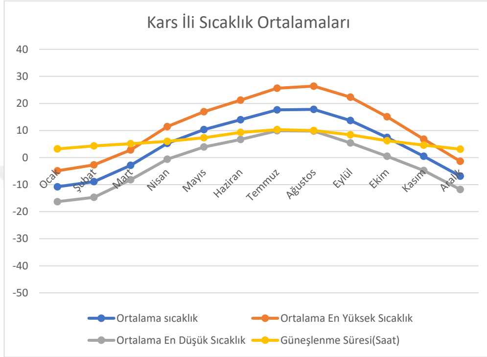
Şekil 2. 1 Kars ili Sıcaklık Ortalamaları ( Ölçüm Periyodu 1931-2022)
