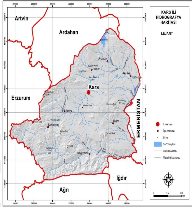
Harita 2.2. Kars İli Hidrografya Haritası
