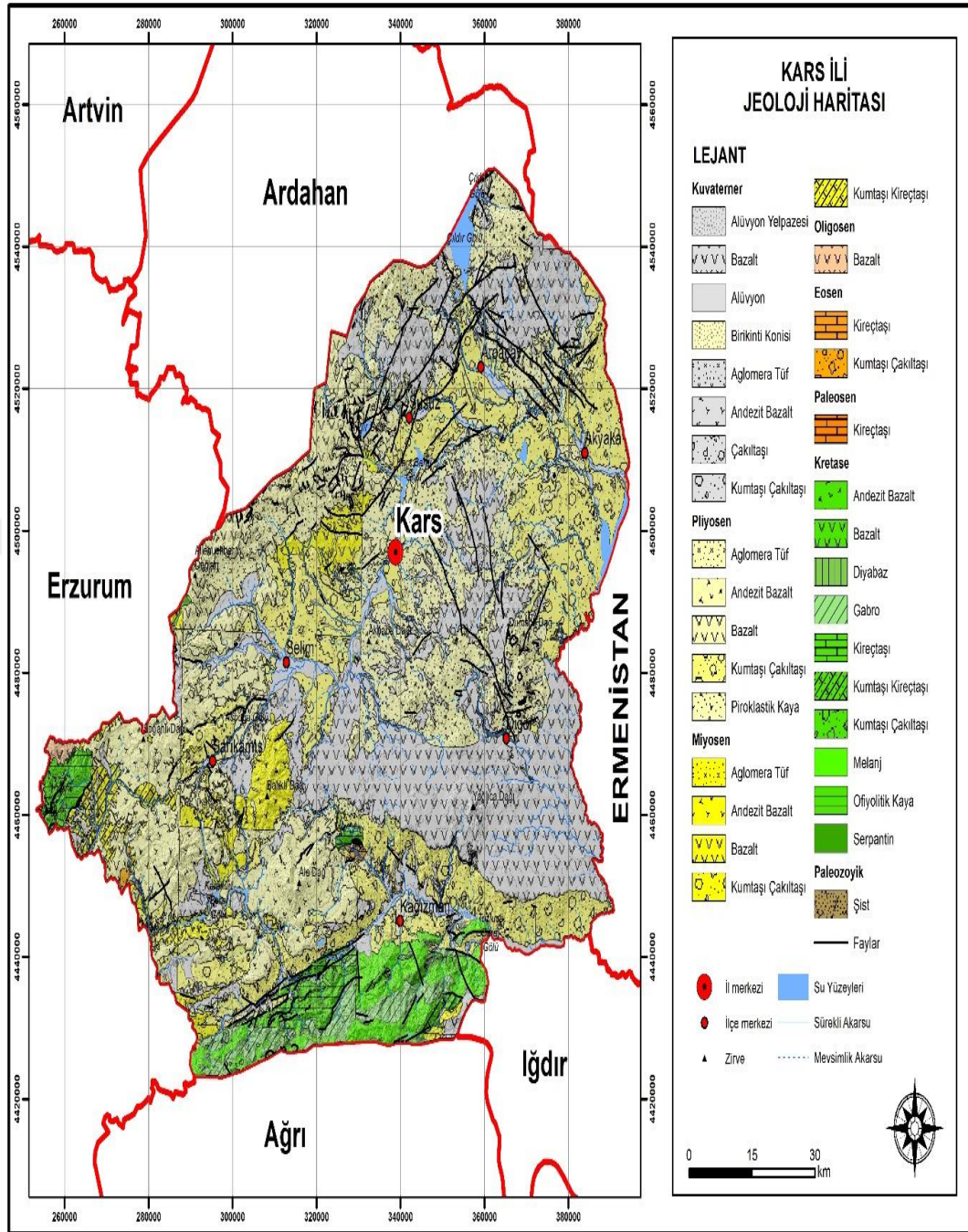
Harita 2.1. Kars İli Jeoloji Haritası
