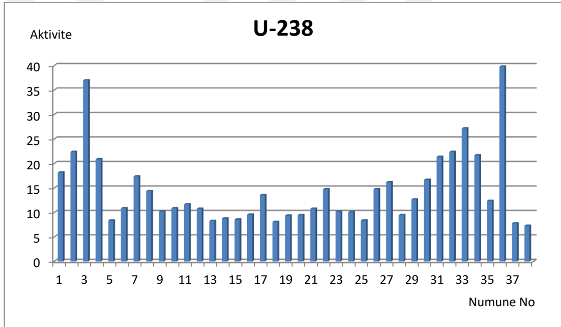
Grafik 4. Cide ilçesi numunelerindeki ^{238}\text{U} aktivite konsantrasyonları
