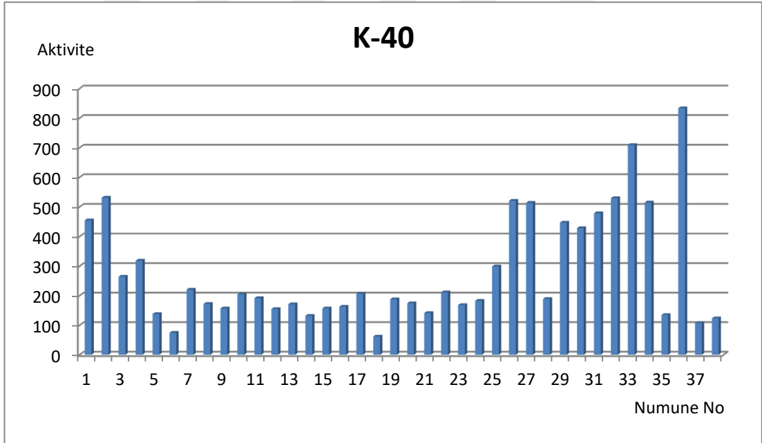
Grafik 6. Cide ilçesi numunelerindeki ^{40}\text{K} aktivite konsantrasyonları
