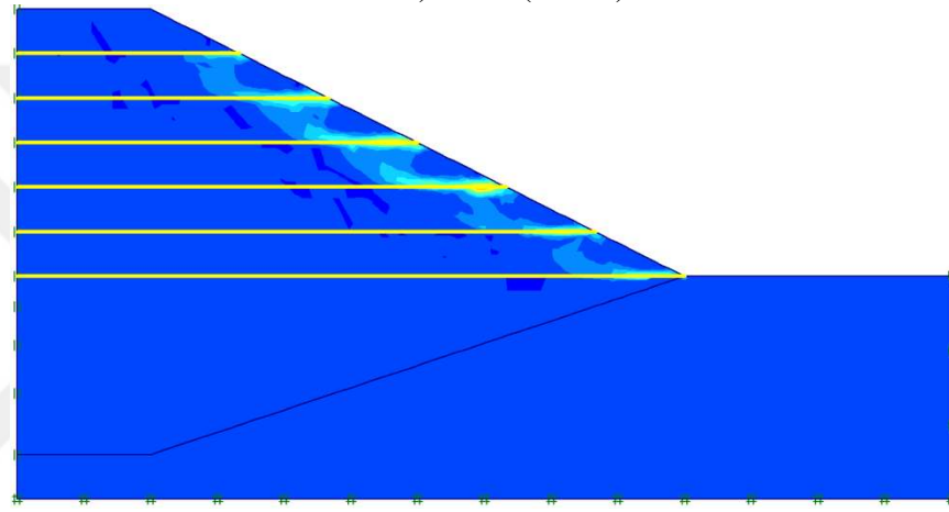
c) N=6 (h=5m.)
