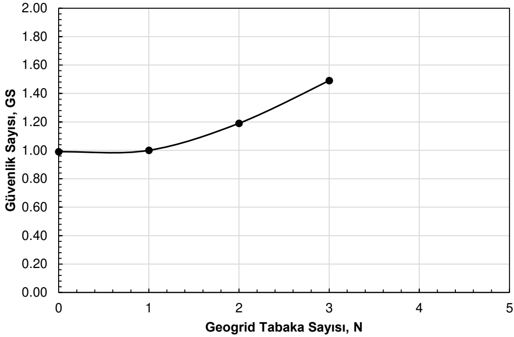
Şekil 4.31. Geogrid sayısı (N) - Güvenlik Sayısı (GS) Eğrisi ( h=10 m. )
