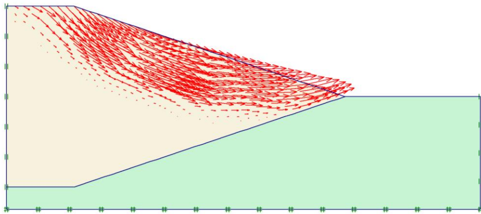
a) Deformasyona Uğramış Sonlu Elemanlar Ağı ( \phi=15^\circ )
