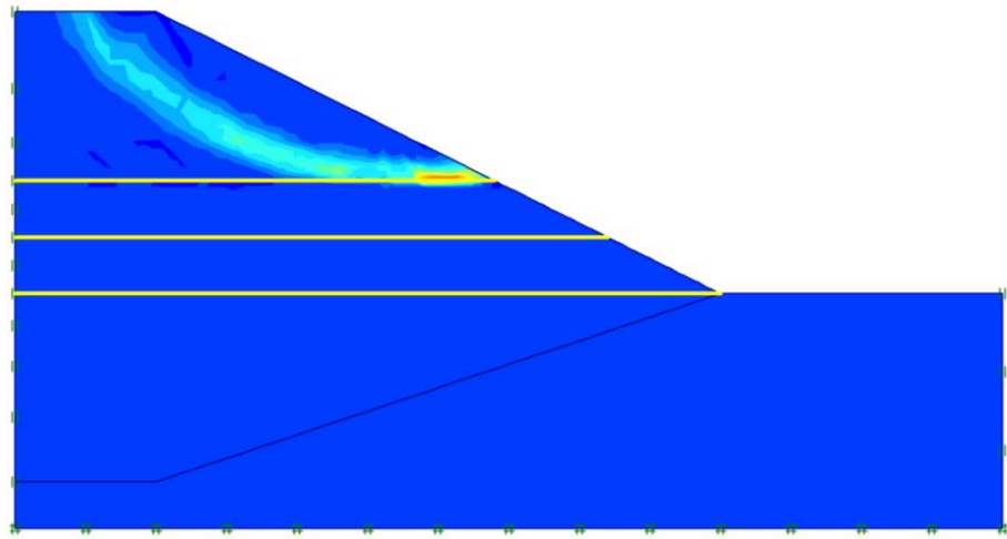
b) N=3 (h=6 m.)
