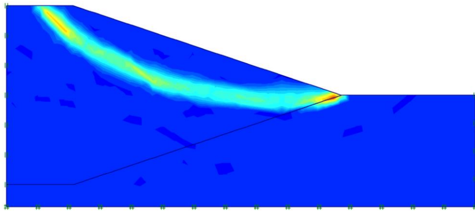
c) \phi=35^\circ
