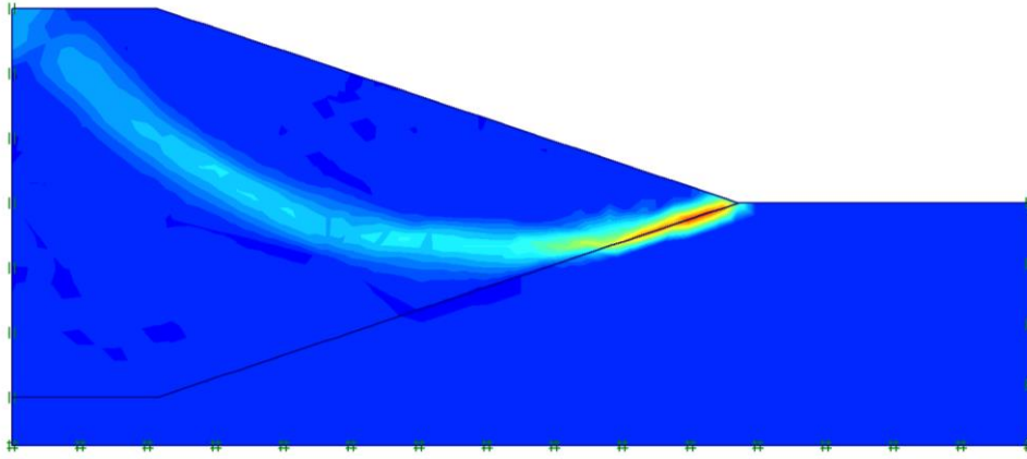
a) \phi=5^\circ
