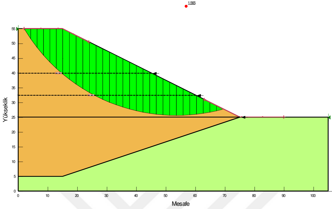
c) N=3 ( h=7.5 m.)
