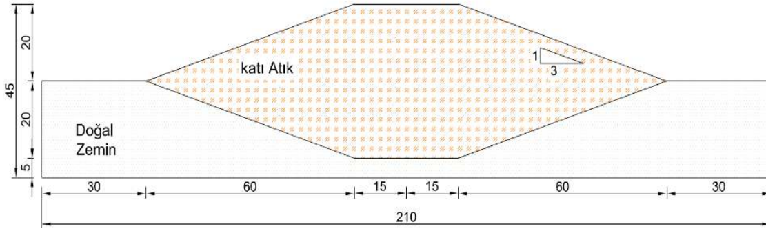
Şekil 4.1. Analizlerde Kullanılan Katı Atık Sahası Geometrisi (ölçüler metre cinsindendir.)
