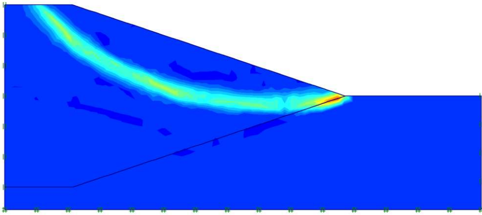
b) \phi=20^\circ
