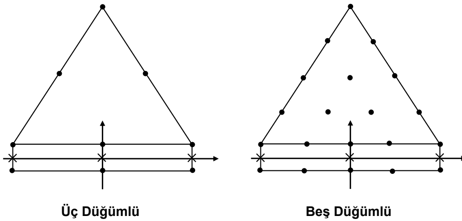
Şekil 3.7. Ara Yüzey Elemanlarının Sisteme Bağlantı Şekli
