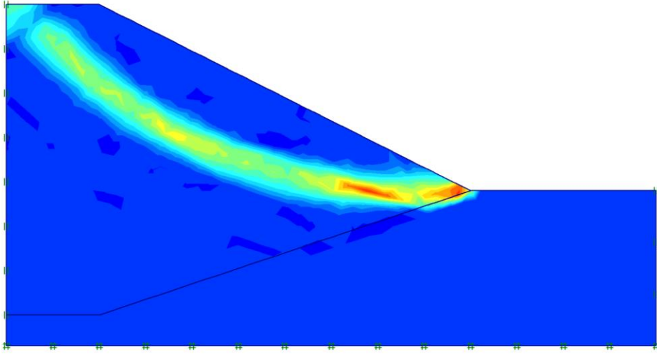
a) Donatısız
