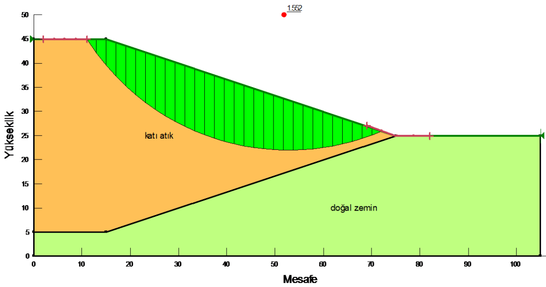
a) \gamma=9 kN/m³
