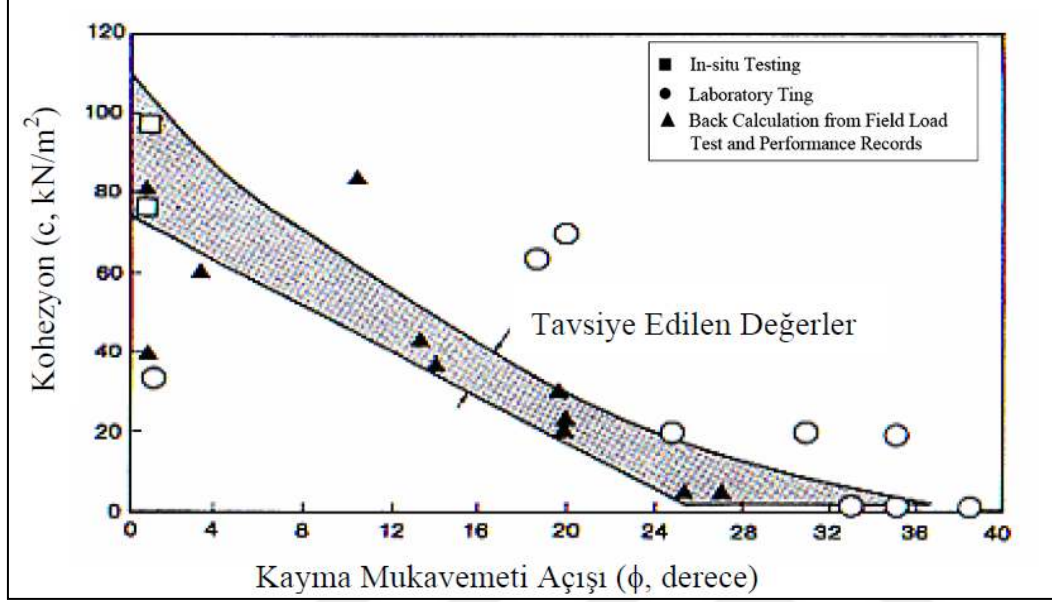
Şekil 2.1. Katı Atıklar İçin Singh ve Murphy’nin Önerdiği Sürtünme Açısı-Kohezyon Diyagramı
