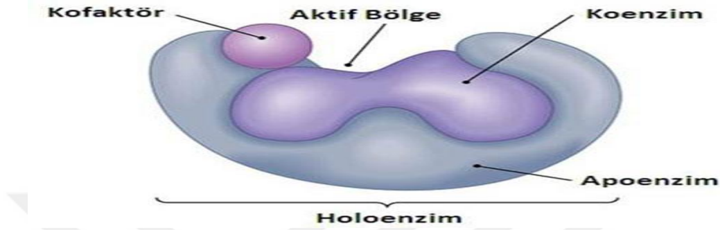
Şekil 2.5 Bir enzimin yapısı [26]
