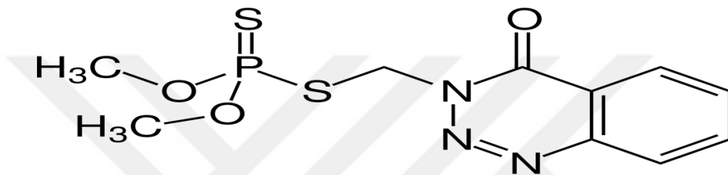
Şekil 2.2 Azinphos-methyl'in molekül yapısı [15]
