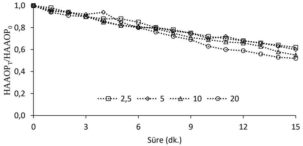
Şekil 4.24: Başlangıç kirletici dozuna bağlı olarak HAAOP azalımı ([DKP]=0.050 g/L, [O 3 ]=10 mg/L, pH=6.8±0.4, n=600 rpm).
