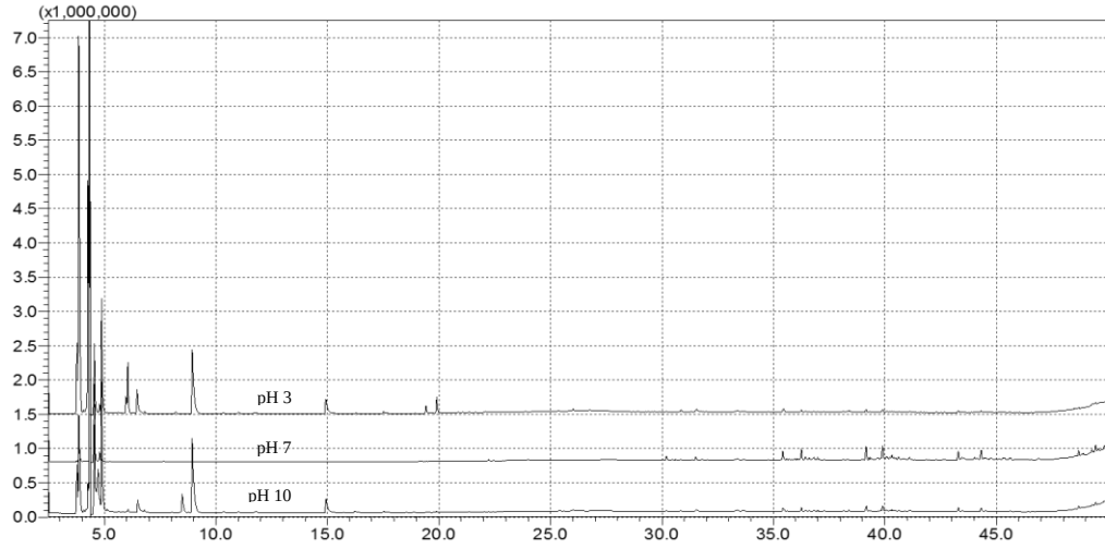
Şekil 4.37: Başlangıç pH'ına bağlı olarak ozonlama yan ürünlerinin değişimi.
