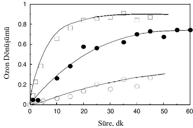
Şekil 2.30: Farklı pH'larda tamponlanmış saf suda ozon bozunması (Şartlar: 17°C, fosfatla tamponlanmış; ■=pH 2, C_{O_3} =8.1 mg/L; •=pH 7, C_{O_3} =4.2 mg/L; o=pH 8.5, C_{O_3} =3.7 mg/L).
