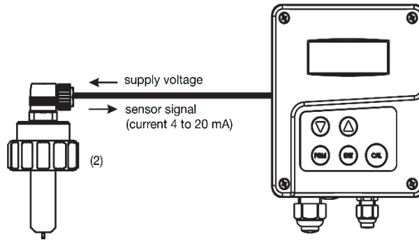
Şekil 3.1: Jumo Aquis 500 ozon analizörünün şematik görünümü.
