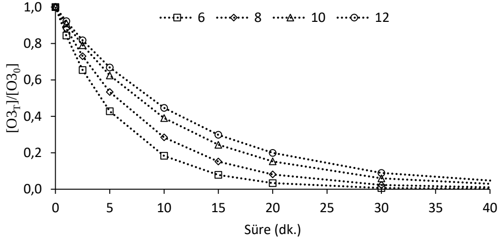
Şekil 4.11: Tekil ozonlamanın ozon dekompozisyonuna etkisi ([HA]=10 mg/L, pH=6.8±0.4).
