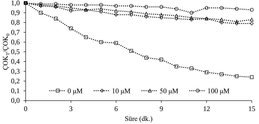
Şekil 4.29: Katalitik ozonlama performansı üzerine fosfat etkisi.
