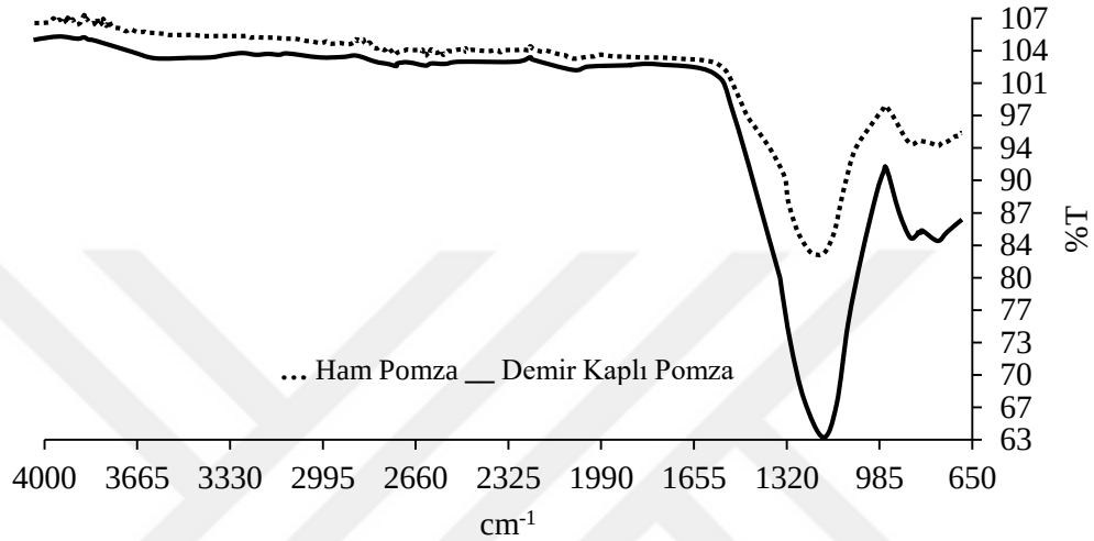
Şekil 4.3: Ham pomza ve demir kaplı pomza örneklerinin FT-IR spektrumu.
