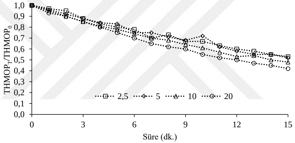
Şekil 4.23: Başlangıç kirletici dozuna bağlı olarak THMOP azalımı ([DKP]=0.050 g/L, [O 3 ]=10 mg/L, pH=6.8±0.4, n=600 rpm).
