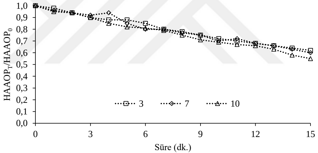
Şekil 4.28: Başlangıç pH değerlerine bağlı olarak HAAOP azalımı ([DKP]=0.050 g/L, [O 3 ]=10 mg/L, [HA]=10 mg/L, n=600 rpm).
