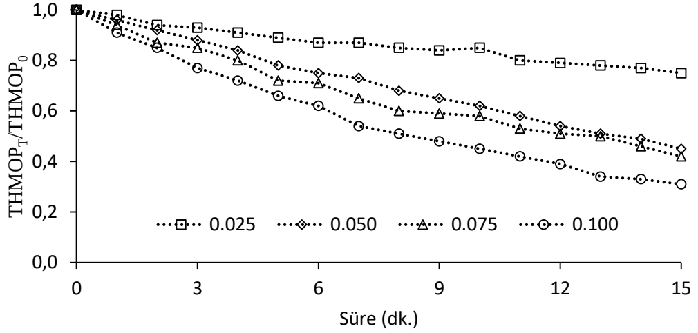
Şekil 4.15: Katalizör dozuna bağlı olarak THMOP azalımı ( [O_3]=10 mg/L, [HA]=10 mg/L, pH=6.8\pm0.4 , n=600 rpm).
