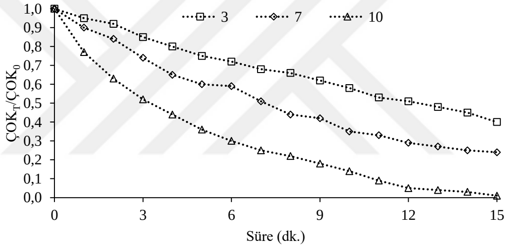
Şekil 4.26: Başlangıç pH değerlerine bağlı olarak ÇOK giderimi ([DKP]=0.050 g/L, [O 3 ]=10 mg/L, [HA]=10 mg/L, n=600 rpm).
