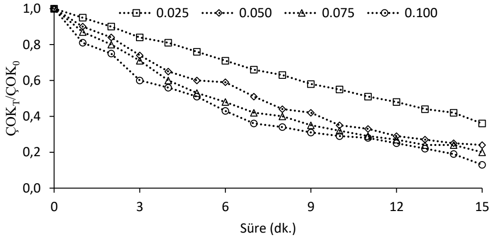
Şekil 4.14: Katalizör dozuna bağlı olarak ÇOK giderimi ( [O_3]=10 mg/L, [HA]=10 mg/L, pH=6.8\pm0.4 , n=600 rpm).
