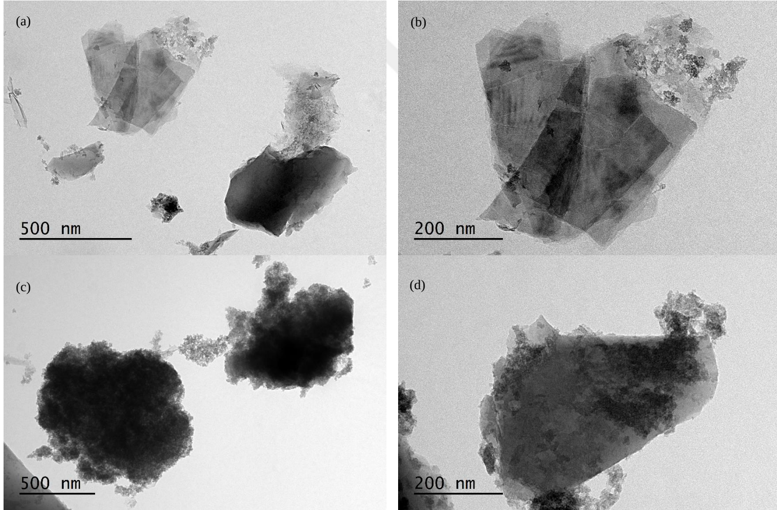
Şekil 4.4: Katalizörün TEM fotoğrafları; Ham Pomza (a,b) ve Demir Kaplı Pomza (c,d).
