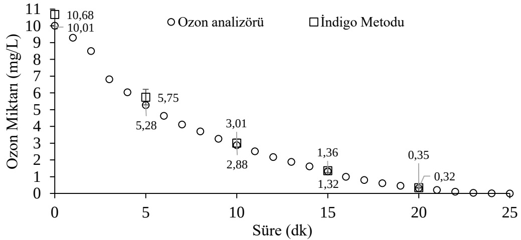
Şekil 3.3: Ozon analizi için metotların kıyaslanması.
