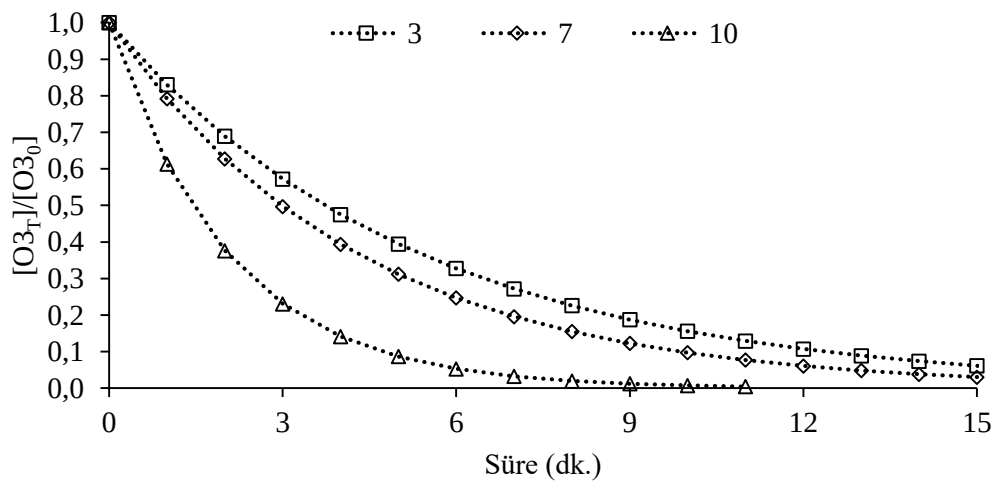
Şekil 4.25: Başlangıç pH değerlerine bağlı olarak ozonun dekompozisyonu ([DKP]=0.050 g/L, [O 3 ]=10 mg/L, [HA]=10 mg/L, n=600 rpm).
