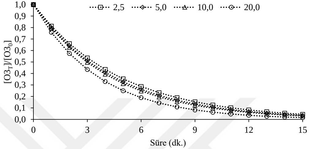
Şekil 4.21: Başlangıç kirletici dozuna bağlı olarak ozonun dekompozisyonu ([DKP]=0.050 g/L, [O 3 ]=10 mg/L, pH=6.8±0.4, n=600 rpm).
