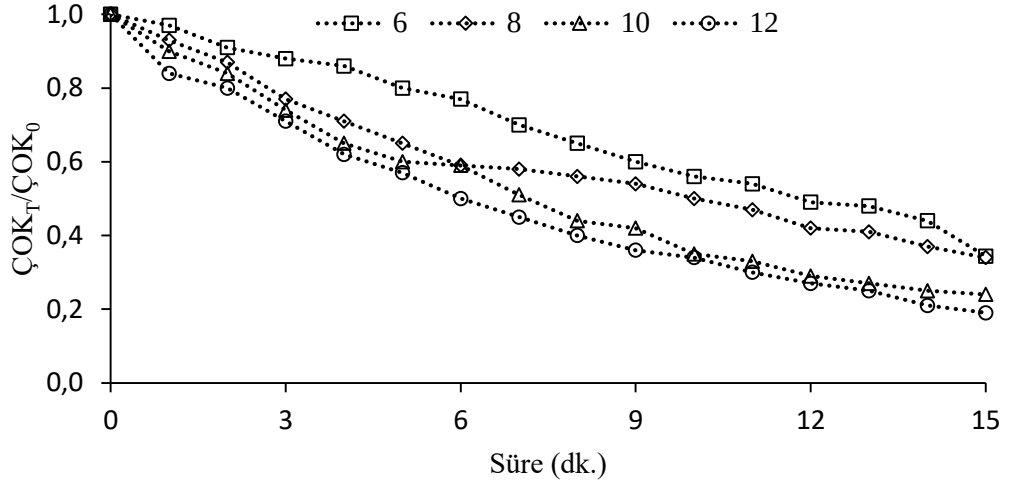
Şekil 4.18: Başlangıç ozon dozuna bağlı olarak ÇOK giderimi ([DKP]=0.050 g/L, [HA]=10 mg/L, pH=6.8±0.4, n=600 rpm).
