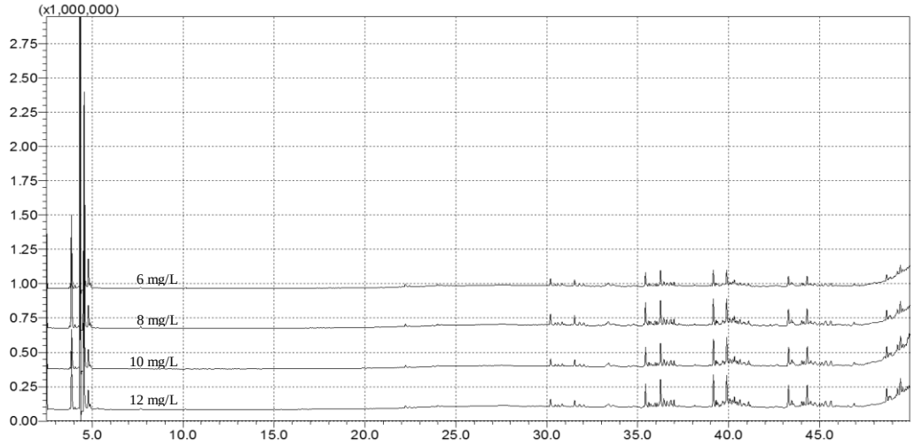
Şekil 4.35: Ozon dozuna bağlı olarak ozonlama yan ürünlerinin değişimi.
