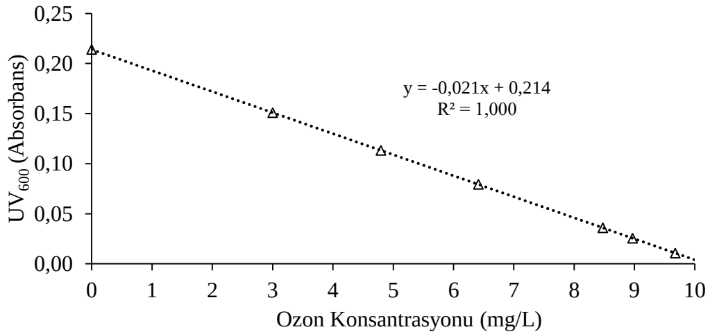
Şekil 3.2: Ozon kalibrasyon eğrisi.
