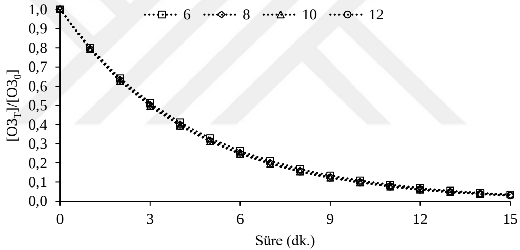
Şekil 4.17: Başlangıç ozon dozuna bağlı olarak ozonun dekompozisyonu ([DKP]=0.050 g/L, [HA]=10 mg/L, pH=6.8±0.4, n=600 rpm).
