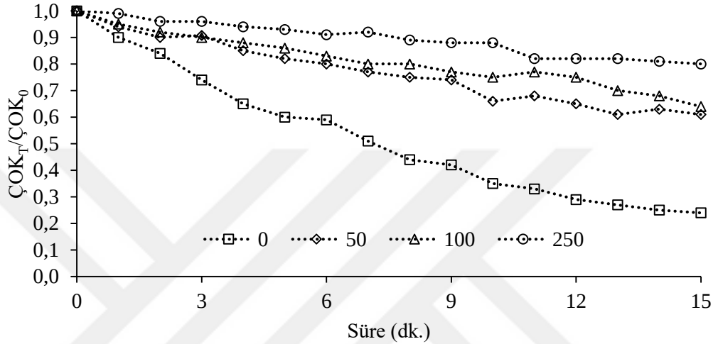
Şekil 4.31: TBA'nın katalitik ozonlama prosesi üzerine etkisi ([HA]= 10 mg/L, [Katalizör]= 0.050 g/L, [O 3 ]= 10 mg/L).
