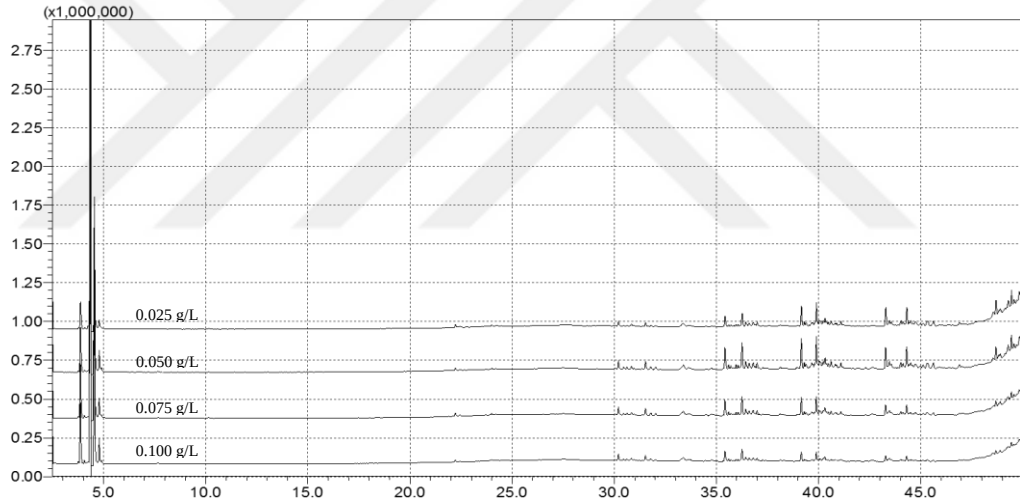
Şekil 4.34: Katalizör dozuna bağlı olarak ozonlama yan ürünlerinin değişimi.
