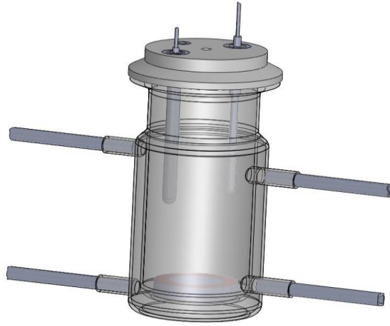
Şekil 3.4: Cam ozon reaktörü.
