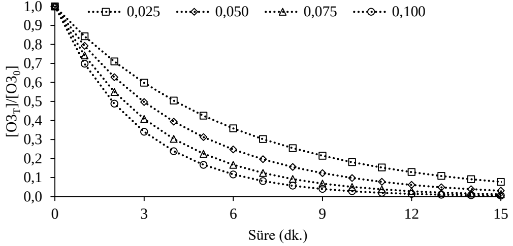
Şekil 4.13: Katalizör dozuna bağlı olarak ozonun dekompozisyonu ( [O_3]=10 mg/L, [HA]=10 mg/L, pH=6.8\pm0.4 , n=600 rpm).
