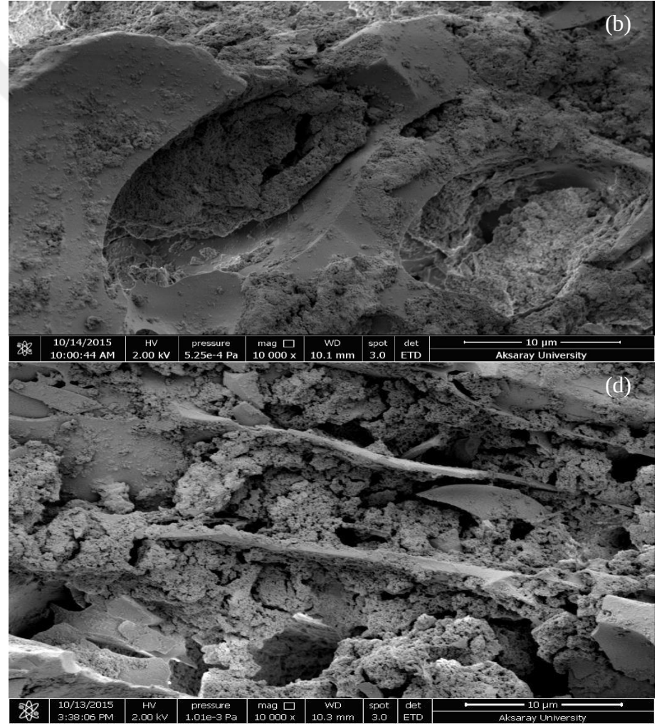
Şekil 4.10: DKP (a,b) ve hümk asit adsorplamış DKP'nin (c,d) karşılaştırılması.
