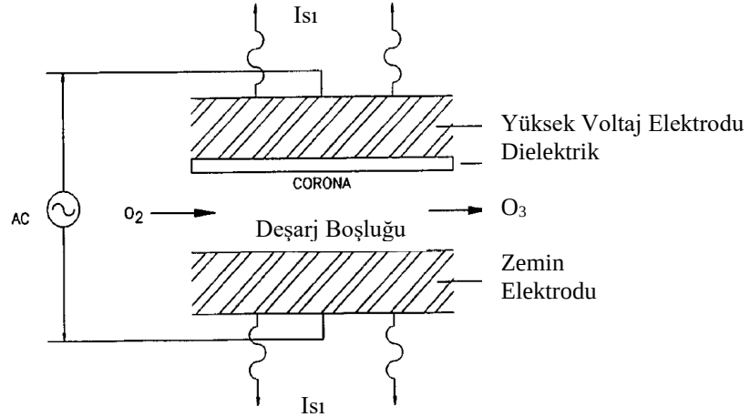
Şekil 2.22: Ozon jeneratörü.
