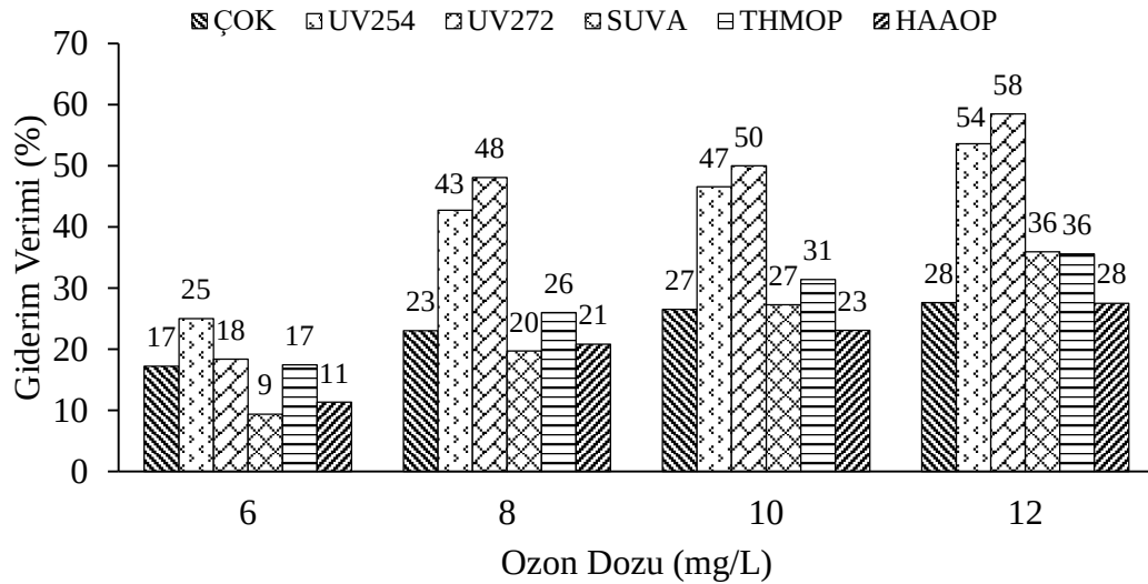
Şekil 4.12: Tekil ozonlamanın doğal organik madde giderimine etkisi ([HA]=10 mg/L, pH=6.8±0.4).
