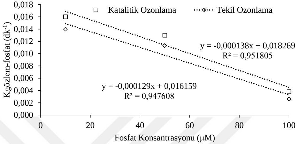
Şekil 4.30: Fosfat konsantrasyonu ve reaksiyon hız sabitlerinin lineer uyumu.
