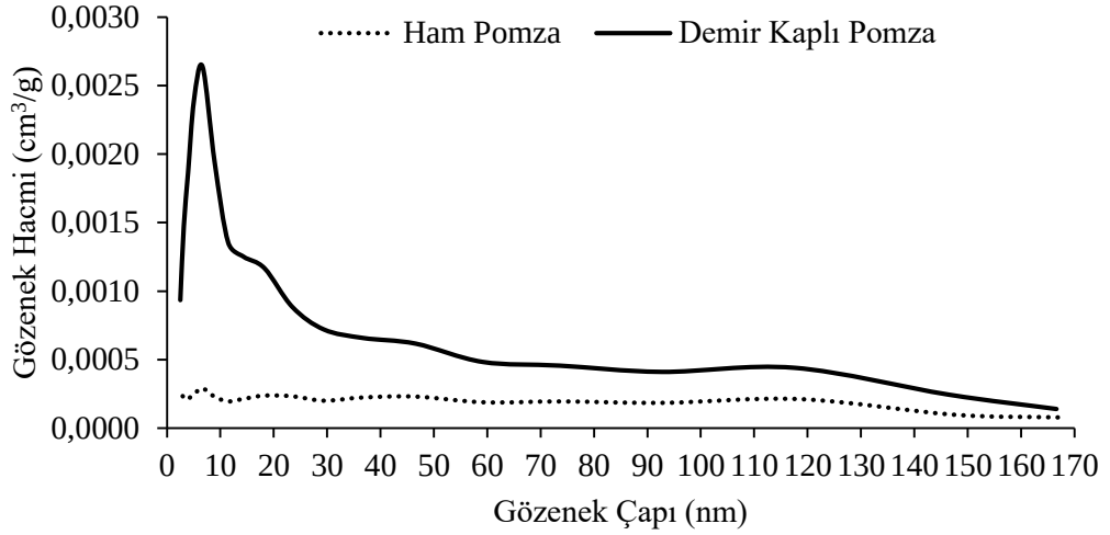
Şekil 4.5: Ham ve demir kaplı pomza örneklerinin gözenek çapı dağılımı.
