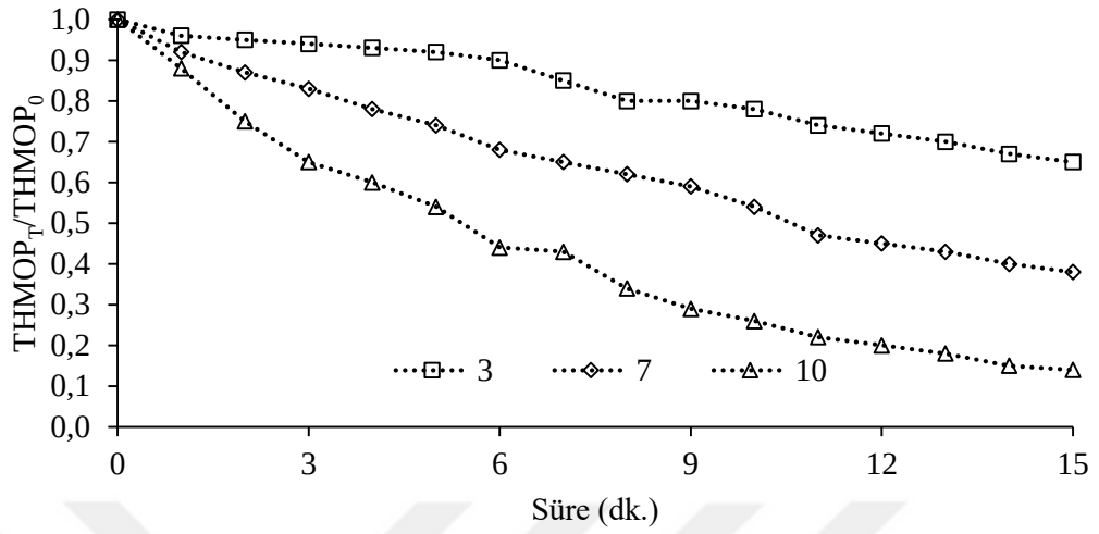
Şekil 4.27: Başlangıç pH değerlerine bağlı olarak THMOP azalımı ([DKP]=0.050 g/L, [O 3 ]=10 mg/L, [HA]=10 mg/L, n=600 rpm).
