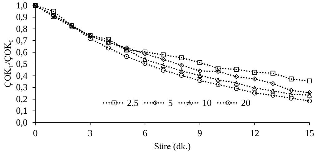
Şekil 4.22: Başlangıç kirletici dozuna bağlı olarak ÇOK giderimi ([DKP]=0.050 g/L, [O 3 ]=10 mg/L, pH=6.8±0.4, n=600 rpm).
