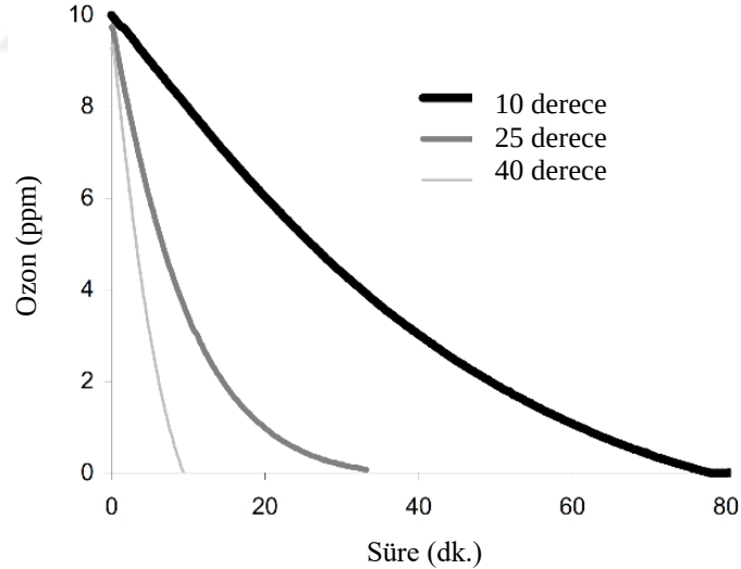
Şekil 2.32: Sıcaklık değişimine göre ozonun bozunma hızı.
