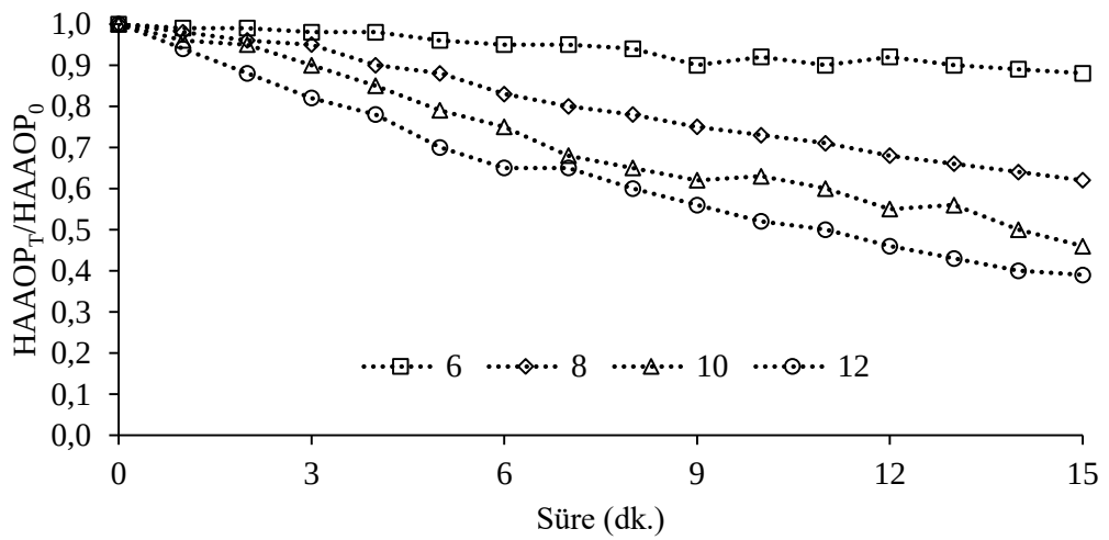
Şekil 4.20: Başlangıç ozon dozuna bağlı olarak HAAOP azalımı ([DKP]=0.050 g/L, [HA]=10 mg/L, pH=6.8±0.4, n=600 rpm).
