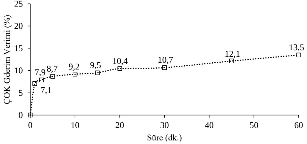
Şekil 4.8: DKP ile hümik asit adsorbsiyonunda ÇOK giderimi ([DKP]=0.050 g/L, [HA]=10 mg/L, pH=6.8±0.4, n=600 rpm).
