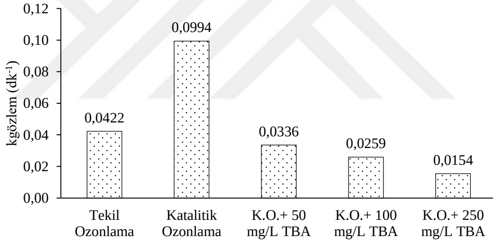
Şekil 4.32: TBA'nın katalitik ozonlama üzerine etkisine bağlı olarak reaksiyon hız sabitlerinin değişimi.
