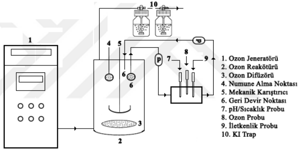
Şekil 3.5: Deney düzeneği.
