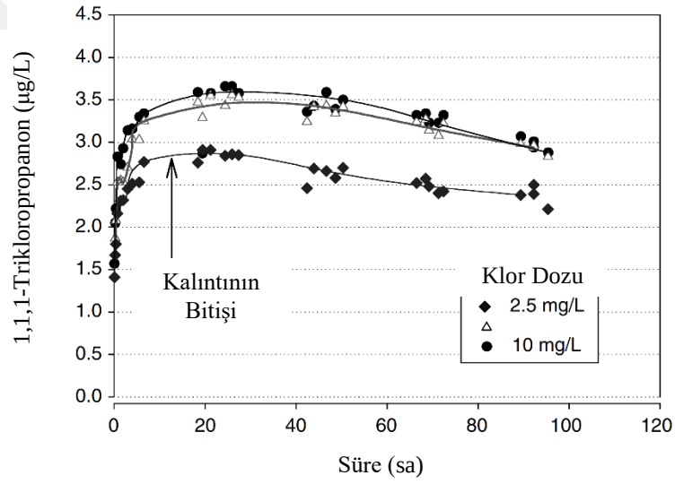
Şekil 2.16: Trikloropropanon oluşumuna reaksiyon süresinin etkisi.
