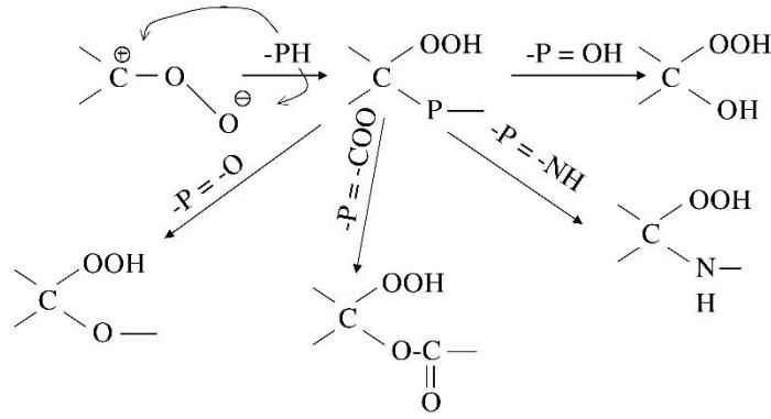
Şekil 2.25: Bir katılımcı çözücü içinde birincil ozonide ayrışma adımı.
