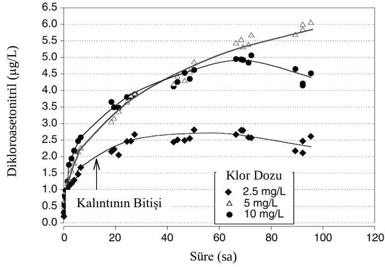
Şekil 2.14: Dikloroasetonitril oluşumuna klor dozu ve klorlama süresinin etkisi.
