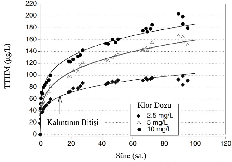
Şekil 2.13: Kloroform oluşumuna klor dozu ve klorlama süresinin etkisi.
