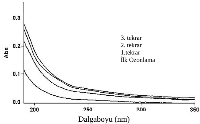
Şekil 2.37: Fosforik asit içerisinde yeniden ozonlamanın UV spektrofotometre analiz sonuçları.
