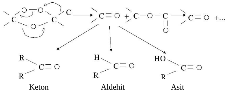
Şekil 2.26: Anormal ozon ayrışımı örneği.
