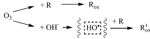
Şekil 2.33: Ozonun sulu çözeltilerde diğer bileşikler (R) ile davranışı.
