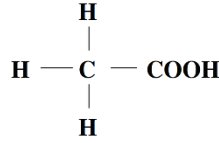
Şekil 2.3: Asetik asitin molekül yapısı.
