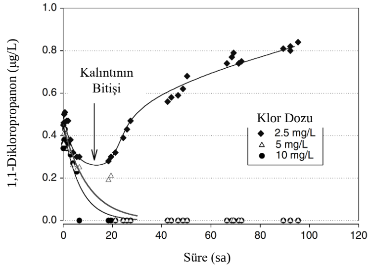
Şekil 2.15: Dikloropropanon oluşumuna klorlama süresinin etkisi.
