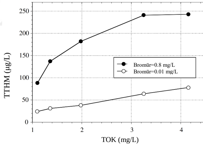
Şekil 2.10: THM oluşumu üzerine TOK'un etkisi.
