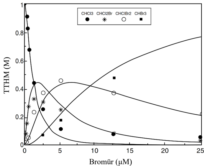
Şekil 2.18: Trihalometan oluşumuna bromürün etkileri.
