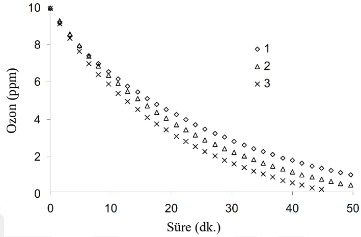
Şekil 2.36: Fosforik asit içerisinde ozonun dekompozisyonu.
