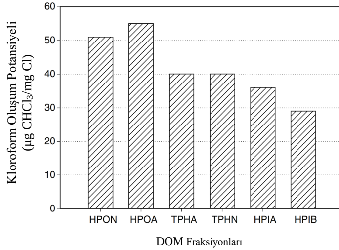
Şekil 2.11: Suwannee Nehri DOM fraksiyonlarının Kloroform oluşturma potansiyeli.
