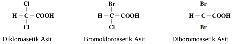
Şekil 2.5: Dihaloasetik asitlerin molekül yapıları.
