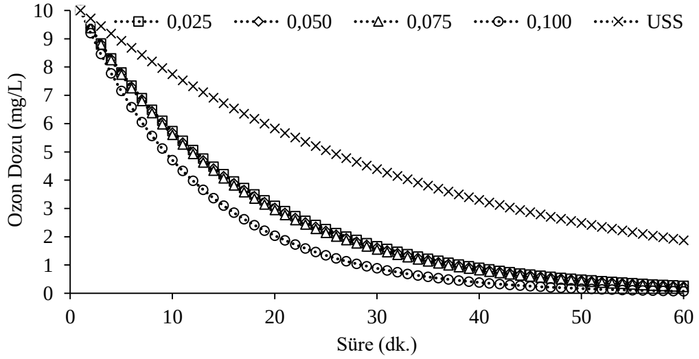
Şekil 4.7: Saf suda farklı demir kaplı pomza dozlarının ozonun bozunmasına etkisi ( [O_3]=10 mg/L, pH=6.8\pm0.4 , n=600 rpm).
