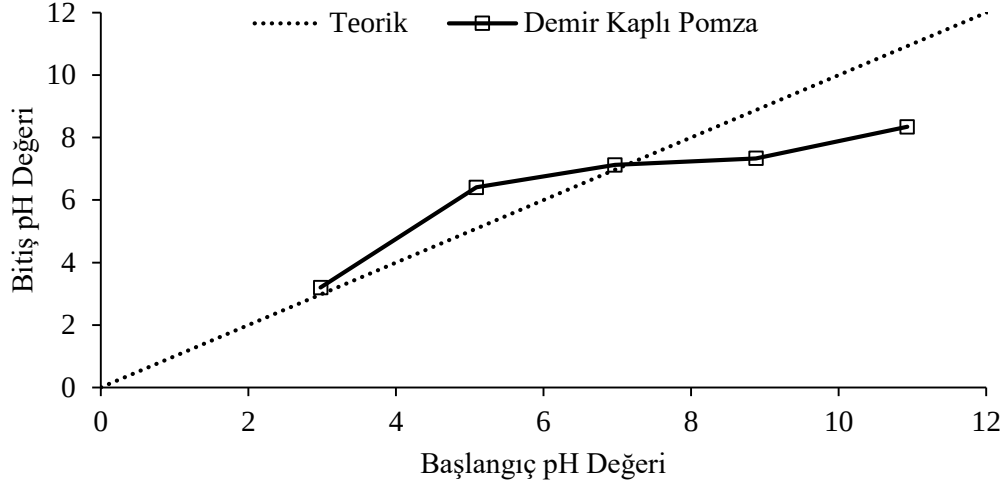
Şekil 4.6: Ham ve demir kaplı pomza örneklerinin pH PZC grafiği.
