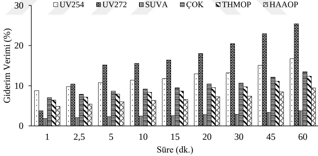
Şekil 4.9: DKP ile hümik asit adsorbsiyonu ([DKP]=0.050 g/L, [HA]=10 mg/L, pH=6.8±0.4, n=600 rpm).
