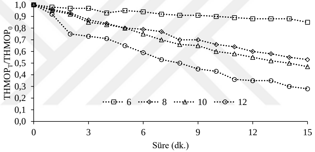
Şekil 4.19: Başlangıç ozon dozuna bağlı olarak THMOP azalımı ([DKP]=0.050 g/L, [HA]=10 mg/L, pH=6.8±0.4, n=600 rpm).
