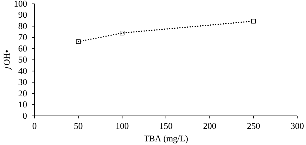
Şekil 4.33: TBA'nın hidroksil radikali fraksiyonuna etkisi.
