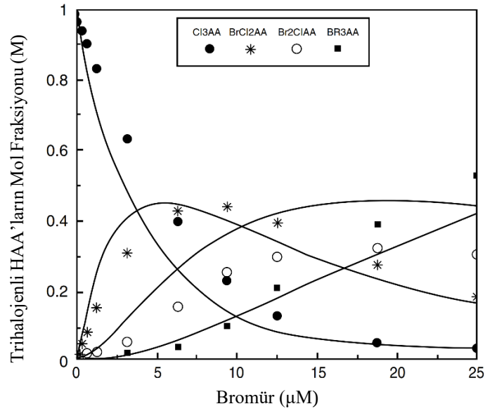
Şekil 2.19: Trihaloasetik asit oluşumuna bromürün etkileri.
