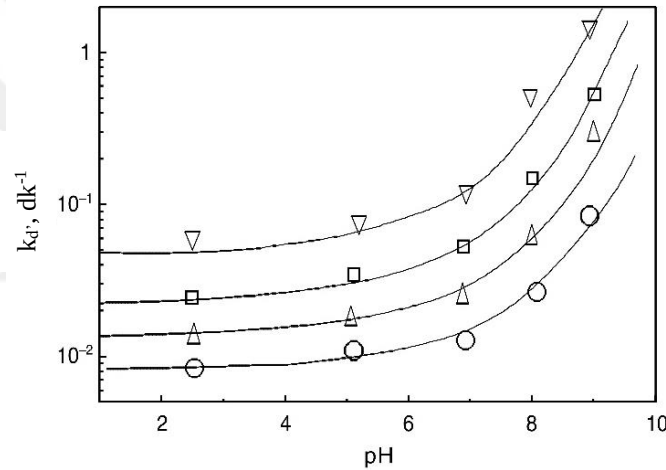
Şekil 2.31: pH'ı tamponlanmış saf su içinde ozon bozunumu için yalancı birinci dereceden hız sabiti değişimi (T, °C: •=10; ▲=20; ■=30; ▼=40).
