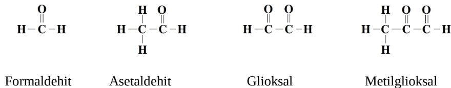
Şekil 2.7: Bilinen aldehytlerin moleküler yapıları.
