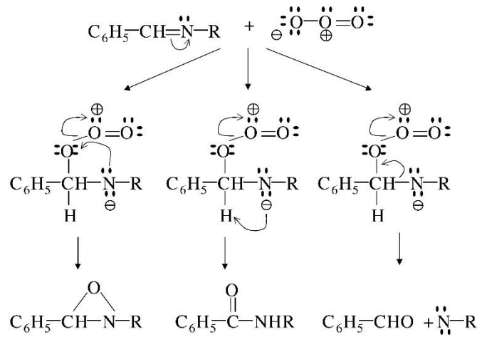
Şekil 2.29: Ozon nükleofilik değişim reaksiyonu.
