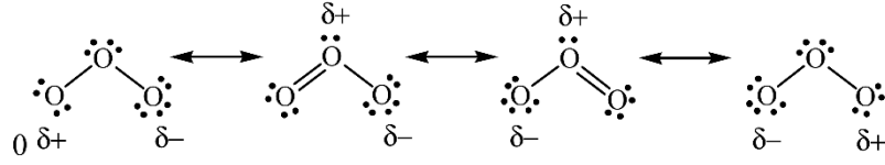
Şekil 2.21: Ozonun rezonans yapısı
