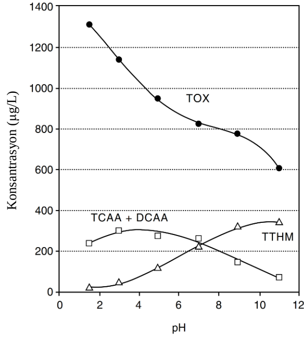
Şekil 2.17: pH'a bağlı olarak klorlama yan ürünlerinin oluşumu.
