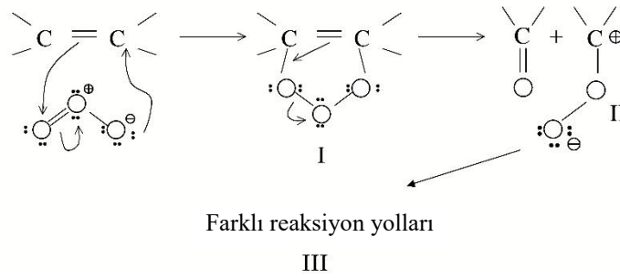
Şekil 2.23: Criegee mekanizması.
