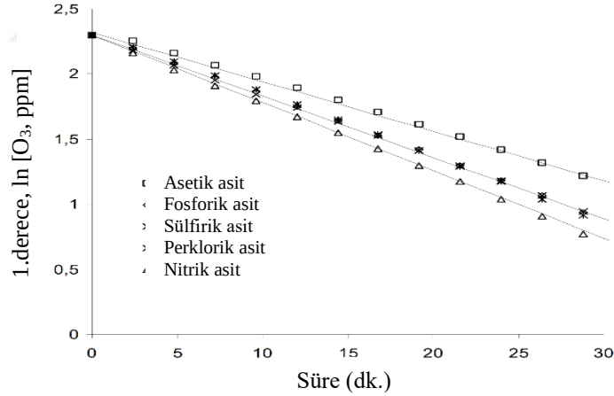
Şekil 2.35: Ozon dekompozisyonunun reaksiyon kinetiği (pH=3, t=25 °C).
