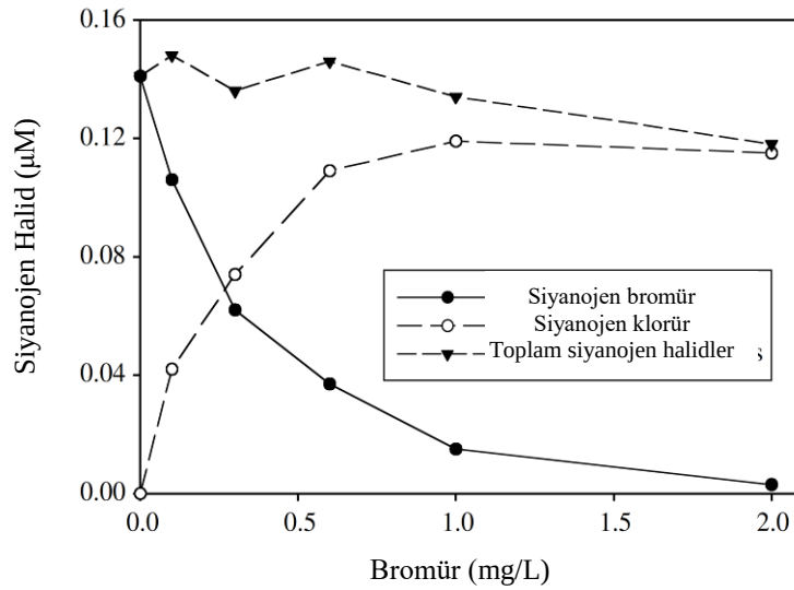
Şekil 2.20: Siyanojen halidlerin oluşumuna bromürün etkileri.
