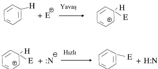
Şekil 2.27: Aromatik elektrofilik değiştirme reaksiyonunun temel adımları.
