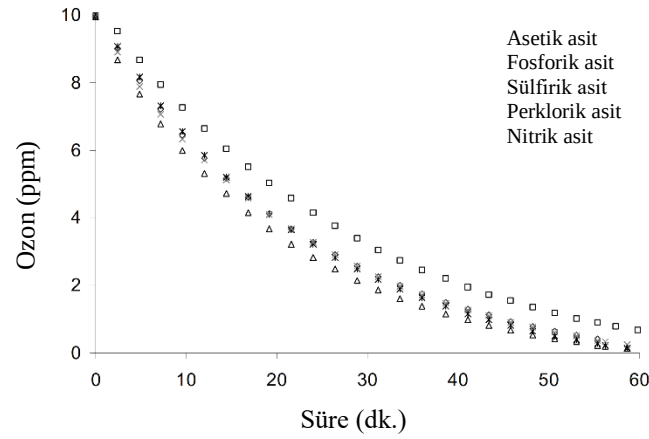
Şekil 2.34: 1 mM asetik, fosforik, sülfürik, perklorik ve nitrik asit ile pH 3 değerinde ozonun dekompozisyon hızı.
