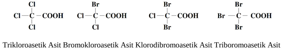
Şekil 2.6: Trihaloasetik asitlerin molekül yapıları.
