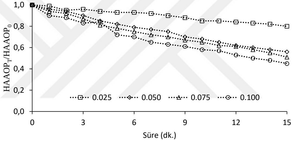
Şekil 4.16: Katalizör dozuna bağlı olarak HAAOP azalımı ( [O_3]=10 mg/L, [HA]=10 mg/L, pH=6.8\pm0.4 , n=600 rpm).
