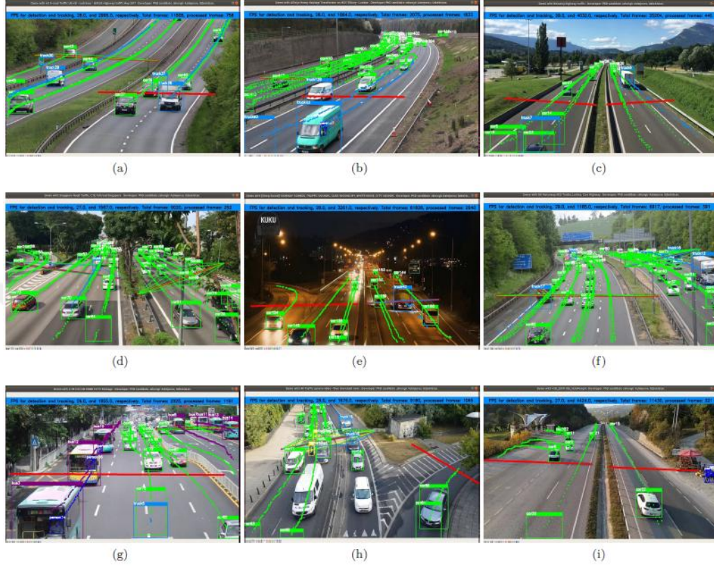
Şekil 4.4. Araçların, araç takip verilerinden çıkarılan yörüngeleri.
