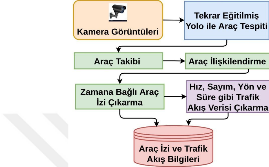
Şekil 1.1. Trafik Akış İzleme Sisteminin Genel Mimarisi.
