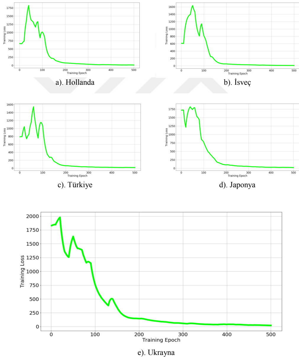
Şekil 4.1. Örnek kavşaklar için geliştirilen araç algılama modellerinin eğitim sürecine ait hata fonksiyonunun değeri ve devir sayısı arasındaki bağlantı grafiği.
