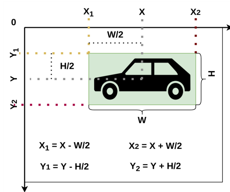
Şekil 3.12. YOLOv3 sınırlayıcı kutu değerlerinin koordinatlara dönüşümü.
