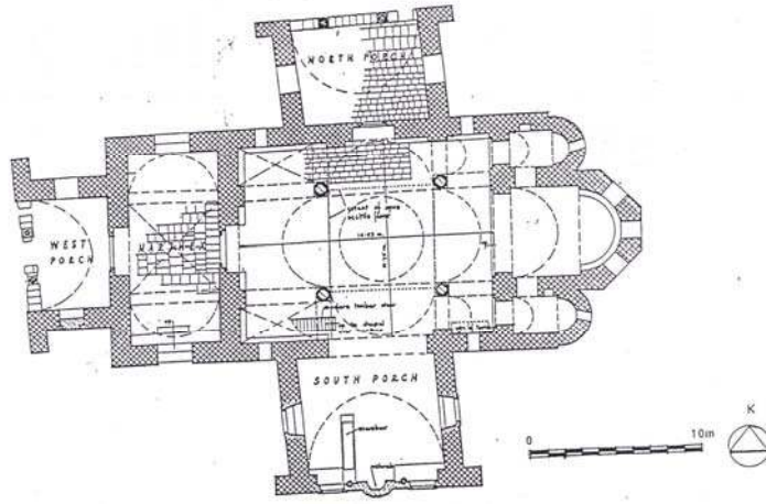
Şekil 6.110. Trabzon Ayasofya Kilisesi plan [24]
