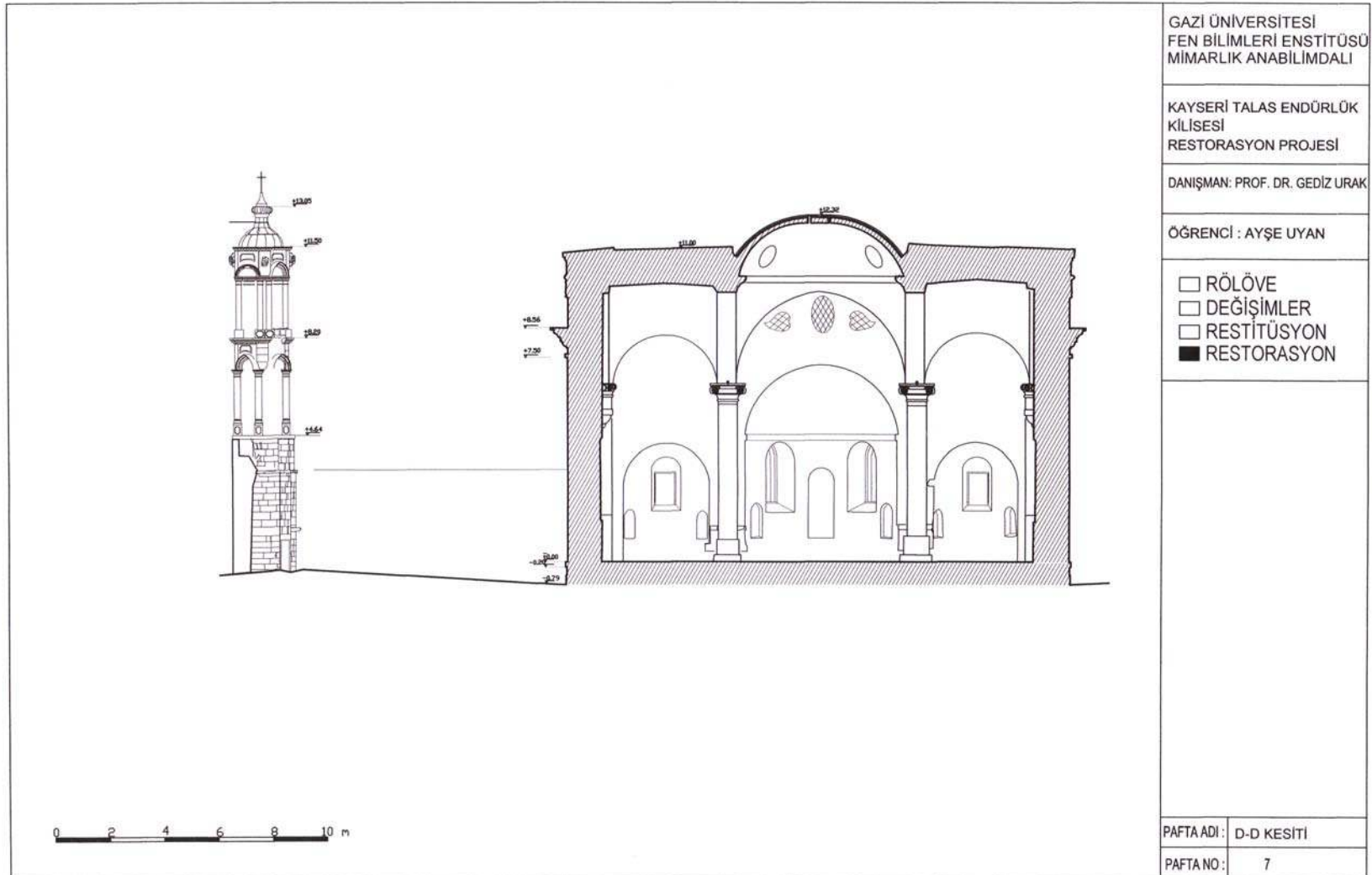
EK-67 Restorasyon D-D kesiti
