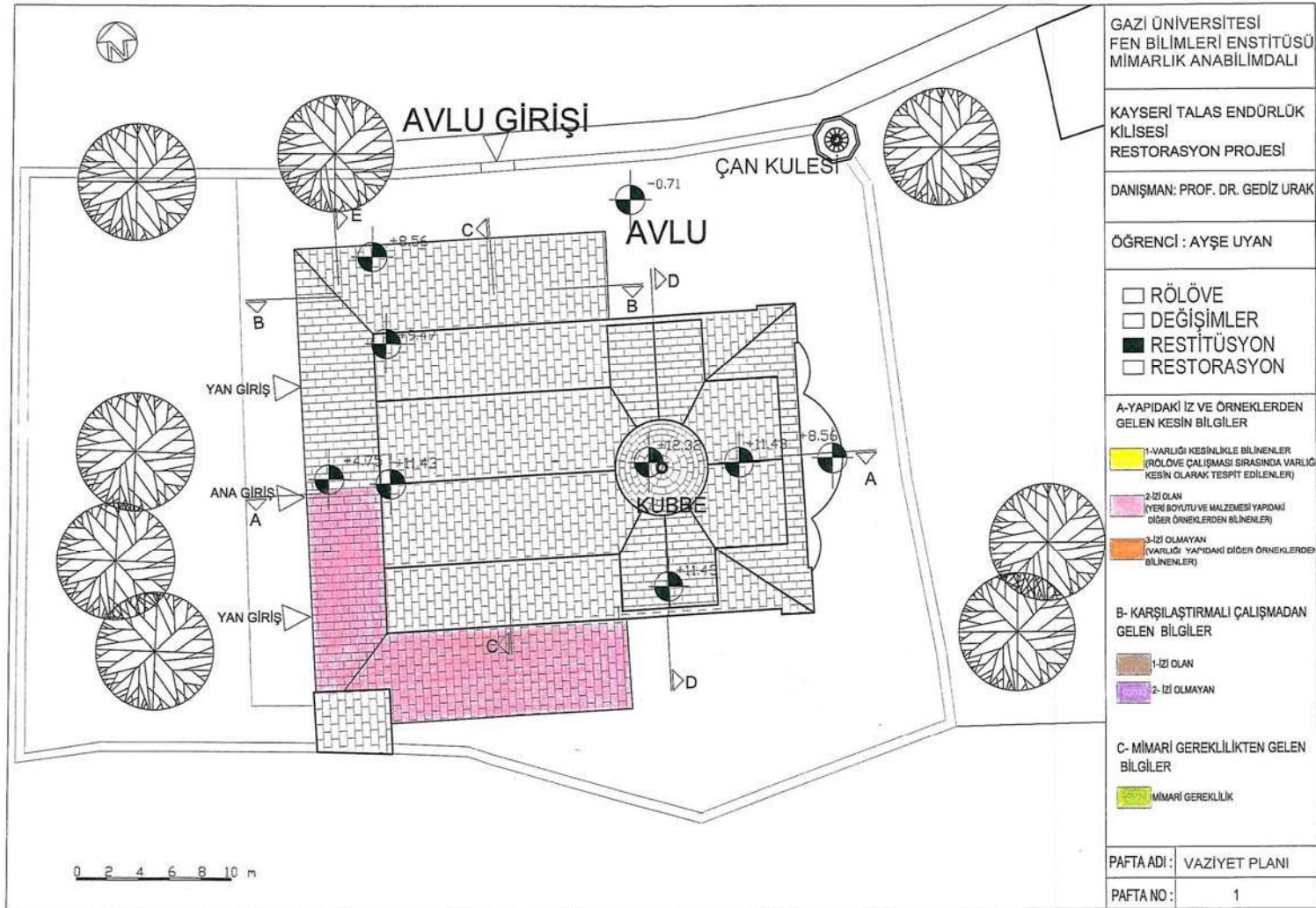
EK-37 Restitüsyon kaynak kullanım paftası vaziyet planı
