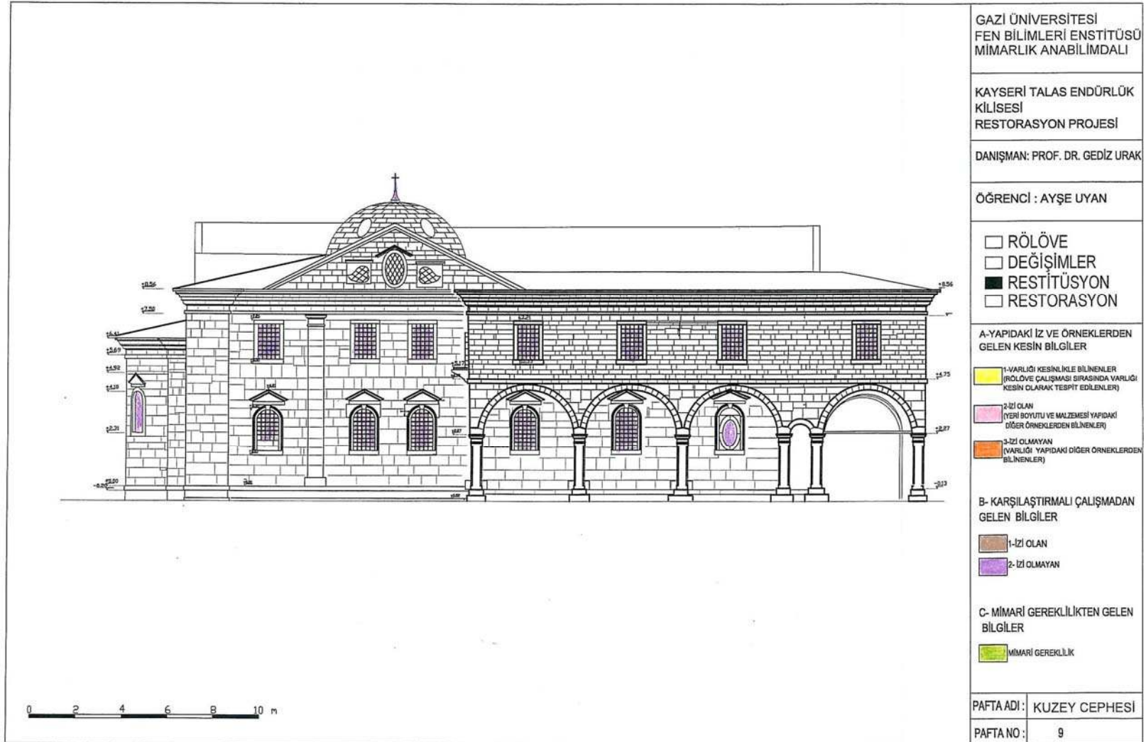
EK-45 Restitüsyon kaynak kullanım paftası kuzey cephesi
