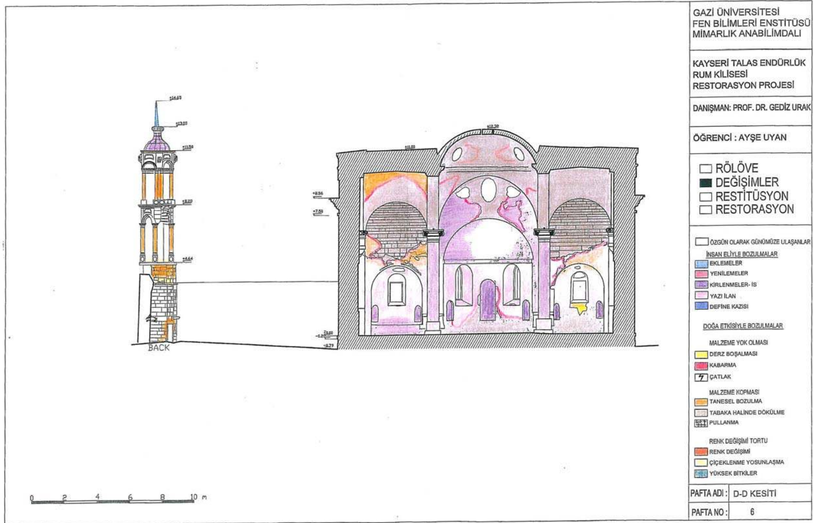
EK-24 Değişim ve bozulmalar D-D kesiti
