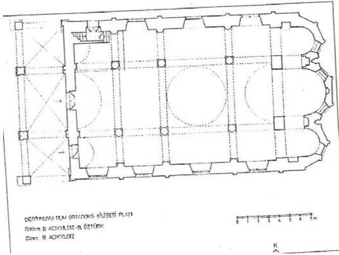
Şekil 6.88. Aziz Theodoros Kilisesi Plan
