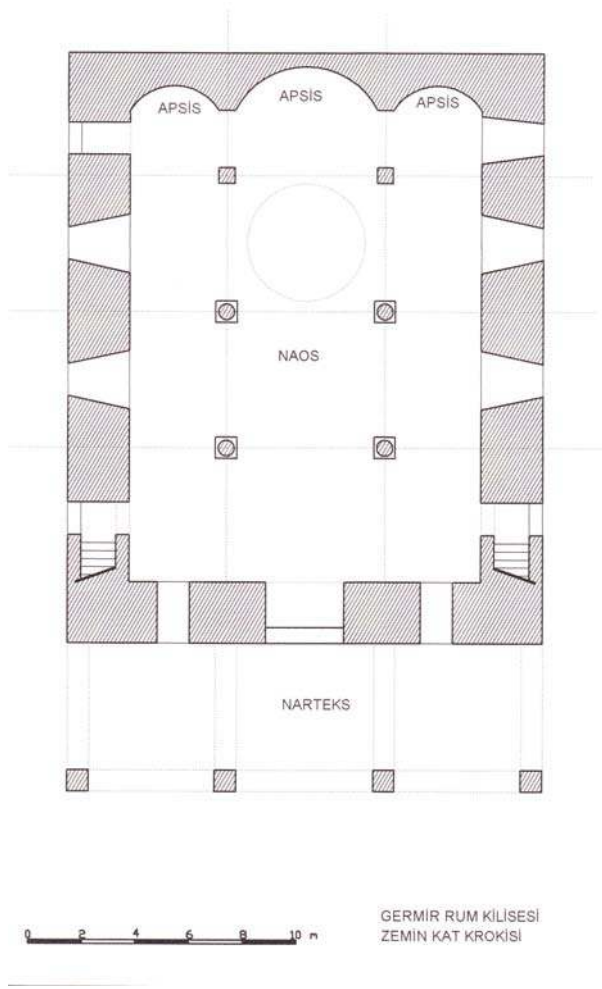
Şekil 6.10. Germir Kilisesi zemin kat planı
