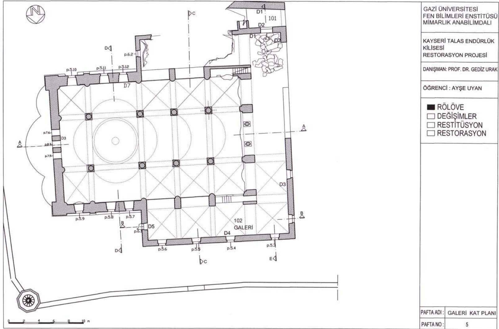
EK-5 Rölöve galeri kat planı
