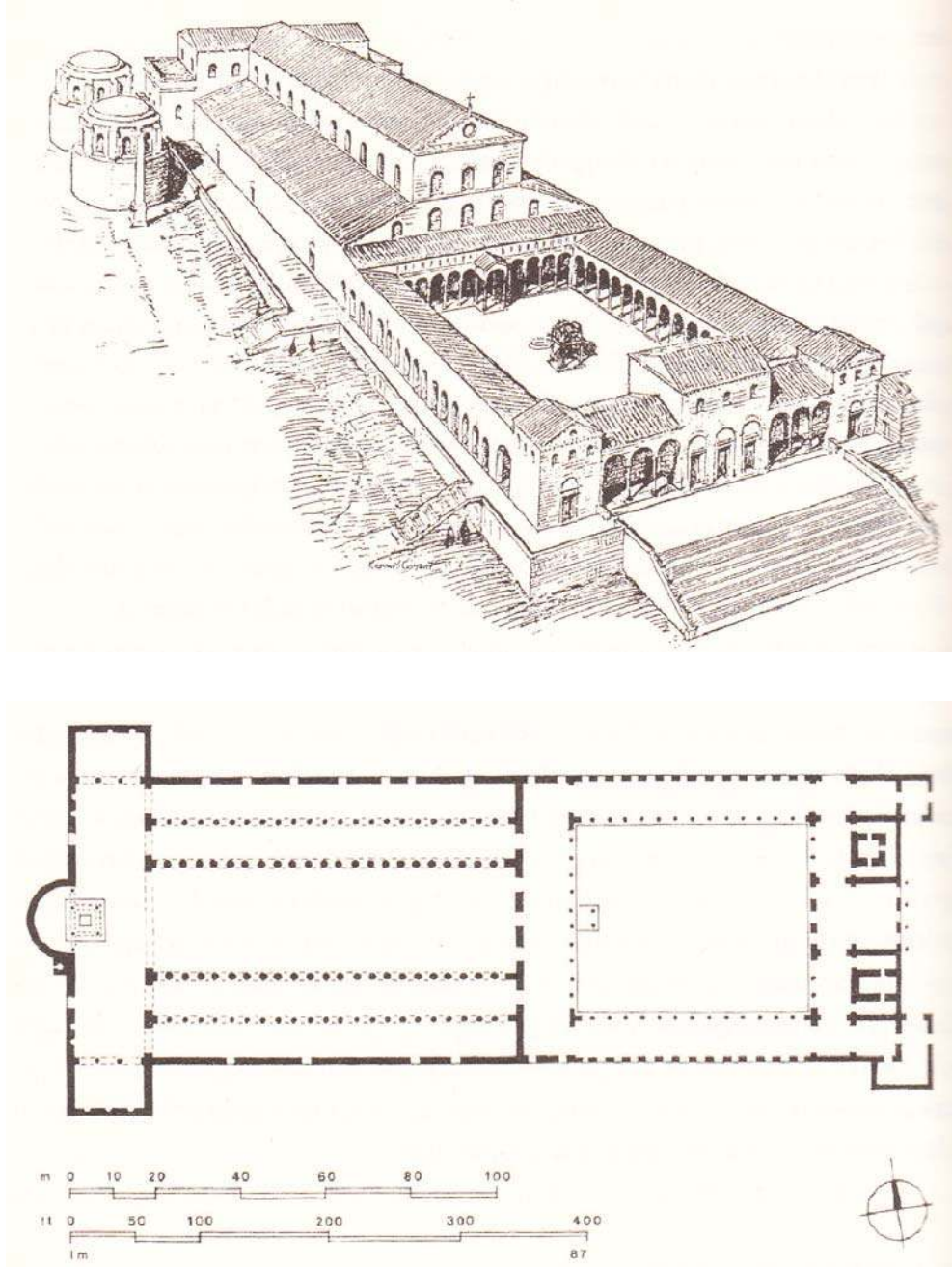
Şekil 3.2. Saint Peter Bazilikası, Roma 319-329 yılları arası [8]
