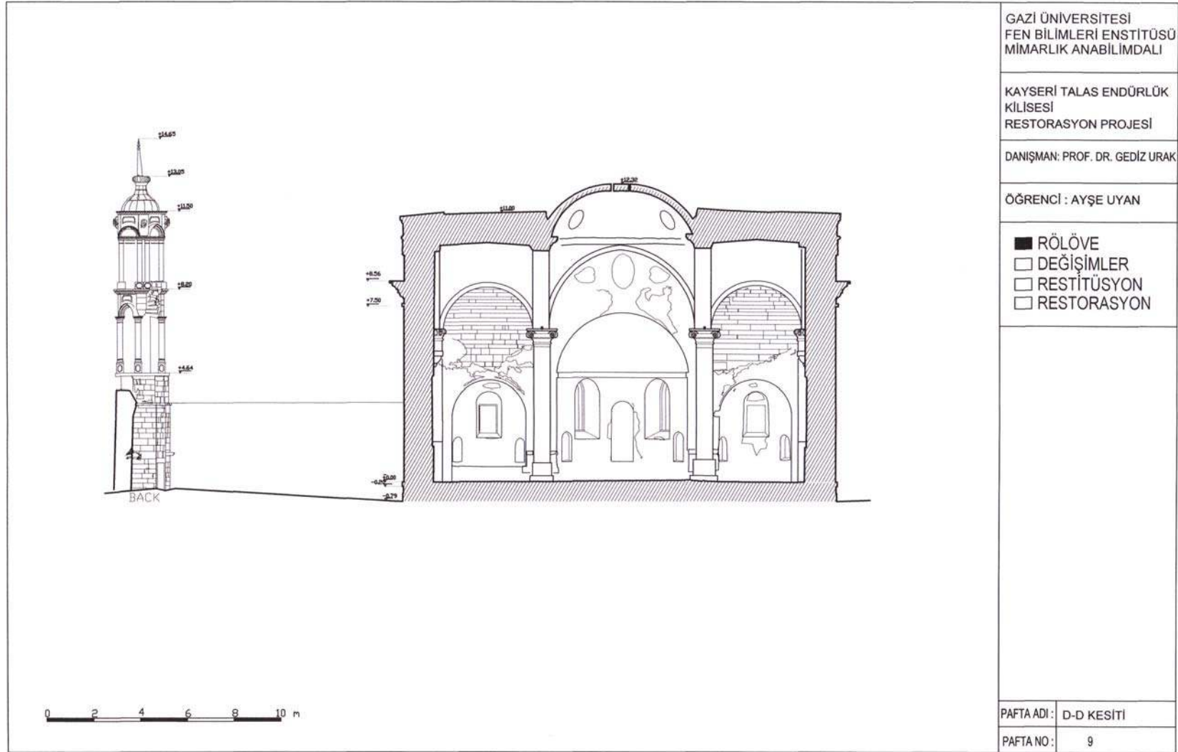
EK-9 Rölöve D-D kesiti
