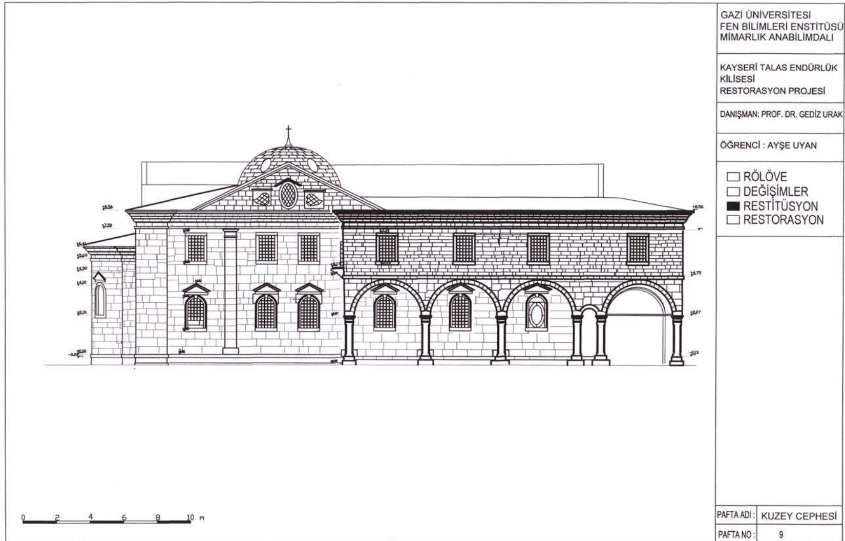
EK-57 Restitüsyon kuzey cephesi
