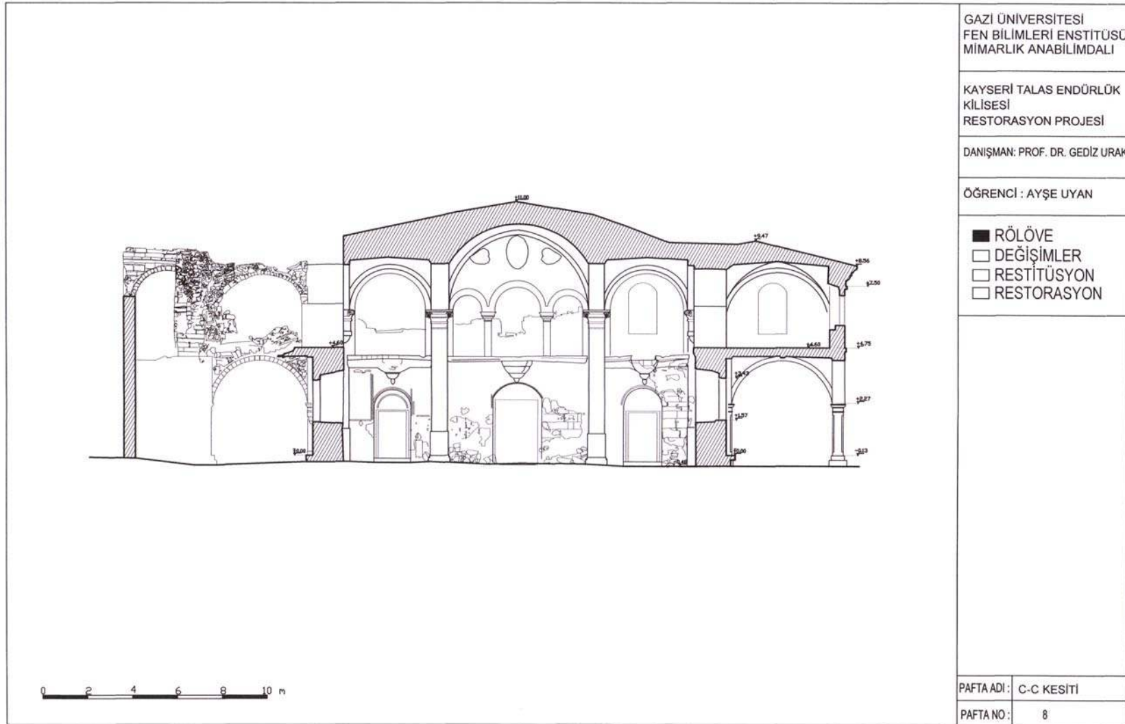
EK-8 Rölöve C-C kesiti
