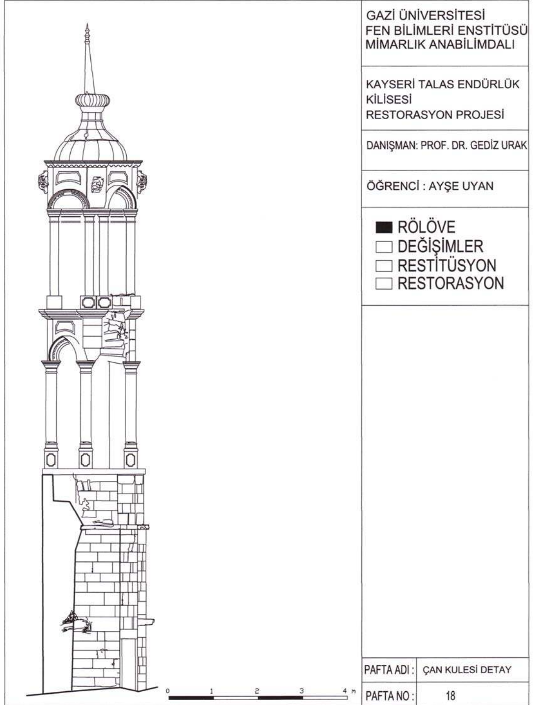
EK-18 Rölöve çan kulesi detay
