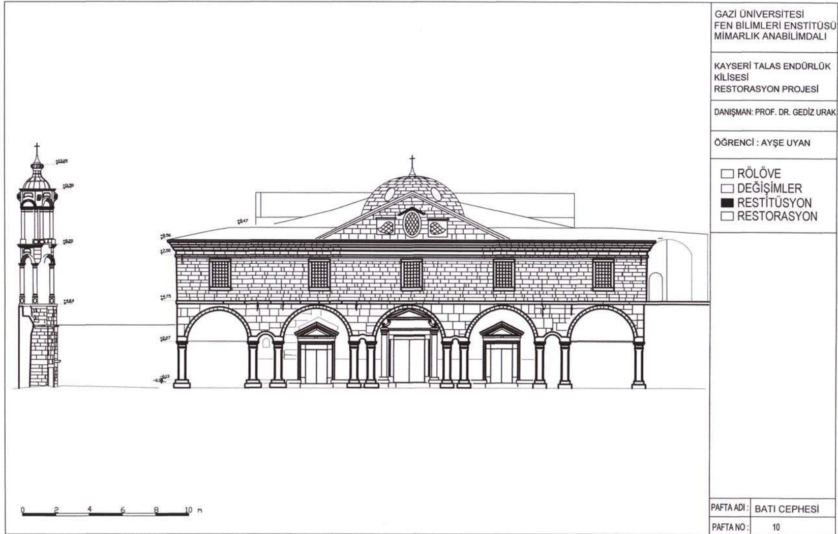
EK-58 Restitüsyon batı cephesi
