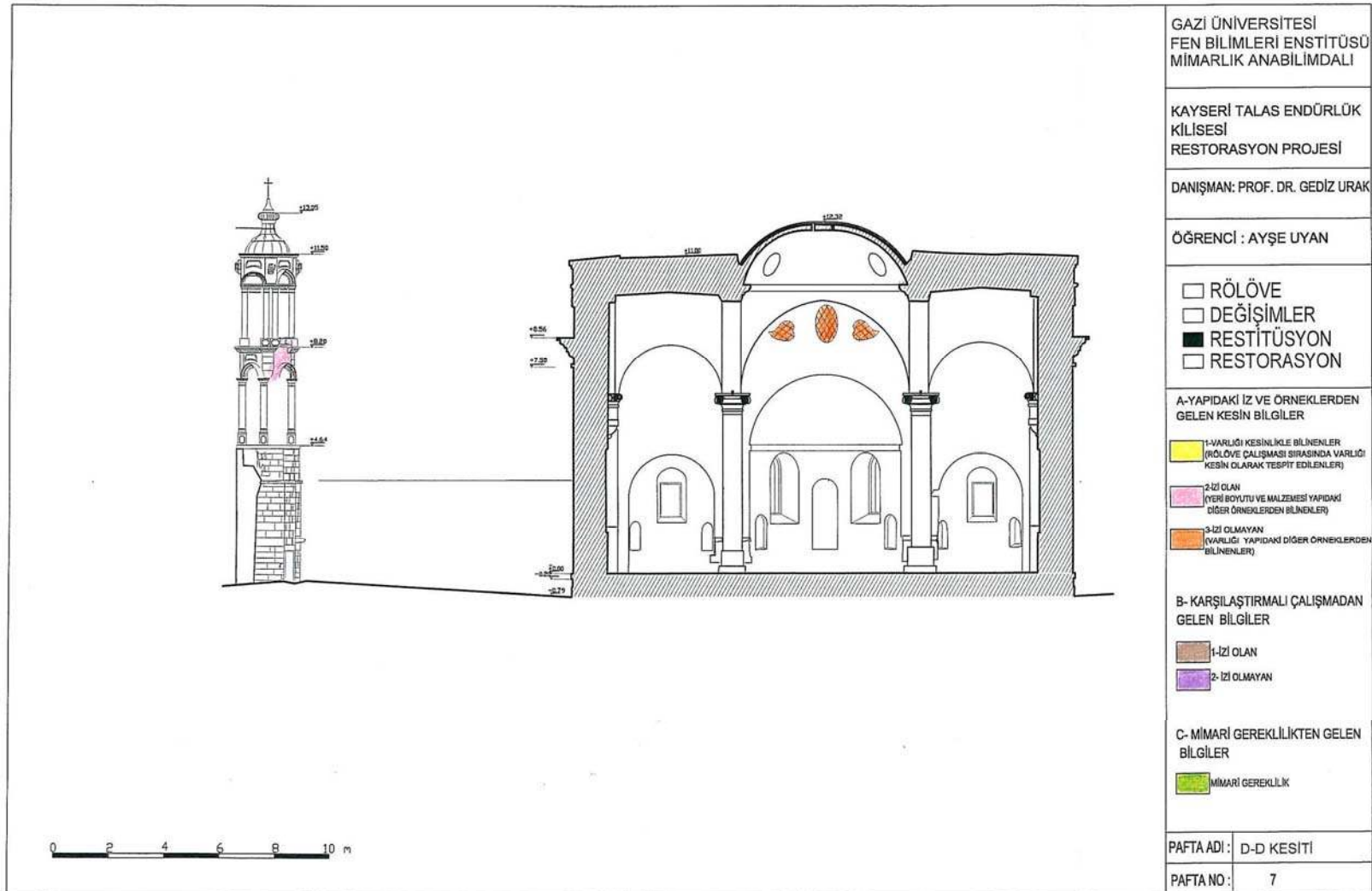
EK-43 Restitüsyon kaynak kullanım paftası D-D kesiti
