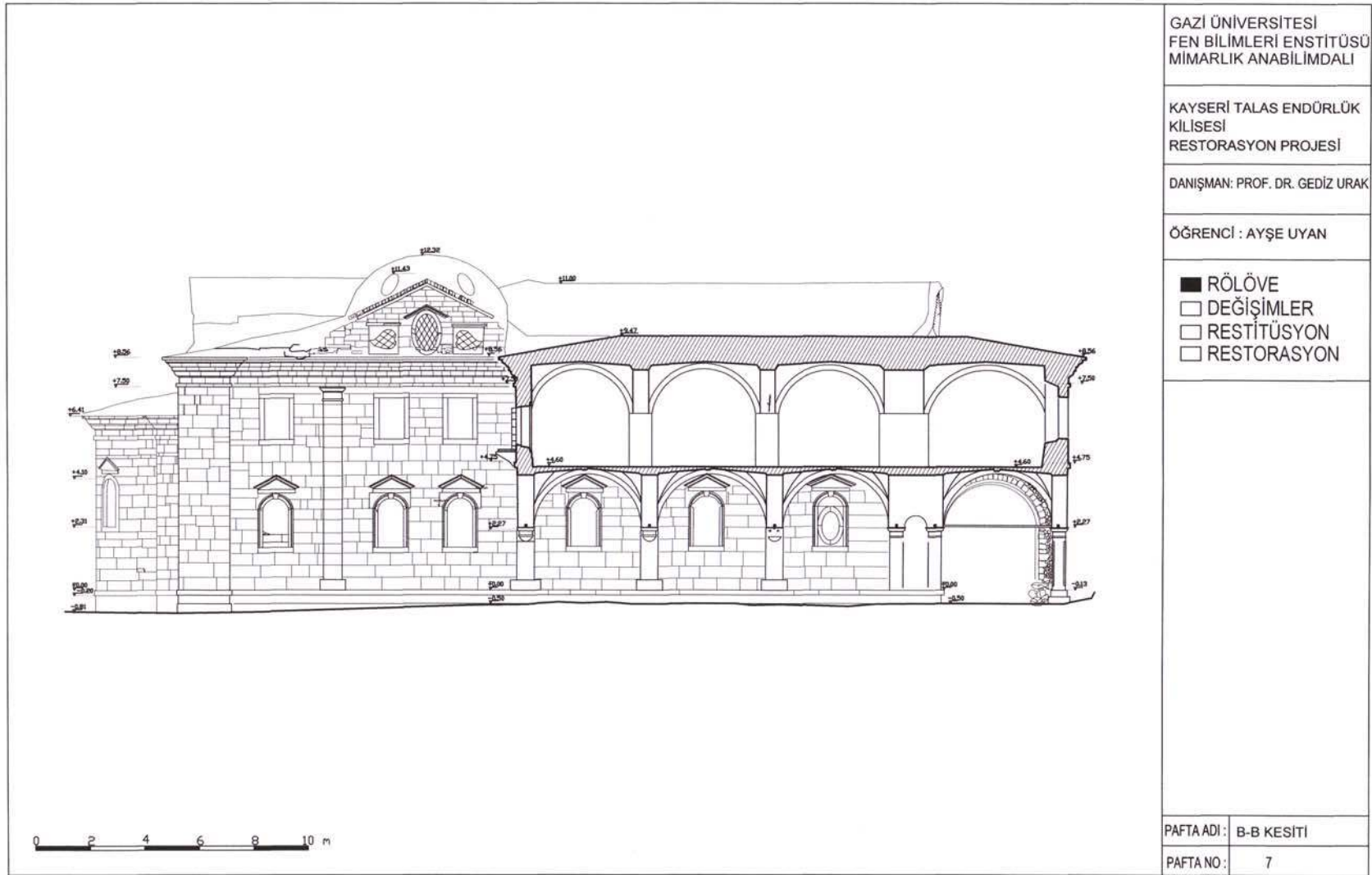
EK-7 Rölöve B-B kesiti
