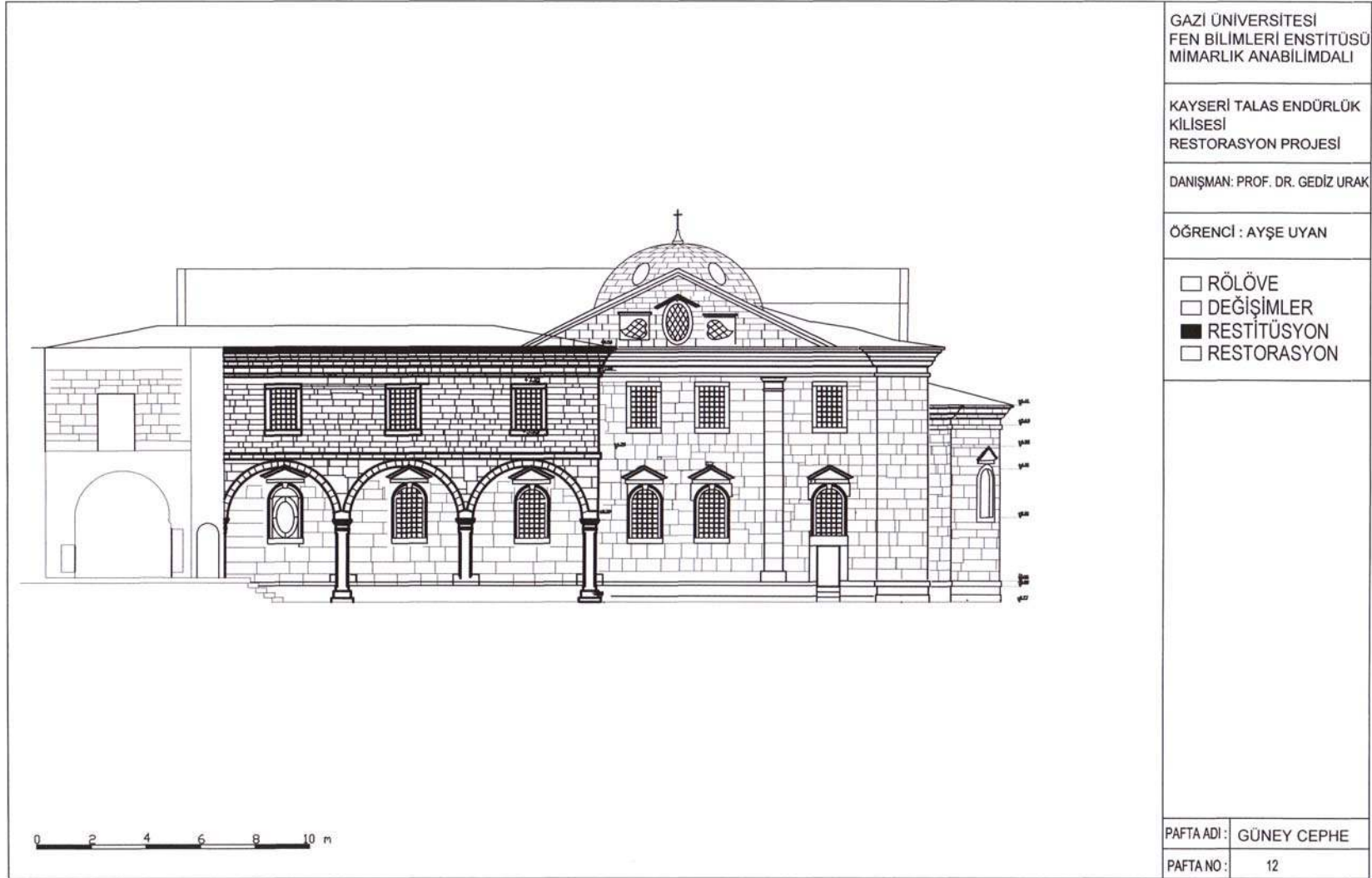
EK-60 Restitüsyon güney cephesi
