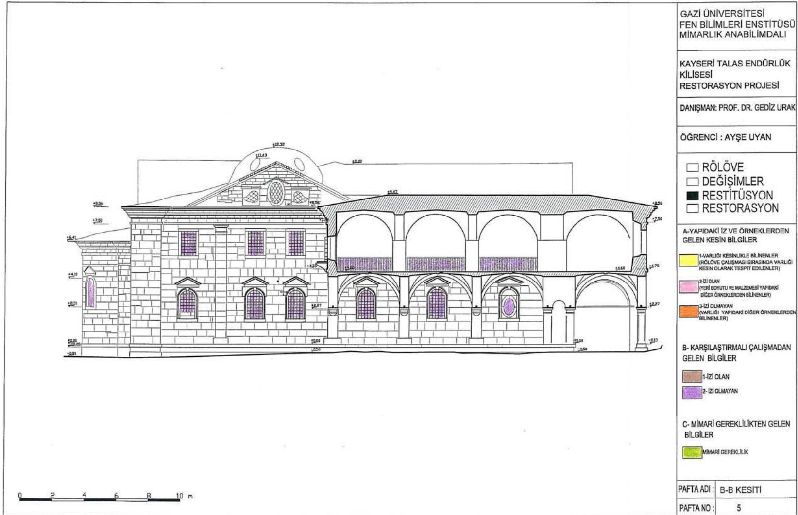
EK-41 Restitüsyon kaynak kullanım paftası B-B kesiti
