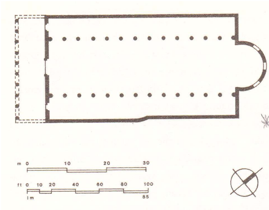
Şekil 3.3. Santa Sabina Kilisesi, Roma 422-432 yılları arası [8]
