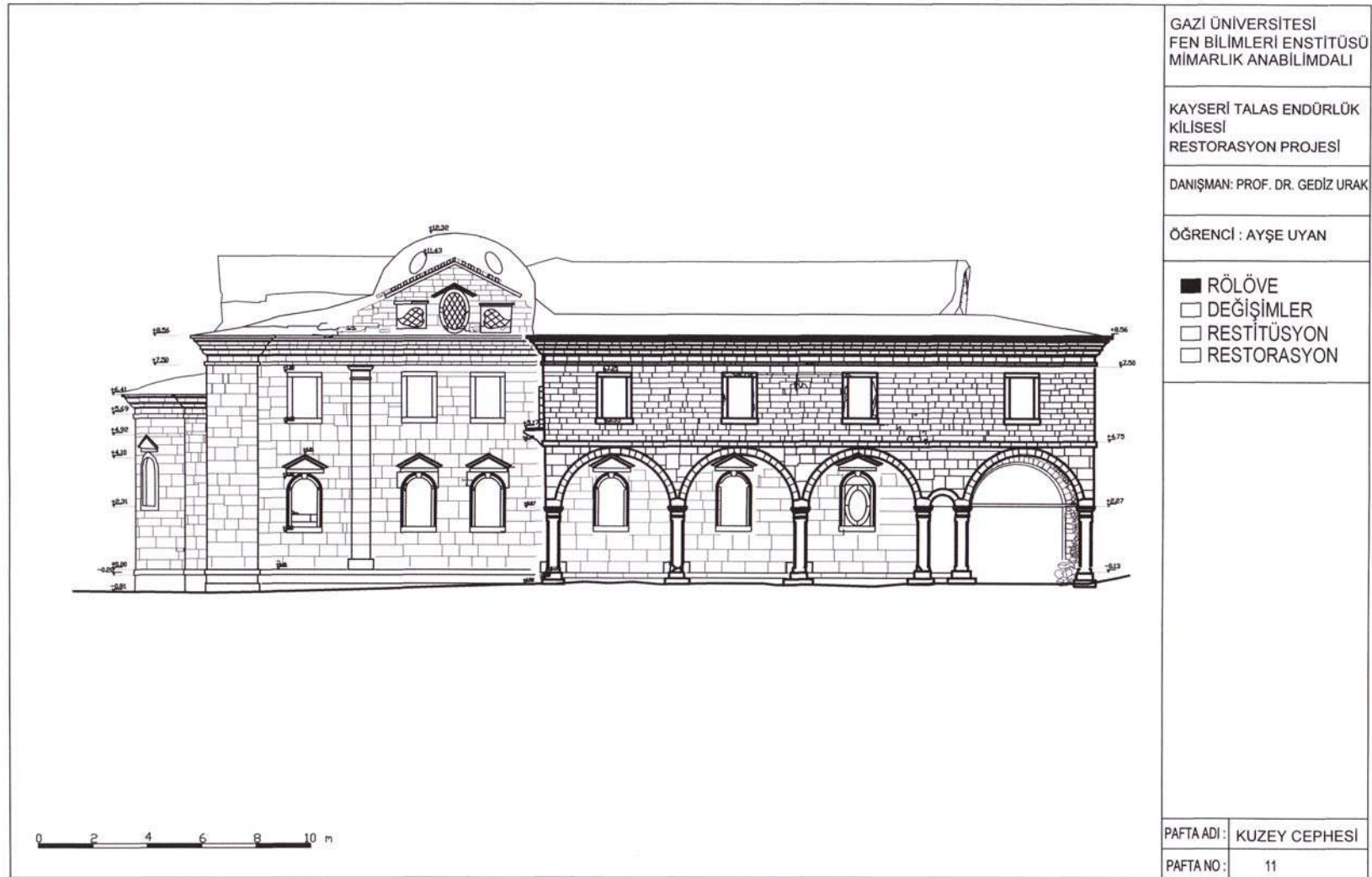
EK-11 Rölöve kuzey cephesi
