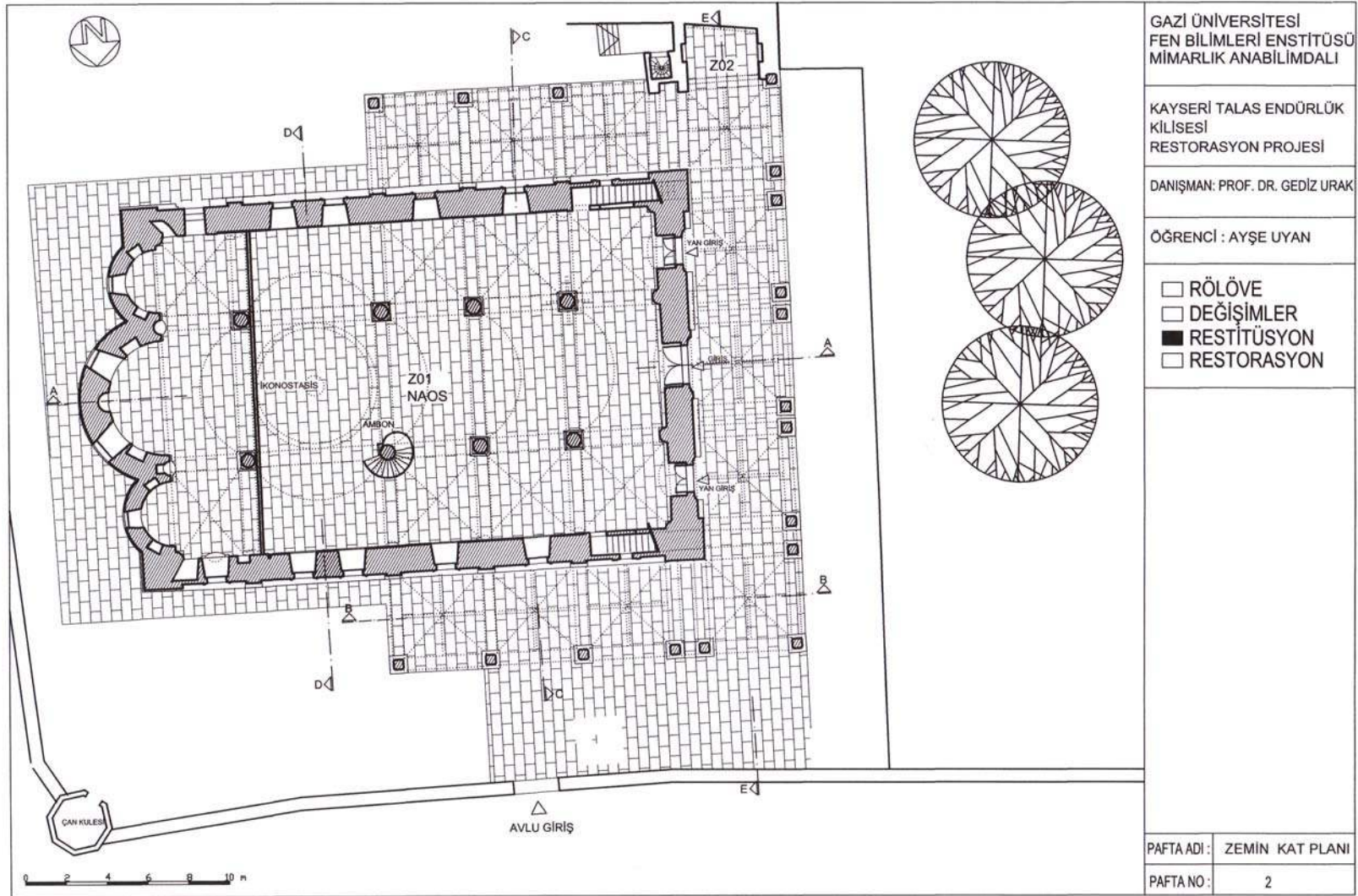
EK-50 Restitüsyon zemin kat planı
