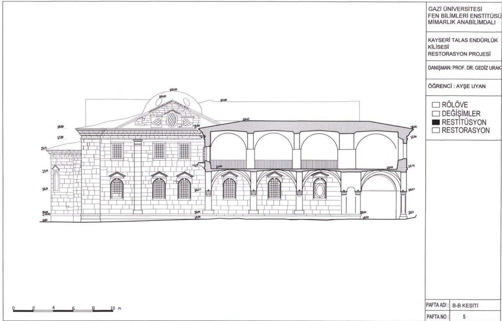
EK-53 Restitüsyon B-B kesiti
