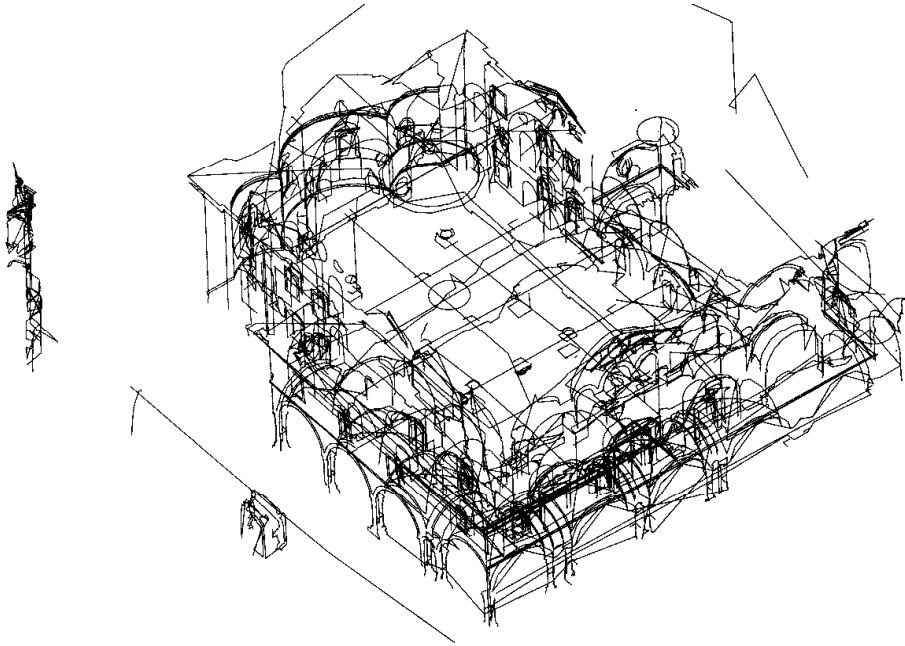
Şekil 5.6. Yapının kuzeybatıdan üç boyutlu hali
