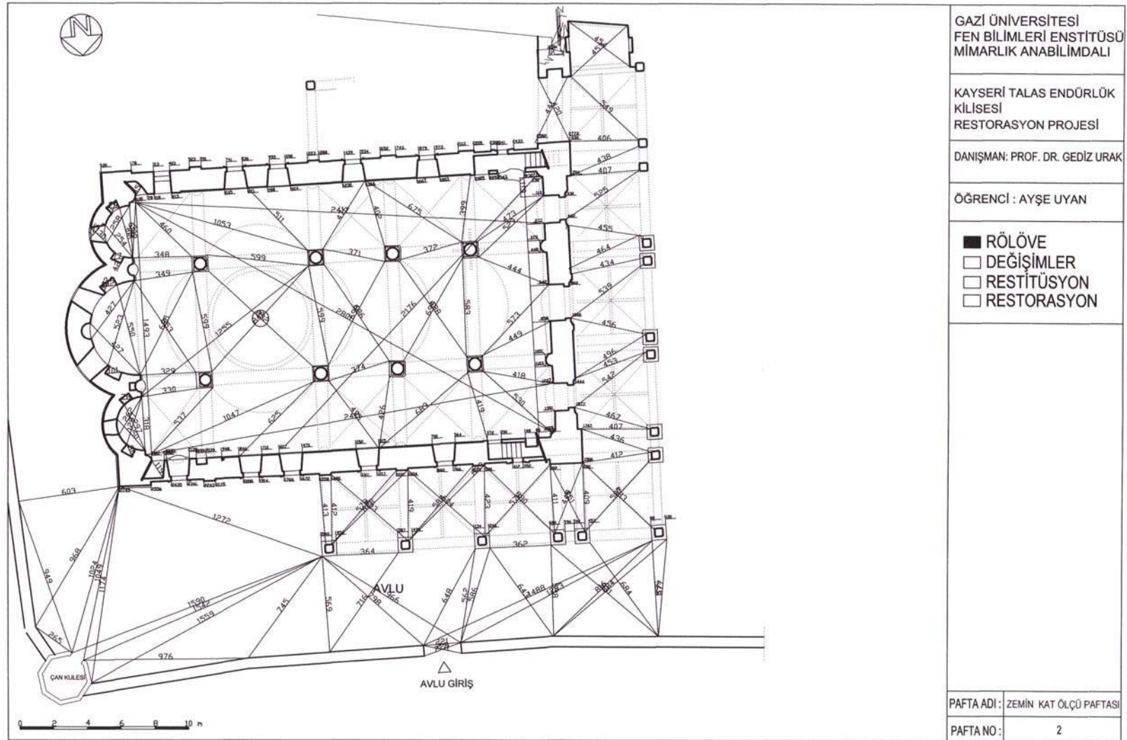
EK-2 Rölöve zemin kat ölçü paftası
