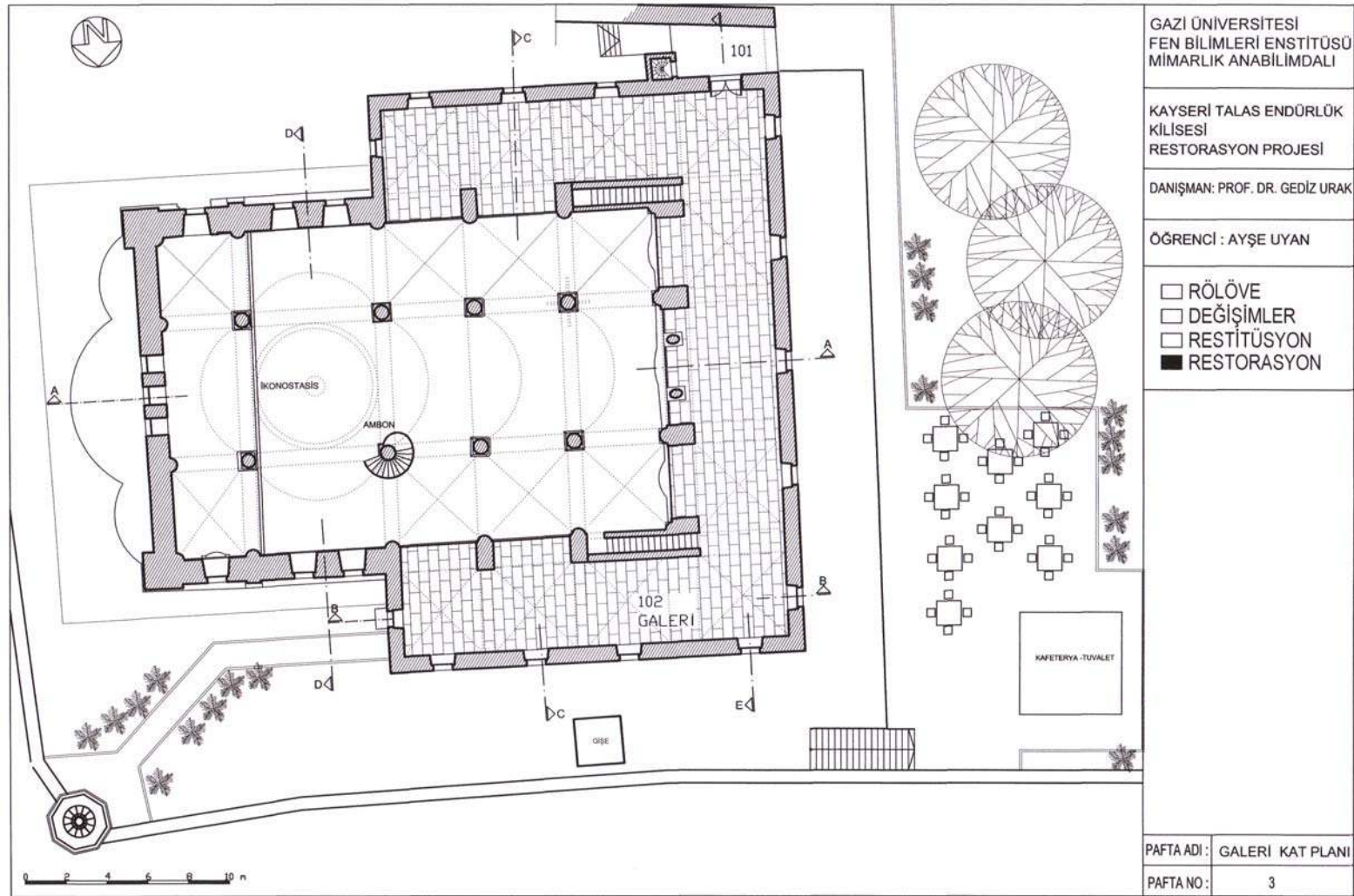
EK-63 Restorasyon galeri kat planı
