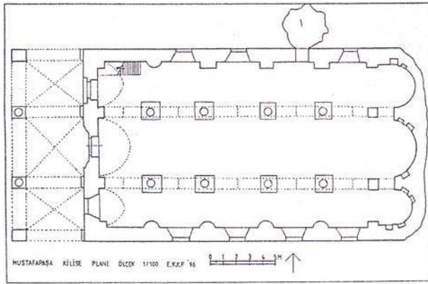
Şekil 6.65. Constantina ve Helena Kilisesi Plan [18]
