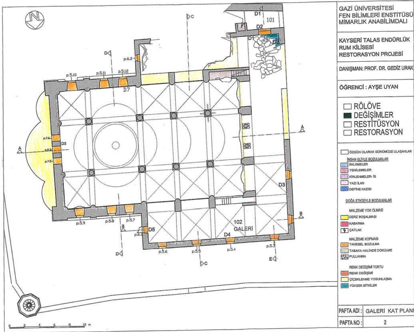
EK-20 Değişim ve bozulmalar galeri kat planı
