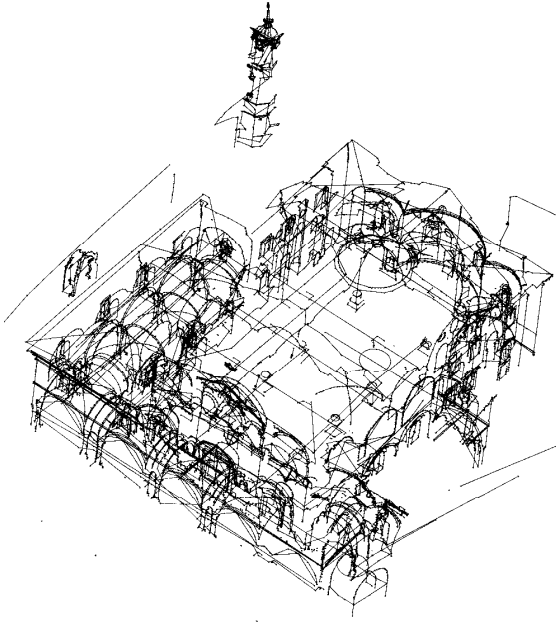
Şekil 5.3. Lazer aletiyle yapının üç boyutunun çıkarılması (güneybatı)
