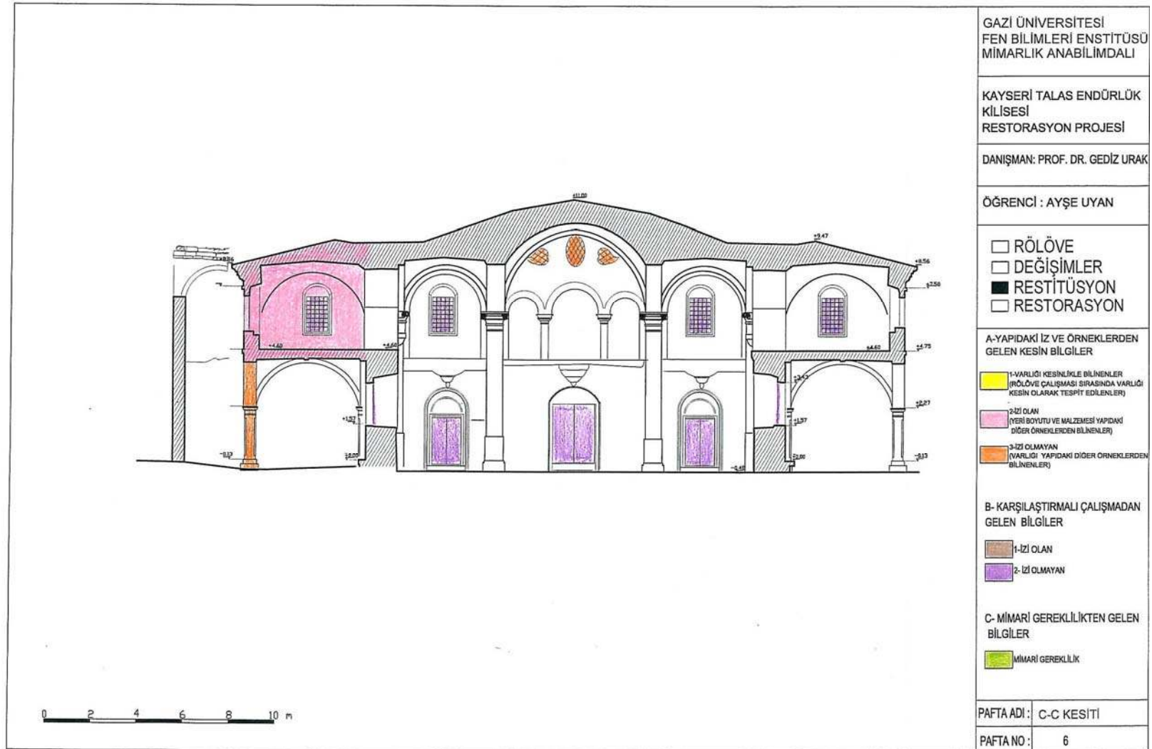
EK-42 Restitüsyon kaynak kullanım paftası C-C kesiti
