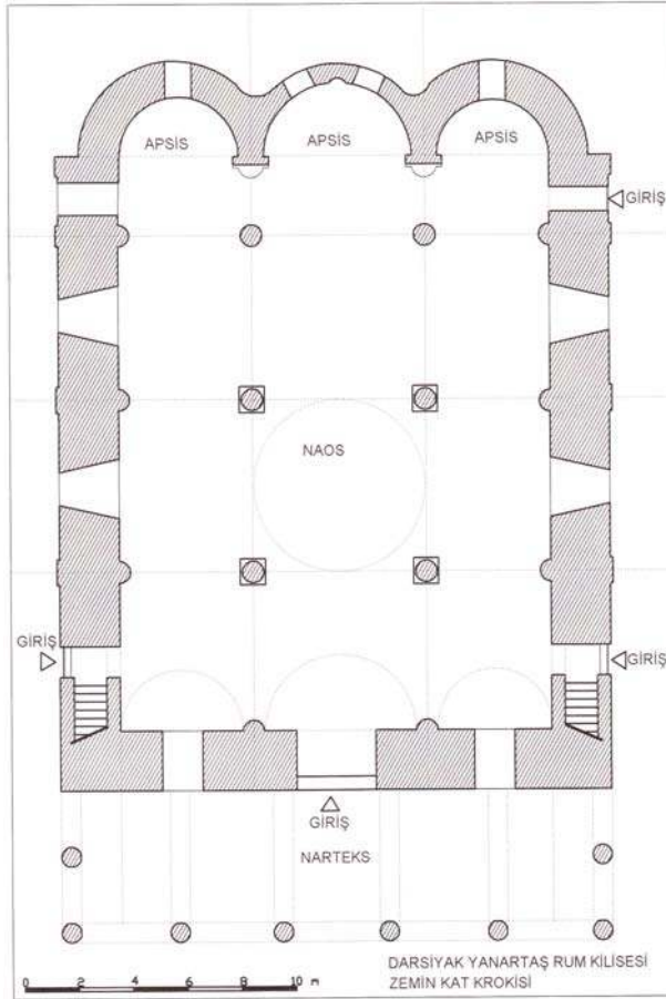
Şekil 6.1. Yanartaş Rum Kilisesi giriş zemin kat planı (Uyan A.)
