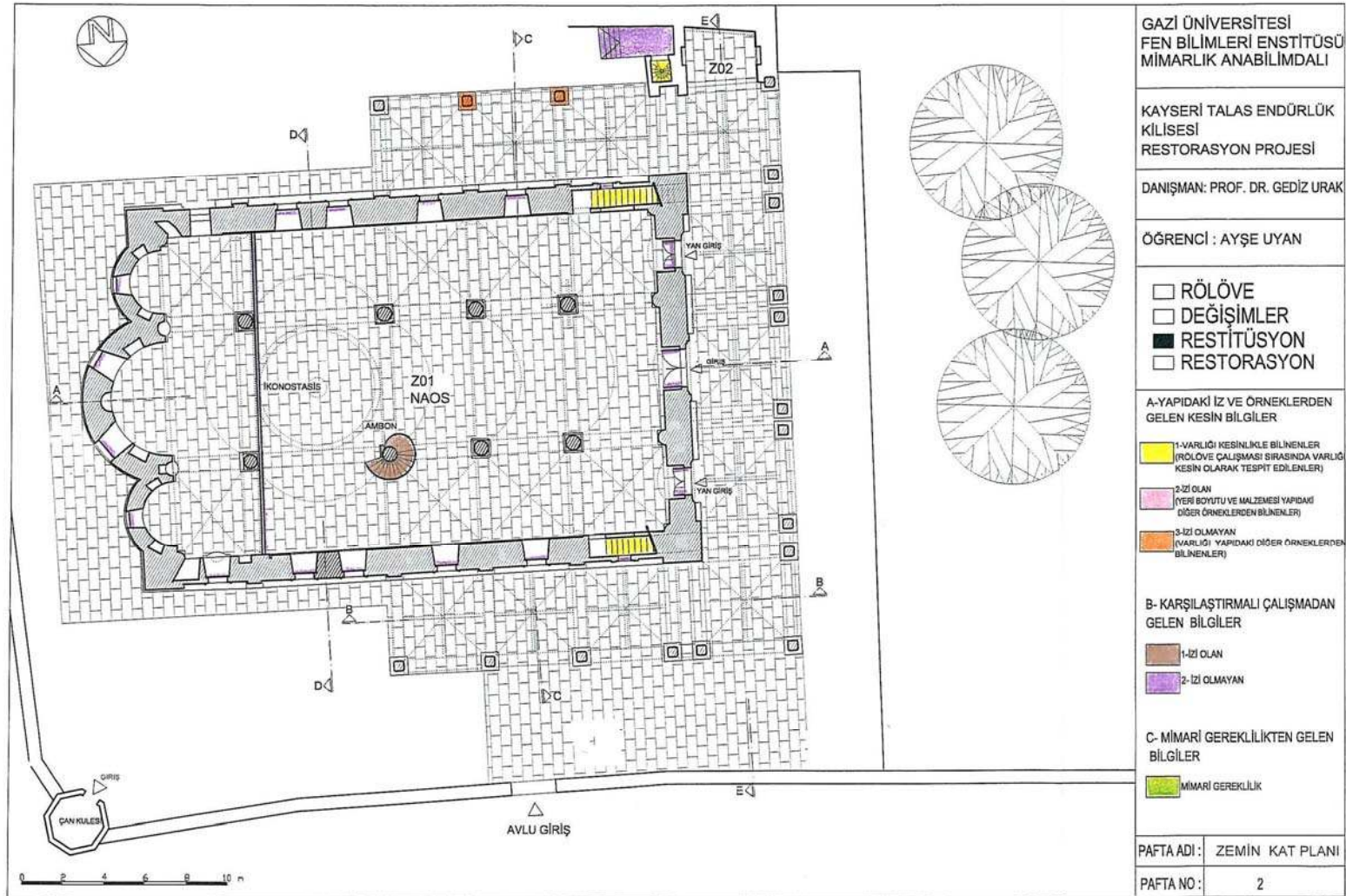
EK-38 Restitüsyon kaynak kullanım paftası zemin kat planı
