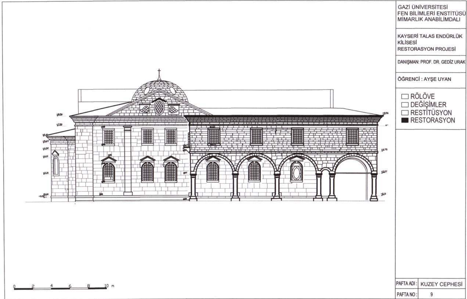
EK-69 Restorasyon kuzey cephesi
