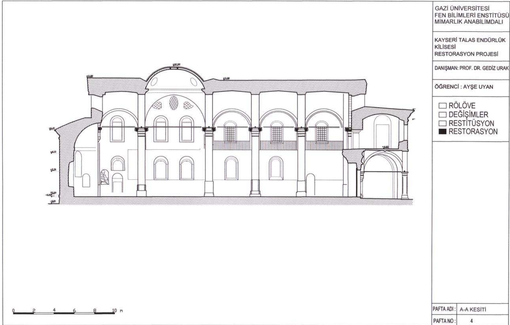
EK-64 Restorasyon A-A kesiti
