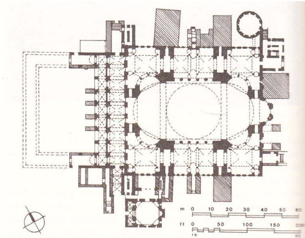
Şekil 3.5. Ayasofya, plan [8]
