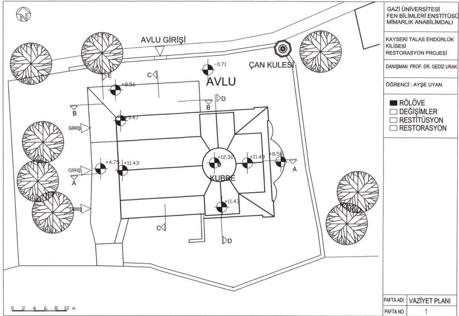
EK-1 Rölöve vaziyet planı
