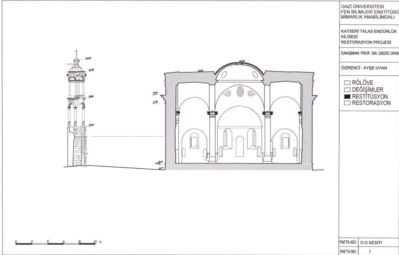
EK-55 Restitüsyon D-D kesiti
