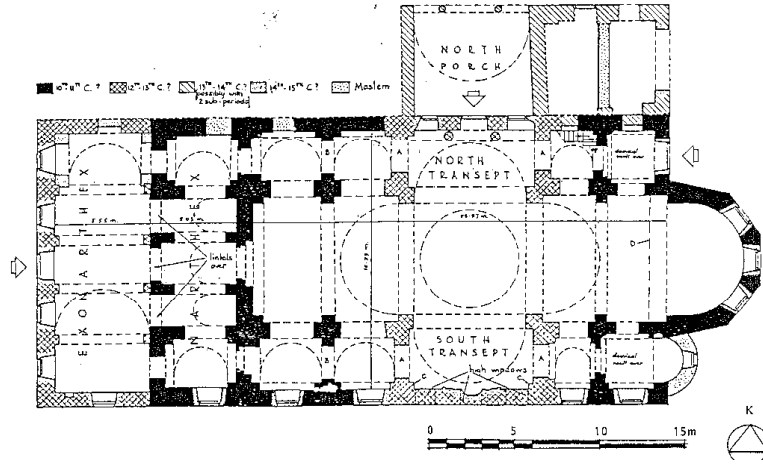
Şekil 6.118. Ortahisar Cami Kilisesi plan [24]
