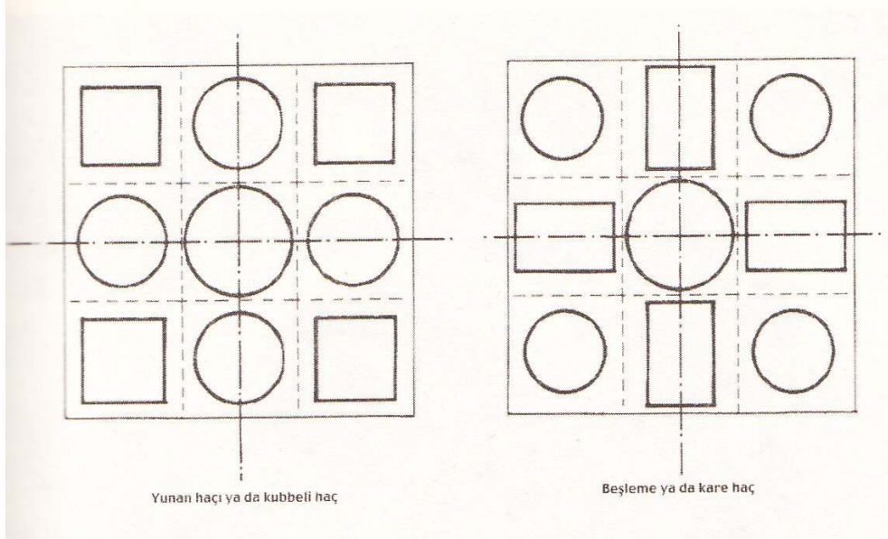
Şekil 3.6. Kubbelerin düzenlenişinin gösterildiği diyagram sayfa 353 [8]
