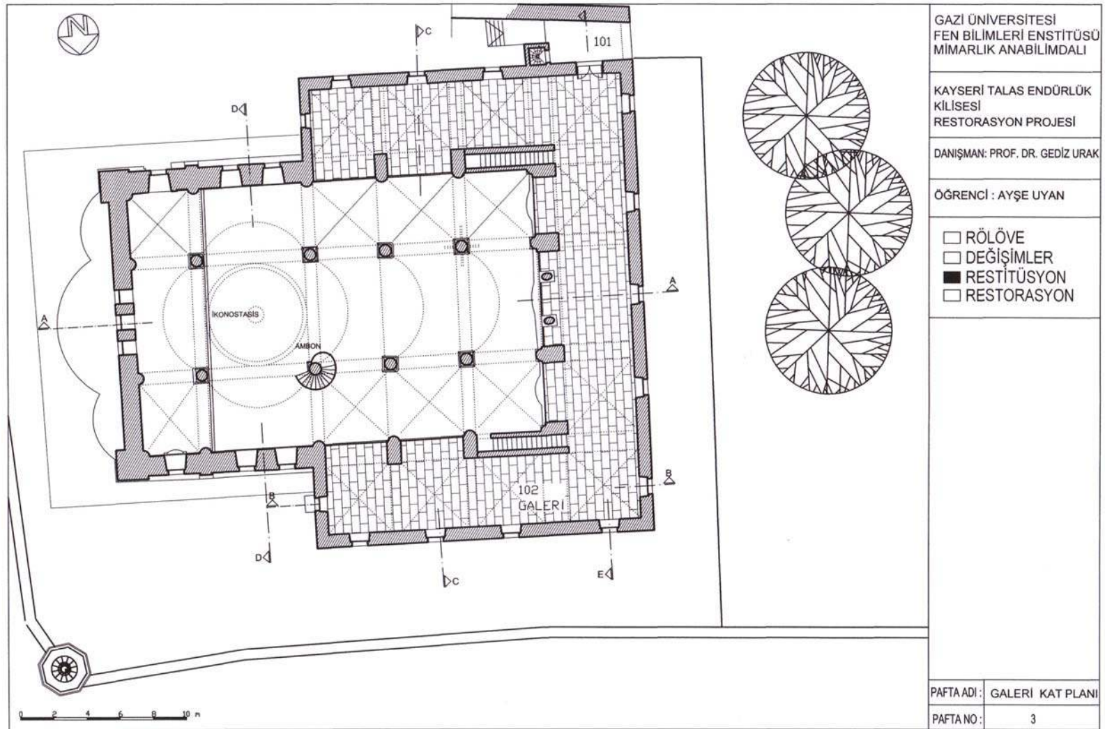
EK-51 Restitüsyon galeri kat planı
