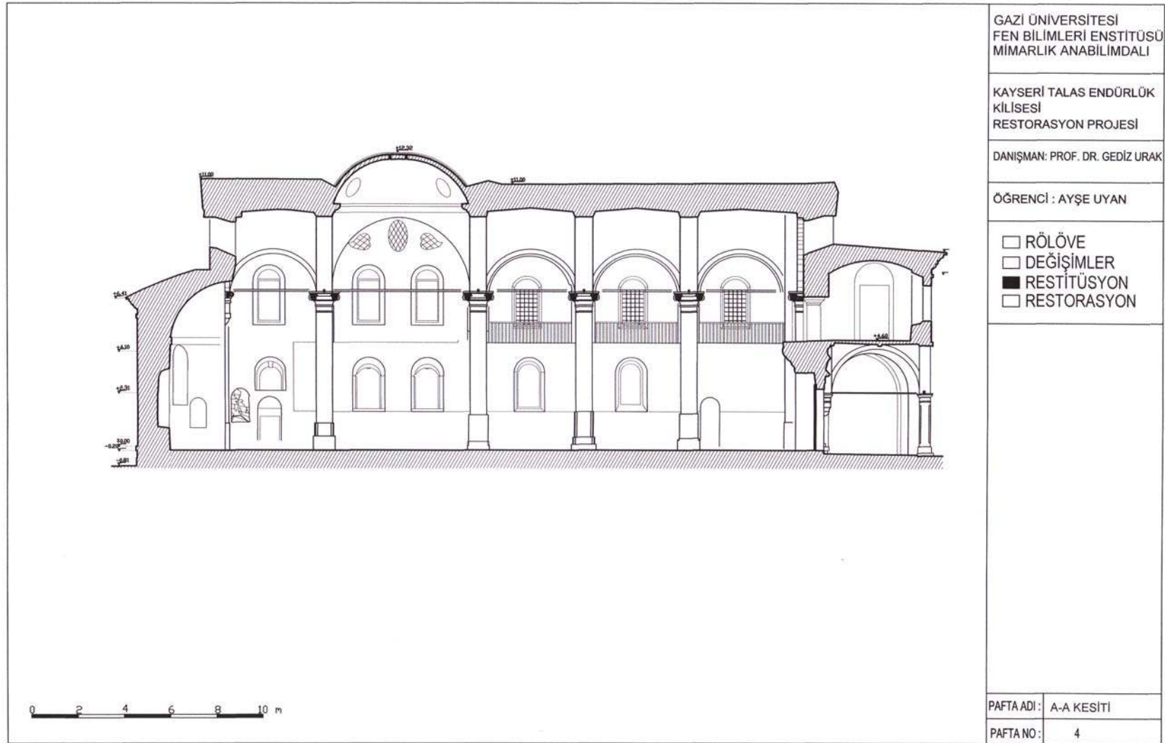
EK-52 Restitüsyon A-A kesiti
