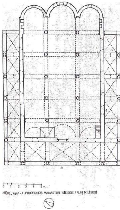
Şekil 6.39. H. Prodromos Manastırı Kilisesi plan [16]
