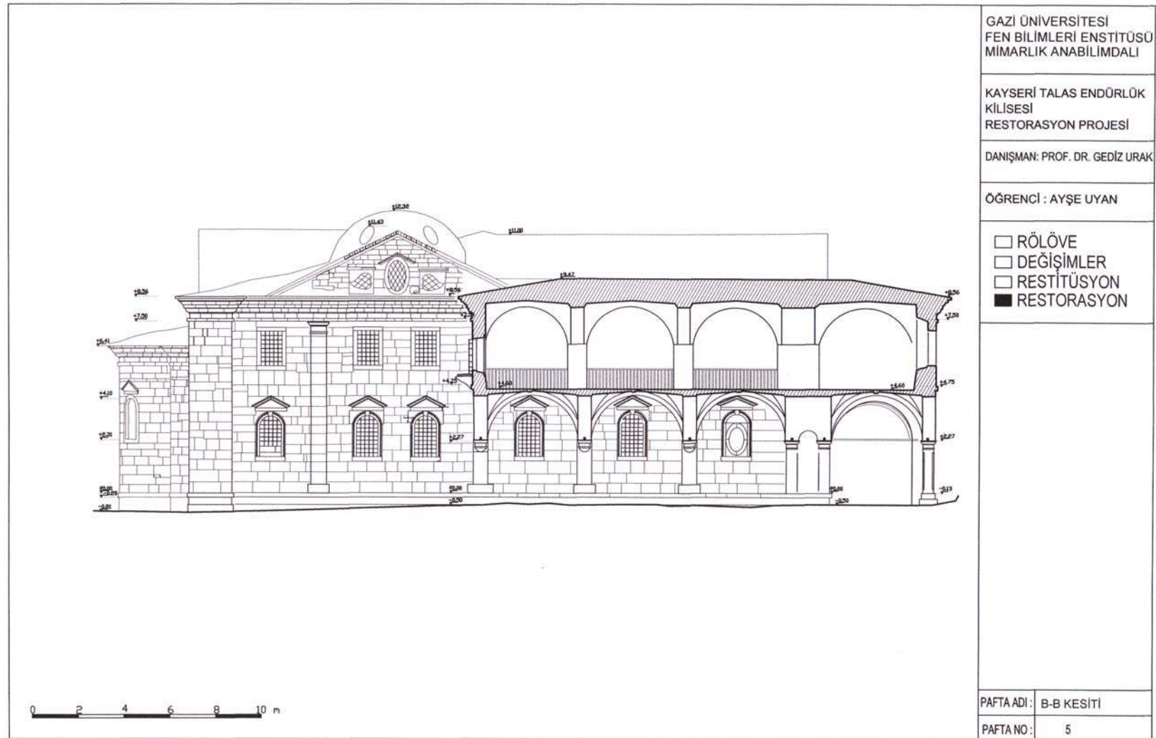
EK-65 Restorasyon B-B kesiti
