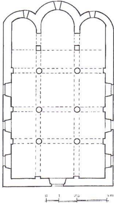
Şekil 6.125. Maçka Aşağı Mahalle Kilisesi plan [23]
