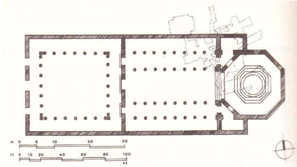
Şekil 3.4. Doğuş Kilisesi, İsrail, 326-333 yılları arası [8]
