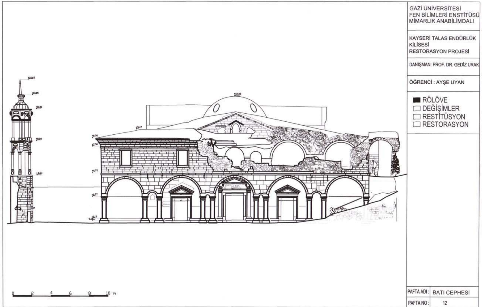
EK-12 Rölöve batı cephesi
