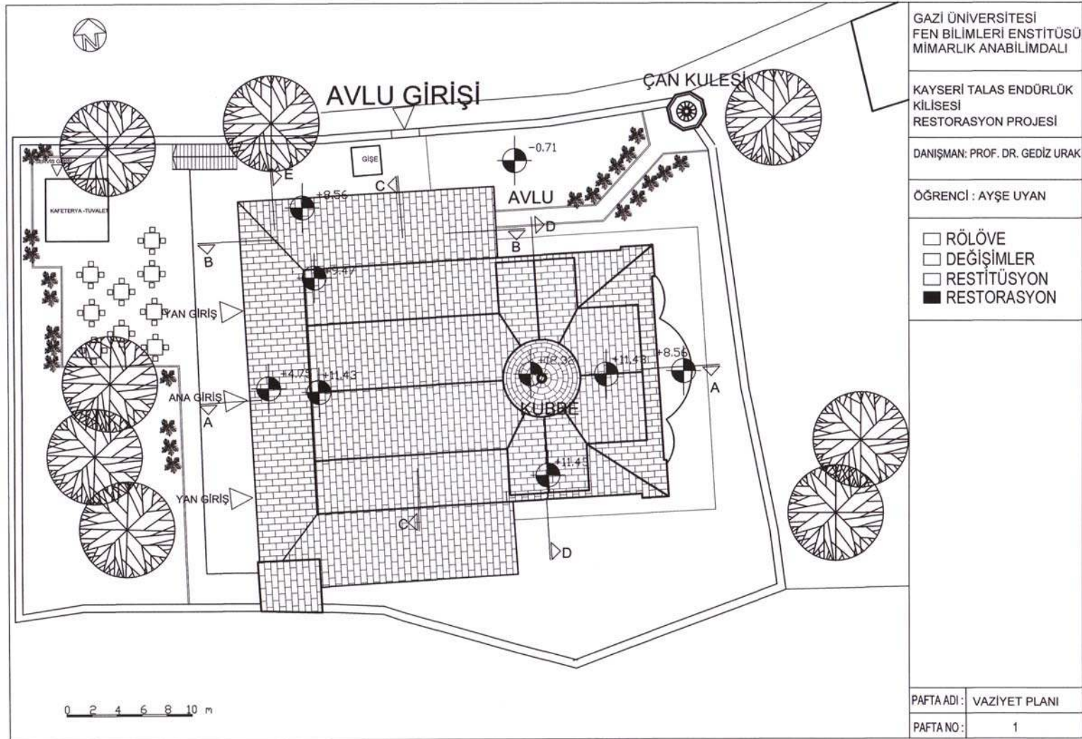
EK-61 Restorasyon vaziyet planı
