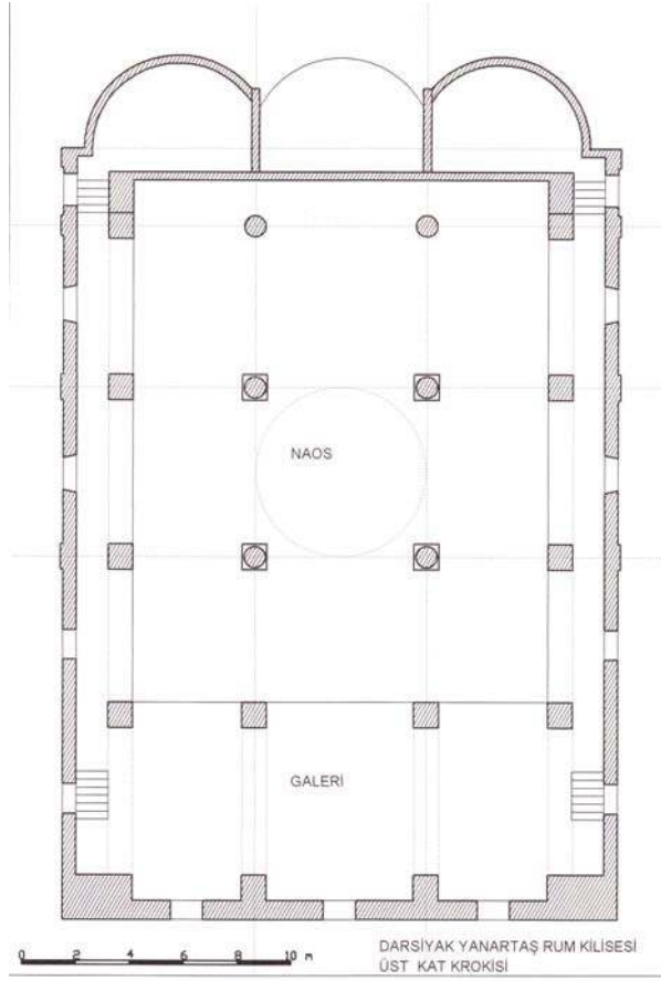
Şekil 6.2. Yanartaş Rum Kilisesi galeri katı planı (Uyan A.)
