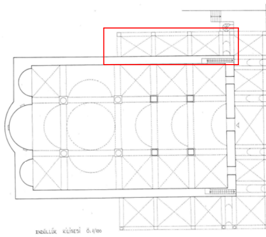
Şekil 7.3. Fügen İlter'in 1989 Endrlük Kilisesi çizimi [20]
