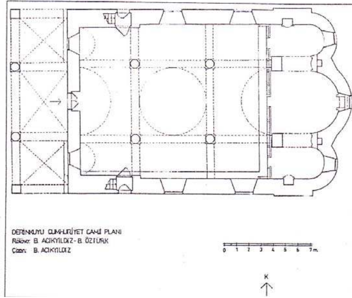
Şekil 6.82. Başmelekler Kilisesi plan [17]
