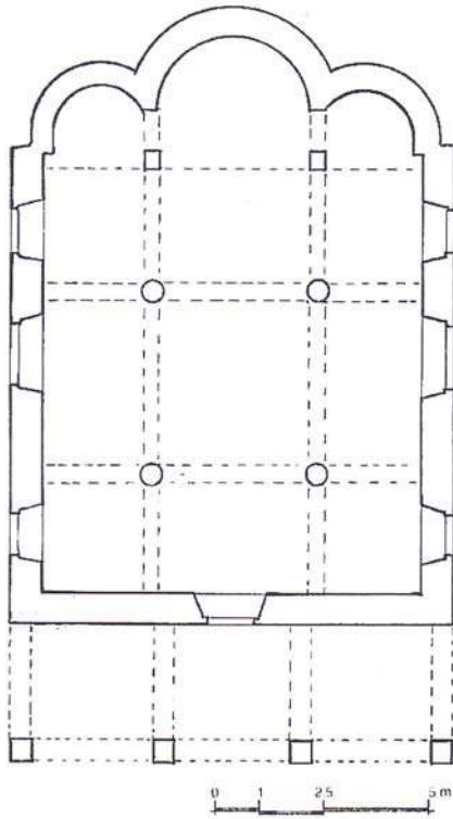
Şekil 6.122. Sürmene Dirlik Köyü Kilisesi plan [23]
