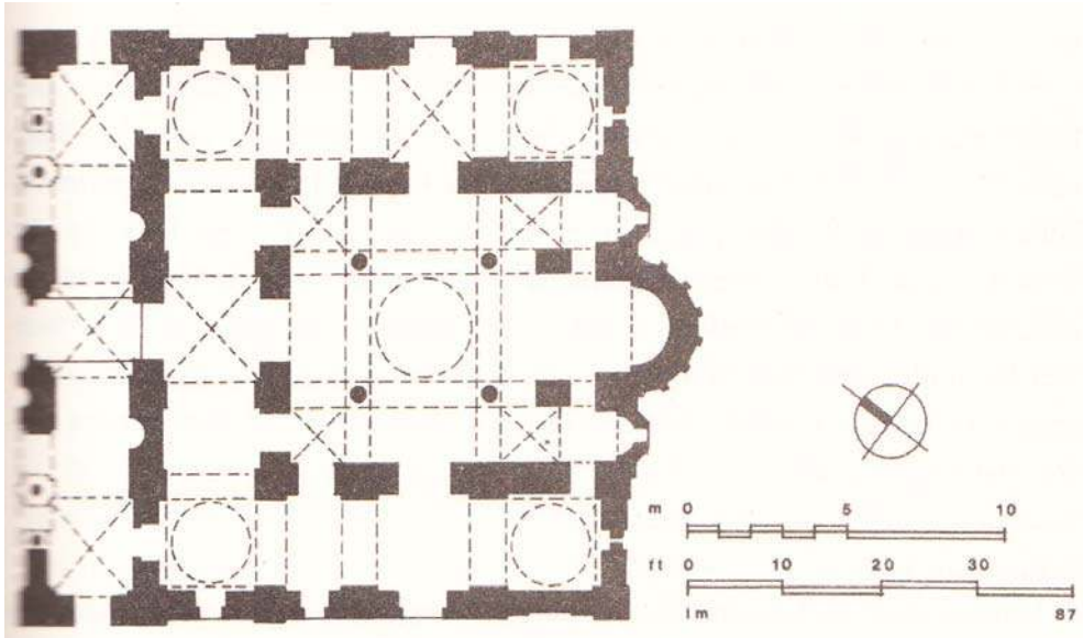
Şekil 3.8. Kutsal Havariler Kilisesi, Selanik, Yunanistan, 1312-1315 [8]
