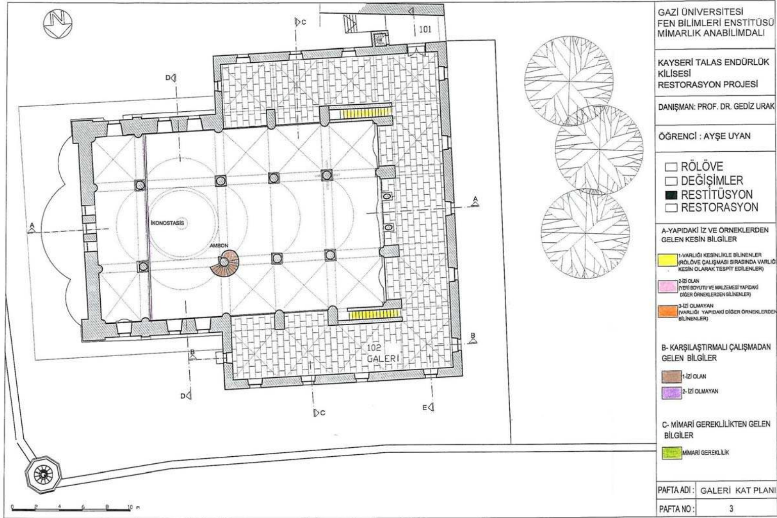
EK-39 Restitüsyon kaynak kullanım paftası galeri kat planı
