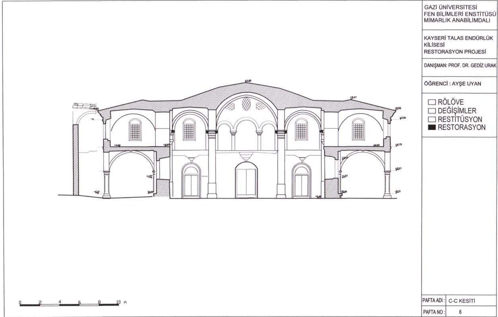
EK-66 Restorasyon C-C kesiti
