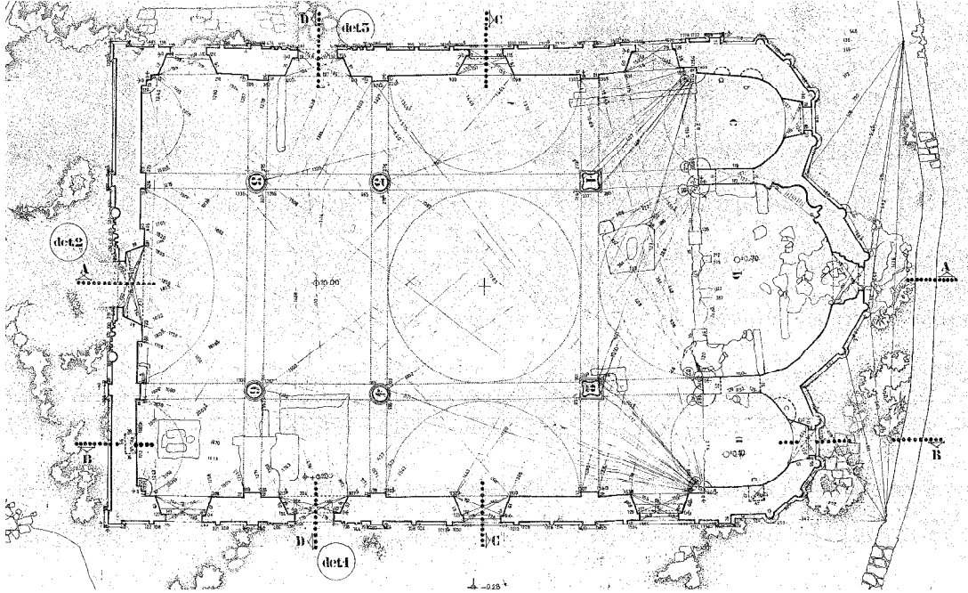
Şekil 6.127. Gogara Kilisesi plan [25]
