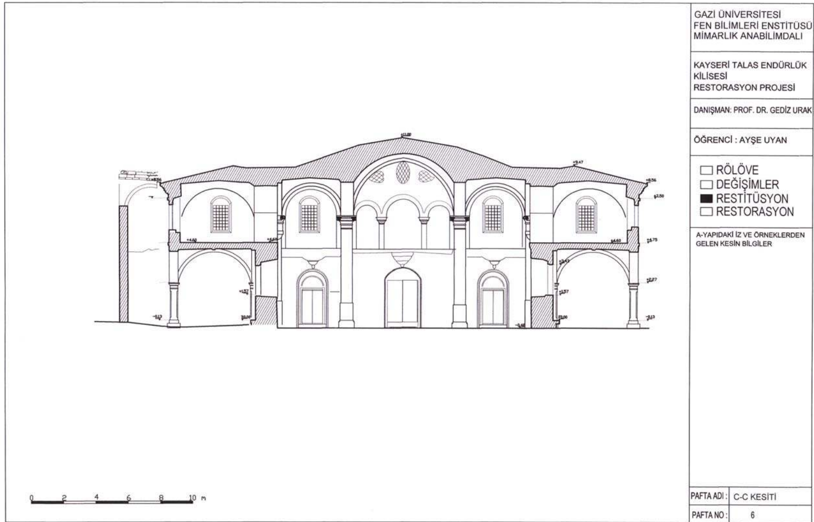
EK-54 Restitüsyon C-C kesiti
