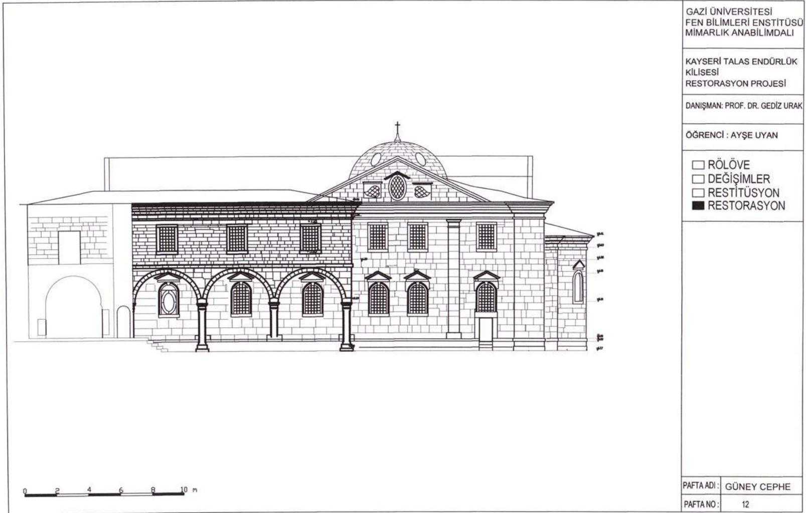
EK-72 Restorasyon güney cephesi
