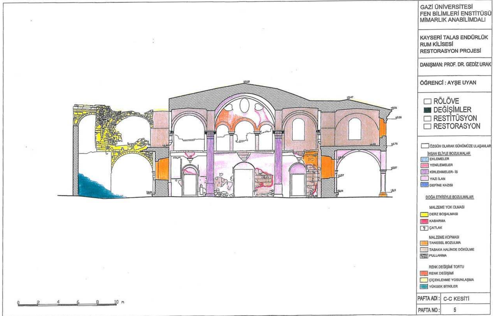
EK-23 Değişim ve bozulmalar C-C kesiti
