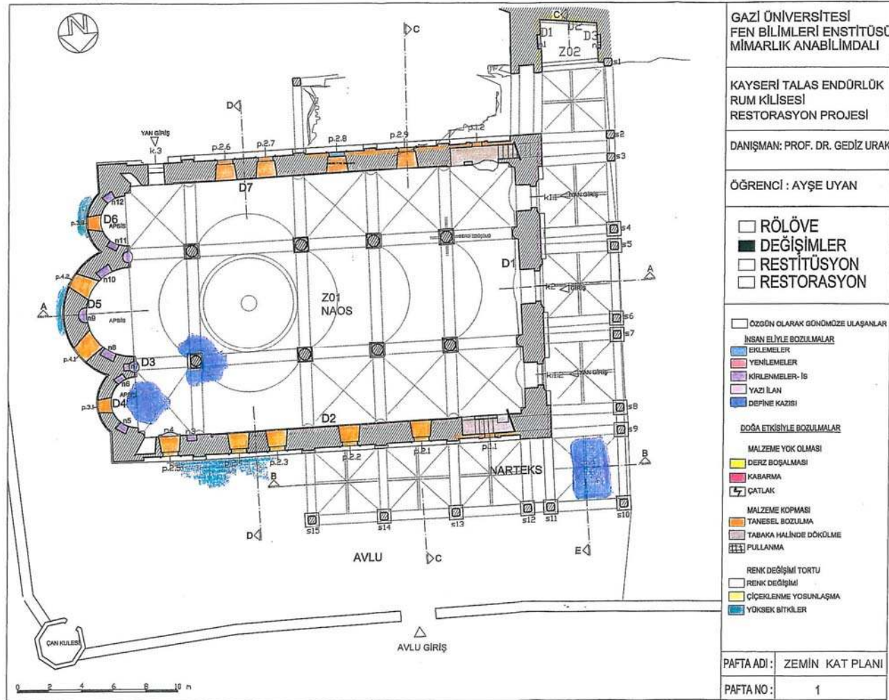
EK-19 Değişim ve bozulmalar zemin kat planı
