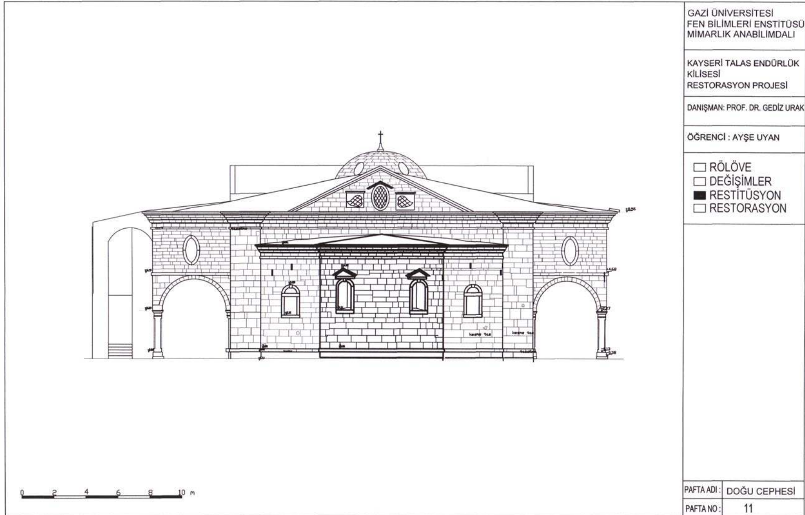
EK-59 Restitüsyon doğu cephesi
