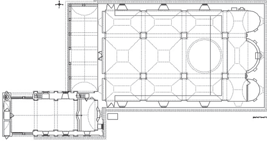
Şekil 6.36. Zincidere Manastırı Kilisesi plan [15]
