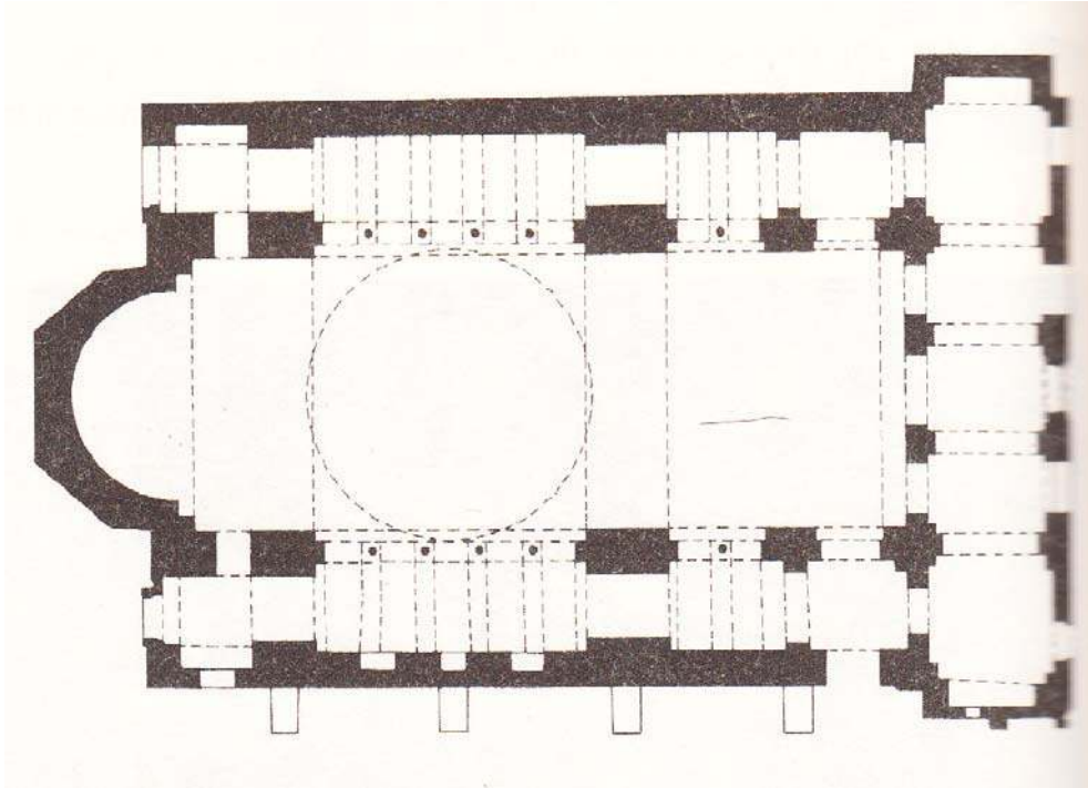
Şekil 3.7. Aya İrini (kutsal huzur), Türkiye 532 [8]
