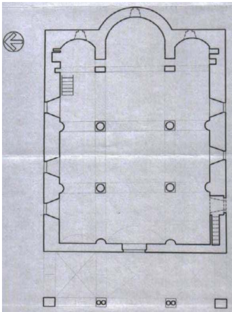
Şekil 6.28. Ağırnas Rum Kilisesi plan [13]
