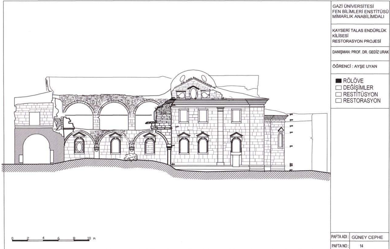
EK-14 Rölöve güney cephesi
