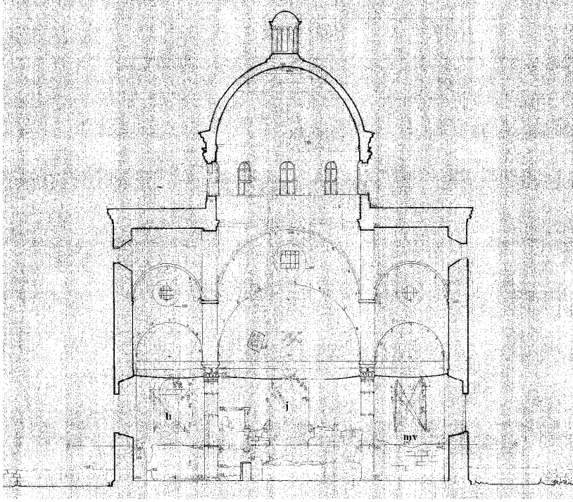
Şekil 6.128. Gogara Kilisesi kesit [25]
