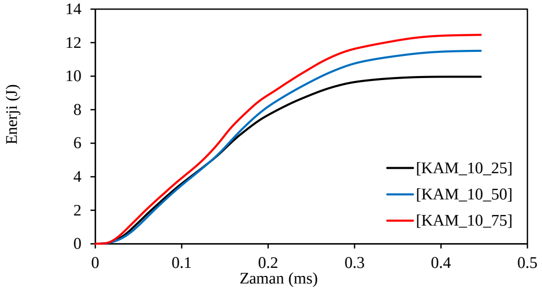
Şekil 6.39 Ortam ısisına göre %5 kam takviyeli kiriş numunelerinin enerji zaman grafiğı
