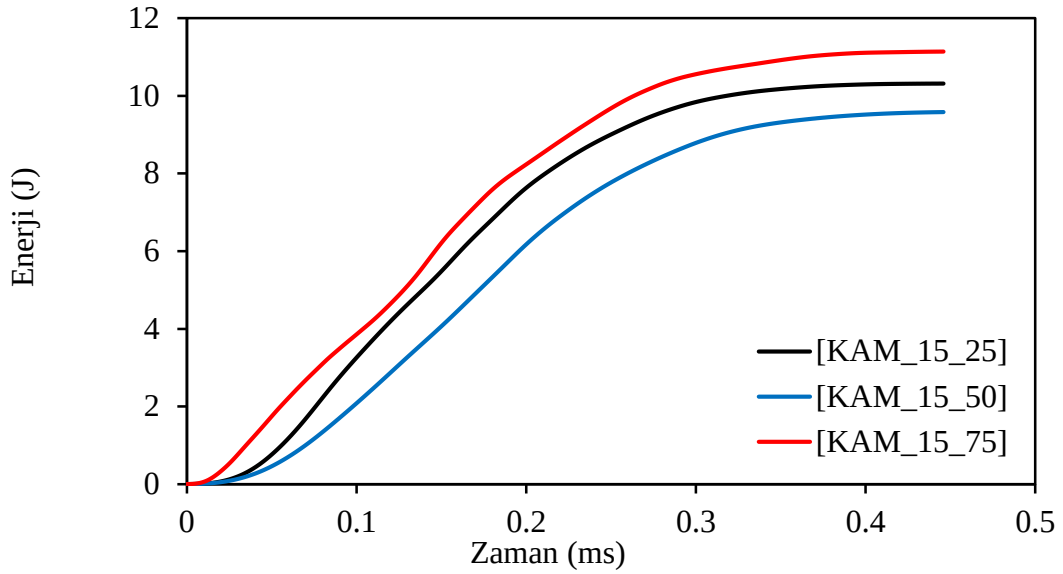
Şekil 6.40 Ortam ısisına göre %15 kam takviyeli kiriş numunelerinin enerji zaman grafiğı
