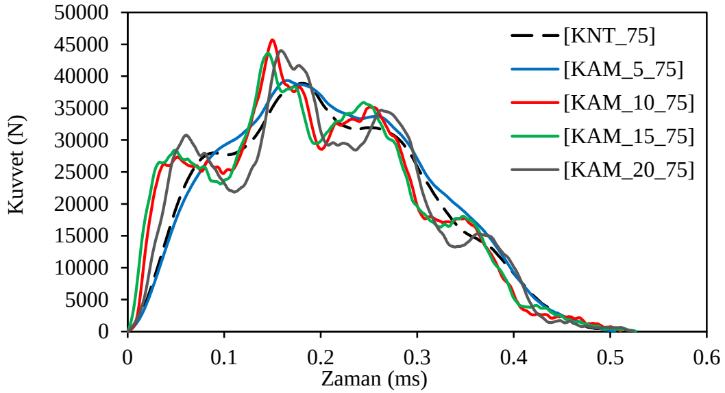
Şekil 6.30 75 °C ortam ısısı şartlarında ağırlık düşürme deneyine tabi tutulan kiriş numunelerinin tepki kuvveti-zaman grafiği
