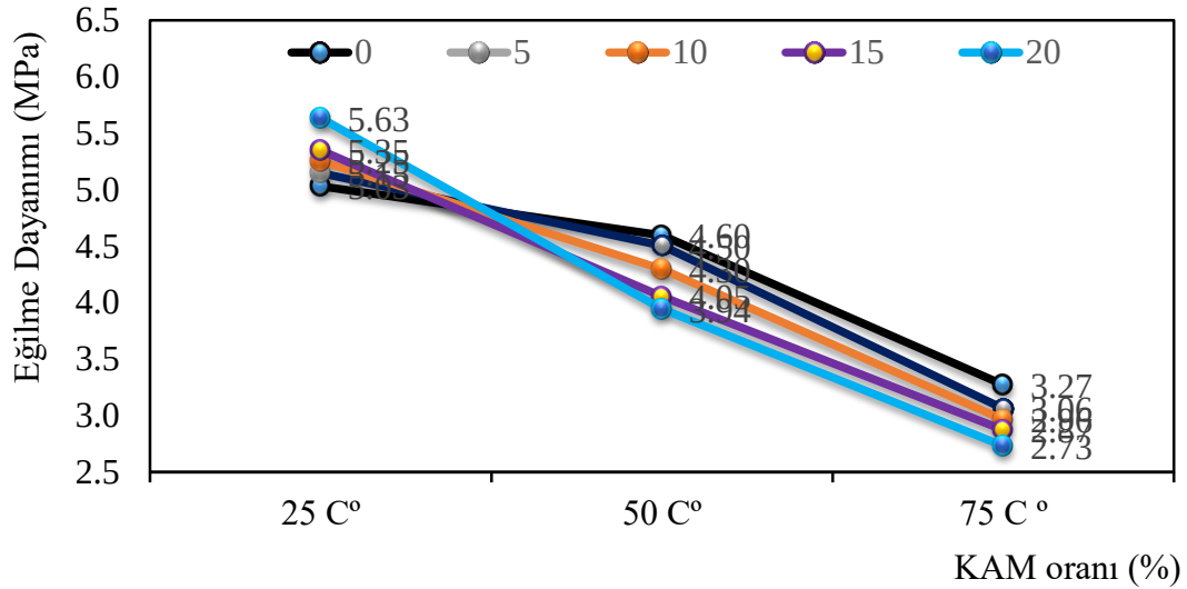
Şekil 6.13 Ortam ısisına bağlı olarak numunelerdeki eğilmede çekme dayanımı değişimi grafiği
