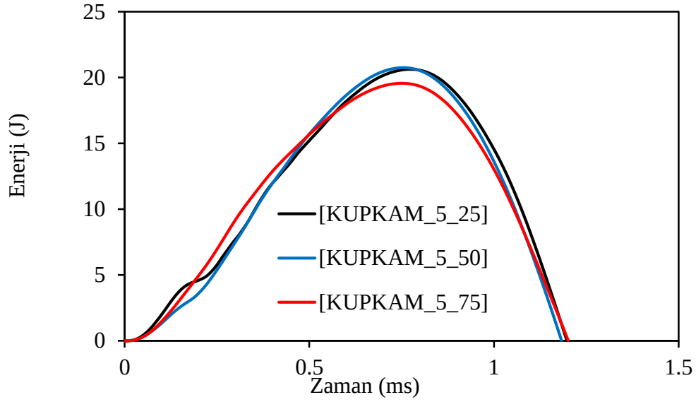
Şekil 6.24 Ortam ısisına göre %5 kam takviyeli k p numunelerinin enerji zaman grafiđi
