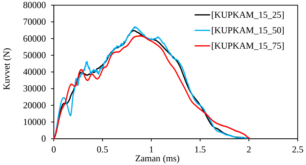
Şekil 6.20 %15 kazınmış asfalt ikameli numunelerin farklı ortam ısıları altında ağırlık düşürme deneyi sonrası oluşan tepki kuvveti-zaman grafiği
