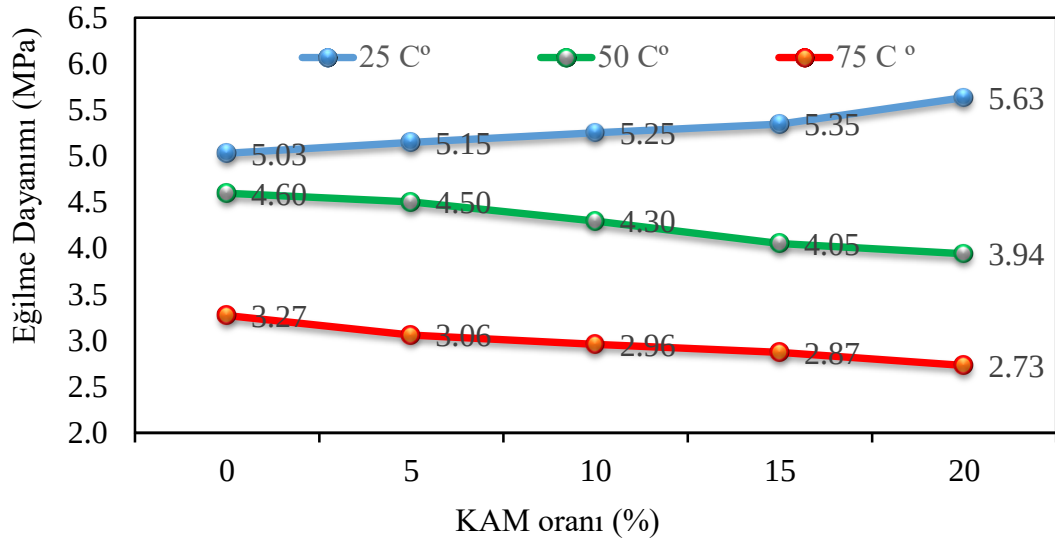
Şekil 6.12 Ortam ısılarına ve içerdiği kam miktarına bağlı olarak numunelerdeki eğilmede çekme dayanım grafiği
