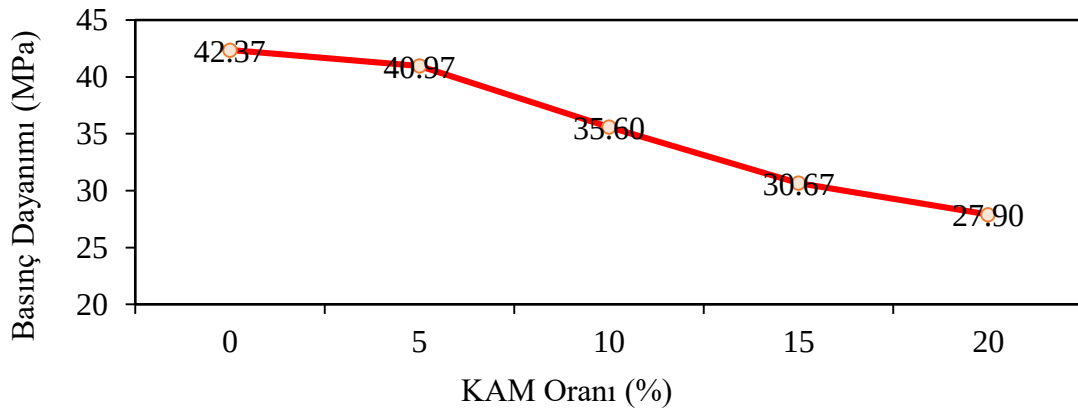
Şekil 6.7 28 günlük numunelerin 25 °C ortam ısisına ve içerdiği kam miktarına göre basınç dayanımları
