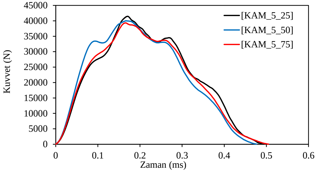
Şekil 6.32 %5 kam ilaveli kiriş numunelerinin ağırlık düşürme deneyi sonrası ortam ısısına bağlı olarak oluşan tepki kuvveti-zaman grafiği
