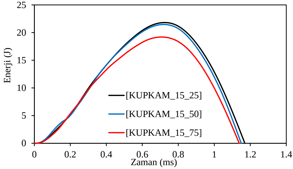
Şekil 6.26 Ortam ısisına göre %15 kam takviyeli küp numunelerinin enerji zaman grafiğı
