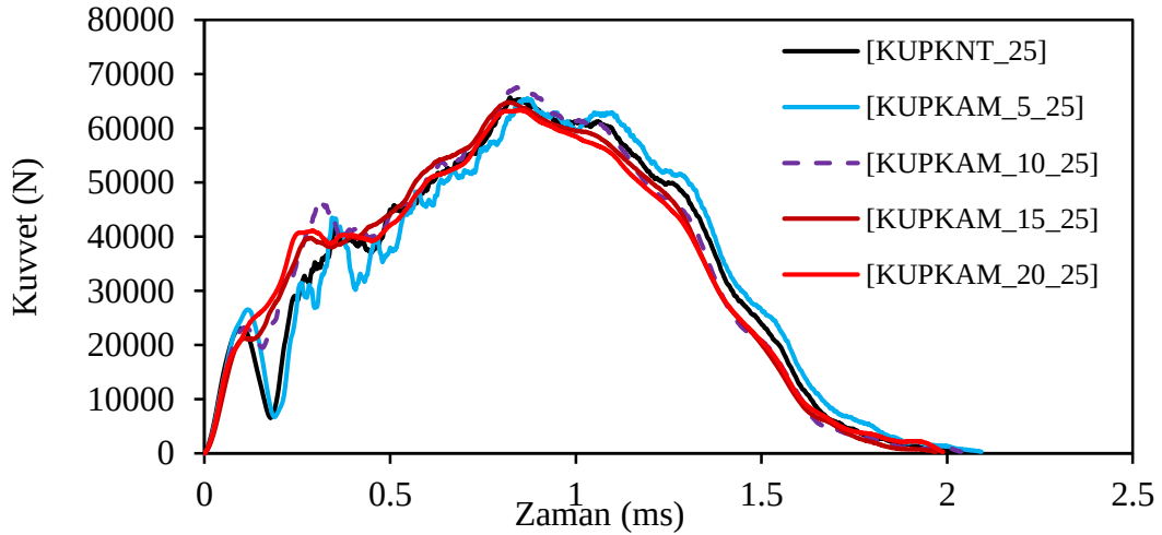
Şekil 6.14 25^{\circ}\text{C} ortam ısısı şartlarında ağırlık düşürme deneyine tabi tutulan küp numunelerin tepki kuvveti-zaman grafiği
