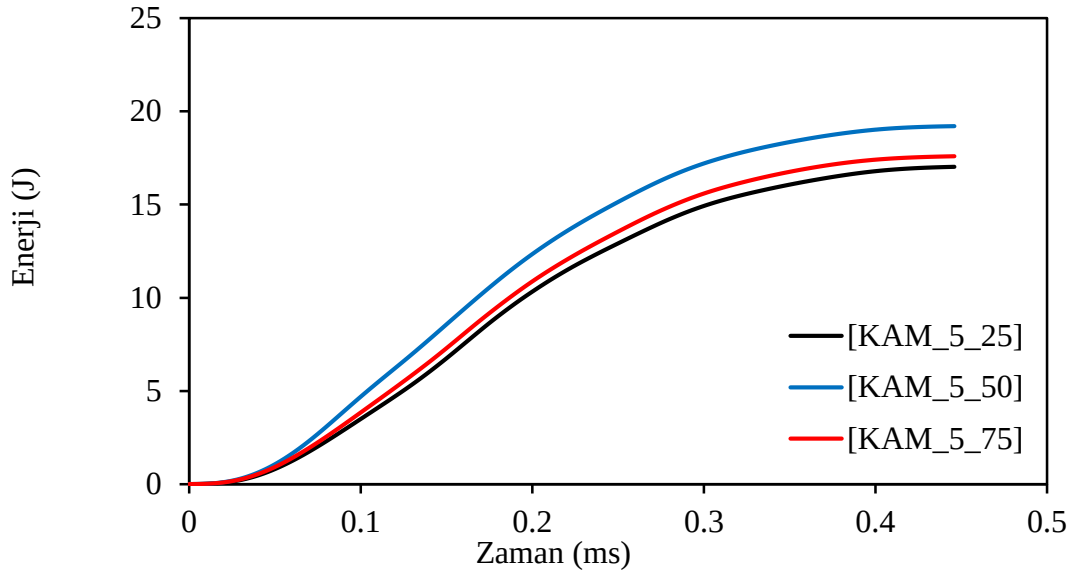
Şekil 6.38 Ortam ısisına göre %5 kam takviyeli kiriş numunelerinin enerji zaman grafiğı
