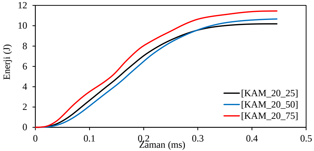
Şekil 6.41 Ortam ısisına göre %20 kam takviyeli kiriş numunelerinin enerji zaman grafiğı
