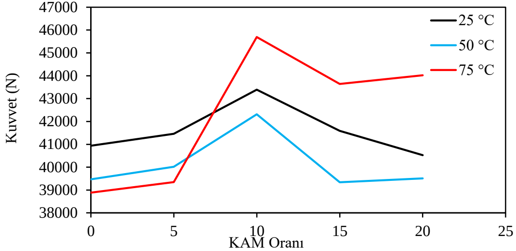
Şekil 6.36 Ortam ısisına göre kiriş numunelerde ağırlık düşürme deneyi sonrası oluşan maksimum tepki kuvvetinin kam miktarına göre değişimi
