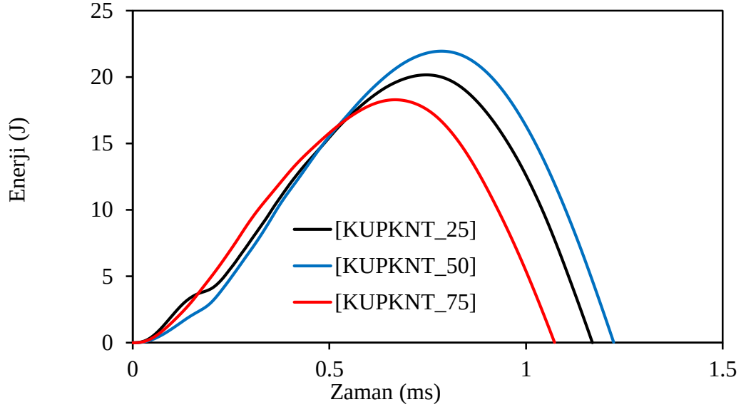
Şekil 6.23 Ortam ısisına göre kontrol küp numunelerinin enerji zaman grafiği
