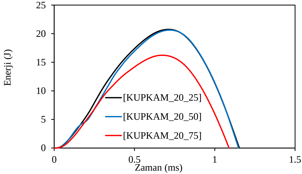
Şekil 6.27 Ortam ısisına göre %20 kam takviyeli küp numunelerinin enerji zaman grafiğı
