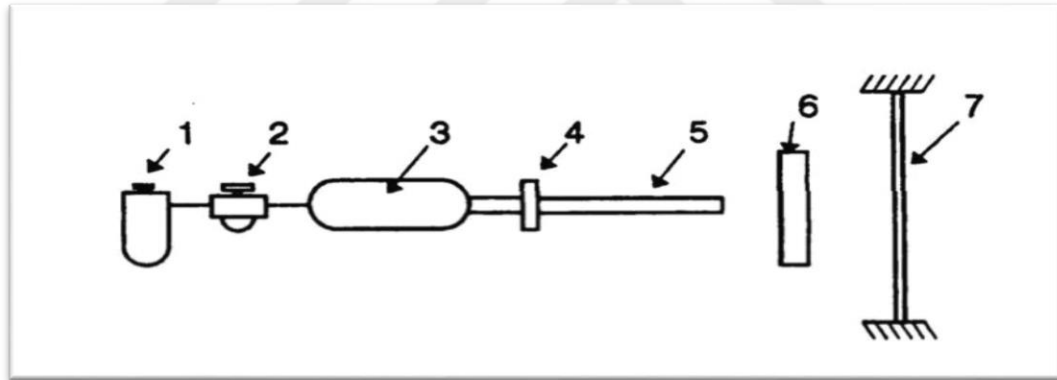
Şekil 4.4 Basınçlı hava ile darbe test düzeneğine ait şematik resim (1- hava filtresi, 2- basınç regülatörü, 3- hava tankı, 4- selenoid valf, 5- namlu (tüp), 6- hız sensörü, 7- numune) [49].
