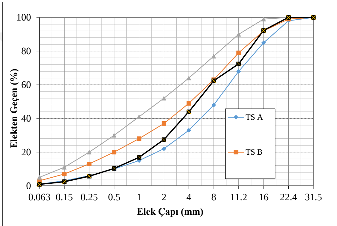
Şekil 5.1. Agreganın granülometri eğrisi
