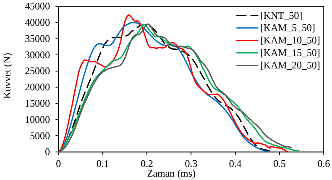
Şekil 6.29 50 °C ortam ısısı şartlarında ağırlık düşürme deneyine tabi tutulan kiriş numunelerin tepki kuvveti-zaman grafiği
