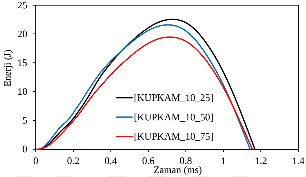
Şekil 6.25 Ortam ısisına göre %10 kam takviyeli k p numunelerinin enerji zaman grafiđi
