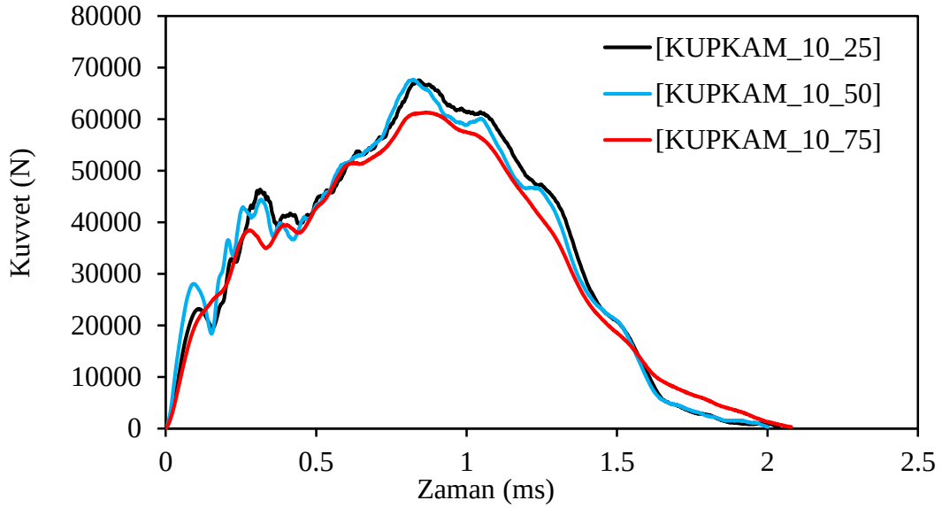
Şekil 6.19 %10 kazınmış asfalt ikameli numunelerin farklı ortam ısıları altında ağırlık düşürme deneyi sonrası oluşan tepki kuvveti-zaman grafiği
