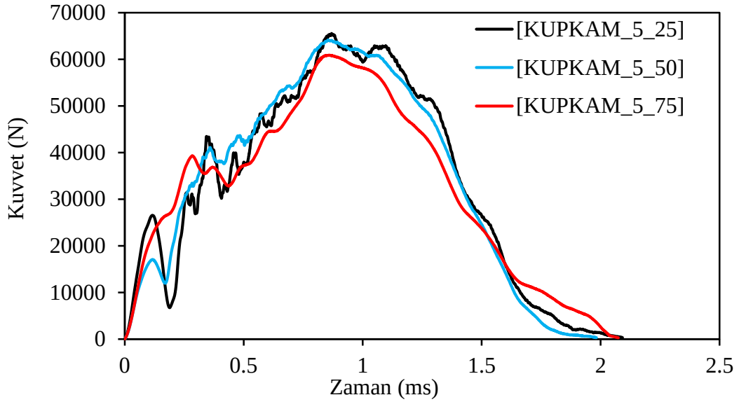
Şekil 6.18 %5 kazınmış asfalt ikameli numunelerin farklı ortam ısıları altında ağırlık düşürme deneyi sonrası oluşan tepki kuvveti-zaman grafiği
