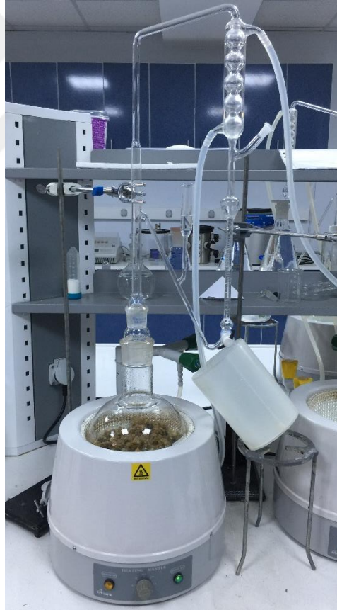
Şekil 3.5. Clevenger apareyi
