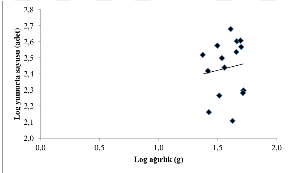
Şekil 10. Kerevitin ağırlığı ile yumurta sayısı arasındaki lineer regresyon
