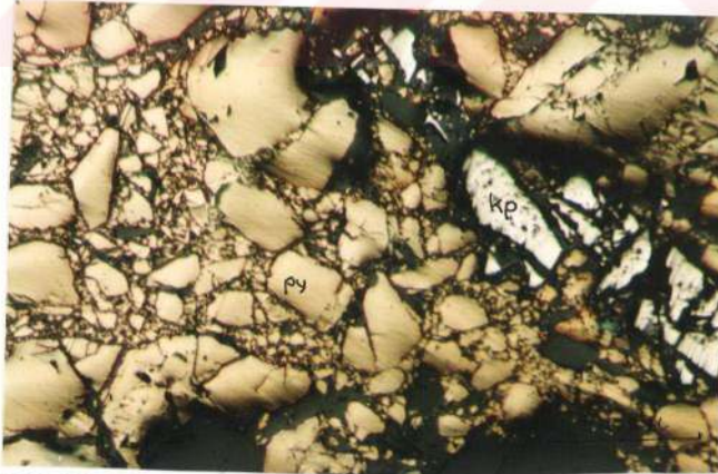
Şekil 5.4. Kalkopiritlerde gözlenen katakalastik doku, kp: kalkopirit, py: pirit, pt:pirotin (T.N., 100).
