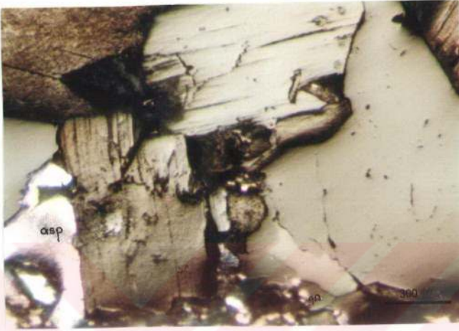
Şekil 5.7. Sfalerit ve galenle birlikte bulunan arsenoprit mineralleri. asp: arsenoprit, gn: galen, sf: sfalerit(T.N., 100).
