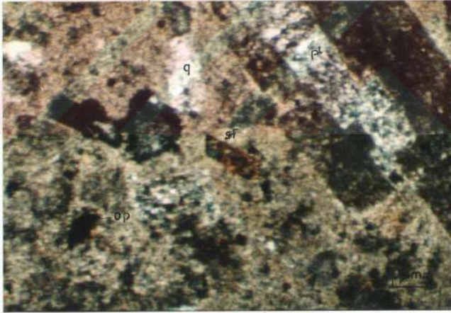
Şekil 4.6. İleri derecede serizitleşmiş magmatik kayaların mikroskopik görünüşü. pl: plajiyoklas, q: kuvars, op:opak min. s:serizitlemiş feldispat. Sf:sfen. (Ç.N. 32).
