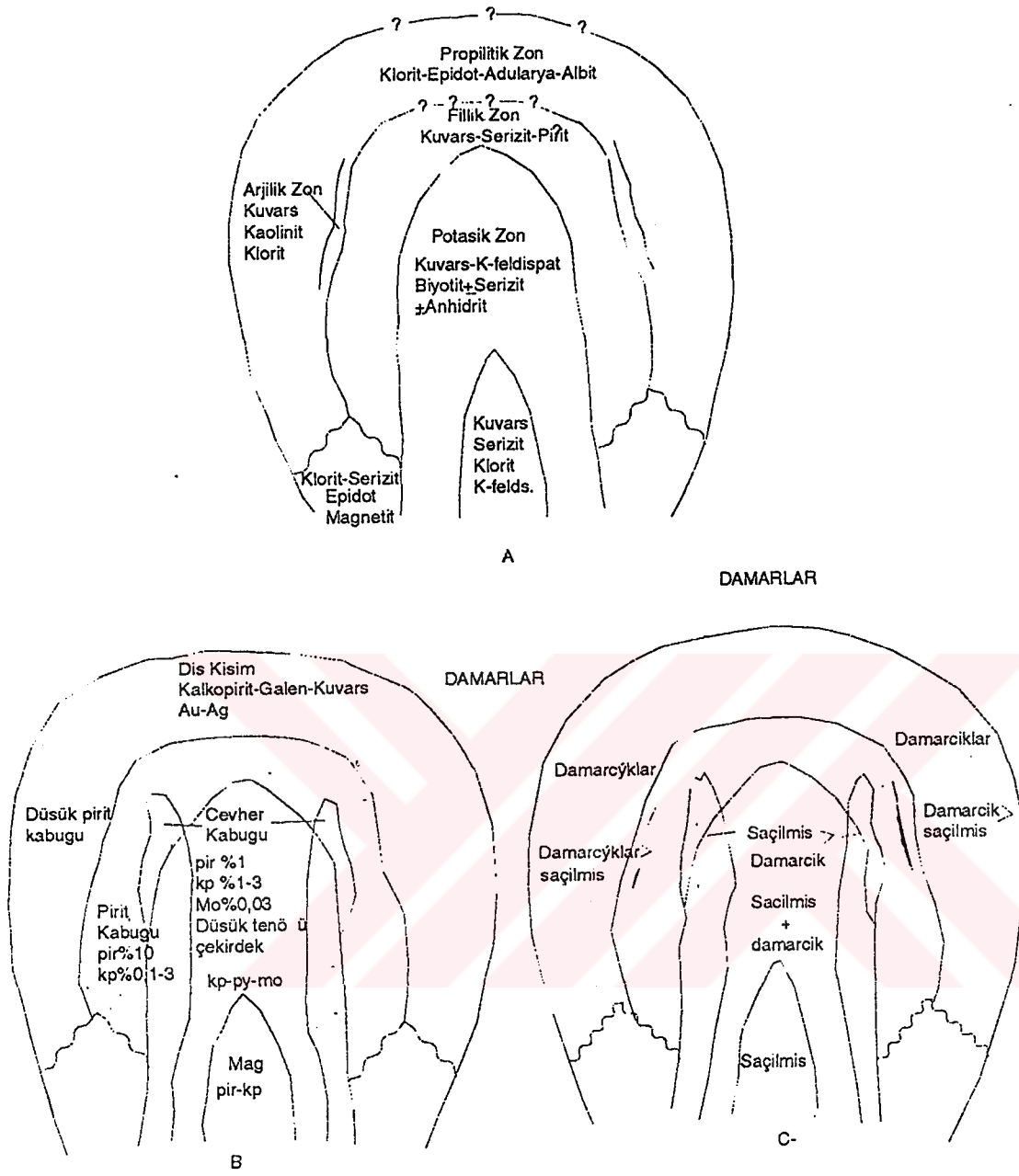
Şekil 9.1. Porfiri bakır yataklarında alterasyon, mineralleşme kuşakları (Erler, 1981'den).
