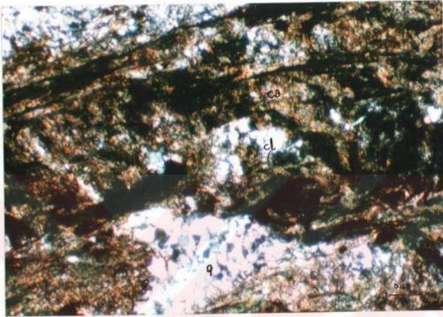
Şekil 4.3. Serizit şistlerin mikroskopik görünüşü. q: kuvars, s:serizit, cl:klorit, ca:kalsit, Ç.N.x32.
