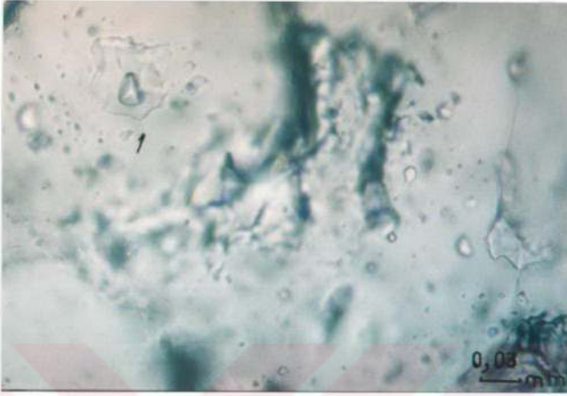
Şekil 6.1. Düzgün olmayan, parçalanmış I,tip sıvı kapanımlarının görünüşü (T.N., 50x10).
