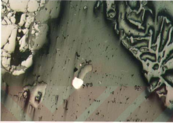
Şekil 5.13 Sfaleritler içerisinde pirit ve kalkopirit ornmatmaları, kp:kalkopirit, py, pirit, sf:sfalerit (T.N. ,100).
