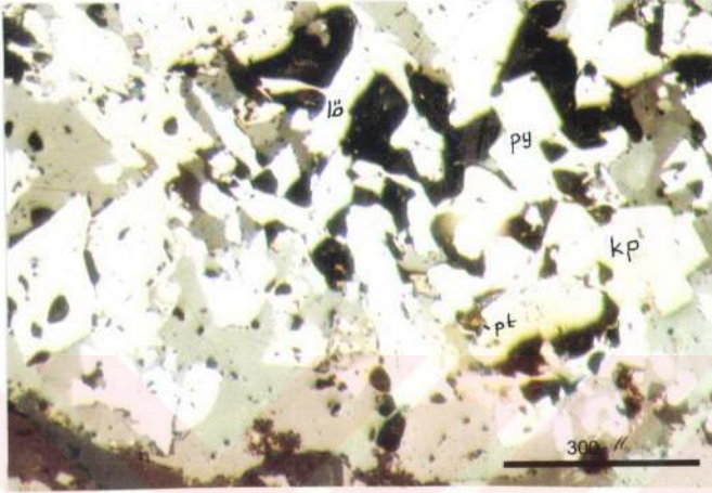
 ekil 5.9. Kalkopirit ile birlikte bulunan l linjitlerin yakından g r n   . l : l linjit kp: kalkopirit, py: pirit, pt: pirotin (T.N., 100).
