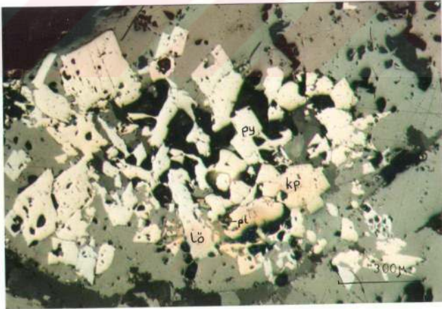
Şekil 5.8 Pirit pirotit dönüşümü. kp:kalkopirit, py: pirit, pt: pirotin, lö: löllingit (T.N., 100).
