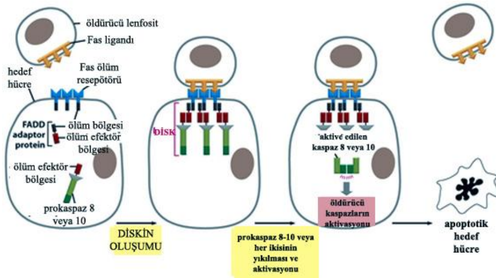
Şekil 1.6. Apoptozun hücre dışı uyarılarla uyarılması (Alberts ve ark. 2003).
