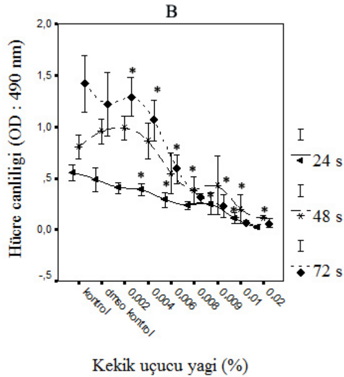
Şekil 3.1. Kekik uçucu yağının HepG2 hücre canlılığı üzerine etkisinin NR alınımlı (A), WST-1 (B) ve tripan mavisi boyaması (C) ile değerlendirilmesi. (*) işareti kontrol grubuna göre anlamlı farklılıkları göstermektedir. Anlamlılık değeri p < 0,001 .
