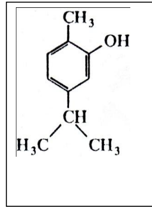
Çizelge 3.1. Origanum onites L. uçucu yağının ana bileşenlerinin GC analizi ile yapılmış sonuçları (A) ve karvakrolün kimyasal formülü (B).
