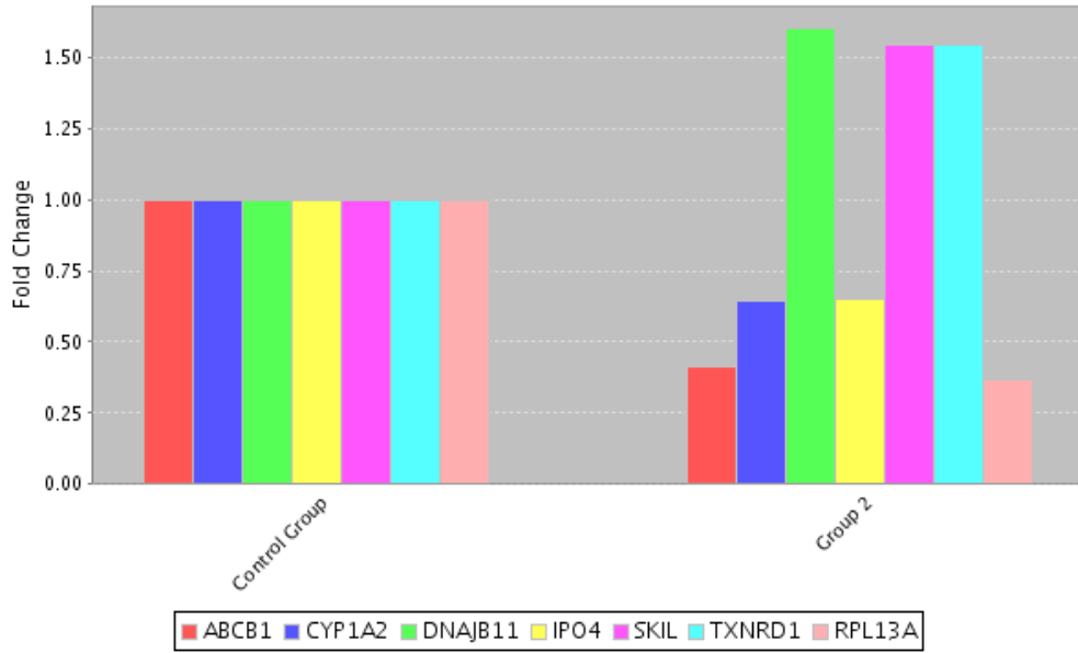
Şekil 3.16. Karvakrol ile HepG2 hücrelerinin muamelesi sonucu ifade seviyesi 1.5 kat ve üzeri değışen genlerin kontrolleri ile karşılaştırmalı olarak çoklu sütun grafiğinde gösterilmesi.
