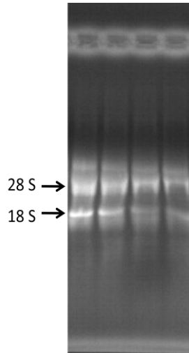
Şekil 3.8. Toplam RNA'nın formaldehit agaroz jel elektroforezi ile elde edilen bandların görüntüsü.
