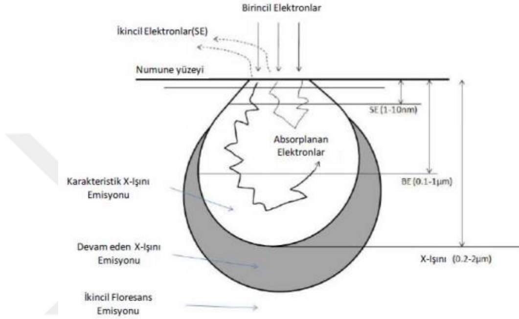
Şekil 3.7. SEM ‘de elektron demetinin numune ile etkileşim hacminin temsili gösterimi (Yaygıngöl, 2012).
