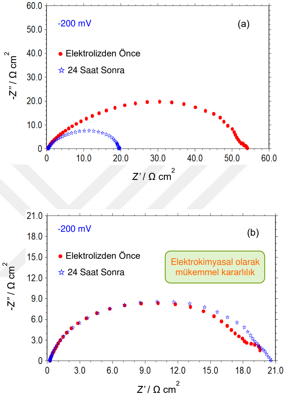
Şekil 4.29. Cu/pRd-SAM (a) ve pRd modifiye dilmiş Cu/pRd-SAM/Pd (b) elektrotların 6 M KOH çözeltisinde elektrolize başlamadan önce ve 24 saat elektrolizden sonra -200 mV katodik aşırı gerilimde elde edilen Nyquist eğrileri
