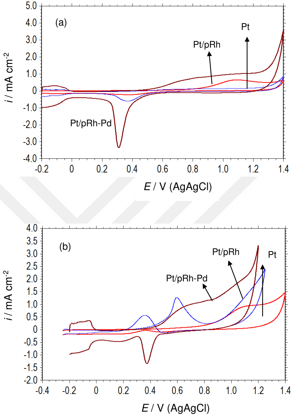
Şekil 4.31. Pt, Pt/pRh ve Pt/pRh-Pd elektrotların 1 \text{ M CH}_3\text{OH} içermeyen (a) ve içeren (b) 0.5 \text{ M H}_2\text{SO}_4 çözeltilerinde 298 \text{ K} 'de elde edilen dönüşümlü voltamogramları ( v : 100 \text{ mV s}^{-1} )
