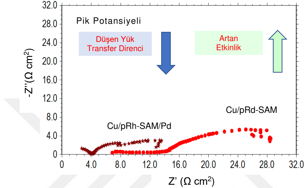
Şekil 4. 36. Cu/pRd-SAM ve Cu/pRh-SAM/Pd elektrotların 1 M CH 3 OH + 0,1 M KOH çözeltisinde 298 K'de metanolün yükseltgenmesine karşılık gelen ve CV eğrilerinden belirlenen metanol pik potansiyellerinde elde edilen Nyquist eğrileri
