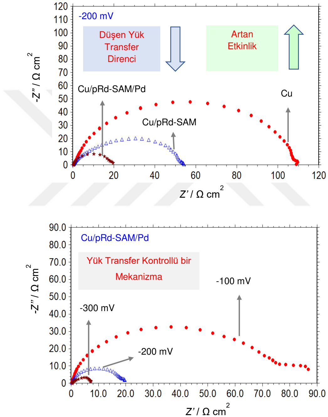
Şekil 4.26. Cu, pRd-SAM modifiye edilmiş Cu ve pRd-SAM/Pd modifiye edilmiş Cu elektrotların 6 M KOH çözeltisinde -200 mV aşırı gerilimde elde edilen Nyquist eğrileri (a), pRd-SAM/Pd modifiye edilmiş Cu elektrotun değişik aşırı gerilimlerde elde edilen Nyquist eğrileri
