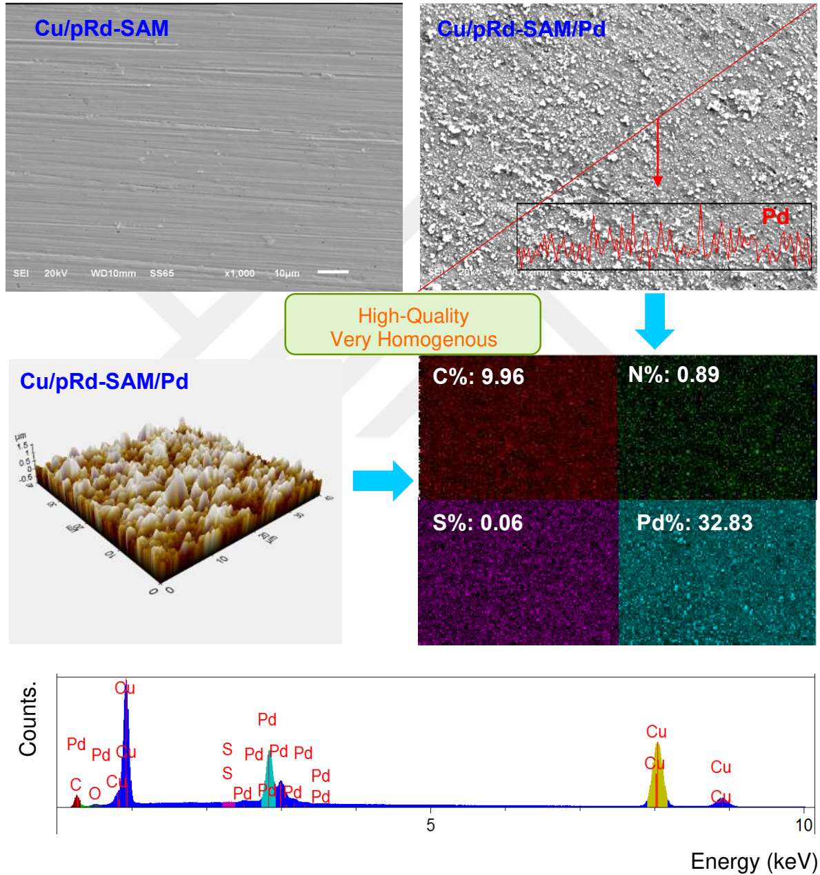
Şekil 4.16. pRd-SAM modifiye edilmiş Cu yüzeyinin SEM görüntüsü, Pd çöktürülmüş pRd-SAM/Pd modifiye edilmiş Cu yüzeyinin SEM ve AFM görüntüleri, polimer yapısında bulunan bazı elementlerin yüzeydeki dağılımları (EDX-haritalama görüntüleri) ve Cu/pRd-SAM/Pd yüzeyinin EDX spektrumu
