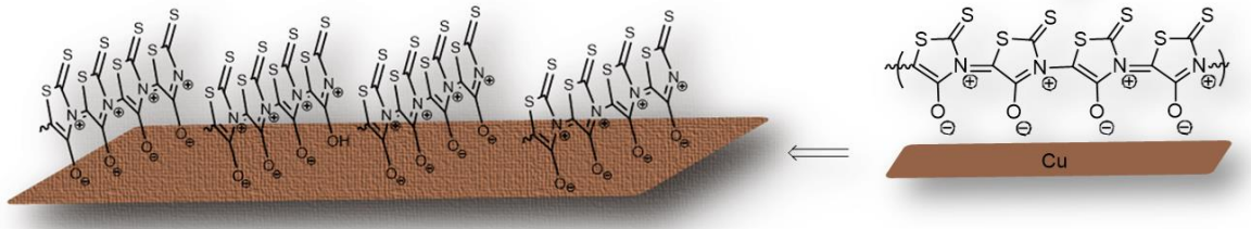
Şekil 4.7. pRd'nin bakır yüzeyine adsorpsiyon mekanizmasının şematik olarak gösterimi (Solmaz, 2018)
