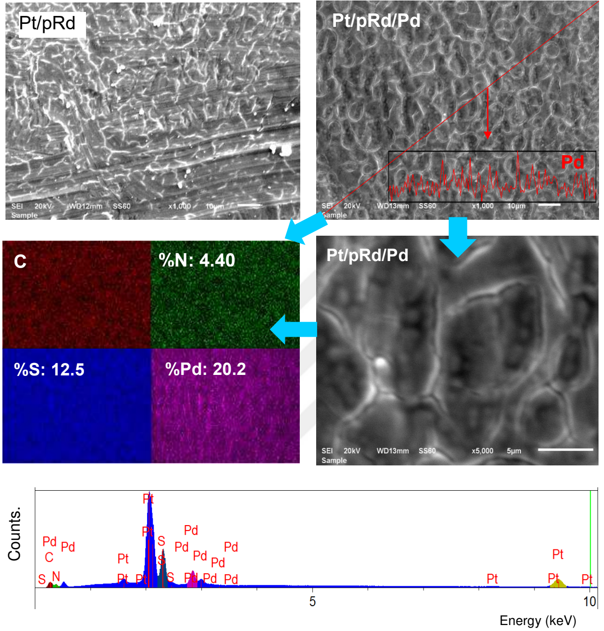
Şekil 4.11. pRd ve pRh/Pd modifiye edilmiş Pt yüzeylerinin değişik büyütmelerde alınmış SEM görüntüleri, Pd metalinin yüzey boyunca değişimi; C, N, S ve Pd elementlerin yüzeydeki dağılımları (Pd-modifiye edilmiş polimer filmin yüzeydeki EDX-haritalama görüntüleri) ve Pt/pRd/Pd yüzeyinin EDX spektrumu
