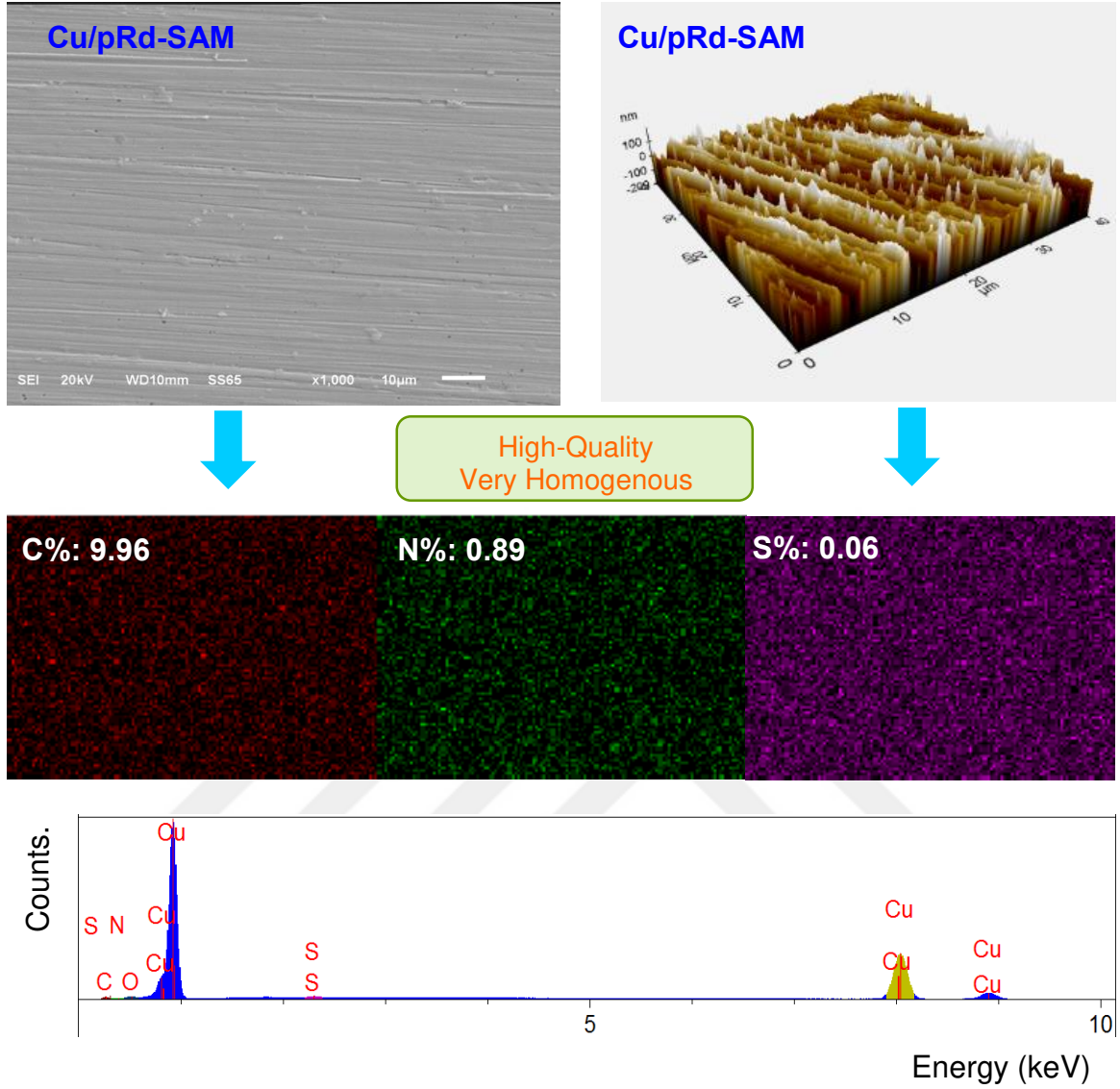
Şekil 4.15. pRd-SAM modifiye edilmiş Cu yüzeyinin SEM ve AFM görüntüleri, polimer yapısında bulunan bazı elementlerin yüzeydeki dağılımları (EDX-haritalama görüntüleri) ve Cu/pRd-SAM yüzeyinin EDX spektrumu
