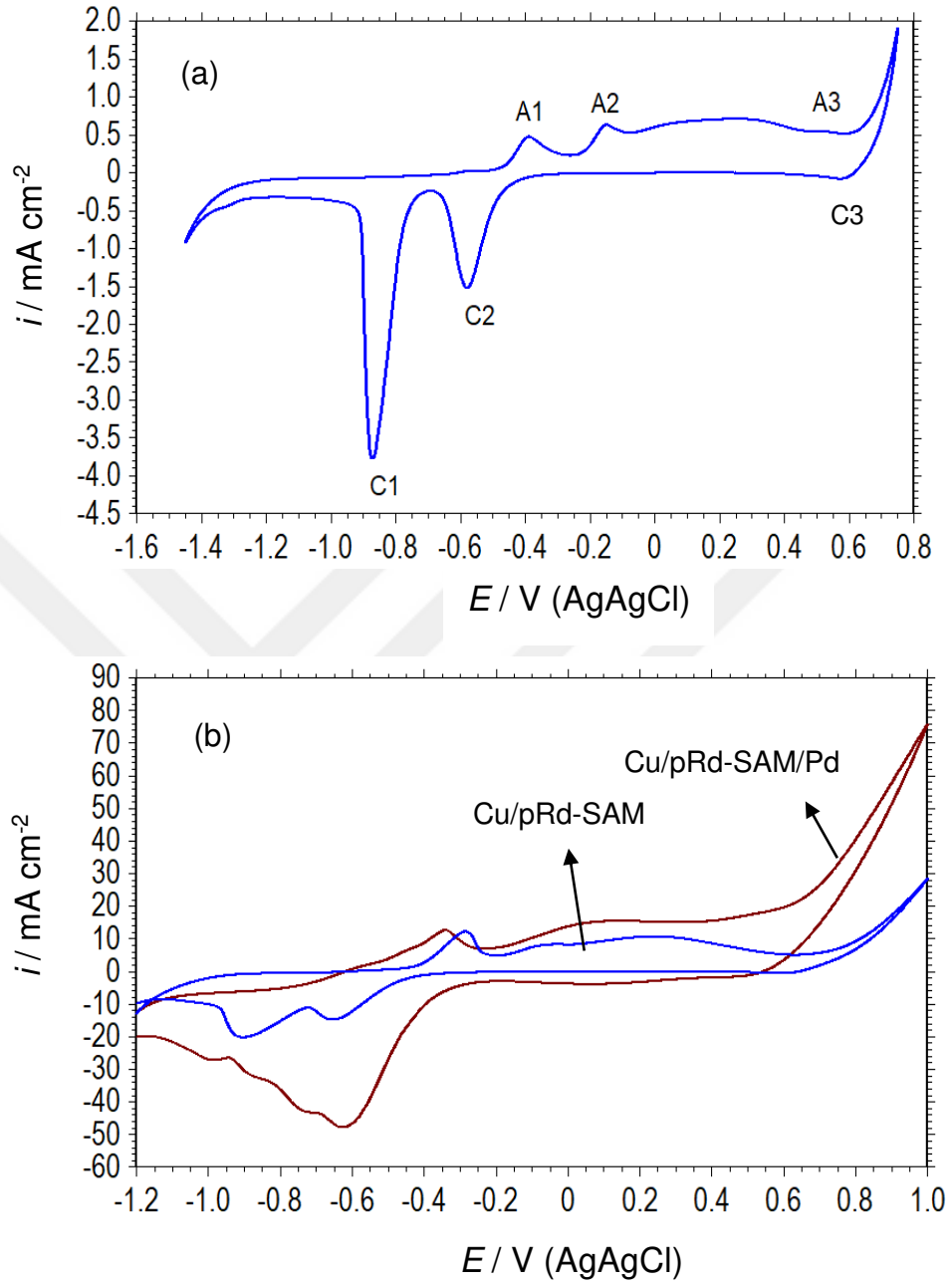
Şekil 4.34. Cu (a), Cu/pRd-SAM ve Cu/pRd-SAM/Pd (b) elektrotların 0,1 M KOH çözeltilerinde 298 K’de elde edilen dönüşümlü voltamogramları ( v : 100 mV s -1 )
