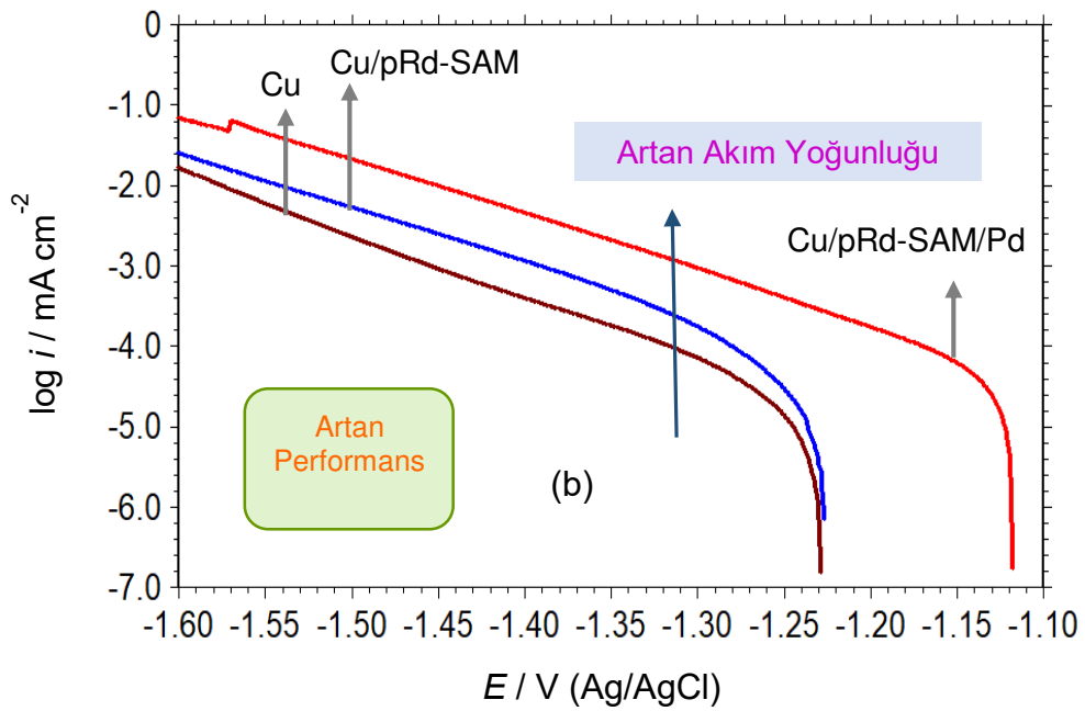
Şekil 4.25. Cu, pRd-SAM modifiye edilmiş Cu ve pRd-SAM/Pd modifiye edilmiş Cu elektrotların 6 M KOH çözeltisinde 298 K’de elde edilen E - i (a) ve yarı logaritmik katodik akım-potansiyel eğrileri (b)
