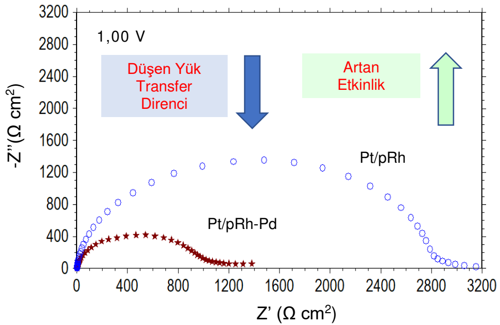
Şekil 4.32. Pt/pRd ve Pt/pRd/Pd elektrotların 1 M \text{CH}_3\text{OH} + 0,5 M \text{H}_2\text{SO}_4 çözeltisinde metanolün yükseltgenmesine karşılık gelen +1,00 V potansiyelde elde edilen Nyquist eğrileri
