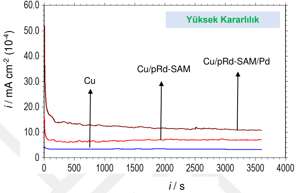
Şekil 4.37. Cu, Cu/pRd-SAM ve Cu/pRd-SAM/Pd elektrotların 1 M \text{CH}_3\text{OH} + 0,1 M KOH çözeltisinde 298 K'de metanolün yükseltgenmesine karşılık gelen ve CV eğrilerinden belirlenen metanol pik potansiyellerinde akım yoğunluğunun zamanla değişimi
