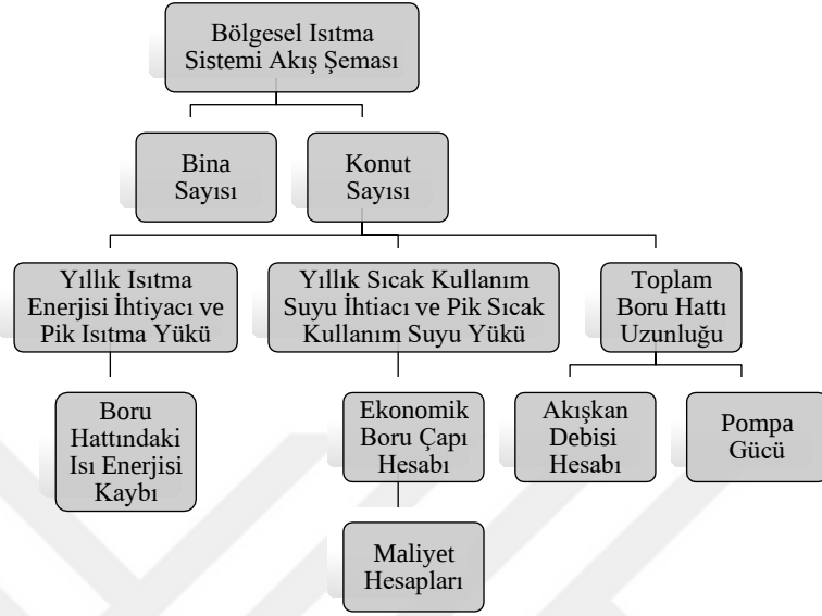
Şekil 2.15. Bölgesel Isıtma Sistemi Hesap Akış Şeması
