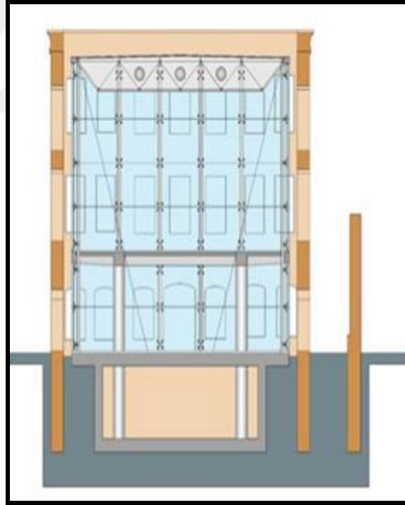
Şekil 5.26. Esmâ Sultan Yalısı Section Kaynak: Gökhan Avcıoğlu&CAD
