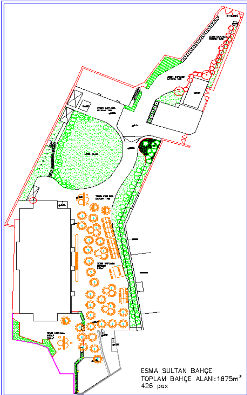
Şekil 5.22. Esma Sultan Yalısı Vaziyet Planı
