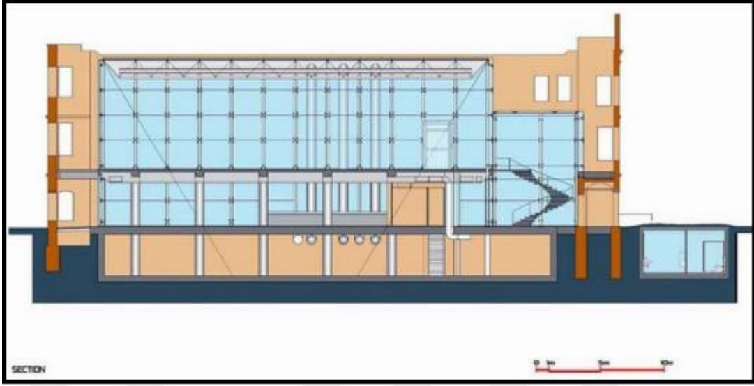
Şekil 5.25. Esmâ Sultan Yalısı Section Kaynak: Gökhan Avcıoğlu&CAD
