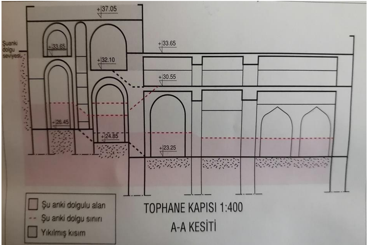
Lev. 18- Tophane Kapısı A kesiti
