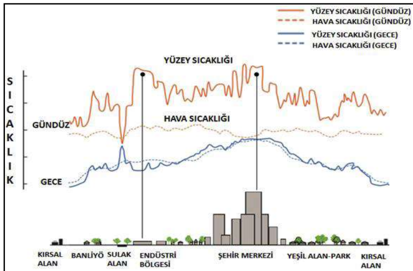
Şekil 2.8. Yüzey ve atmosferik sıcaklık değişimleri (EPA, 2008)
