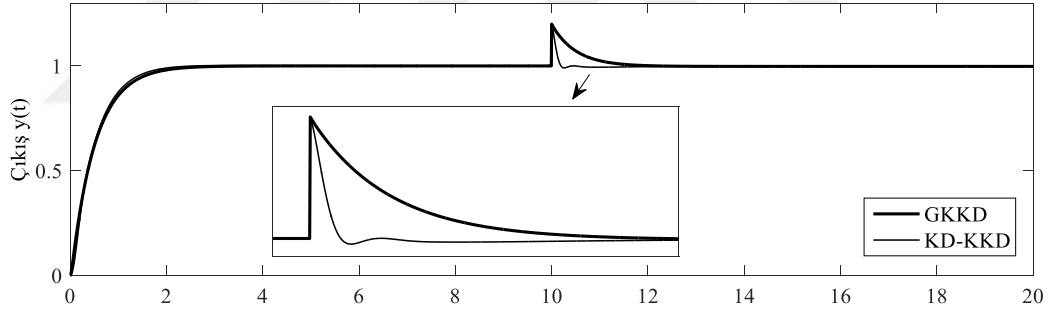
Şekil 4.22. Bozucu durumunda sistemin birim basamak cevabı ( \alpha_0 = -0.41, \alpha_1 = -0.4, \beta_0 = 0.2 )
