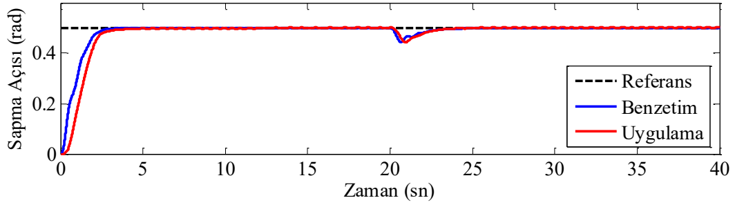
Şekil 4.34. Bozucu etkinin olduğu durum için sapma açısı cevabı
