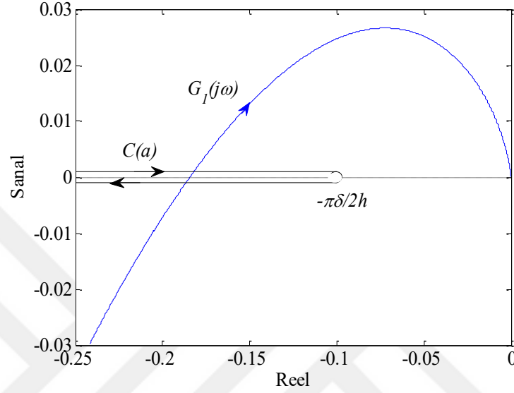
Şekil 4.104. K = 1 için G_6(j\omega) ve C(a) ’ya ait Tsypkin Eğrisi
