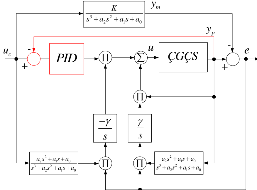
Şekil 4.66. İleri ve geri beslemeli MRUD yapısı
