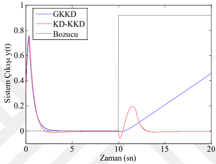
Şekil 4.16. GKKD ve KD-KKD için sistem çıkışı ve bozucu giriş
