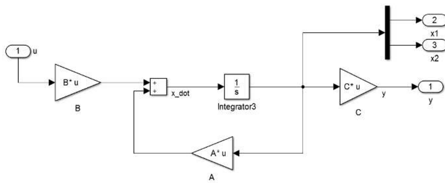
“Sistem” bloğunun iç yapısı
