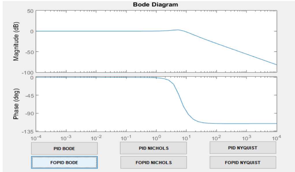
Şekil 7.14 Kesir Dereceli PI^\lambda D^\mu için Bode Analizi
