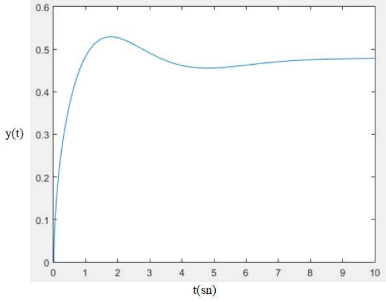
Şekil 6.6 Kapalı Çevrim Sistemim Birim Basamak Cevabı (Ziegler Nichols)
