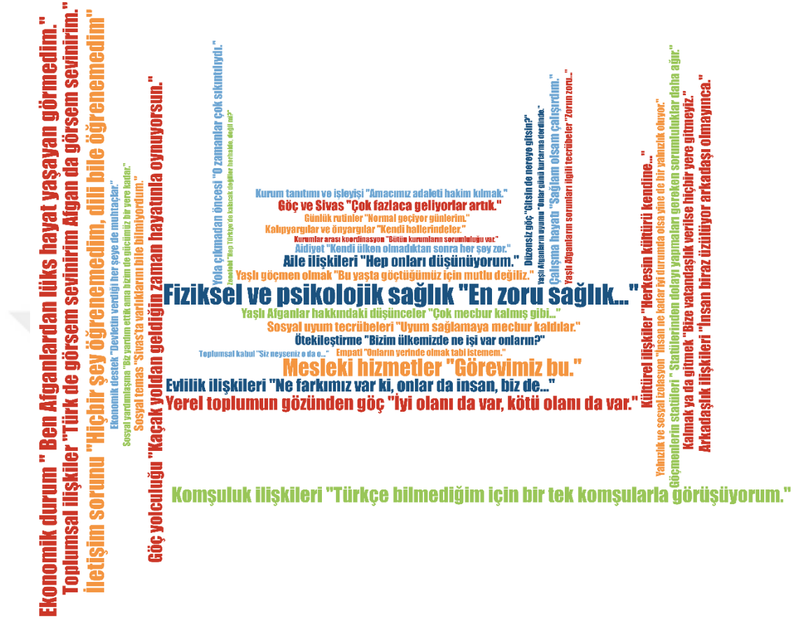
Şekil 4.2. Kod bulutu
