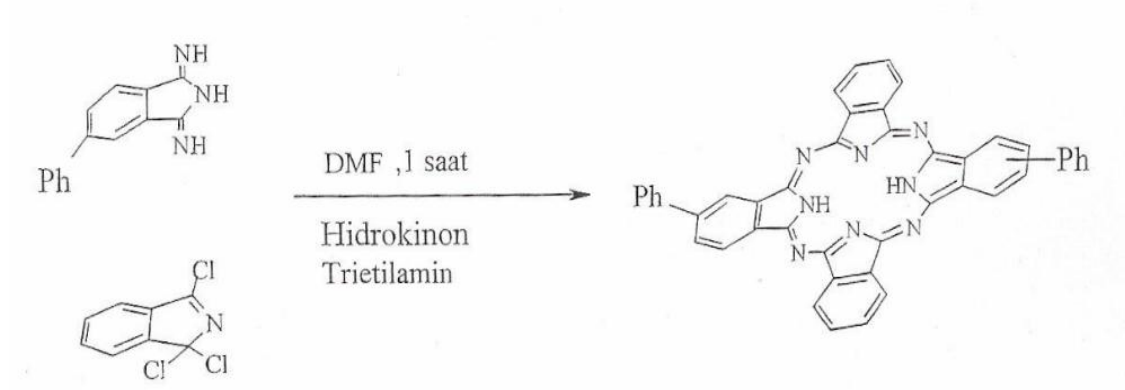
Şekil 1.20. 2,16- ve 2,17-difenil ftalosiyaninlerin sentezi.
