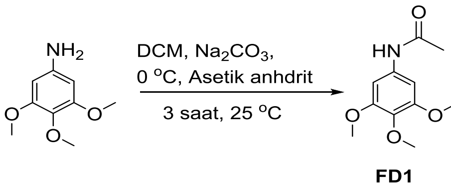
Şekil 3.1. N-(3,4,5-trimetoksifenil)asetamit (FD1) bileşiğinin sentezi.
