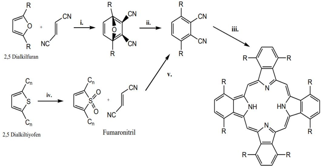
Şekil 1.19. Non-periferel Okta-süstitüe ftalosiyeninlerin sentezi ( H_2Pc-onp-C_n ).
