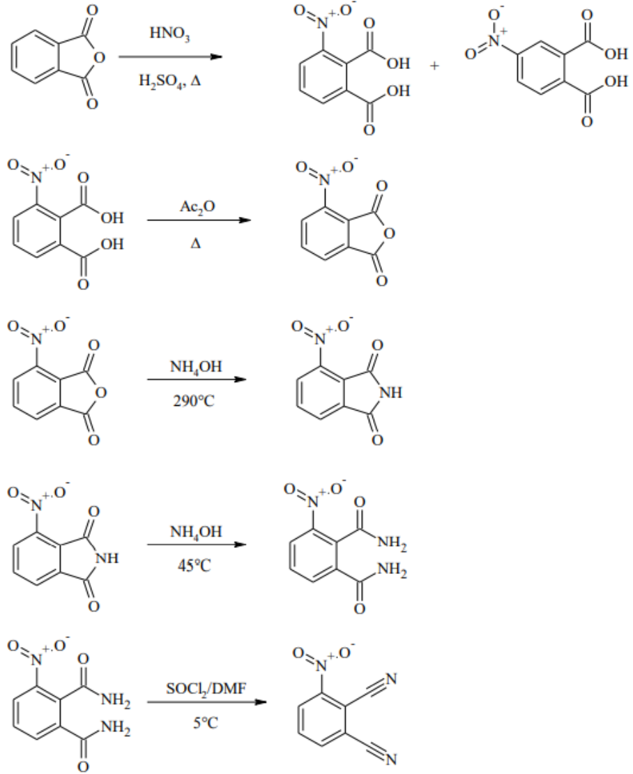
Şekil 1.17. ZnPc ve MnPc bileşiklerinin fotofiziksel özellikleri 3-Nitroftalonitril sentezi.
