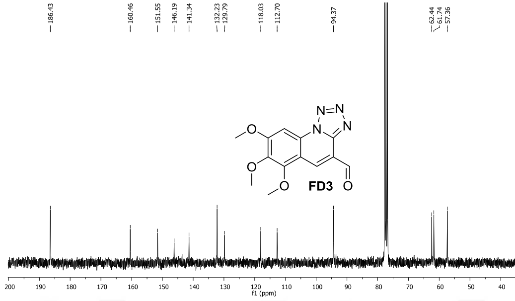
Şekil 4.6. FD3 bileşiğinin ^{13}\text{C} NMR spektrumu (75 MHz, \text{CDCl}_3 ).
