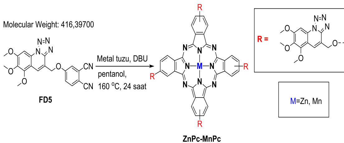
Şekil 3.6. Fitalosiyanın bileşiklerinin sentezi (ZnPc ve MnPc) .
