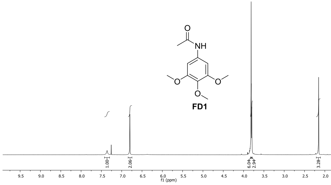
Şekil 4.1. FD1 bileşiğinin 1 H NMR spektrumu (300 MHz, CDCl 3 ).
