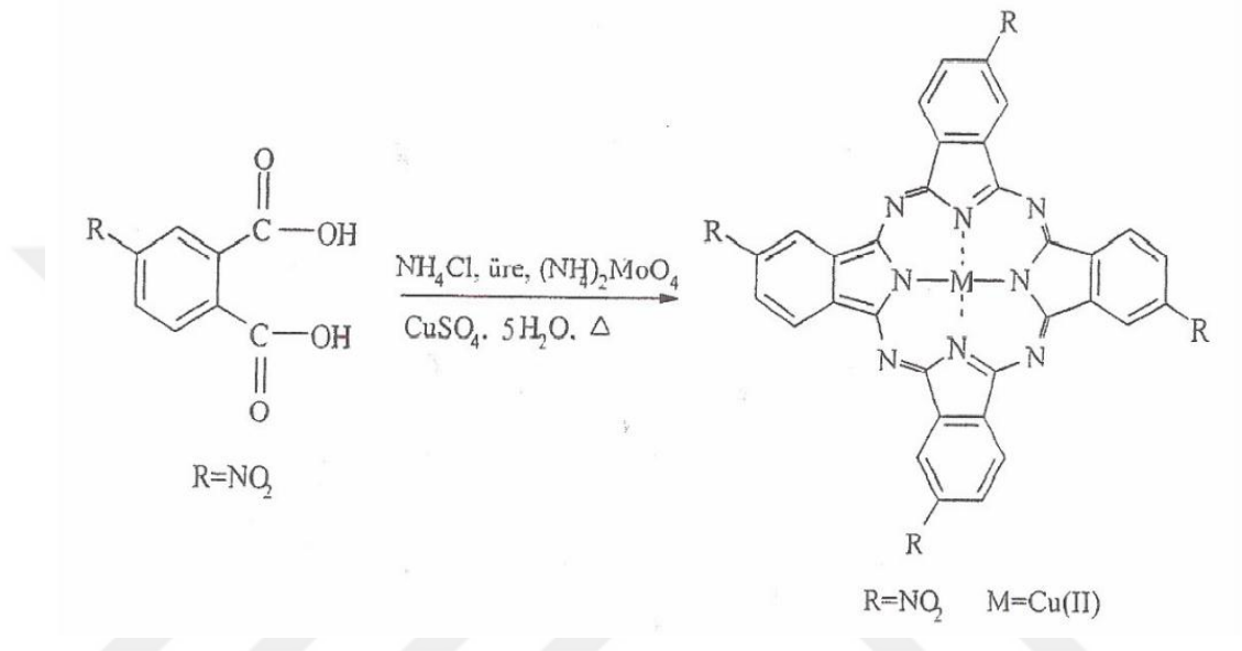
Şekil 1.25. 4-sübstitüe ftalik asitten ftalosiyanin sentezi.
