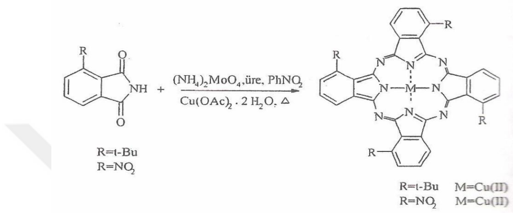
Şekil 1.28. Ftalimidden ftalosiyanın sentezi.
