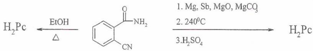
Şekil 1.23. o-sianobenzamid kullanılarak ftalosiyanin sentezi.
