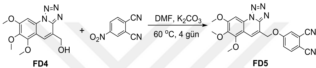
Şekil 3.5. 4-((6,7,8-trimetoksitetrazolo[1,5-a]kinolin-4-il)metoksi)ftalonitril ( FD5 ) bileşiğinin sentezi.
