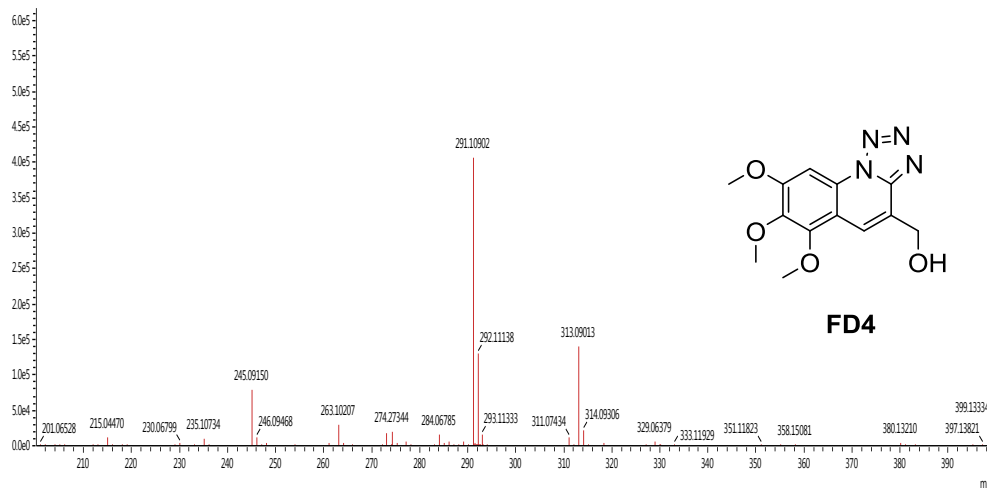
Şekil 4.10. FD4 bileşiğinin LC-MS spektrumu.
