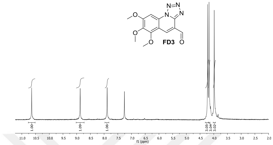
Şekil 4.5. FD3 bileşiğinin 1 H NMR spektrumu (300 MHz, CDCl 3 ):
