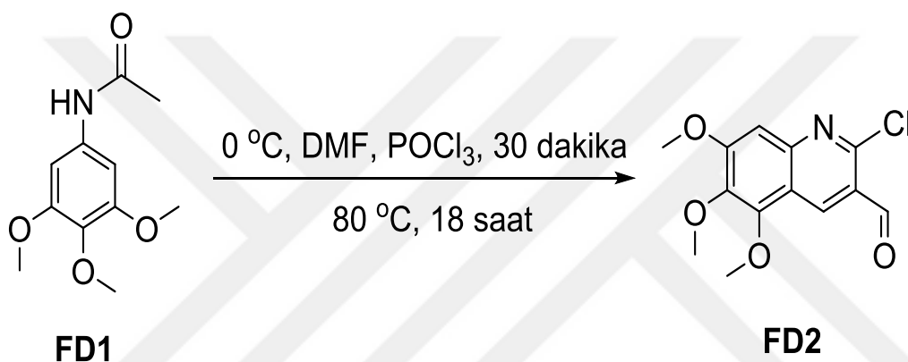
Şekil 3.2. 2-kloro-5,6,7-trimetoksikinolin-3-karbaldehit (FD2) bileşiğinin sentezi.
