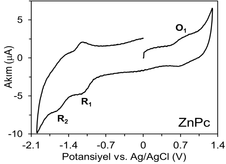
Şekil 4.24. 0.1 M TBAPF 6 içeren DMSO çözücüsündeki ZnPc bileşiğinin camısı karbon elektrot (GCE) üzerinde 100 mV s -1 tarama hızında alınmış dönüşümlü voltamogramı.
