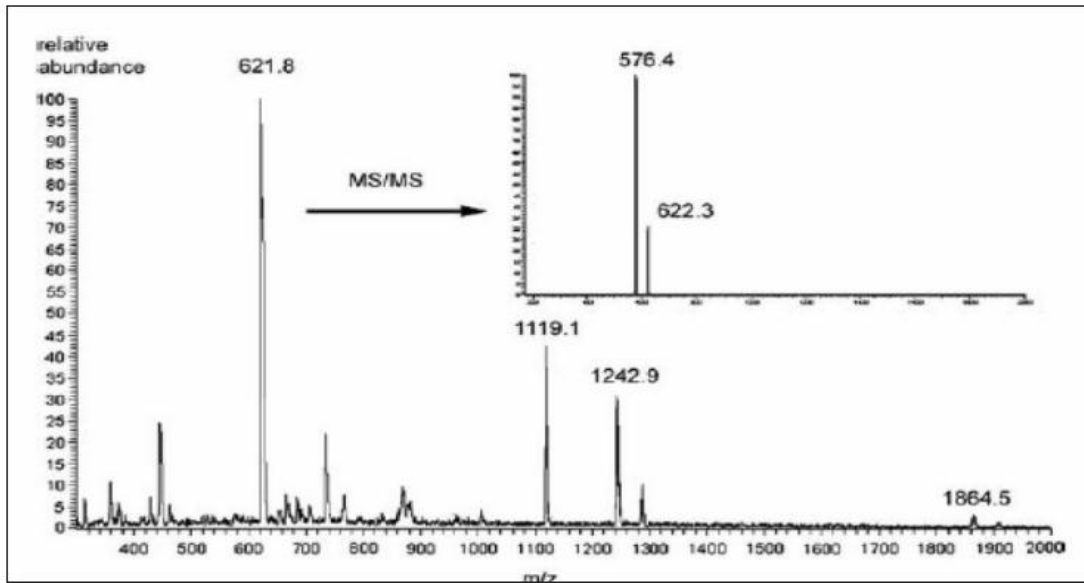
Şekil 2.5. 2-Karboksiftalosiyenin çinko (II) nin kütle spektrumu.
