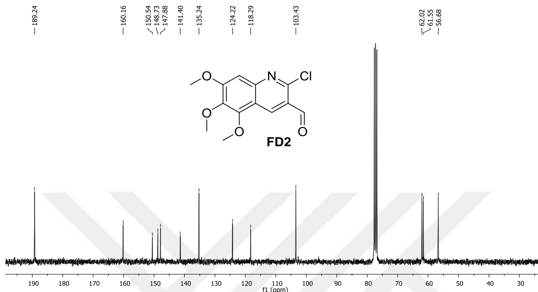
Şekil 4.4. FD2 bileşiğinin ^{13}\text{C} NMR spektrumu (75 MHz, \text{CDCl}_3 ).
