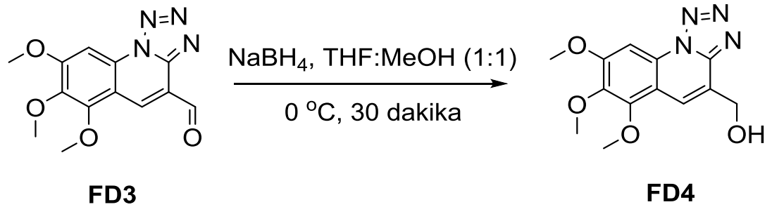
Şekil 3.4. (6,7,8-trimetoksitetrazolo[1,5-a]kinolin-4-il)metanol bileşığının sentezi.
