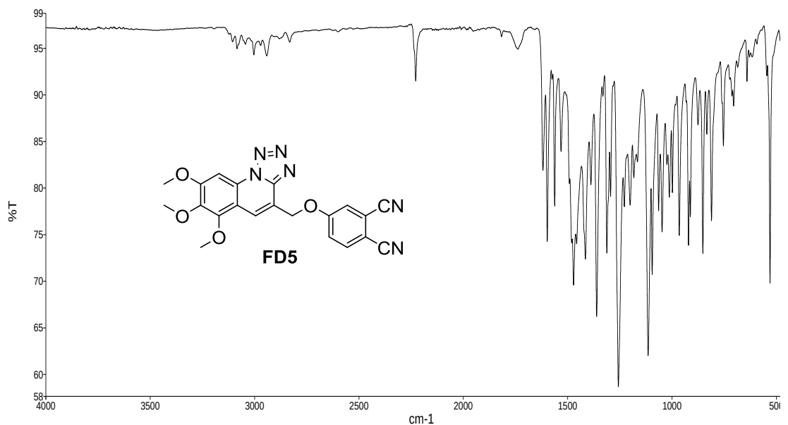
řekil 4.11. FD5 bileřiđinin FT-IR spektrumu (cm -1 ).
