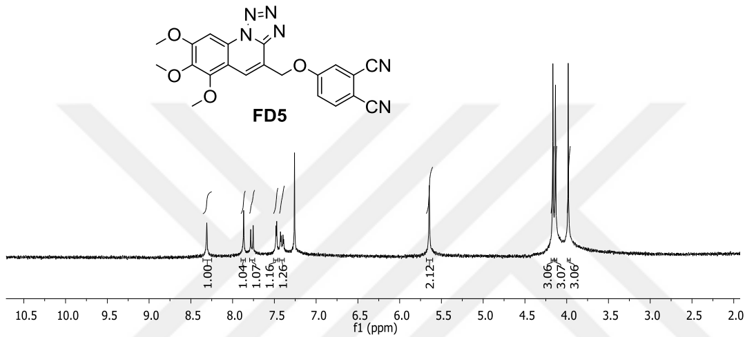
Şekil 4.12. FD5 bileşiğinin ^1\text{H} NMR spektrumu (300 MHz, \text{CDCl}_3 ).
