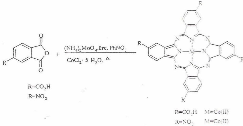
Şekil 1.26. Ftalikanhidritten ftalosiyanın sentezi.
