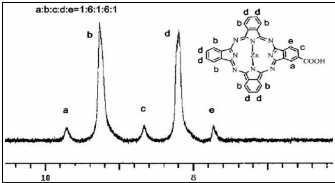
Şekil 2.4. 2-Karboxilftalosiyaniçinko (II) nin proton NMR spektrumu.
