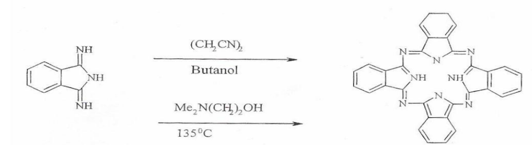
Şekil 1.29. 1,3-diiminoizindolin kullanılarak ftalosiyanın sentezi.
