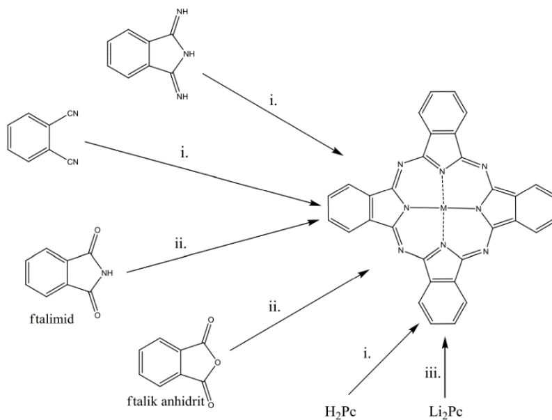
Şekil 1.14. M-ftalosiyenin sentez şeması: ham maddeler ve koşullar, i. Kinolin gibi yüksek kaynama noktalı bir çözücü içinde bir metal tuzu ile ısıtma, ii. üre ve bir metal tuzu ile yüksek kaynama noktasına sahip bir solvent içinde ısıtma, iii. metal tuzu içeren etanol içinde ısıtma.
