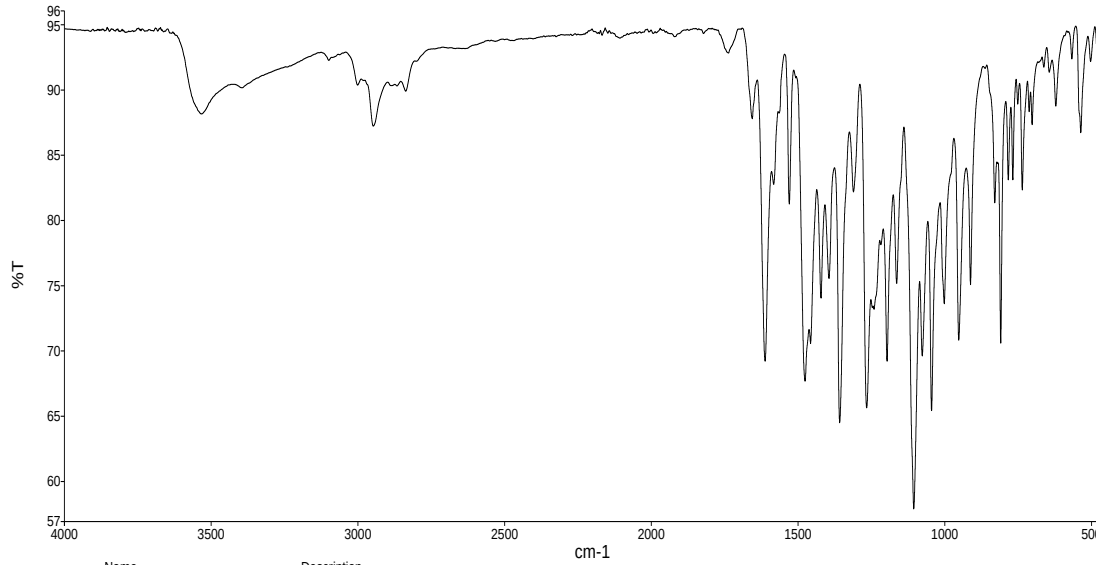
Şekil 4.7. FD4 bileşiğinin FT-IR spektrumu (cm -1 ).
