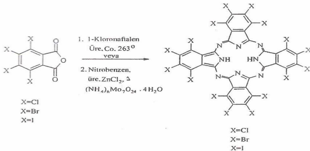
Şekil 1.27. Perhalosüstitüe ftalikanhidritten ftalosiyanın sentezi.
