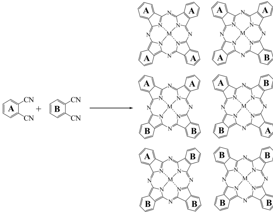
Şekil 1.21. İki farklı başlangıç maddesinden asimetrik ftalosiyaninlerin sentezi.
