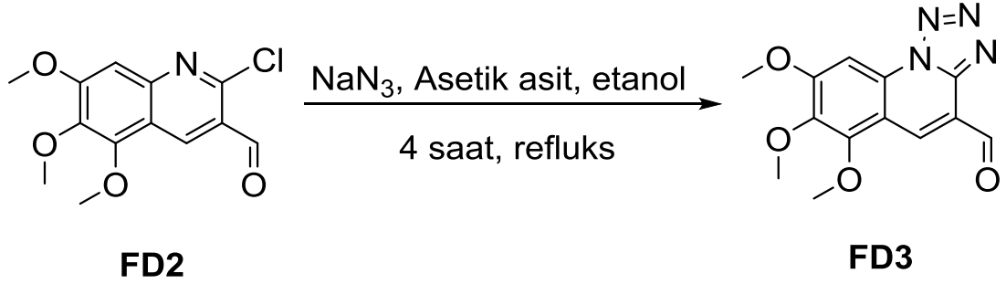
Şekil 3.3. 6,7,8-trimetoksitetrazolo[1,5-a]kinolin-4-karbaldehit bileşığının sentezi.
