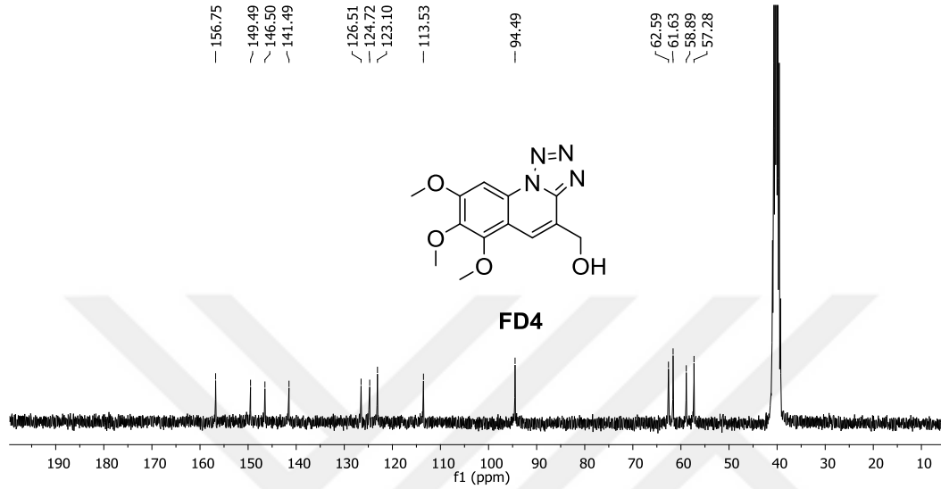
Şekil 4.9. FD4 bileşiğinin 13 C NMR spektrumu (75 MHz, DMSO-d 6 ).
