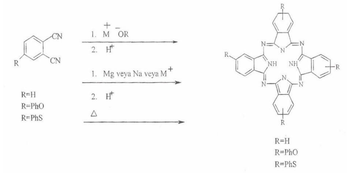
Şekil 1.24. Ftalonitril kullanılarak ftalosiyanin sentezi.
