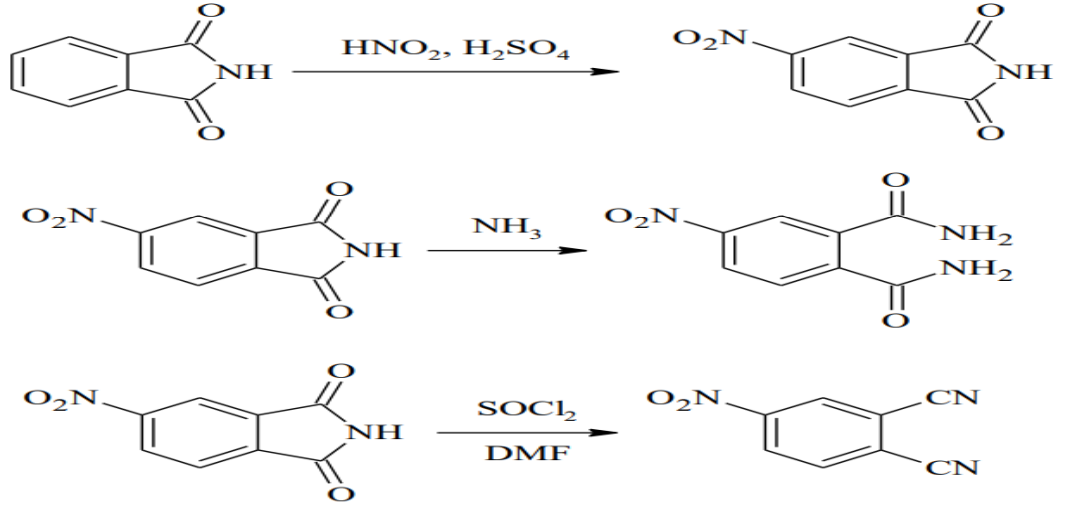
Şekil 1.15. 4-Nitroftalonitril sentezi.
