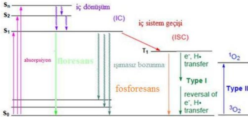
Şekil 1.38. Işımlar.
