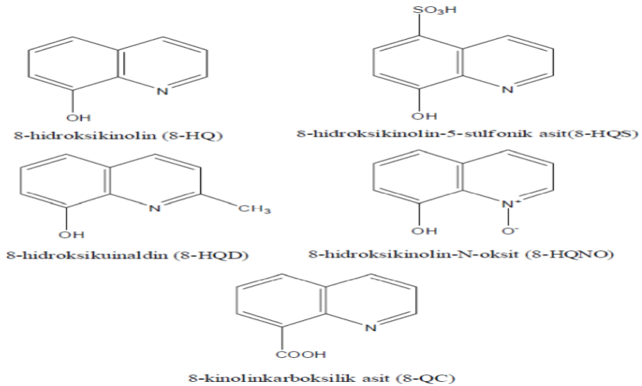
Şekil 1.54. Kinolin türevleri.
