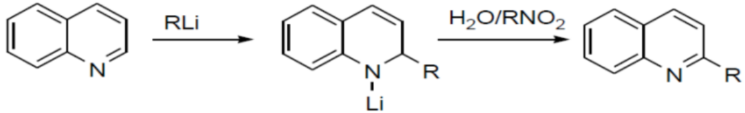
Şekil 1.52. Kinoline yükseltgeme.
