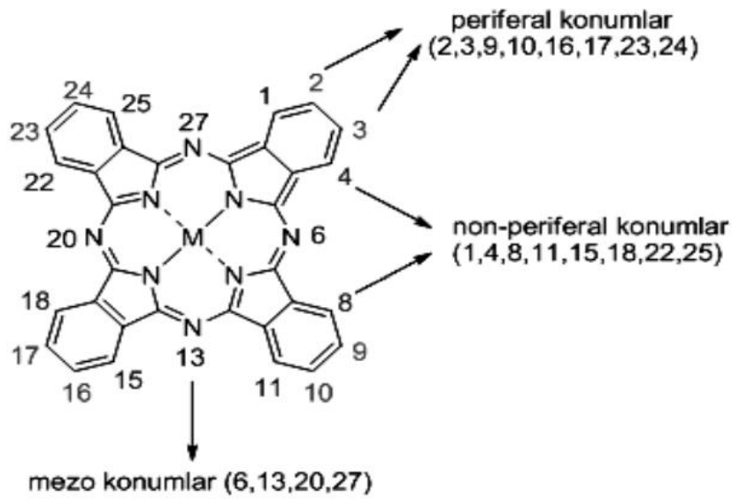
Şekil 1.9. Ftalosiyaninin numaralandırmasında kabul edilen sistemdir.
