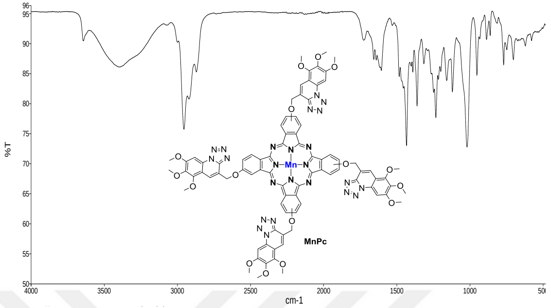
Şekil 4.16. MnPc bileşiğinin FT-IR spektrumu (cm -1 ).
