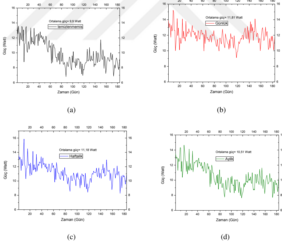
Şekil 5.18. Yatay panellerin güç-zaman grafikleri.
