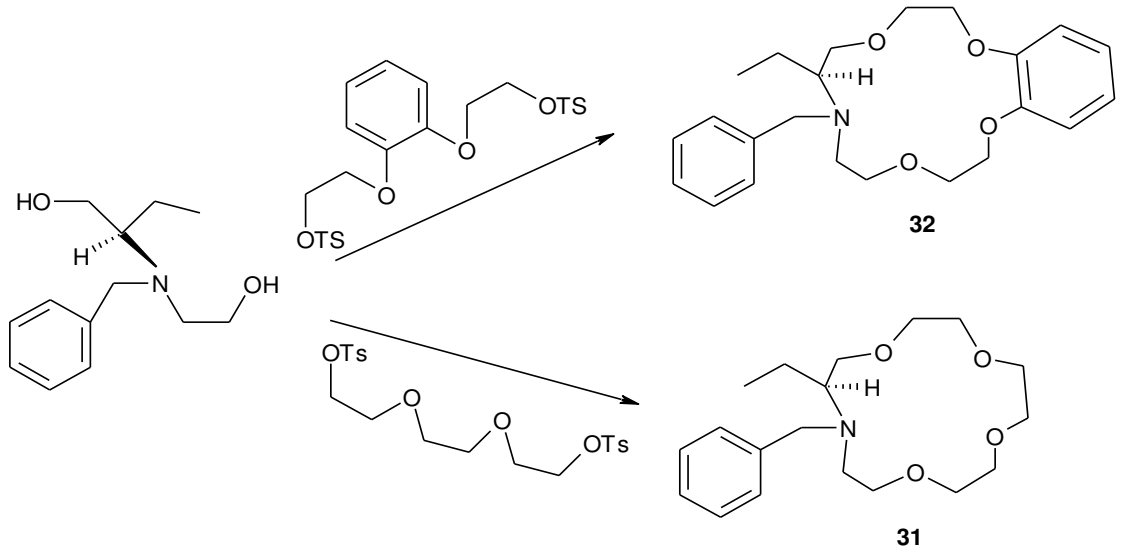
Şekil 2.19. Ditosilat ile amino alkol halkalaşması
