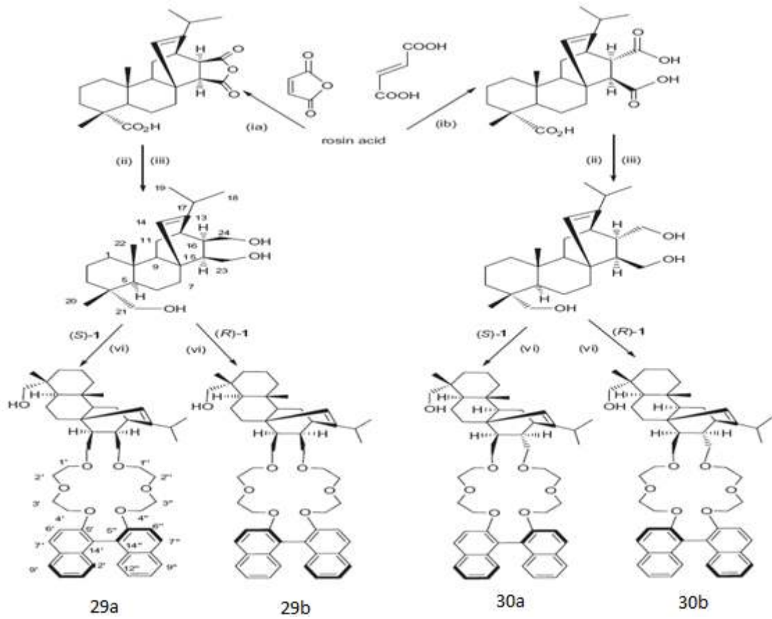
Şekil 2.18. (i) 1a 140°C, 1b 200°C, 3 saat; (ii) \text{PCl}_3 sonra \text{MEOH} , riflaks, 4 saat; (iii) \text{LiAlH}_4 , \text{Et}_2\text{O} , riflaks, 8 saat; (vi) \text{NaH} , 1, THF, 50 saat.
