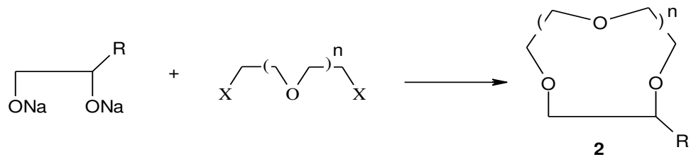
Şekil 2.4. Süstitüe etilen glikol ile C-Pivot lariat eterlerin hazırlanması
