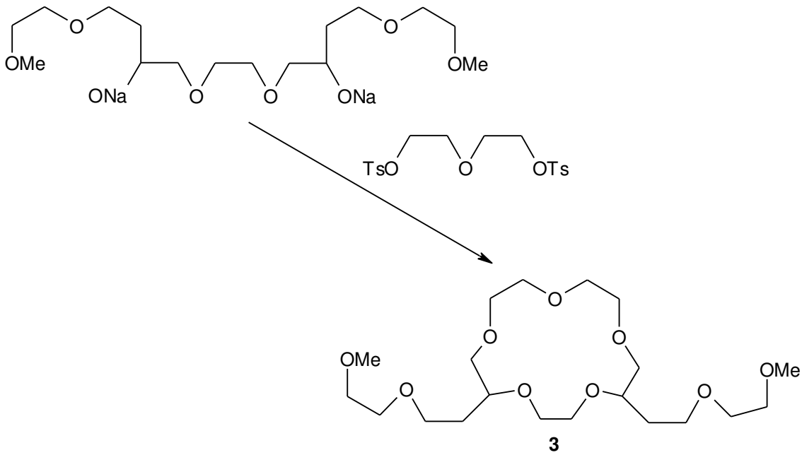
Şekil 2.5. Sübstitüe etilen glikol ile C-Pivot lariat eterlerin hazırlanması-2
