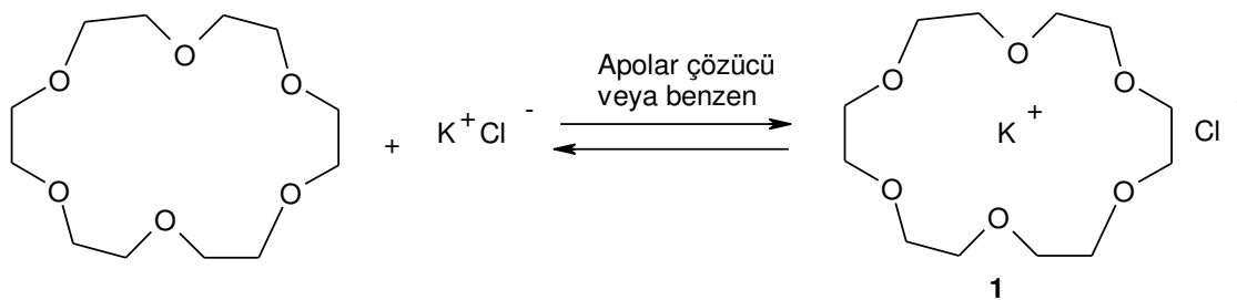
Şekil 2.2. Taç eterin metal katyonu ile kompleksleşmesi
