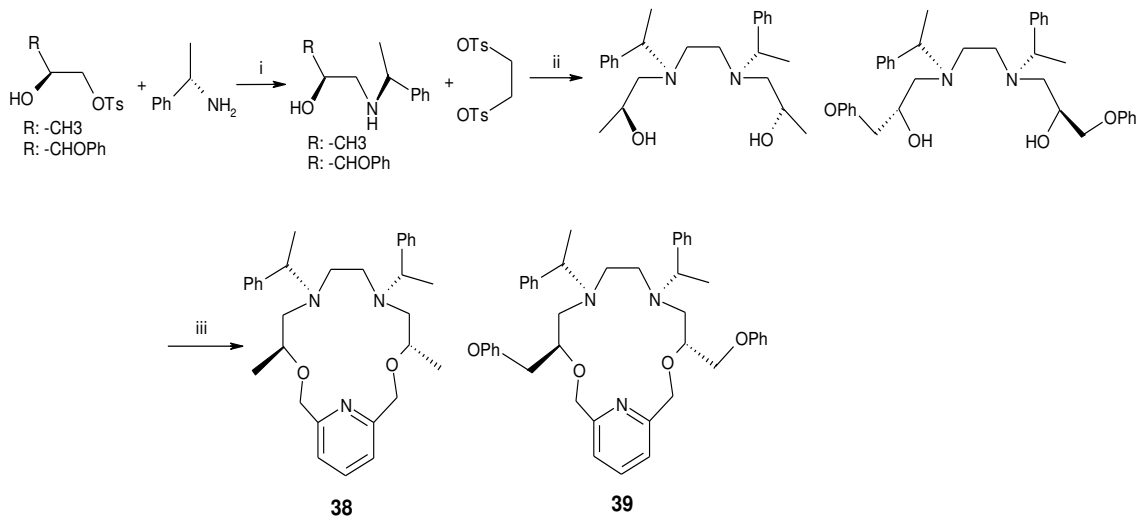
Şekil 2.24. Kiral amino alkol ve kirale piridin ünitesi içeren makrosiklik sentezi(i) ve (ii) Na 2 CO 3 , 12 saat, 110 °C, (iii) (1) NaH/THF, rifkaks (2) 2,6-piridinmetil ditosilat/ THF, 50 saat.
