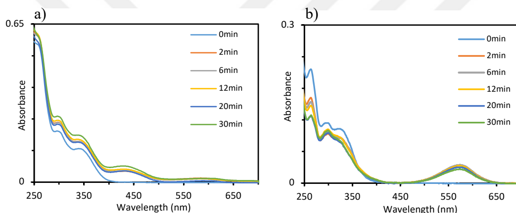
Figure 21. UV-Vis spectra of SPA-I in ( 10^{-5} M) a) dichloromethane b) hexane
