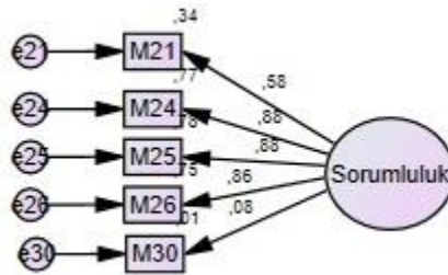
Şekil 10: Sorumluluk Alt Boyutu Tek Faktörlü Doğrulamalı Faktör Analizi
