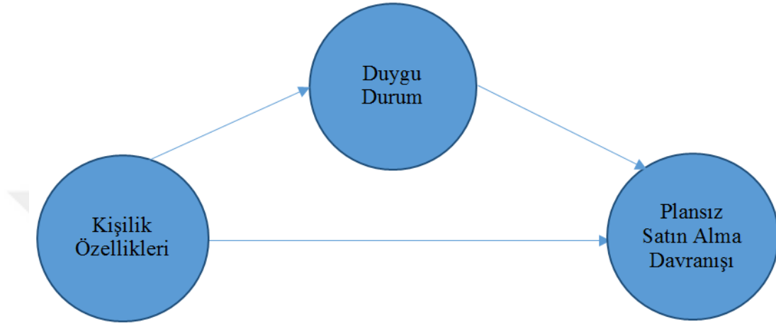
Şekil 6: Alternatif Araştırma Modeli 1
