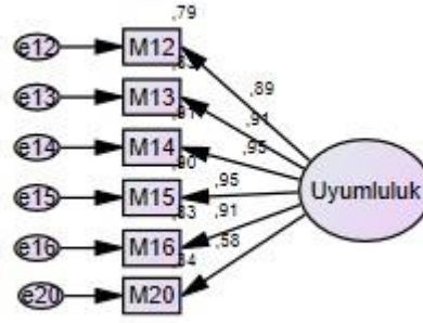
Şekil 9: Uyumluluk Alt Boyutu Tek Faktörlü Doğrulamalı Faktör Analizi
