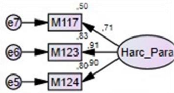
Şekil 15: Harcanan Para Alt Boyutuna İlişkin DFA
