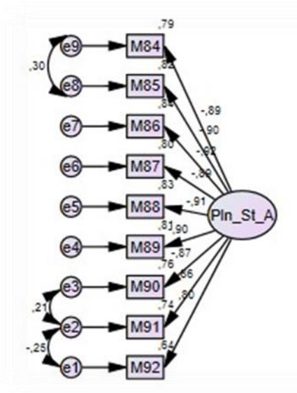
Şekil 18: Plansız Satın Alma Alt Boyutu Tek Faktörlü Doğrulayıcı Faktör Analizi
