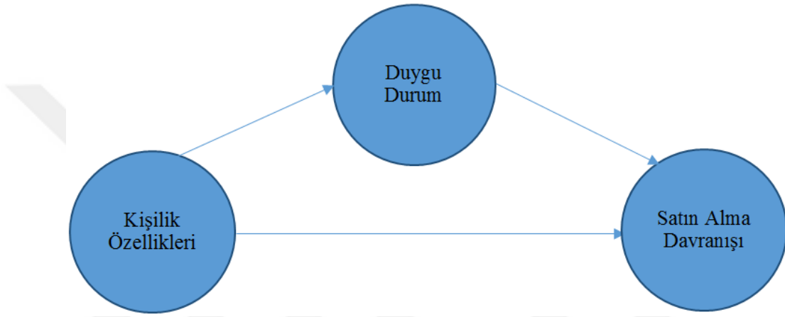
Şekil 32: Altıncı Hipotez Kapsamında Oluşturulan Model
