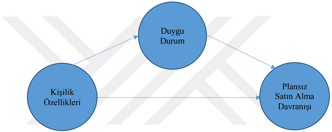
Şekil 29: Beşinci Hipotez Kapsamında Oluşturulan Model
