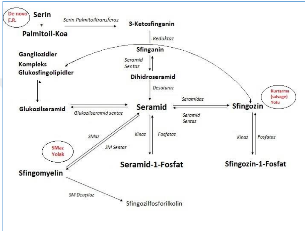
Şekil 2. 6. Sfingolipit metabolizması
