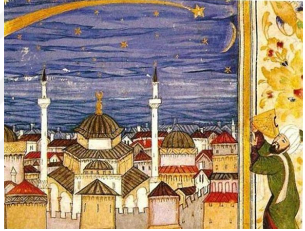
Resim 9: Şecâatname adlı eserde Takiyuddin'in kuyruklu yıldız gözlemi, Şecâatname İÜ Ktp., TY, nr. 6043
