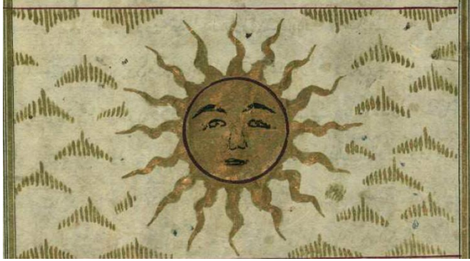
Resim 3: Nasani'nin Acaib eserinde hale tasviri, s. 40b.
