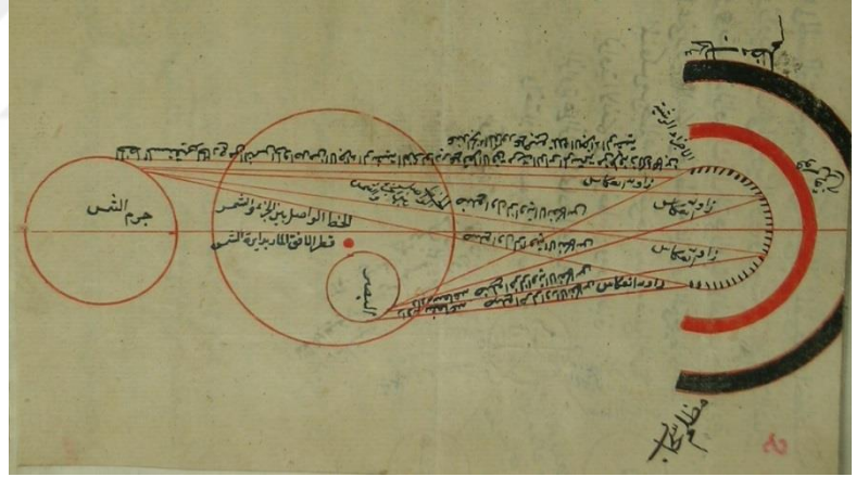
Resim 4: Hocaşade'nin Risale fî Mağrifeti Kavsi Kuzah adlı eserinde gökkuşağı çizimi
