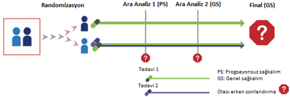
Şekil 2. 2. Grup Ardışık Tasarım
