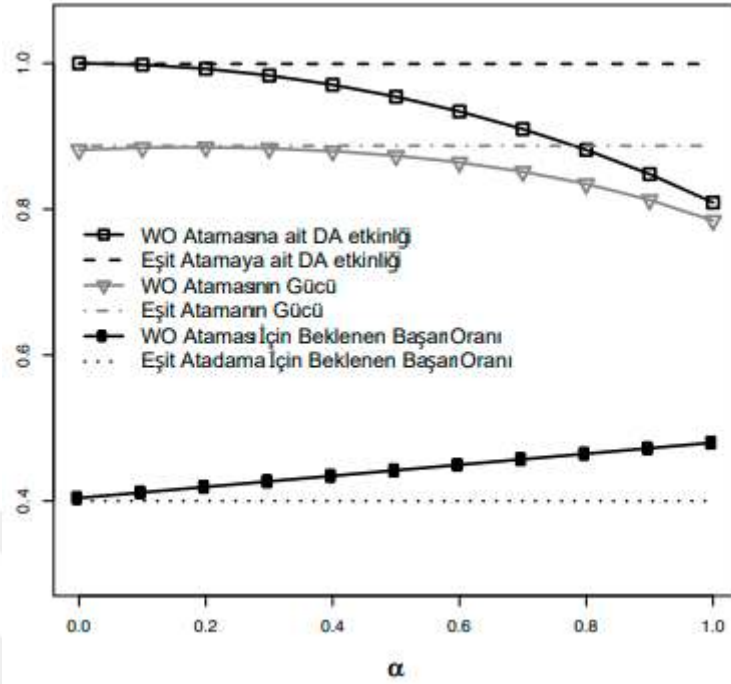
Şekil 4. 1. Eşit Atama Tasarımı ve Ağırlıklı Optimal (WO) Atama Tasarımına Ait Operasyonel Özellikler
