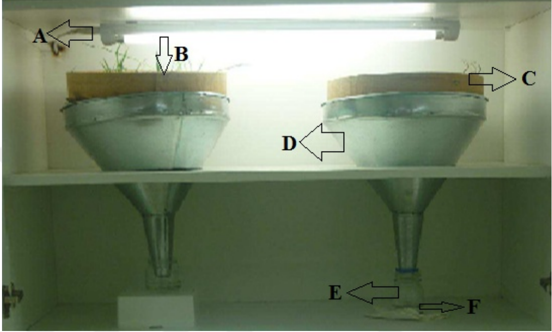
Şekil 2.4. Berlese hunisi düzenneği: A) ışık kaynağı, B) toprak örneği, C) elek, D) metal huni, E) toplama şişesi, F) toplama sıvısı (% 70' lik alkol)
