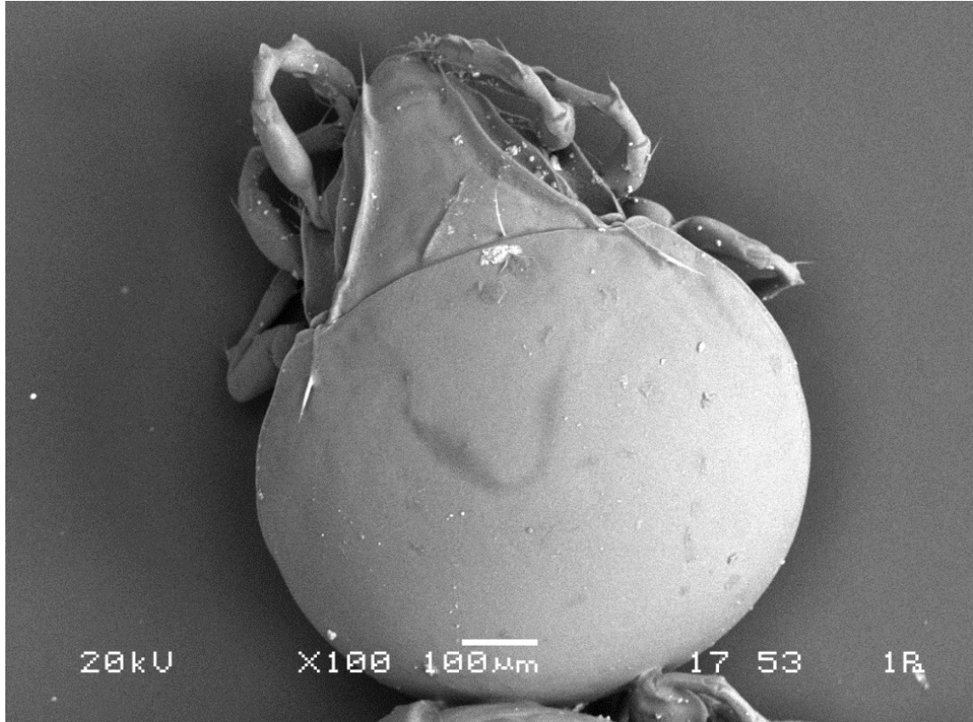
Şekil 3.1. Conoppiapalmicincta SEM görüntüsü, dorsal görüntü
