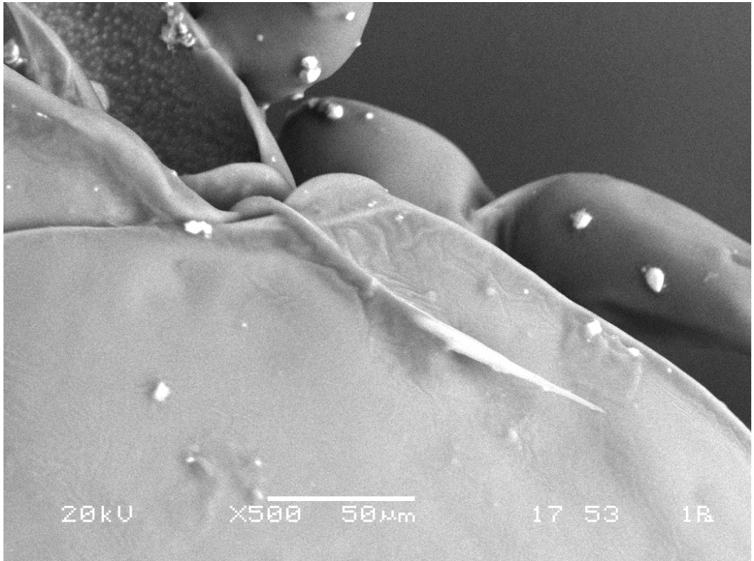
Şekil 3.3. Conoppiapalmicincta SEM görüntüsü, sensillus
