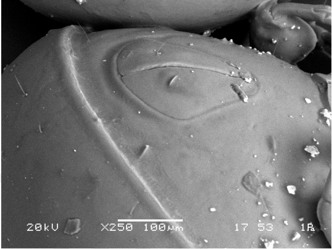
Şekil 3.5. Conoppiapalmicincta SEM görüntüsü, anal plak
