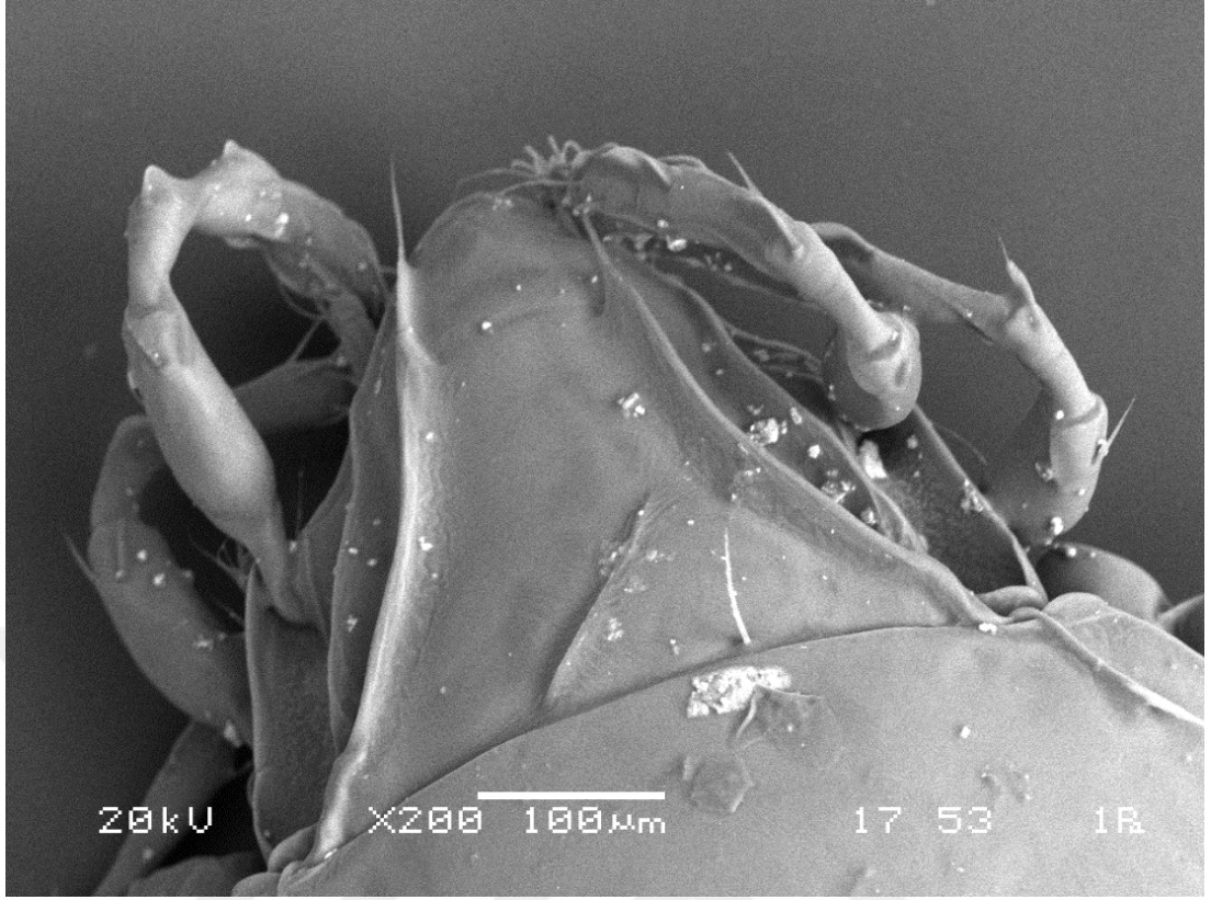
Şekil 3.2. Conoppiapalmicincta SEM görüntüsü, prodorsal bölge
