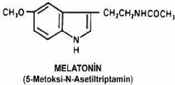
Şekil 11. Melatoninin yapısı (77)
