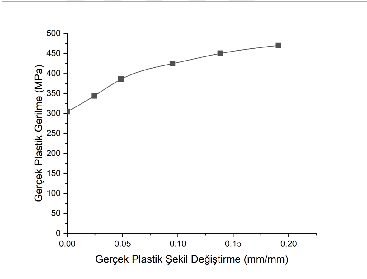
Şekil 20. Enerji sönümleyici tüp malzemesinin gerçek plastik gerilme-şekil değiştirme eğrisi [65].
