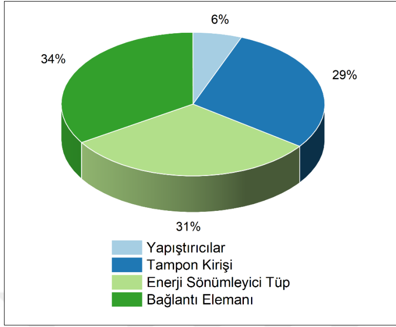
Şekil 81. Hibrit ön tampon sistemi bileşenlerinin toplam sönümlenen enerjiye katkı oranları
