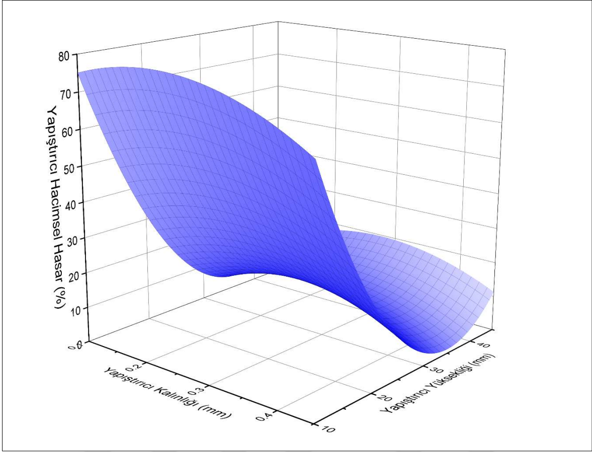
Şekil 89. Yan yapıştırıcı kalınlığı ve yüksekliğinin yapıştırıcıda meydana gelen hasara olan etkisi
