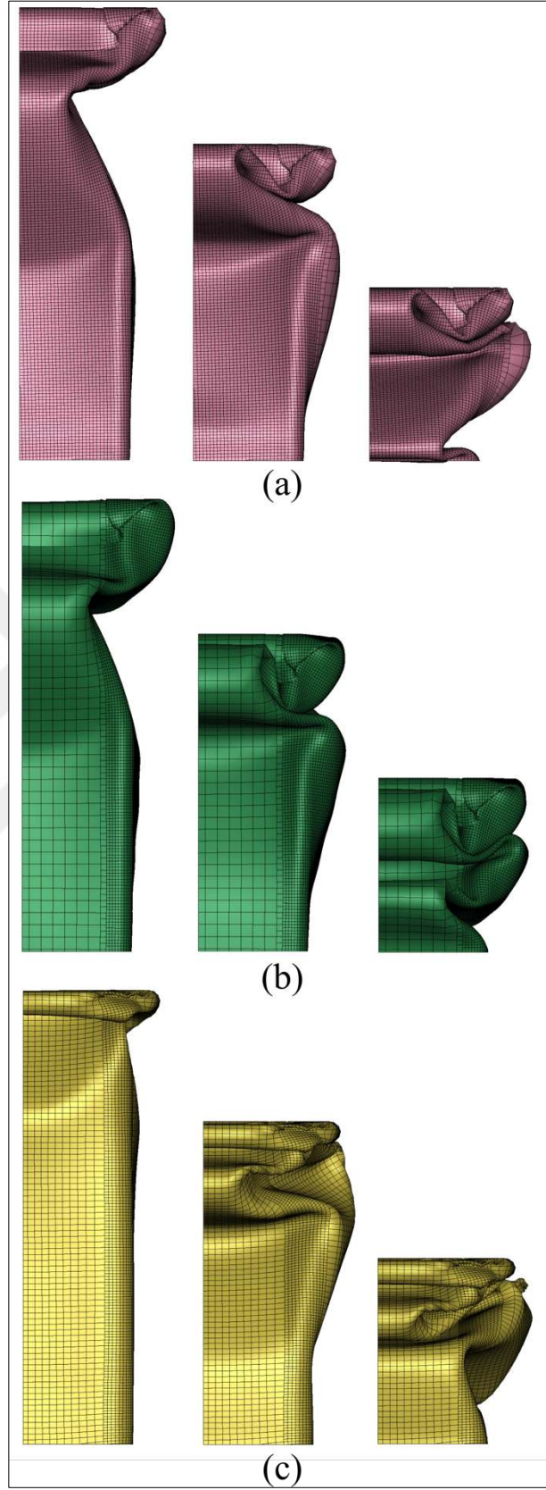
Şekil 53. (a) Derin çekme, (b) kenar bükme ve (c) hidroforming ile elde edilen enerji sönmleyici tüplerde darbe yüklemesi sonucu oluşan deformasyonlar
