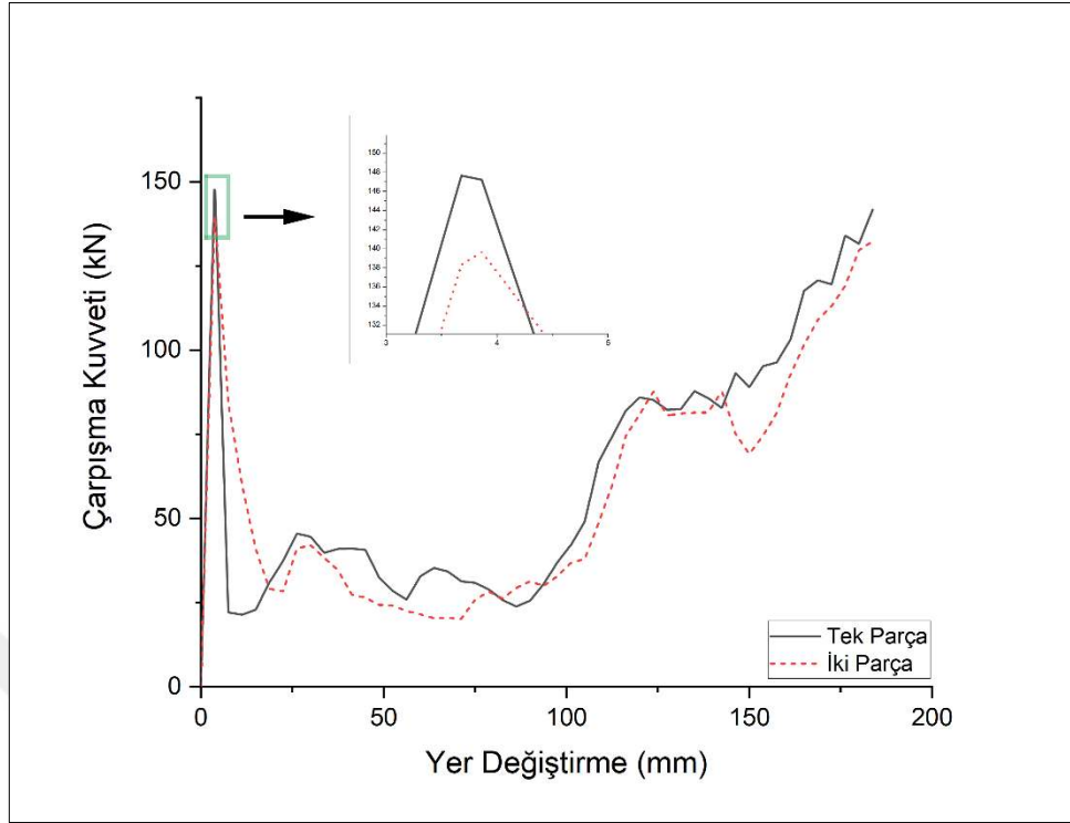
Şekil 63. Kalınlık optimizasyonu sonrası tek parçalı ve iki parçalı enerji sönümleyici tüpün çarpışma kuvveti dağılımı
