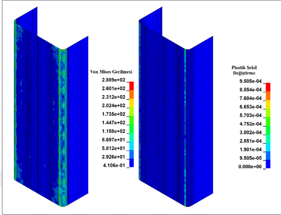
Şekil 49. Kenar bükme işlemi sonrasında elde edilen gerilme ve şekil değişirme değerleri
