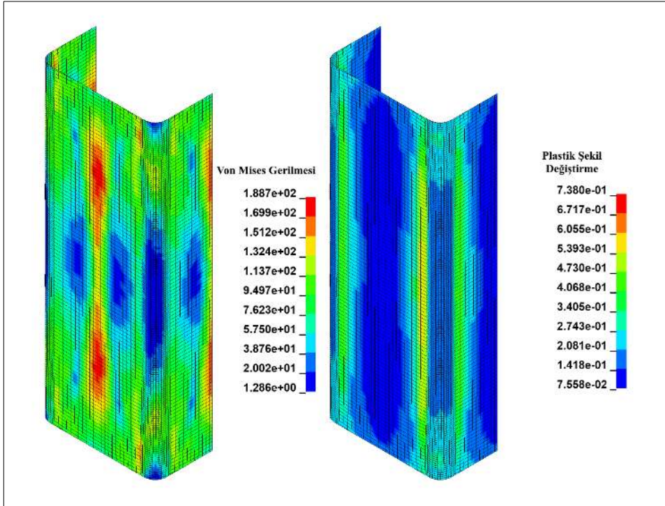
Şekil 50. Hidroforming işlemi sonrasında elde edilen gerilme ve şekil değişirme değerleri
