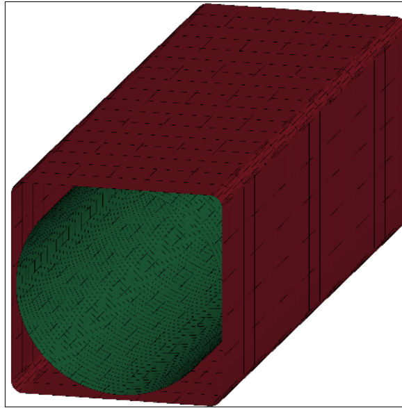
Şekil 29. Hidroforming prosesi sonlu elemanlar modeli
