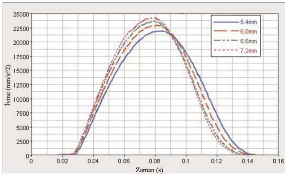
Şekil 15. Karbon fiber tampon kirişi için kalınlığın ivmelenmeye olan etkisi [56].
