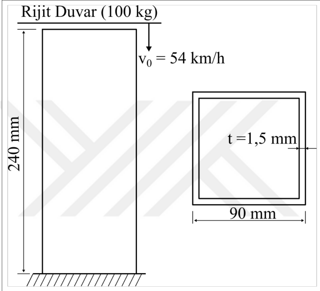
Şekil 21. Enerji sönümleyici tüpün başlangıç geometrisi
