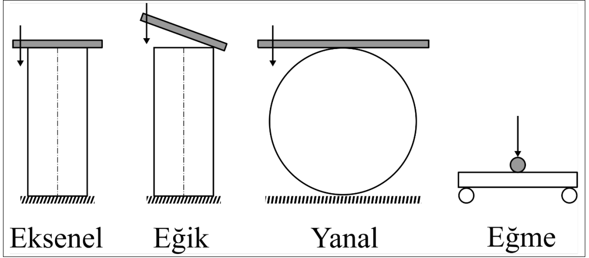
Şekil 2. Enerji sönümleyici tüplerde yükleme çeşitleri
