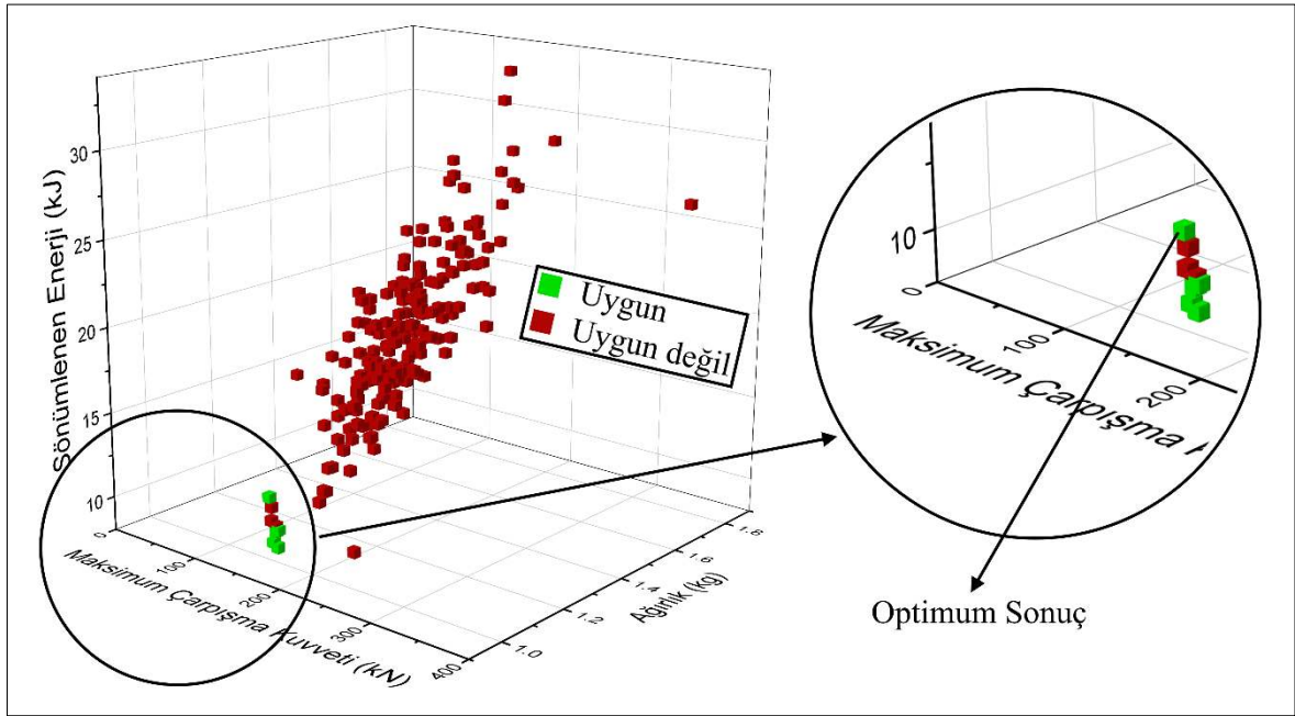
Şekil 54. Enerji sönümleyici tüpün kalınlık optimizasyonu serpmeye diyagramı
