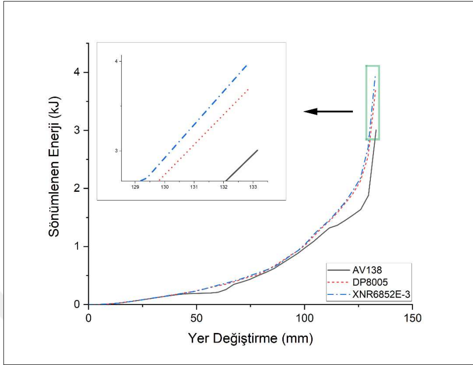
Şekil 75. AV138, DP8005 ve XNR6852E-3 Yapıştırıcıları için hibrit ön tampon sistemi sönümlenen enerji-yer değiştirme eğrisi
