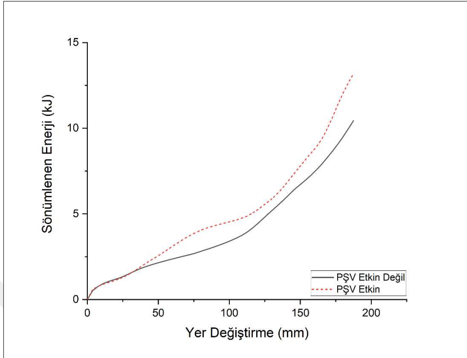
Şekil 66. Plastik şekil verme işleminin sönümlenen enerji miktarına olan etkisi
