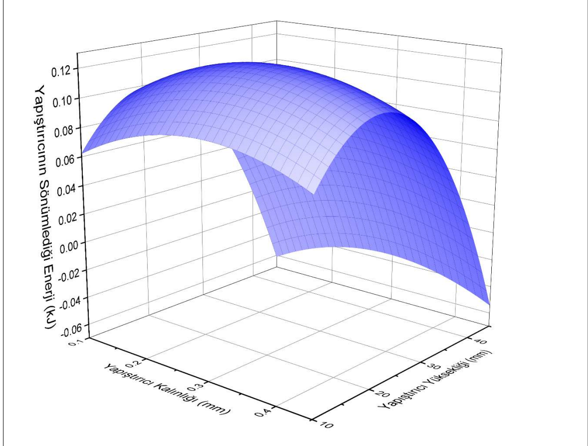
Şekil 88. Yan yapıştırıcı kalınlığı ve yüksekliğinin yapıştırıcı tarafından sönümlenen enerjiye olan etkisi
