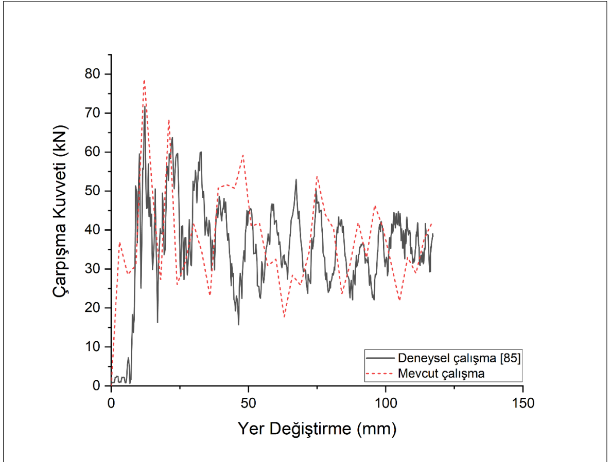
Şekil 69. Kompozit tampon kirişi doğrulama modelinden elde edilen çarpışma kuvveti dağılımı
