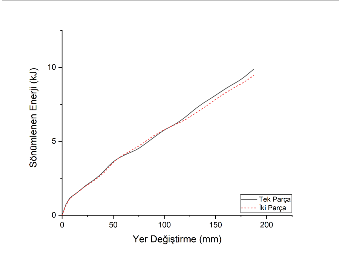
Şekil 62. Sabit kalınlığa sahip tek parçalı ve iki parçalı enerji sönümleyici tüpün enerji sönümleme kapasitesi
