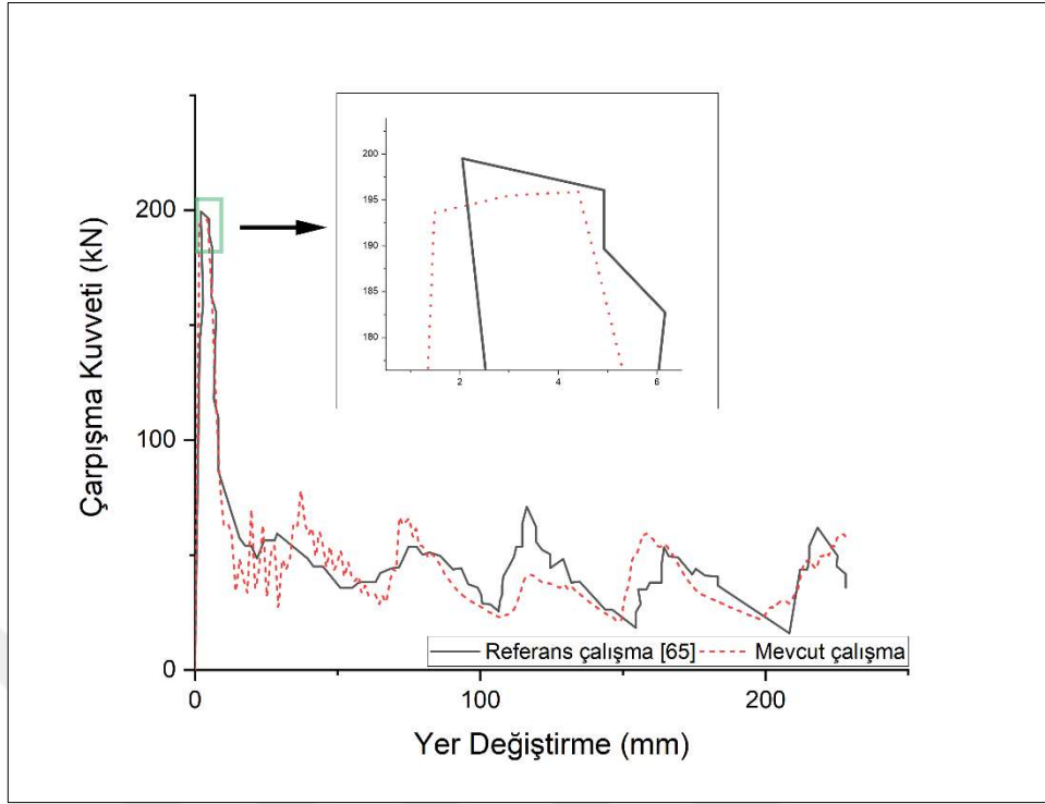
Şekil 45. Enerji sönümleyici tüpün sonlu elemanlar modelinin doğrulanması sonuçları
