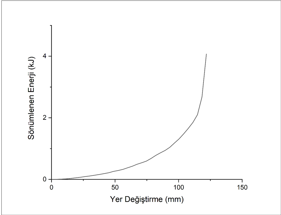
Şekil 85. Üst yapıştırıcının optimizasyonu sonrası optimum konfigürasyon için sönümlenen enerji-yer değiştirme eğrisi
