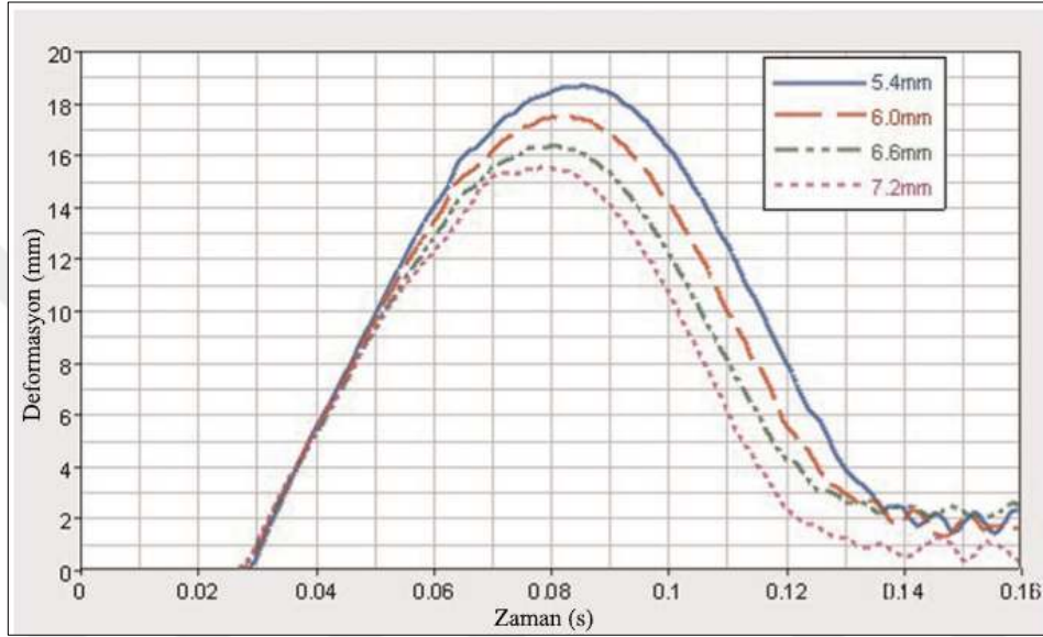
Şekil 14. Karbon fiber tampon kirişi için kalınlığın deformasyona olan etkisi [56].
