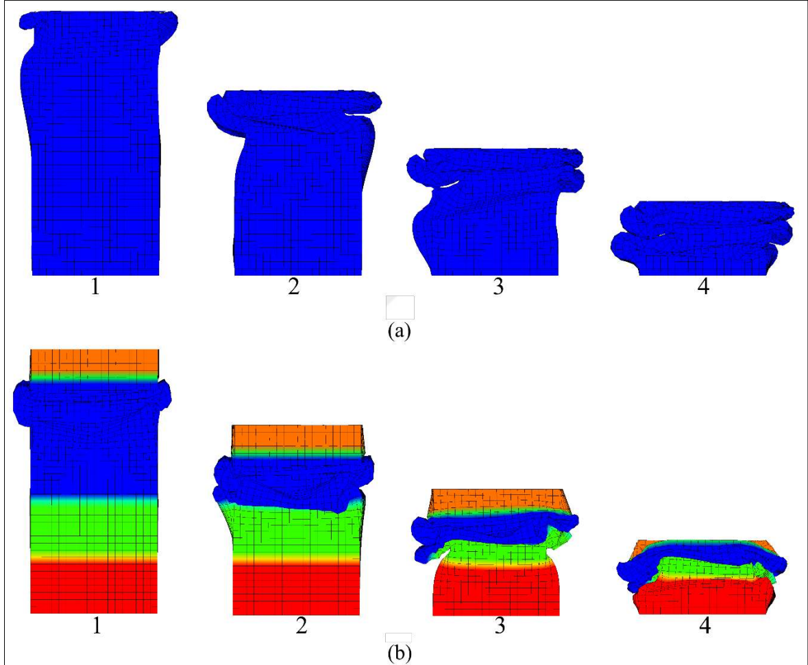
Şekil 57. Kare kesitli enerji sönmleyici tüpün deformasyon davranışı: (a) Sabit kalınlık; (b) optimize edilmiş kalınlık
