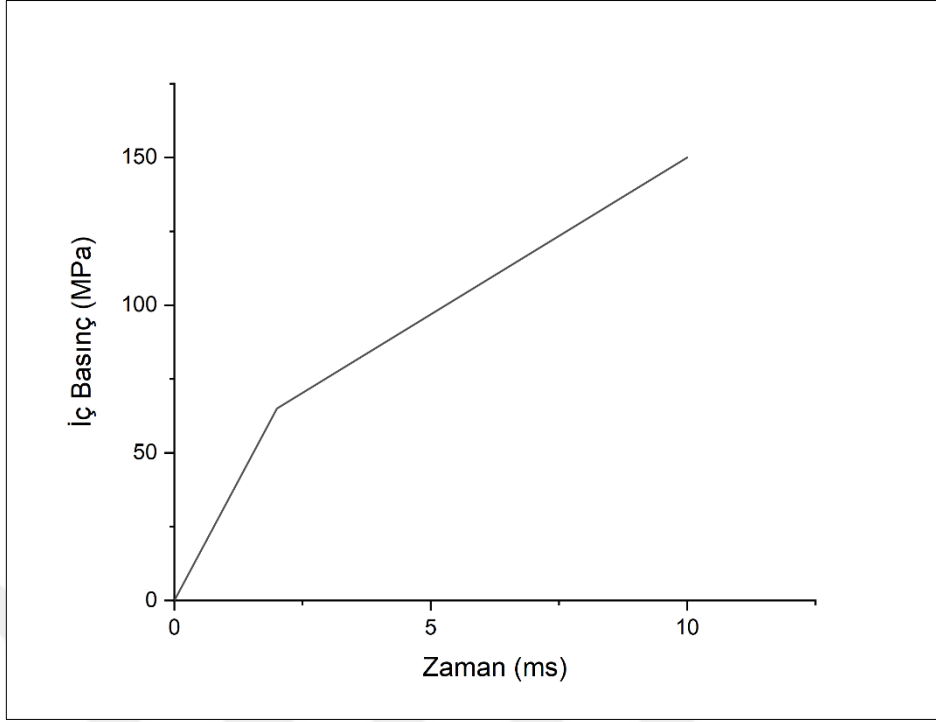
Şekil 31. Hidroforming prosesinde uygulanan iç basınç profili
