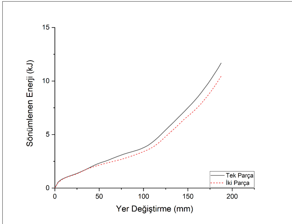
Şekil 64. Kalınlık optimizasyonu sonrası tek parçalı ve iki parçalı enerji sönümleyici tüpün enerji sönümlenme kapasitesi
