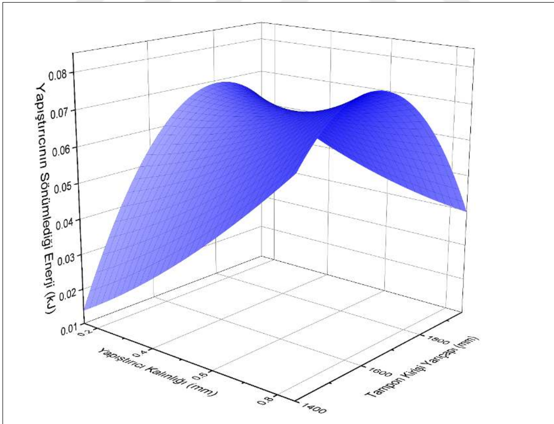
Şekil 82. Üst yapıştırıcı kalınlığının ve tampon kirişi yarıçapının üst yapıştırıcının sönümlediği enerjiye olan etkisi
