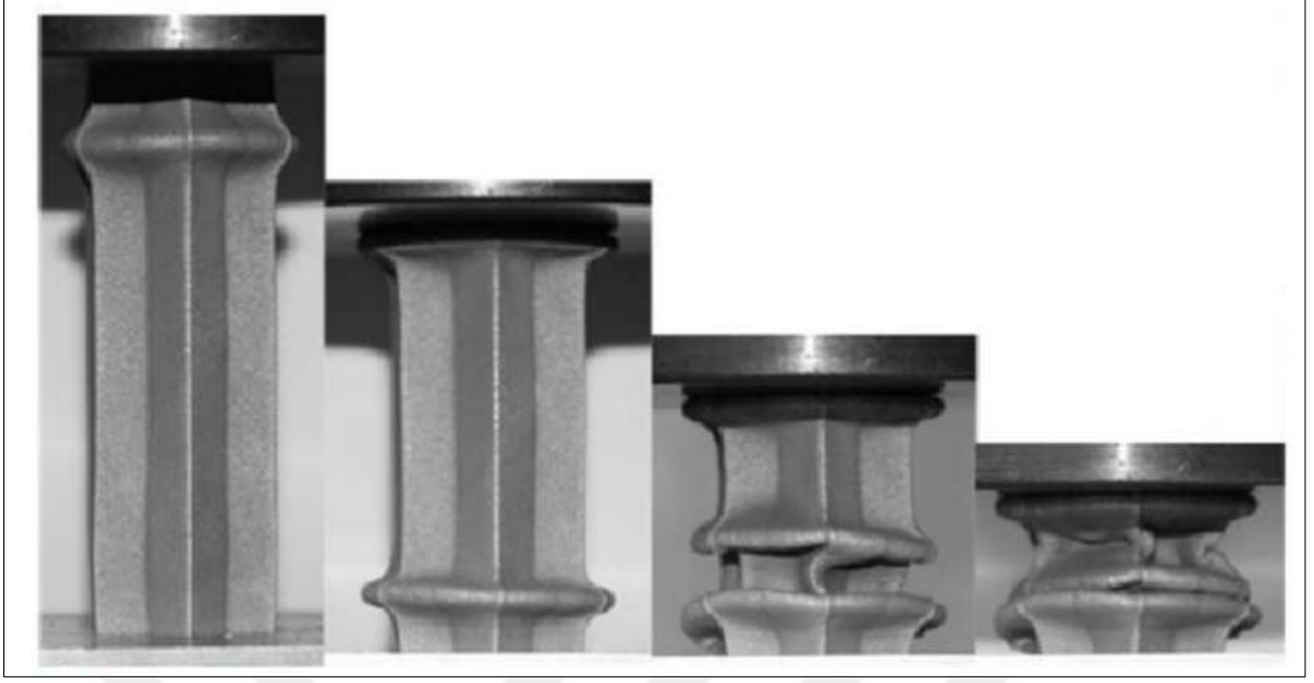
Şekil 5. Yıldız şekilli içbükey çokgen enerji sönümleyici tüpün aksenal yük altında deformasyon davranışı [28].
