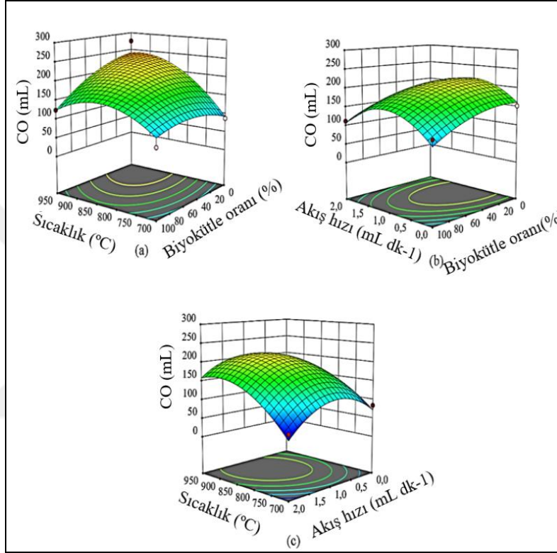
Şekil 4.32. CO hacmine ait (mL) 3 boyutlu yanıt yüzey grafikleri;
