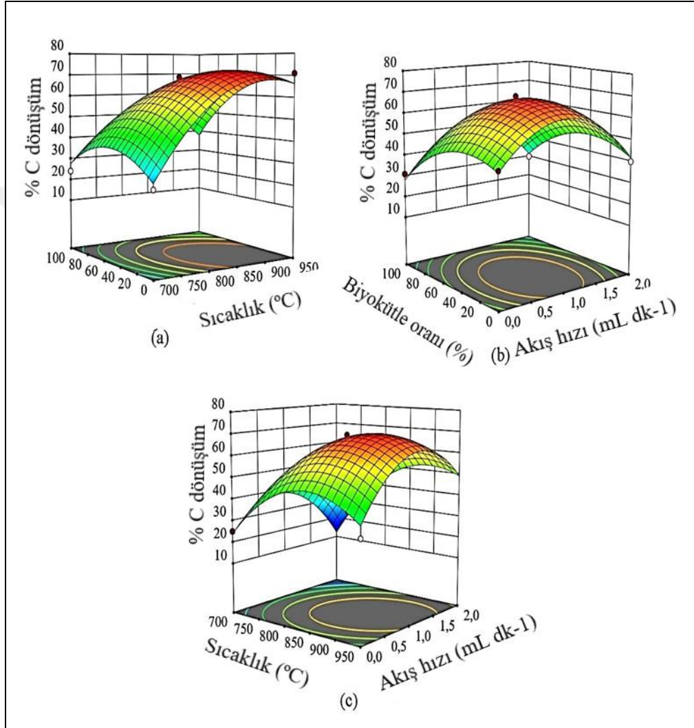
Şekil 4.26. Karbon dönüşüm verimine ait 3 boyutlu yanıt yüzey grafikleri (%); a) sıcaklık (°C) ve biyokütle oranı (%) sabit akış hızında (1,1 mL dk -1 ); b) biyokütle oranı (%) ve akış hızı (mL dk -1 ) sabit sıcaklıkta (888 °C) c) sıcaklık (°C) ve akış hızı (mL dk -1 ) sabit biyokütle oranında (%25).
