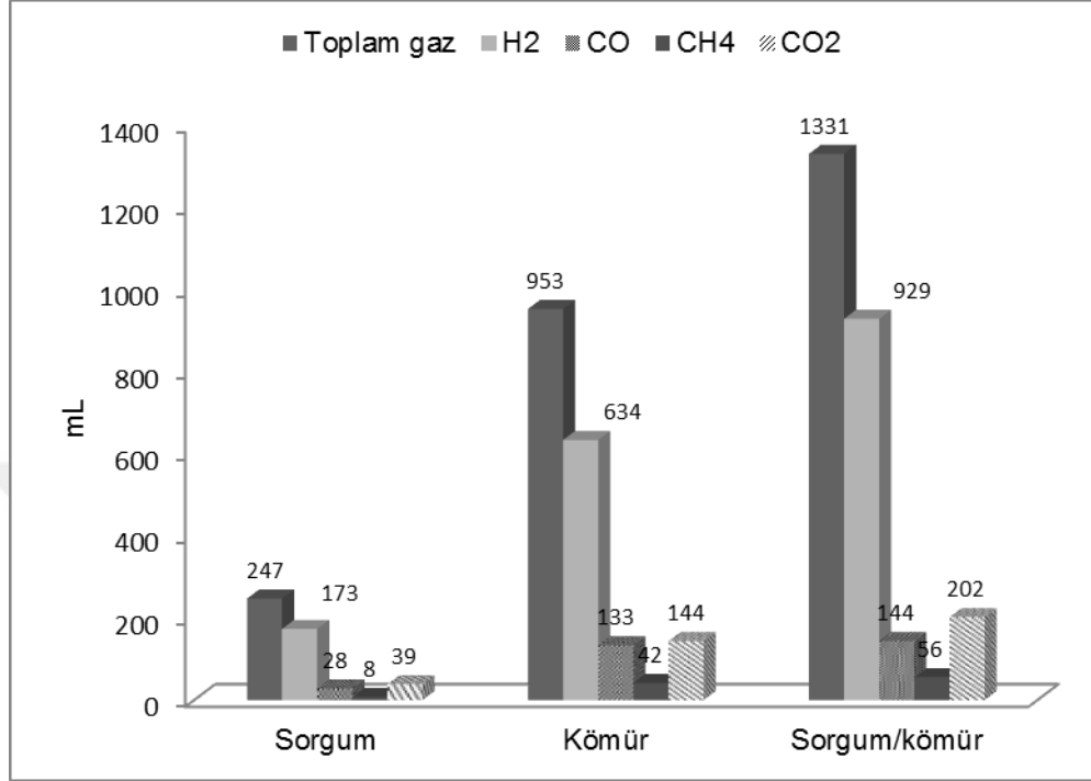
Şekil 4.12. Sorghum, kömür (Çan) ve kömür/sorghum karışımlarının birlikte gazlaştırılmalarından elde edilen gaz hacimlerinin karşılaştırılması (Proses koşulları: 700°C sıcaklık; 0,5 mL dk -1 su akış hızı)
