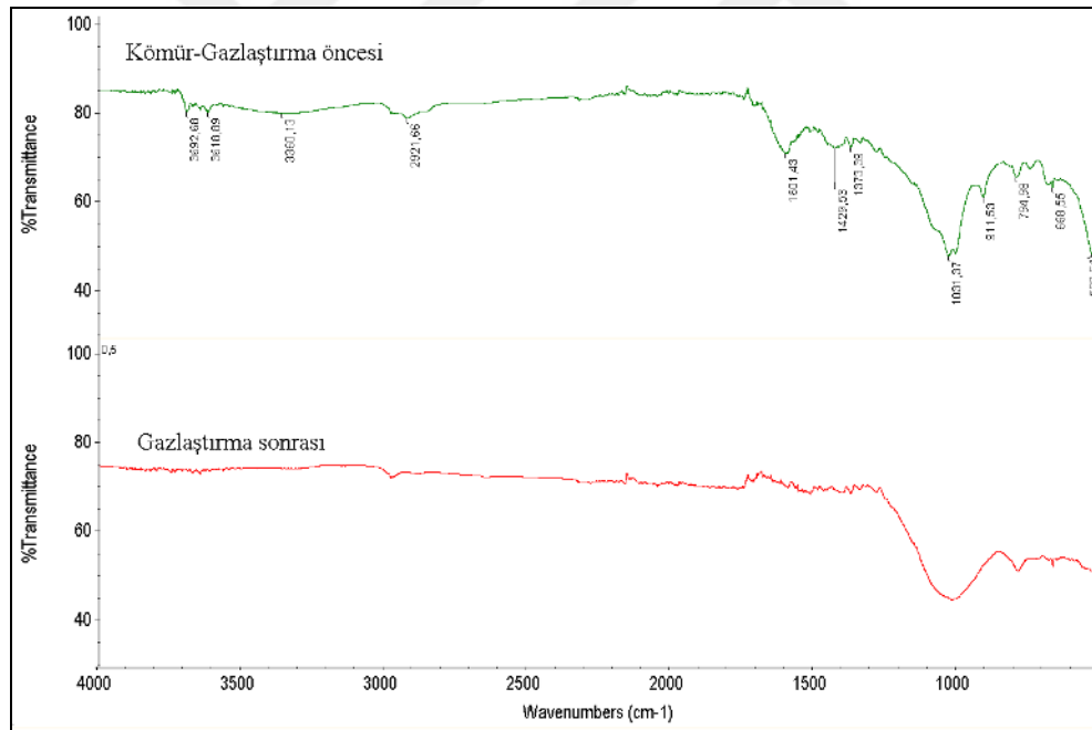
Şekil 4.3. Gazlaştırma deneylerinde önce orijinal kömürün (Çan) ve gazlaştırma sonrası reaktörde kalan katının FT-IR spektrumları (Proses koşulları: 0,5 mL dk -1 su akış hızı ve 700°C gazlaştırma sıcaklığı).
