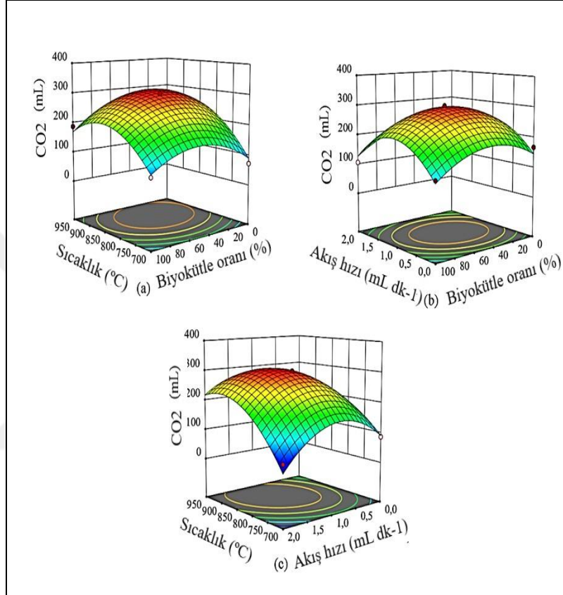
Şekil 4.31. CO 2 hacmine ait 3 boyutlu yanıt yüzey grafikleri
