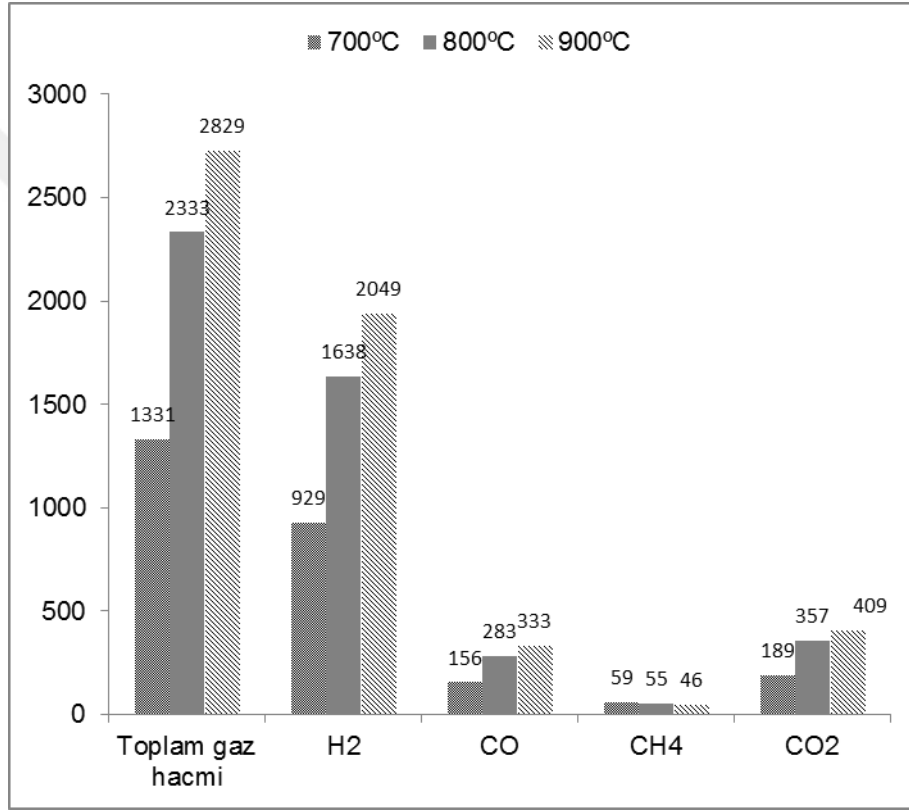
Şekil 4.14. %25 sorgum içeren Çan kömürü/sorgum karışımlarının farklı sıcaklıklarda gazlaştırılmalarından elde edilen gaz hacimlerinin karşılaştırılması (Proses koşulları: 0,5 \text{ mL dk}^{-1} su akış hızı).
