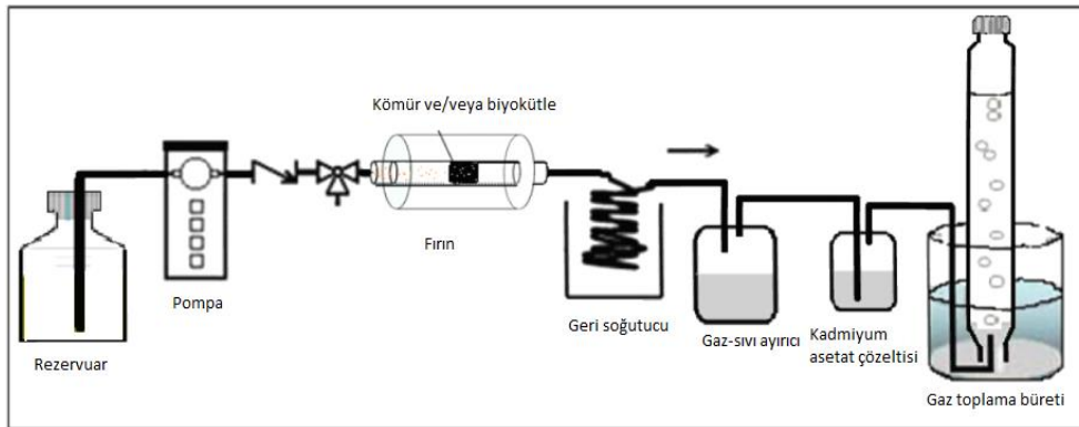
Şekil 3.1. Gazlaştırma sistemi
