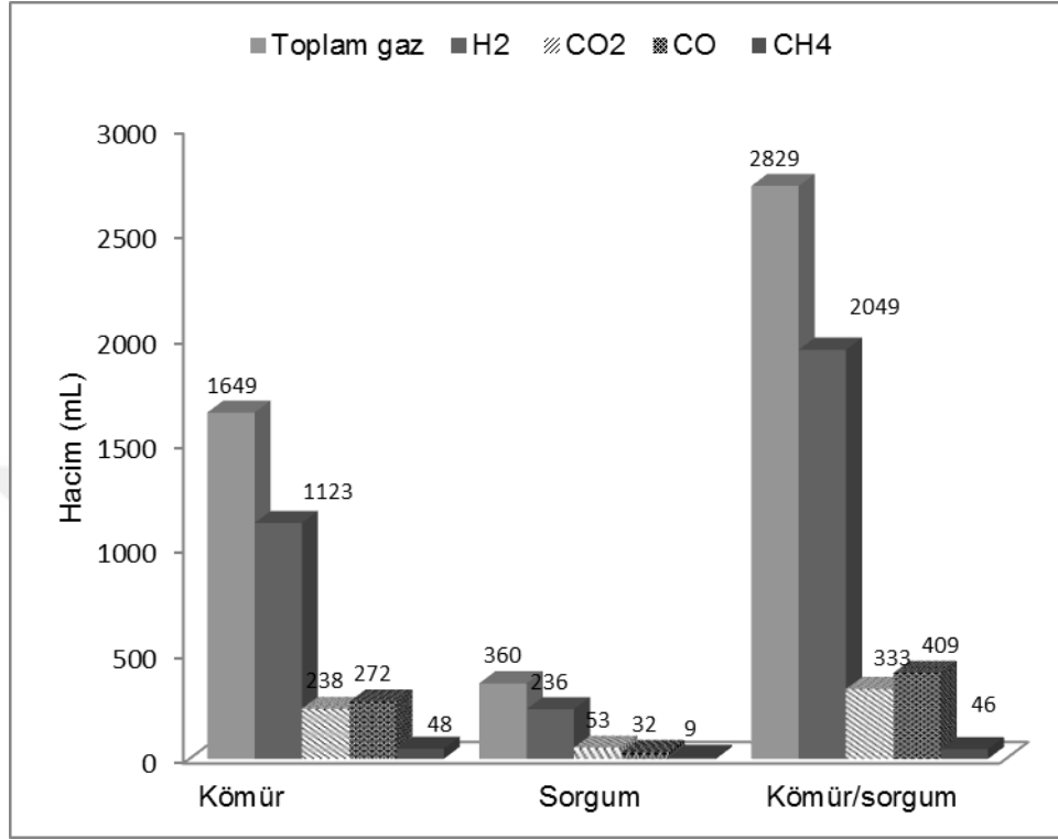
Şekil 4.16. Kömür (Çan), sorgum ve kömür/sorgum karışımlarının gazlaştırılmalarından elde edilen gaz hacimlerinin karşılaştırılması (Proses koşulları: 900°C sıcaklık; 0,5 mL dk -1 su akış hızı)
