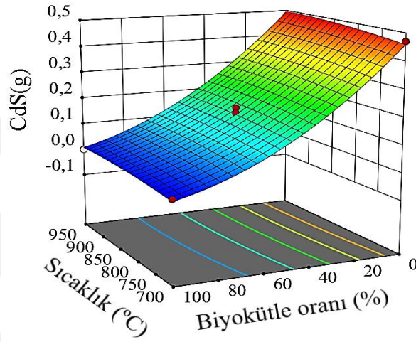
Şekil 4.34. CdS miktarının sıcaklık ( ^{\circ}C ve biyokütle oranına (%) bağlı 3 boyutlu yanıt yüzey grafiği.
