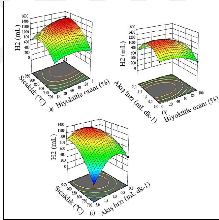
Şekil 4.30. Hidrojen hacmine ait 3 boyutlu yanıt yüzey grafikleri; a) Sıcaklık ve biyokütle oranı, sabit akış hızında (1,1 mL dk -1 ); b) Akış hızı ve biyokütle oranı, sabit sıcaklıkta (888°C) c) Sıcaklık ve akış hızı, sabit biyokütle oranında (%25)
