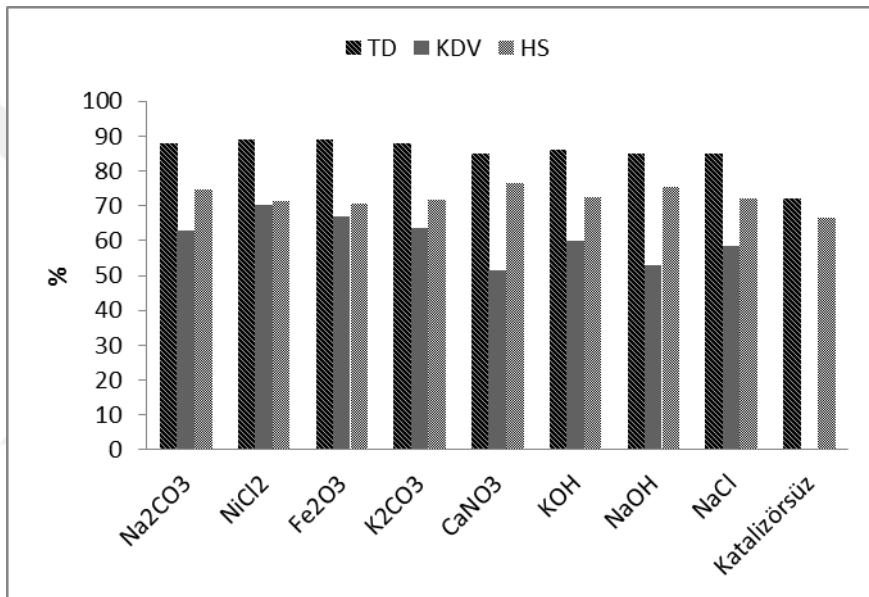
Şekil 4.9. Farklı katalizörlerin toplam dönüşüm (TD), karbon dönüşüm verimi (KDV) ve hidrojen seçiliğine (HS) etkisi (Proses koşulları: 700°C sıcaklık; 0,5 mL dk -1 su akış hızı).
