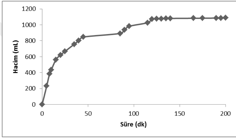
Şekil 4.1. Çan kömürünün gazlaştırılmasına ait zaman–toplam gaz oluşum grafiği (Proses koşulları: 700°C sıcaklık; 1,0 g (kkb) kömür; 0,5 mL dk -1 su akış hızı).
