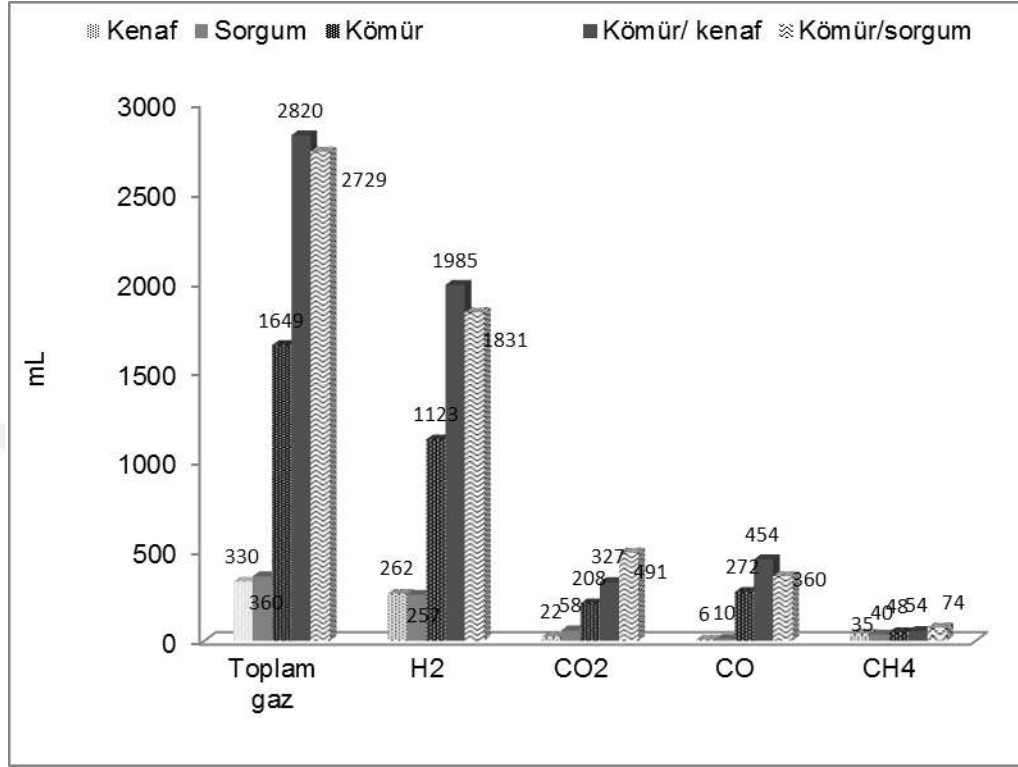
Şekil 4.17. Kömür (Çan), sorgum ve kenaf ile kömür/sorgum ve kömür kenaf karışımlarının gazlaştırılmalarından elde edilen gaz hacimlerinin karşılaştırılması (Proses koşulları: 900°C sıcaklık; 0,5 mL dk -1 su akış hızı)
