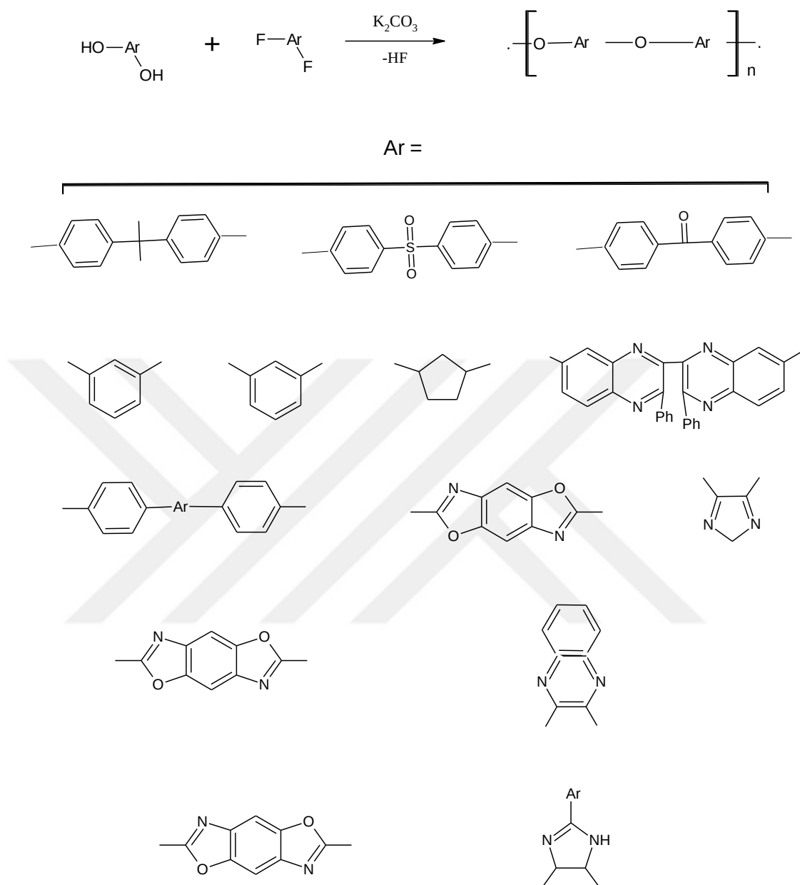
Şekil 2.4 Bazı heterosiklik monomerlerin nükleofilik aromatik sübsitüsyon reaksiyonu
