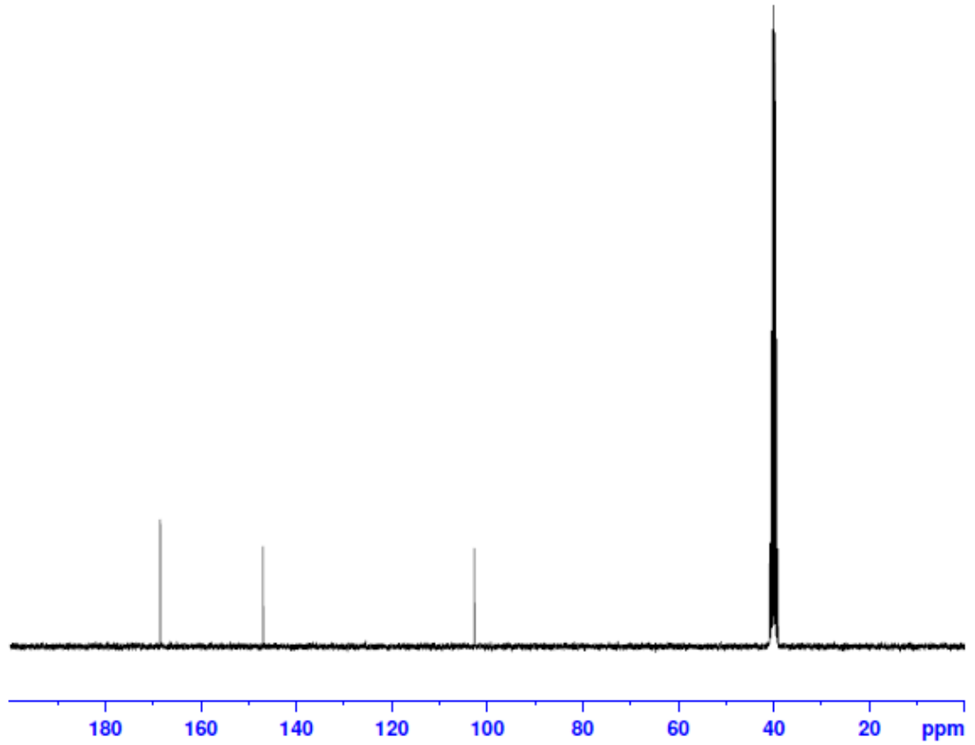
Şekil 4.32, 2'-diamino-4,4'-bitiyazol bileşiğinin 13 C-NMR spektrumu
