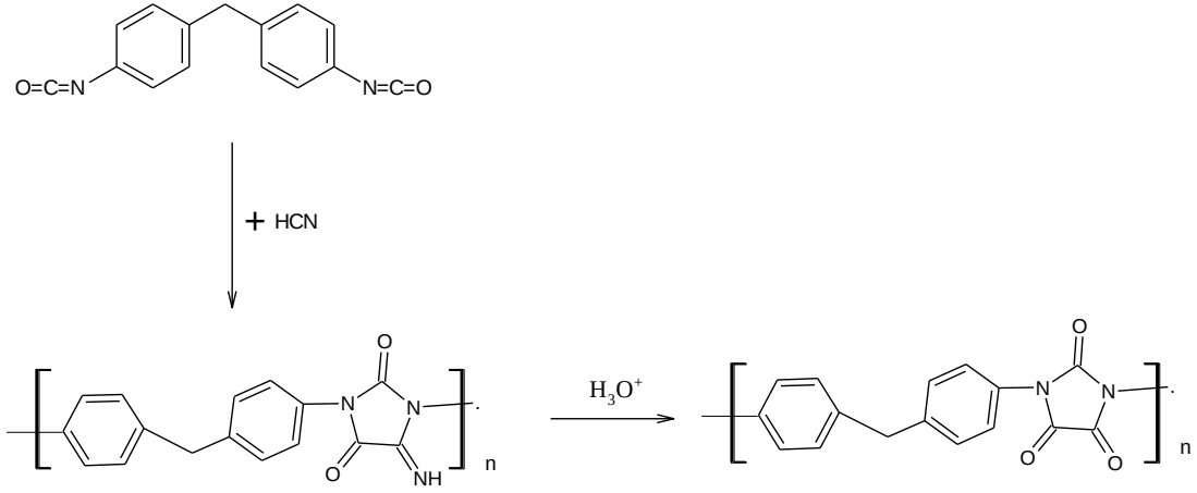
Şekil2.2 Poliparabanik asitlerin sentezi
