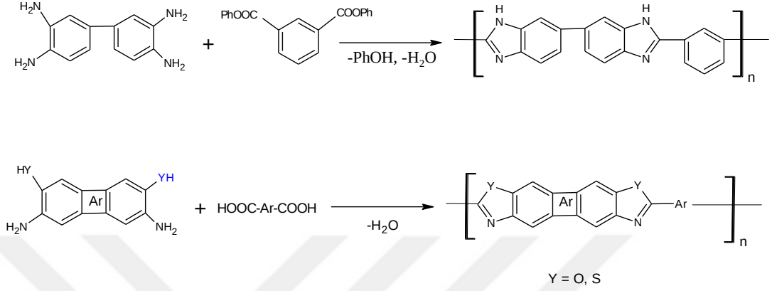
Şekil2.1 Polibenzimidazollerin sentezi
