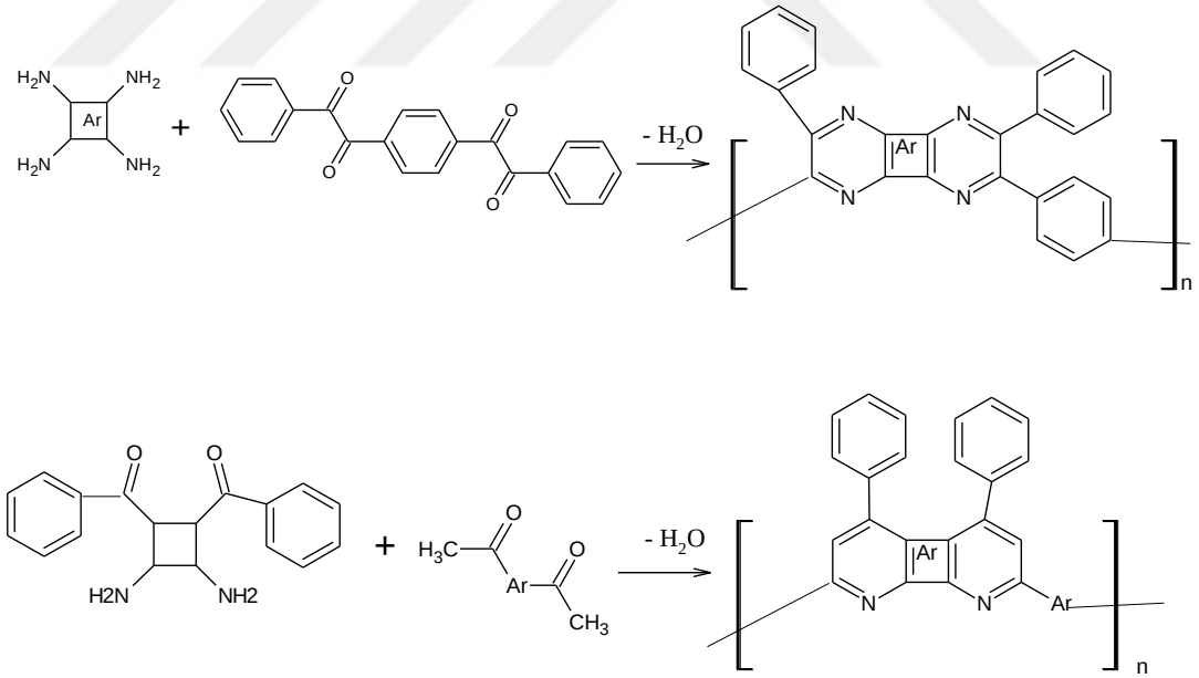
Şekil2.3 Polikinolinlerin sentezi
