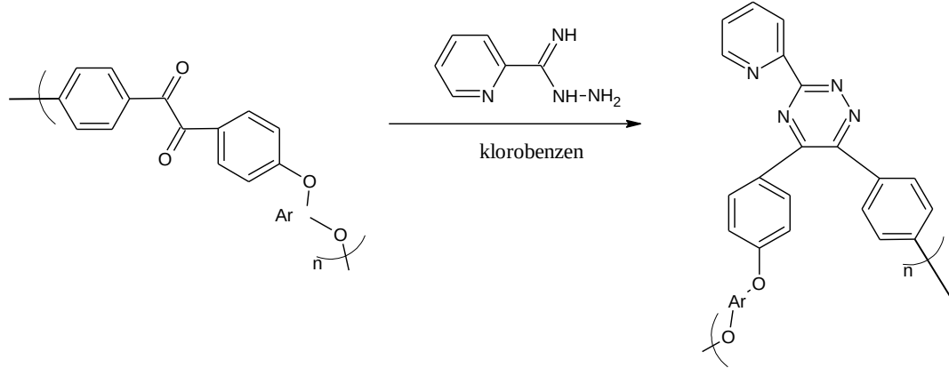
Şekil2.7Heterosiklik poli(arileter-piridiltriazin)’lerin sentezi
