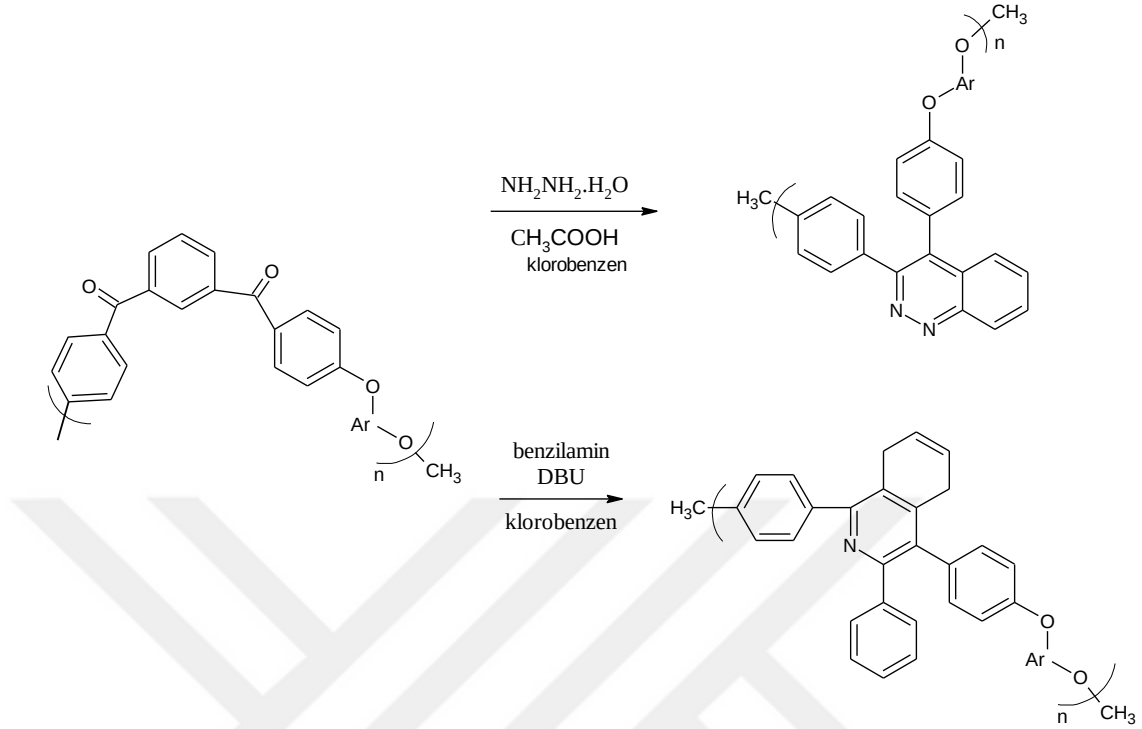
Şekil 2.6 Heterosiklik poli(arileter-izokinolin) ve poli(arileter-fitalazin)'lerin sentezi
