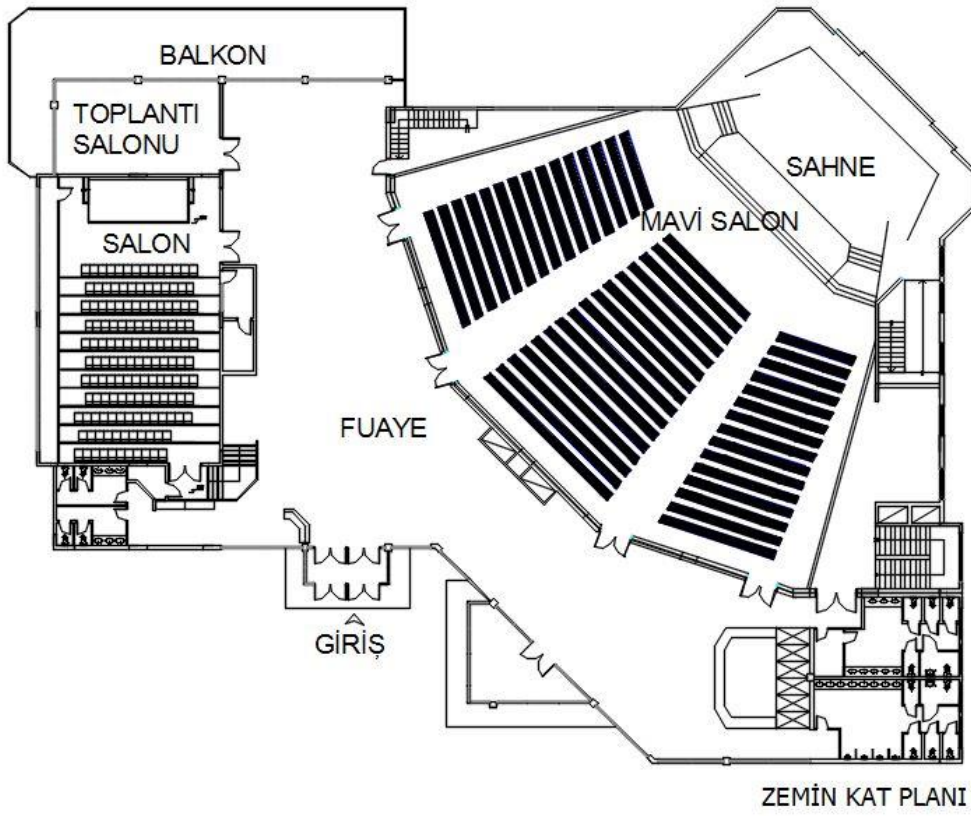
Şekil 58. Atatürk Kültür ve Kongre Merkezi Planı
