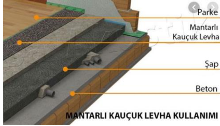
Şekil 22. Zemin İzolasyonu
