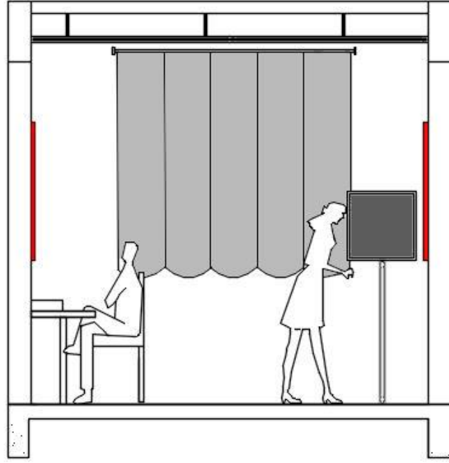
Şekil 45.Kayıt Stüdyosu Kesit
