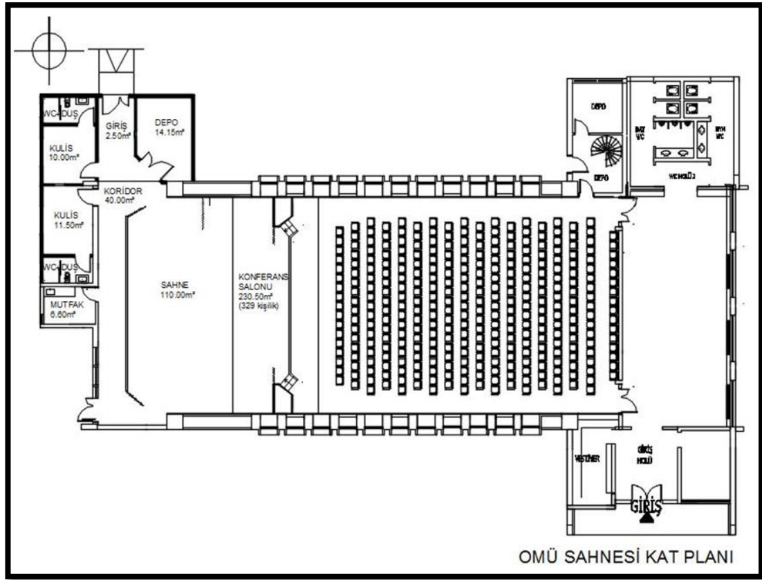
řekil 50. Om Sahnesi Planı
