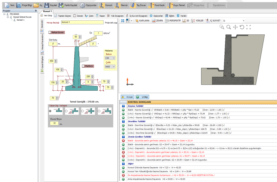
Şekil 5.2. Konsol tipi istinat duvarı veri giriş ekranı.
