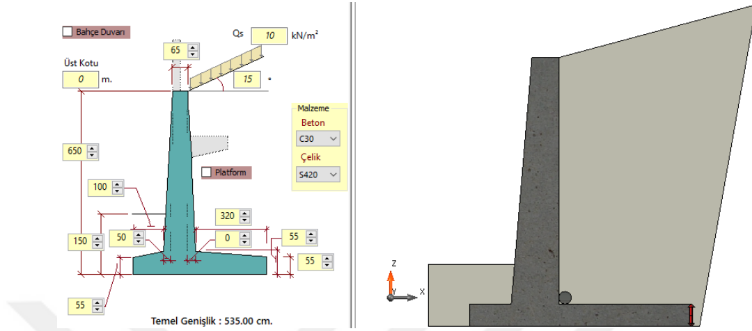
Şekil 6.4. istCAD programında konsol istinat duvarının boyutlandırılması.
