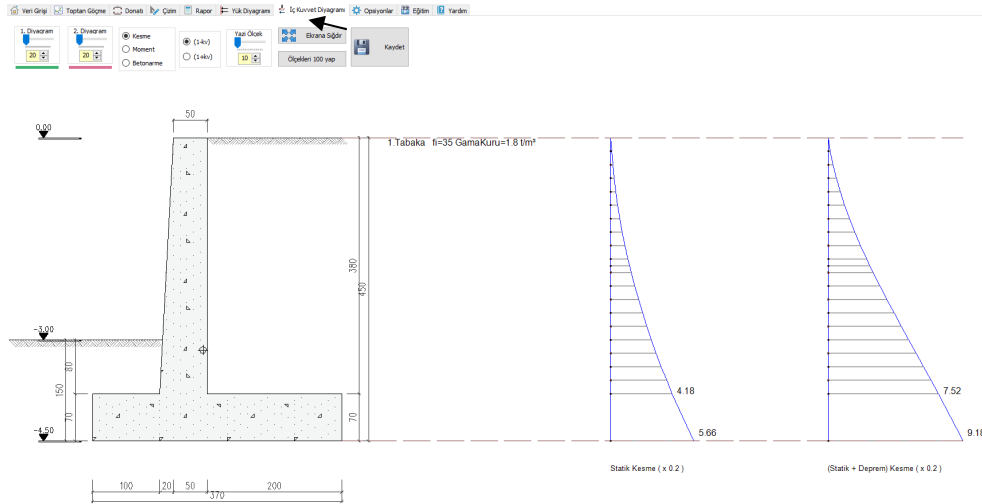
Şekil 5.11. İç kuvvetler diyagramlarının görüntüsü.
