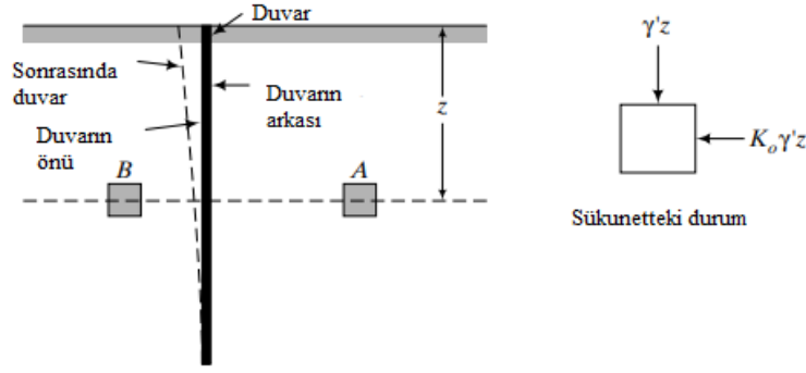
Şekil 2.8. Sükunetteki zemin basıncı (Budhu, 2011).
