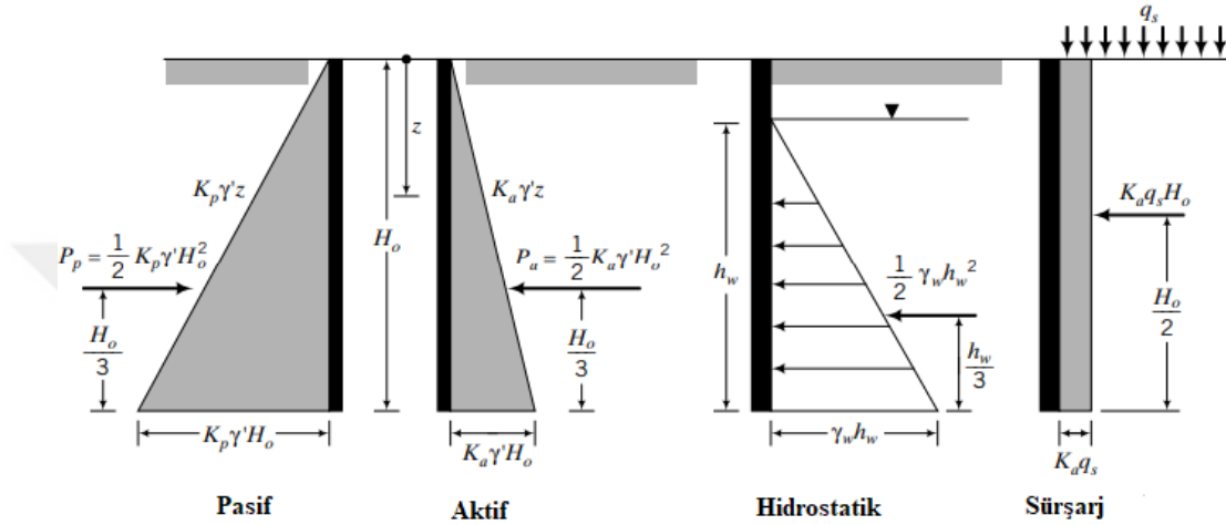
Şekil 2.7. Aktif, pasif yanal toprak basıncı, hidrostatik ve sürşarj etkisinin duvar derinliğiyle değişimi (Budhu, 2011).
