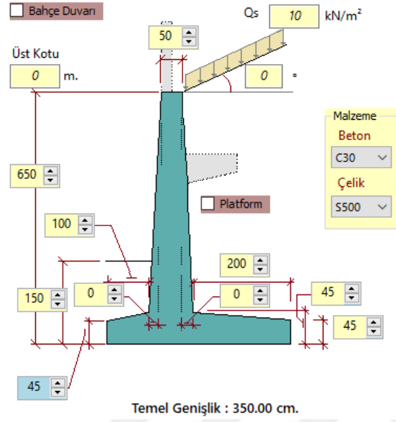
Şekil 6.16. Zemin eğimi 0^\circ olması durumunda duvar boyutu.
