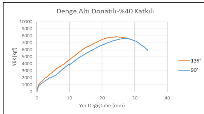
Şekil 6.15. A-10-a-2-z ve A-10-b-2-z numunelerinin Yük-Yer Değiştirme grafikleri
