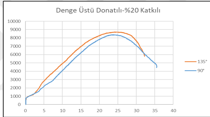
Şekil 6.14. B-10-a-2-y ve B-10-b-2-y numunelerinin Yük-Yer Değiştirme grafikleri
