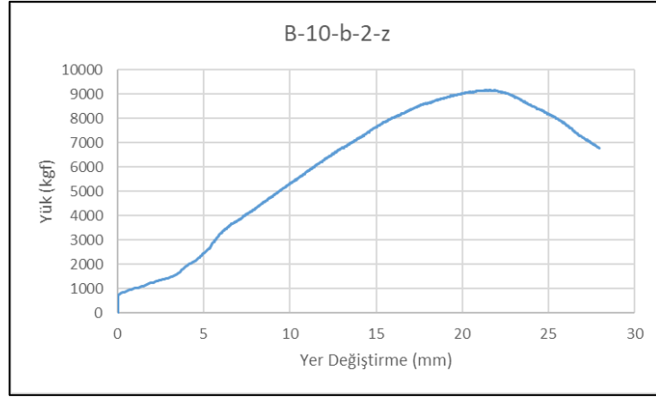
Şekil 5.23. B-10-b-2-z numunesinin Yük-Yer Değiştirme grafiği
