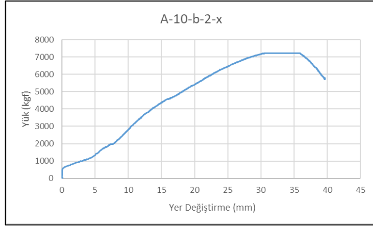
Şekil 5.17. A-10-b-2-x numunesinin Yük-Yer Değiştirme grafiği
