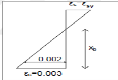
Şekil 3.3. Dengeli donatılı kesitte birim şekil değiştirme
