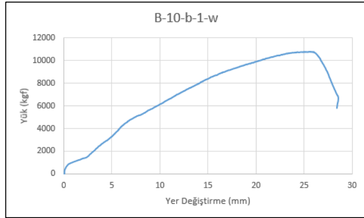
Şekil 5.11. B-10-b-1-w numunesinin Yük-Yer Değiştirme grafiği
