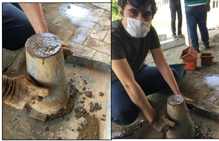
Şekil 4.19. Slump deneyi
