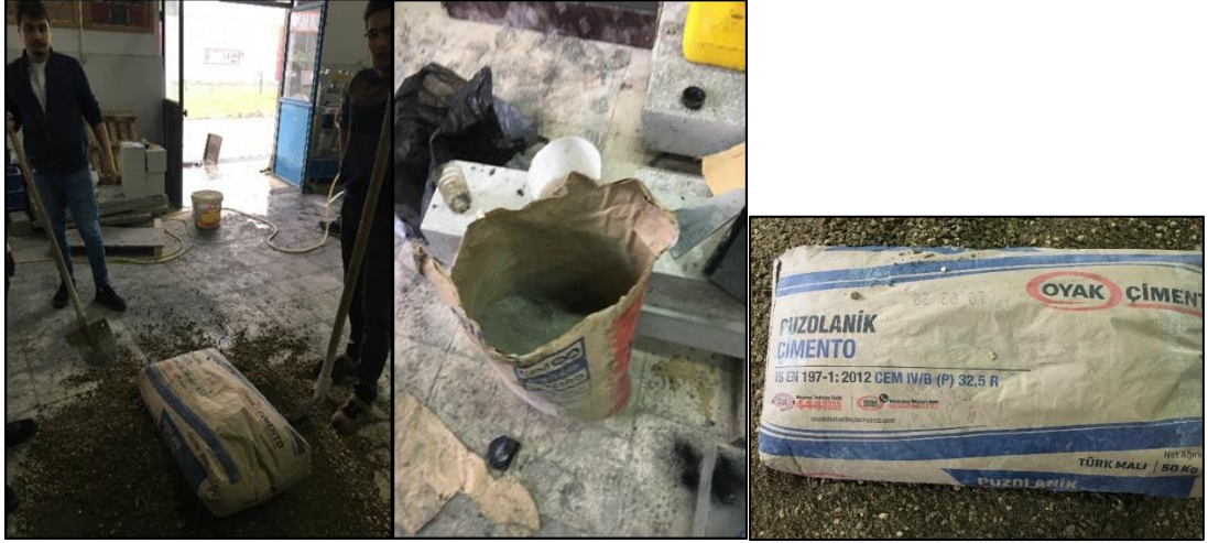
Şekil 4.3. Kullanılan çimento ile ilgili görseller
