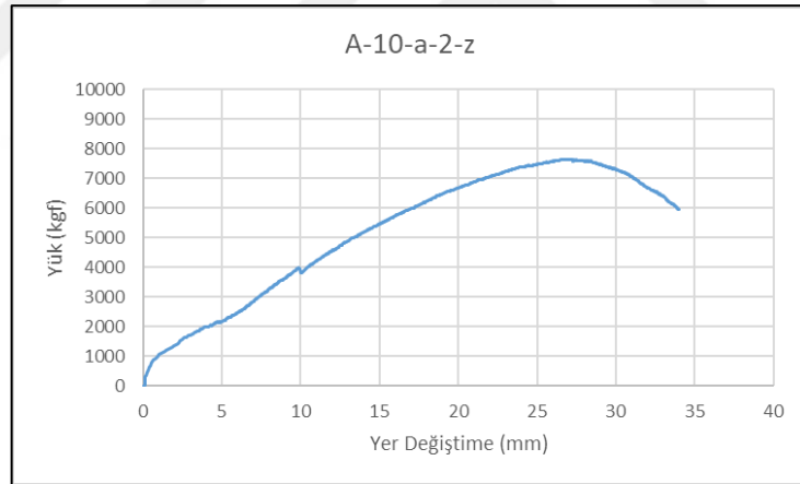
Şekil 5.20. A-10-a-2-z numunesinin Yük-Yer Değiştirme grafiği
