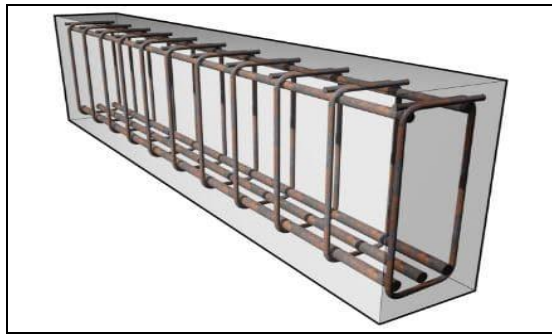
Şekil 2.5. Betonarme kiriş modellemesi [26]
