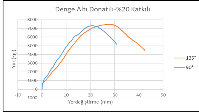
Şekil 6.13. A-10-a-2-y ve A-10-b-2-y numunelerinin Yük-Yer Değiştirme grafikleri
