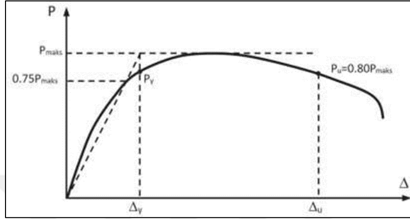
Şekil 5.7. Süneklilik grafiği [29]
