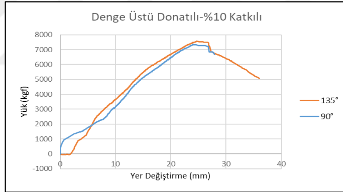
Şekil 6.12. B-10-a-2-x ve B-10-b-2-x numunelerinin Yük-Yer Değiştirme grafikleri
