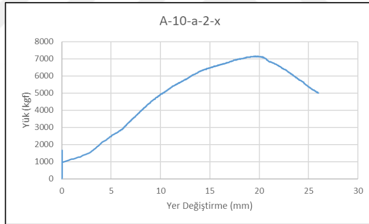
Şekil 5.16. A-10-a-2-x numunesinin Yük-Yer Değiştirme grafiği
