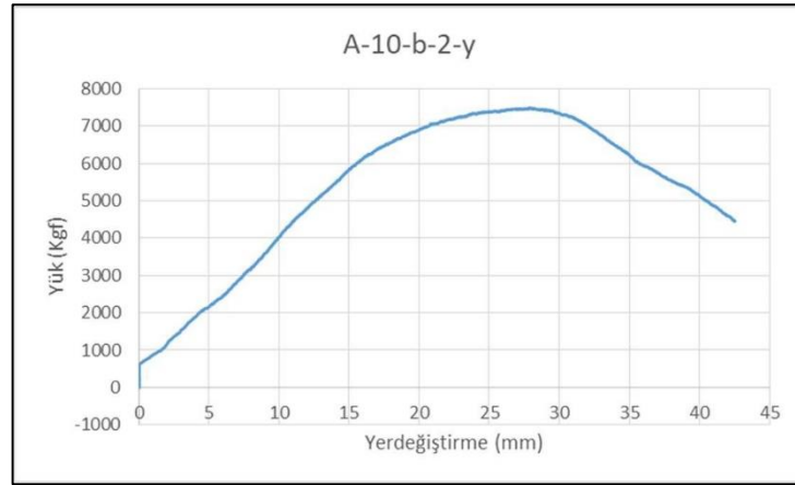
Şekil 5.13. A-10-b-2-y numunesinin Yük-Yer Değiştirme grafiği
