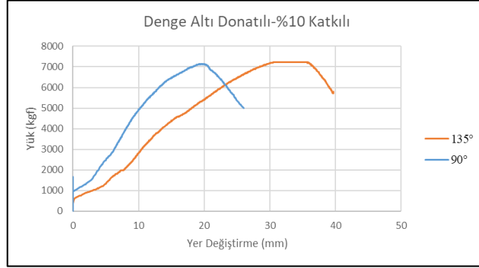
Şekil 6.11. A-10-a-2-x ve A-10-b-2-x numunelerinin Yük-Yer Değiştirme grafikleri
