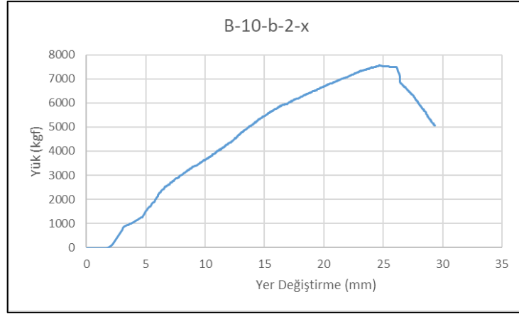
Şekil 5.19. B-10-b-2-x numunesinin Yük-Yer Değiştirme grafiği
