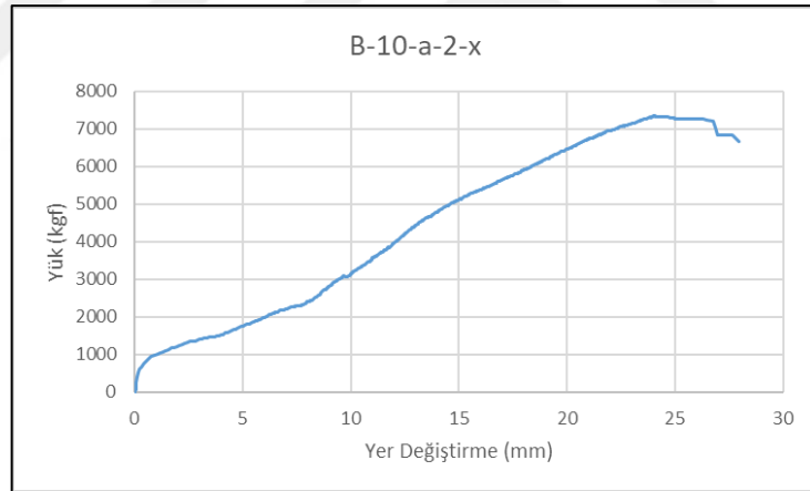
Şekil 5.18. B-10-a-2-x numunesinin Yük-Yer Değiştirme grafiği
