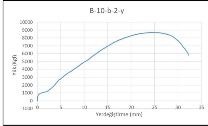
Şekil 5.15. B-10-b-2-y numunesinin Yük-Yer Değiştirme grafiği
