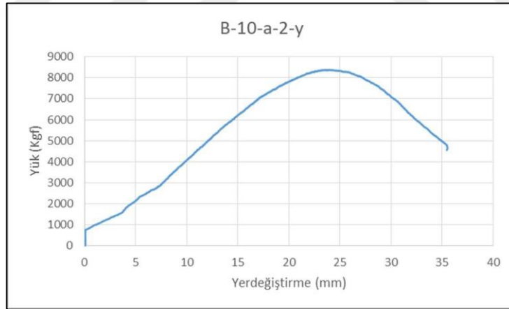
Şekil 5.14. B-10-a-2-y numunesinin Yük-Yer Değiştirme grafiği
