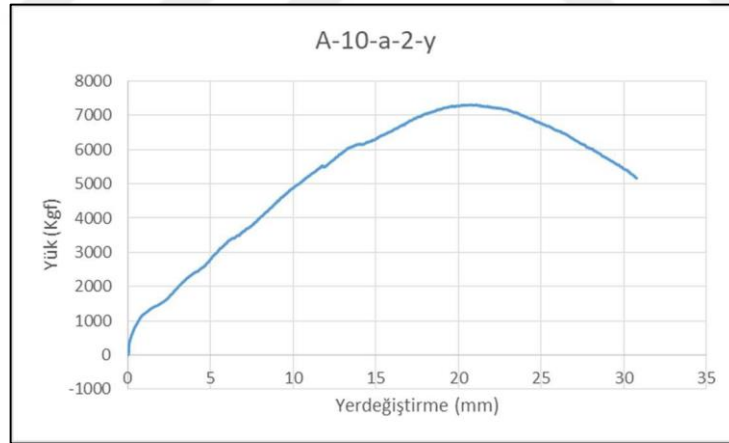
Şekil 5.12. A-10-a-2-y numunesinin Yük-Yer Değiştirme grafiği
