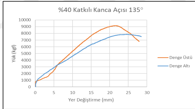
Şekil 6.8. A-10-b-2-z ve B-10-b-2-z numunelerinin karşılaştırma grafiği
