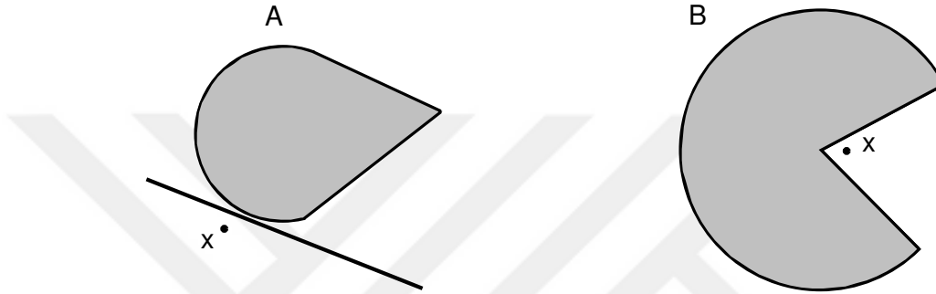
Şekil 4.5. x noktası A 'dan ayrılabilir, B 'den ayrılamaz
