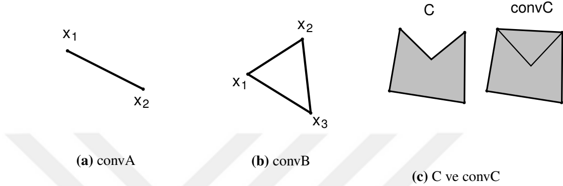
Şekil 3.1. A, B, C kümelerine ait konveks kabuklar
