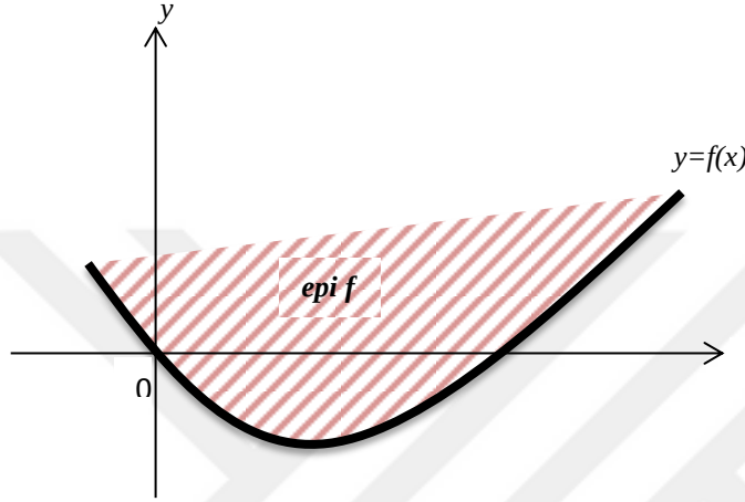
Şekil 3.2. f fonksiyonunun grafiküstü kümesi
