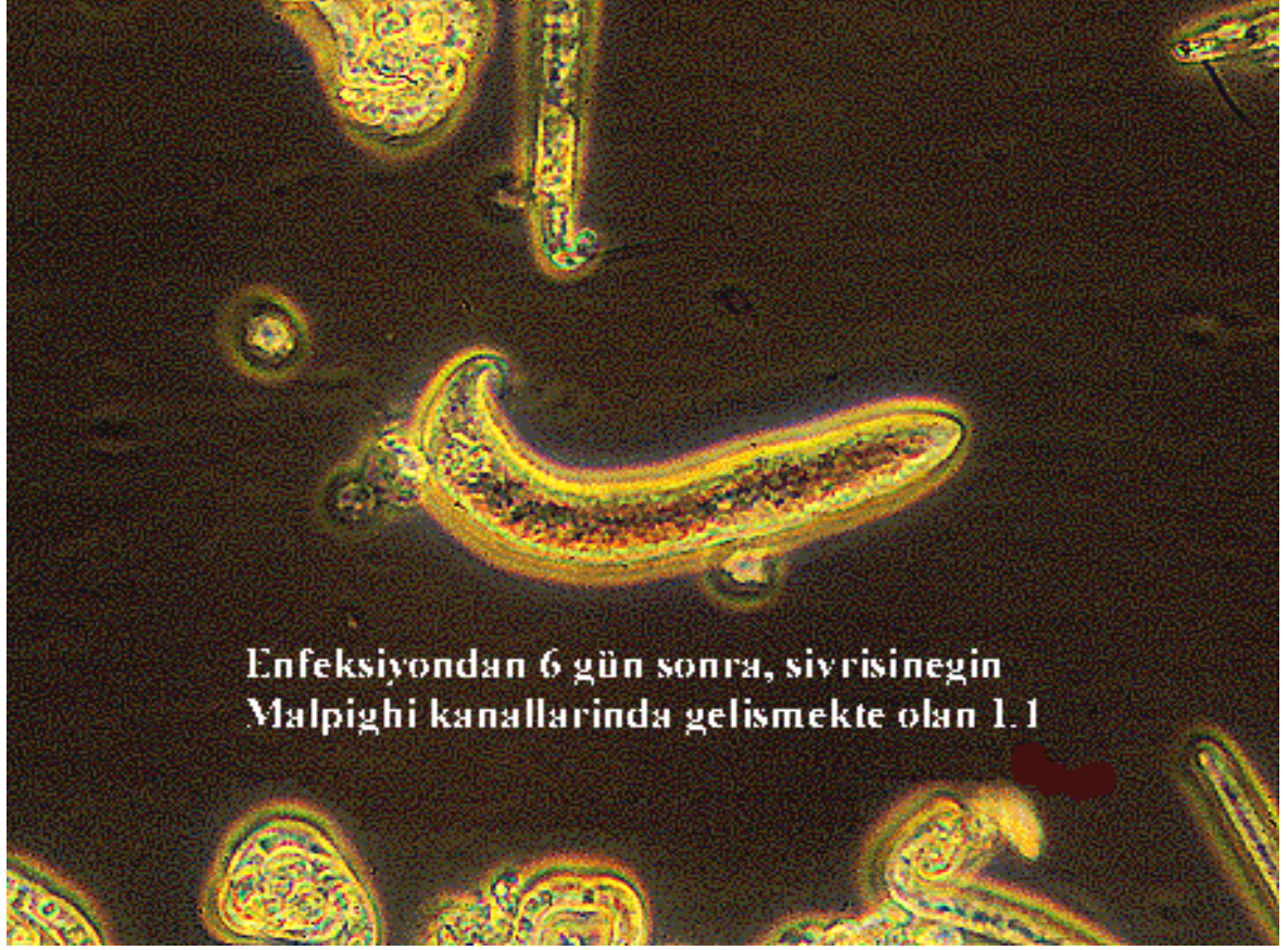
Şekil 1.1.4. Sivrisinekte malpighi kanalında Dirofilaria immitis larvası (L 1 ) (Johnstone, 2000)
