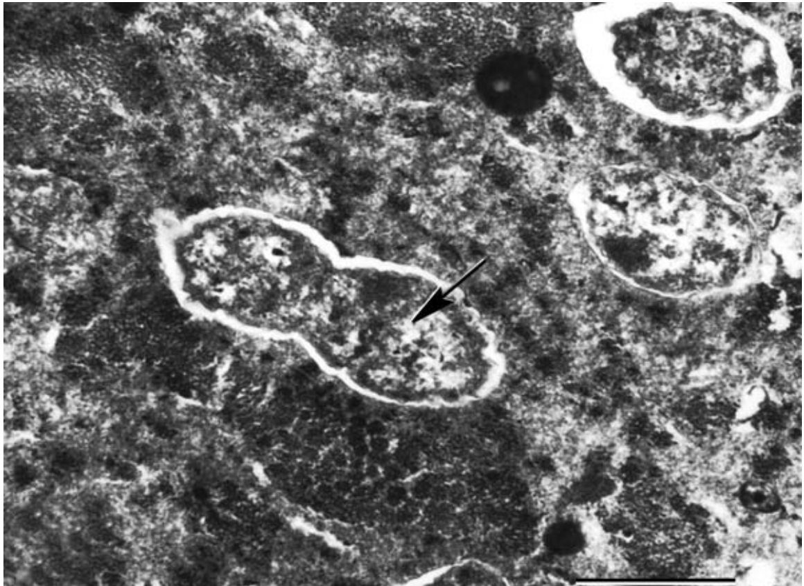
řekil 1.2.3. İkiye blnerek oęalan bir Wolbachia 'nın elektron mikroskopik grnts. Skala bar=0,5 \mu m) (Kozek 2005).
