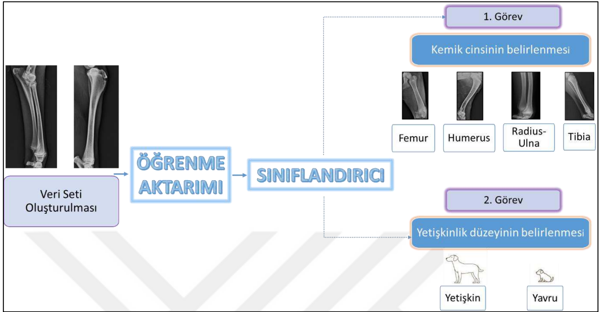
Şekil 1.1. Yazılım iskeleti: 1. ve 2. görevler.
