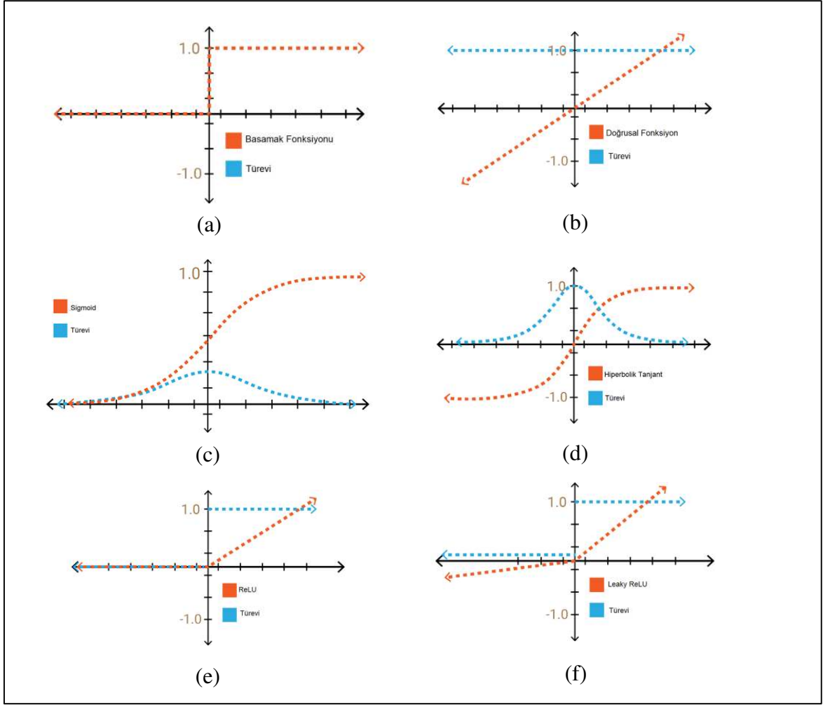
Şekil 2.20. Sinir ağlarında kullanılan aktivasyon fonksiyonları ve türevleri. a) basamak fonksiyonu, b) doğrusal fonksiyon, c) sigmoid fonksiyonu, d) tanh fonksiyonu, e) ReLU fonksiyonu ve f) sızıntı ReLU fonksiyonu [60].
