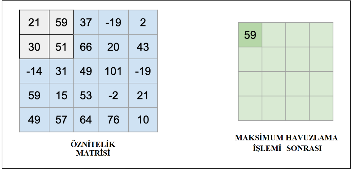
Şekil 2.17. Havuzlama işlemi.
