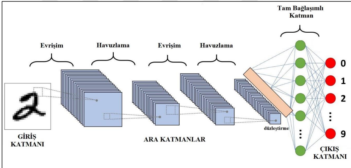
Şekil 2.10. Klasik bir derin öğrenme modeli katmanları [56].
