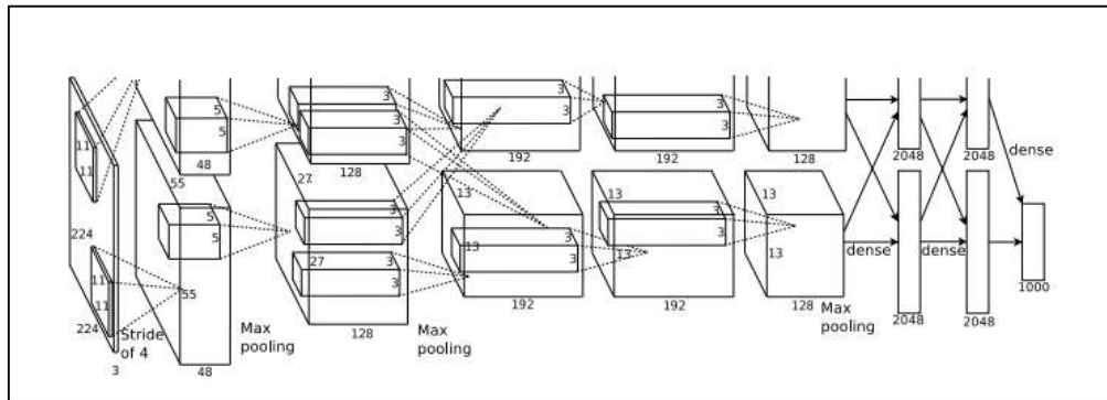
Şekil 2.26. AlexNet mimarisi [63].
