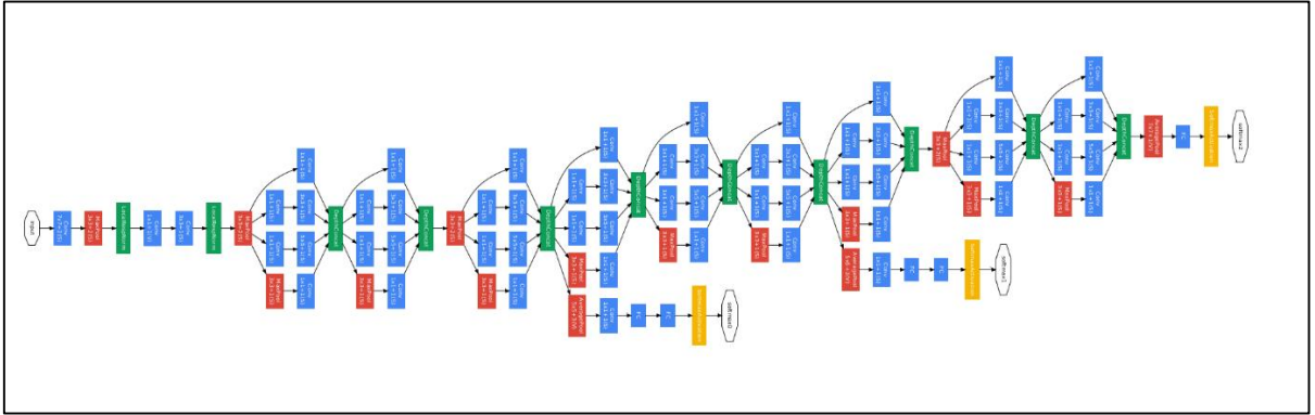
Şekil 2.27. GoogLeNet mimarisi [64].
