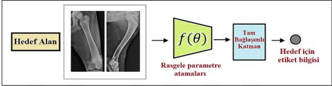
Şekil 2.23. Sıfırdan öğrenme.
