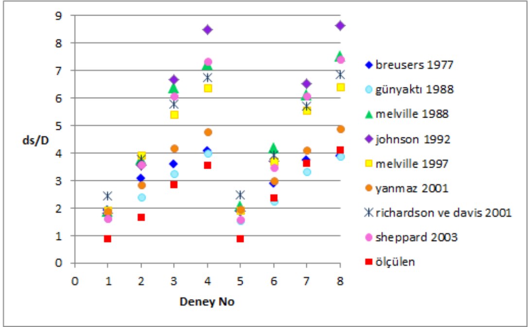
Şekil 4.11 Deneyler sırasında ölçülen ve literatürde verilen bağıntılarla hesaplanan oyulma derinlikleri
