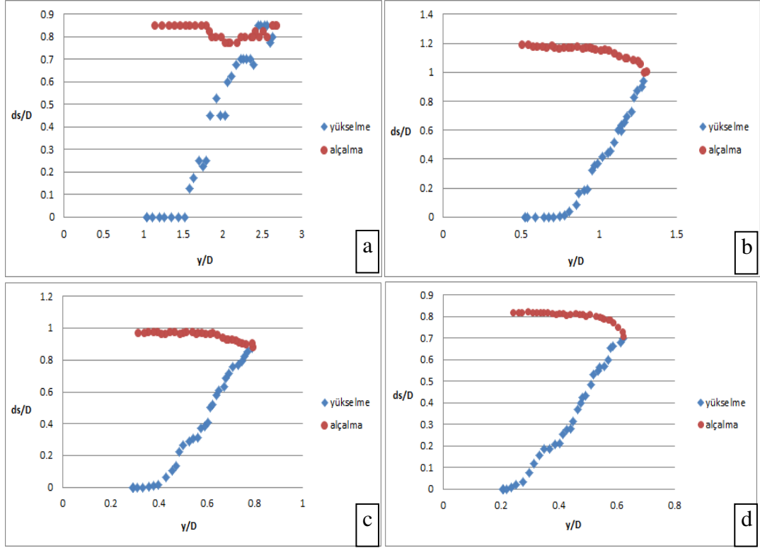
Şekil 4.6 a) 4 cm, b) 8 cm, c) 15 cm, d) 20 cm çapındaki köprü ayakları ve Hid 2 hidrografi ile yapılan deneylerde ds/D 'nin y/D ile değişimi grafikleri
