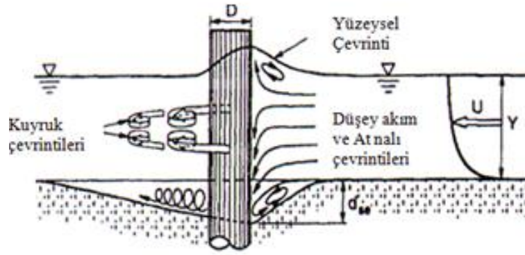
Şekil 2.3 Bir köprü ayağı etrafındaki çevrintiler ve oyulma çukuru (Ettema, 1998)
