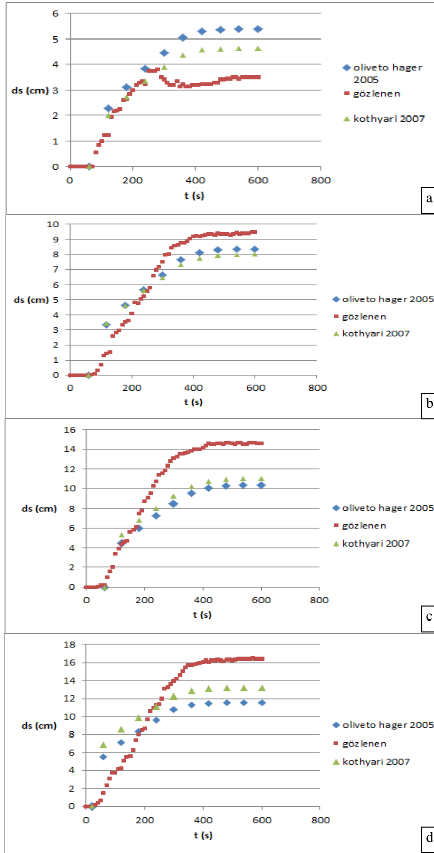
Şekil 4.14 a) 4 cm, b) 8 cm, c) 15 cm, d) 20 cm çapındaki köprü ayakları ve Hid 2 hidrografi ile yapılan deneylerde oyulma derinliklerinin karşılaştırılması
