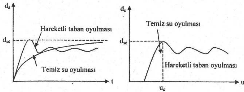
Şekil 2.2 Köprü ayakları etrafındaki oyulma derinliğinin değişimi (Yanmaz,2002)
