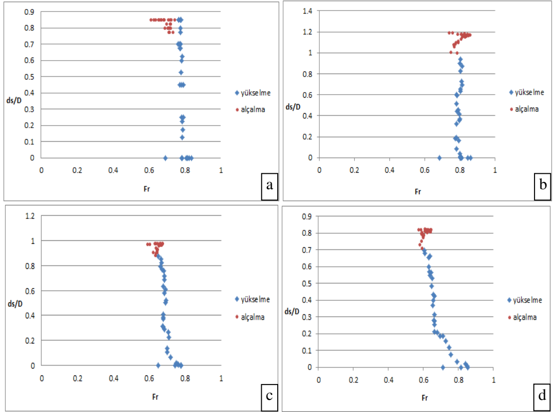
Şekil 4.10 a) 4 cm, b) 8 cm, c) 15 cm, d) 20 cm çapındaki köprü ayakları ve Hid 2 hidrografi ile yapılan deneylerde ds/D 'nin Fr ile değişimi grafikleri
