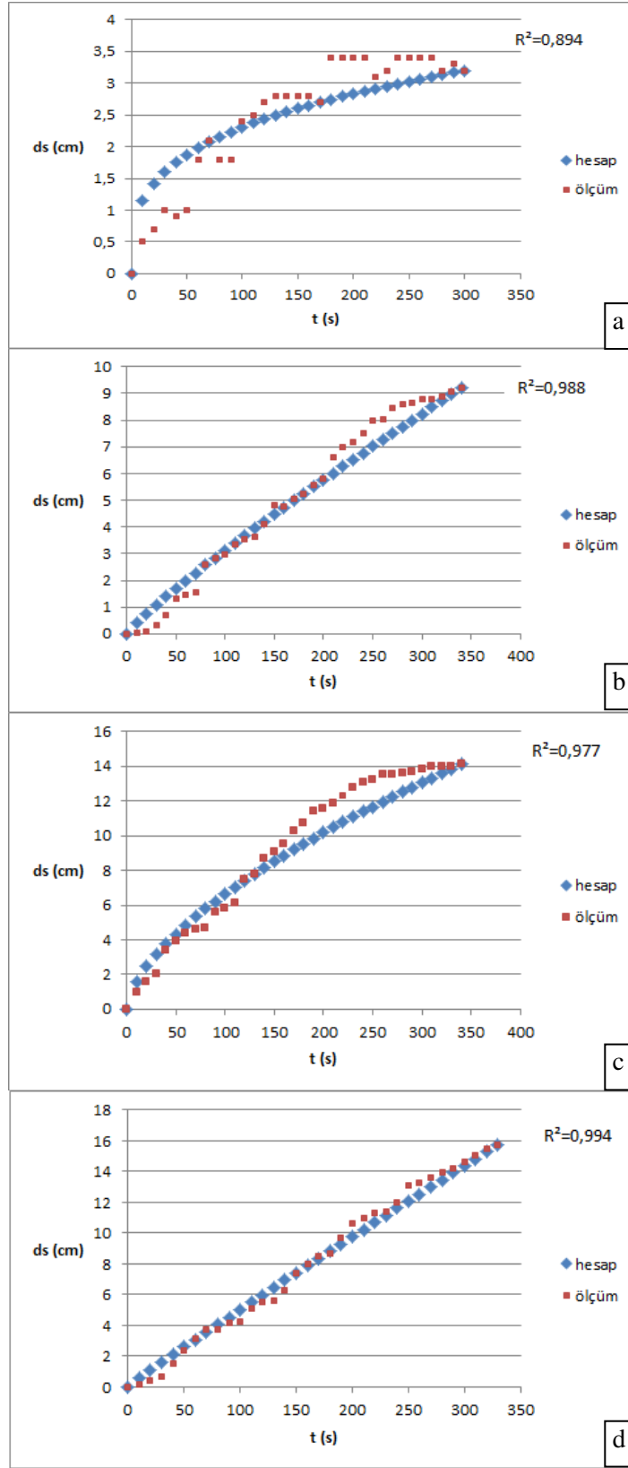
Şekil 4.17 a) Hid2D4 b) Hid2D8, c) Hid2D15, d) Hid2D20 deneylerinde ölçülen ve 4.3 ampirik bağıntısıyla hesaplanan oyulma değerlerinin karşılaştırılması
