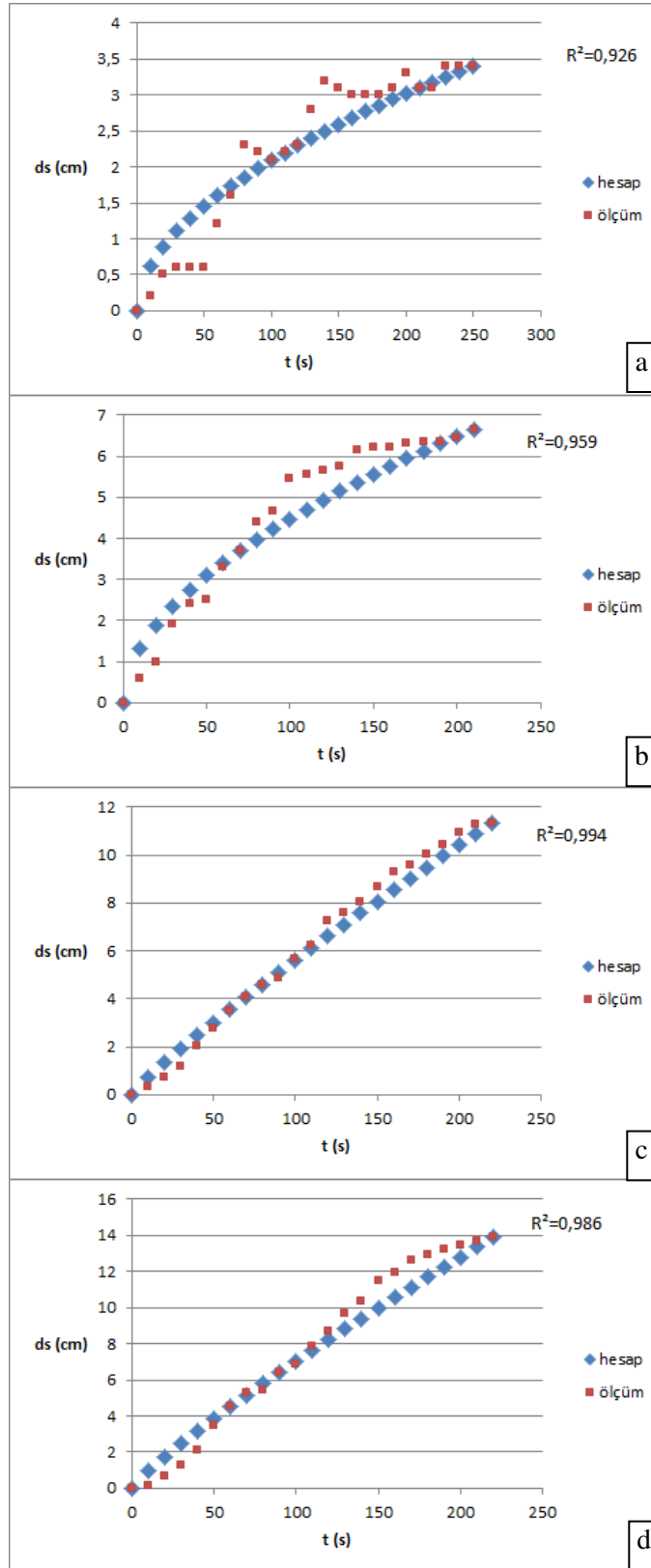
Şekil 4.16 a) Hid1D4 b) Hid1D8, c) Hid1D15, d) Hid1D20 deneylerinde ölçülen ve 4.3 ampirik bağıntısıyla hesaplanan oyulma değerlerinin karşılaştırılması
