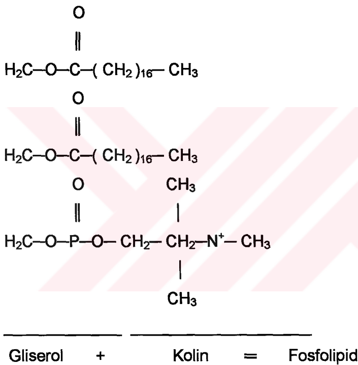
Şekil 2.12. Fosfolipid
