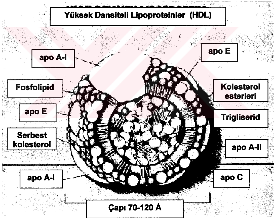
Şekil 2.19. HDL yapısı
