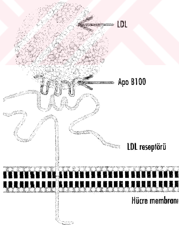
Şekil 2.15.a. LDL partikülü
