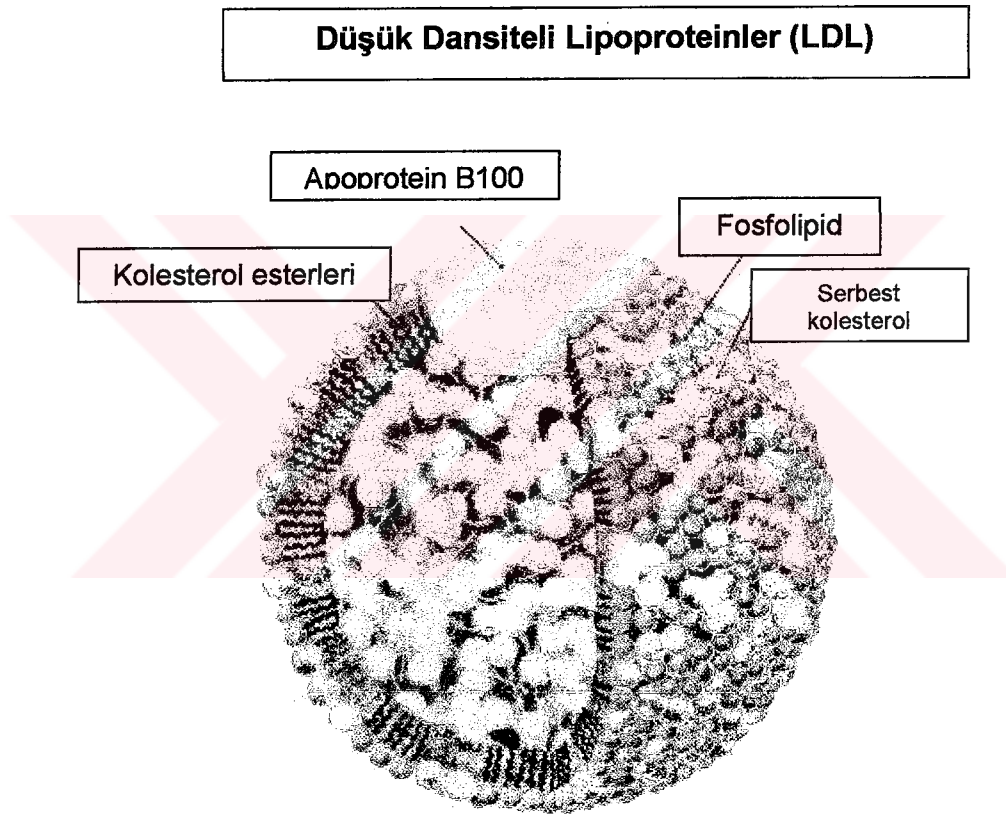
Şekil 2.18. LDL yapısı
