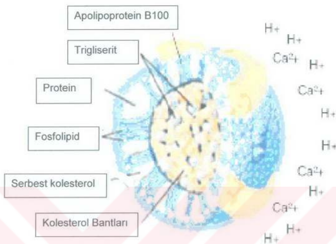
Şekil 2.8.b Lipoprotein elemanları
