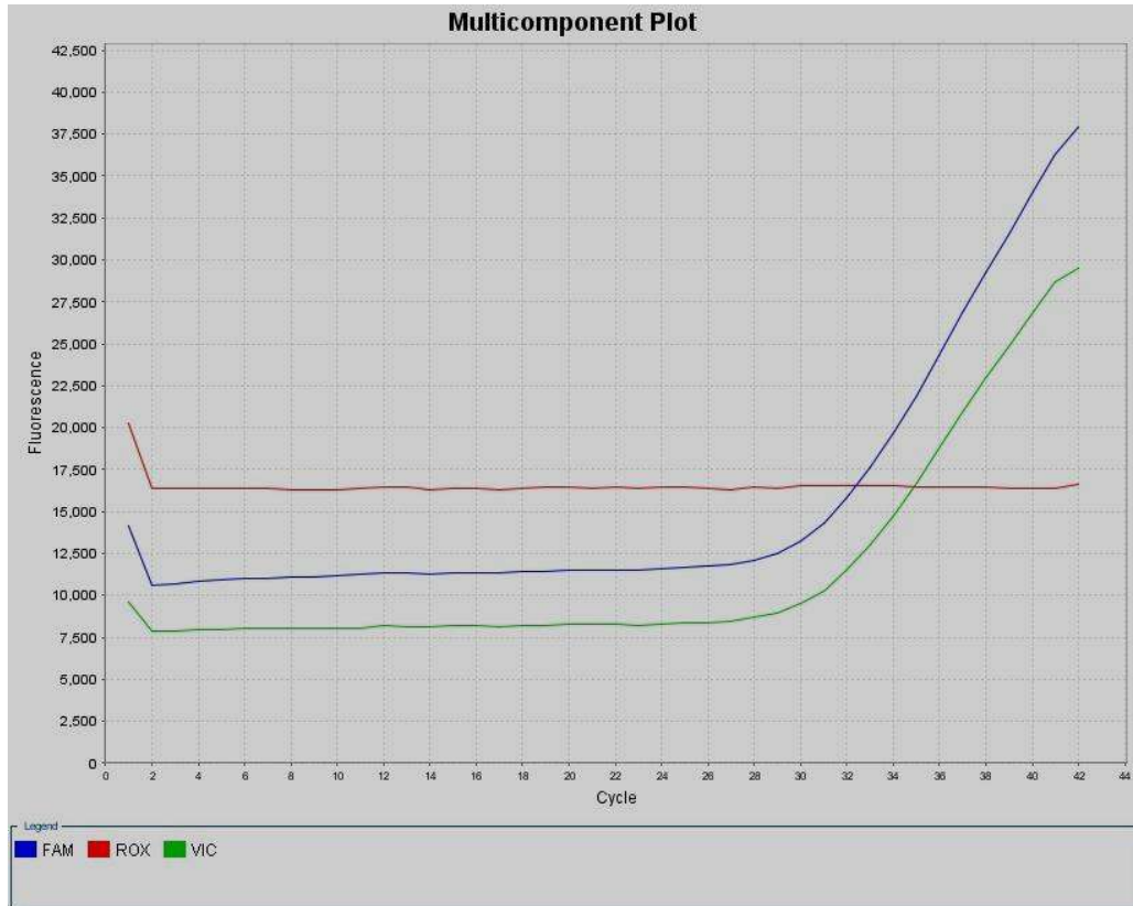
Şekil 8. Heterozigot tip multicomponent plot görünümü
