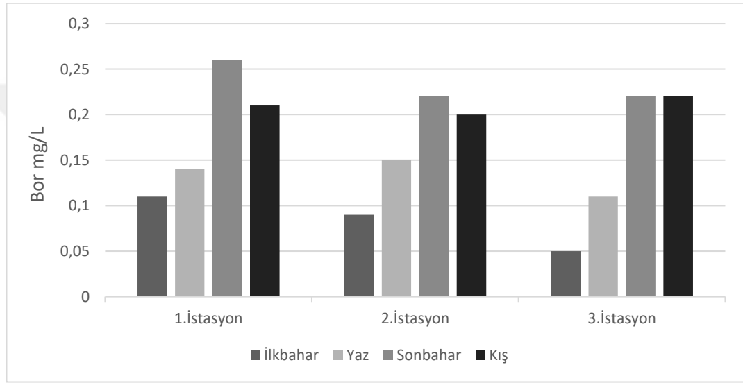
Şekil 4.12 Araştırmada ölçülen borun mevsimsel grafiği
