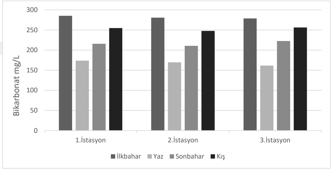
Şekil 4.10 Araştırmada ölçülen bikarbonatın mevsimsel grafiği
