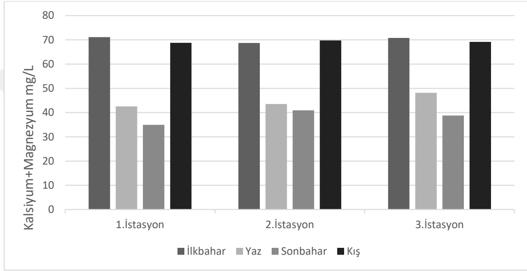
Şekil 4.13 Araştırmada ölçülen kalsiyum+magnezyumun mevsimsel grafiği
