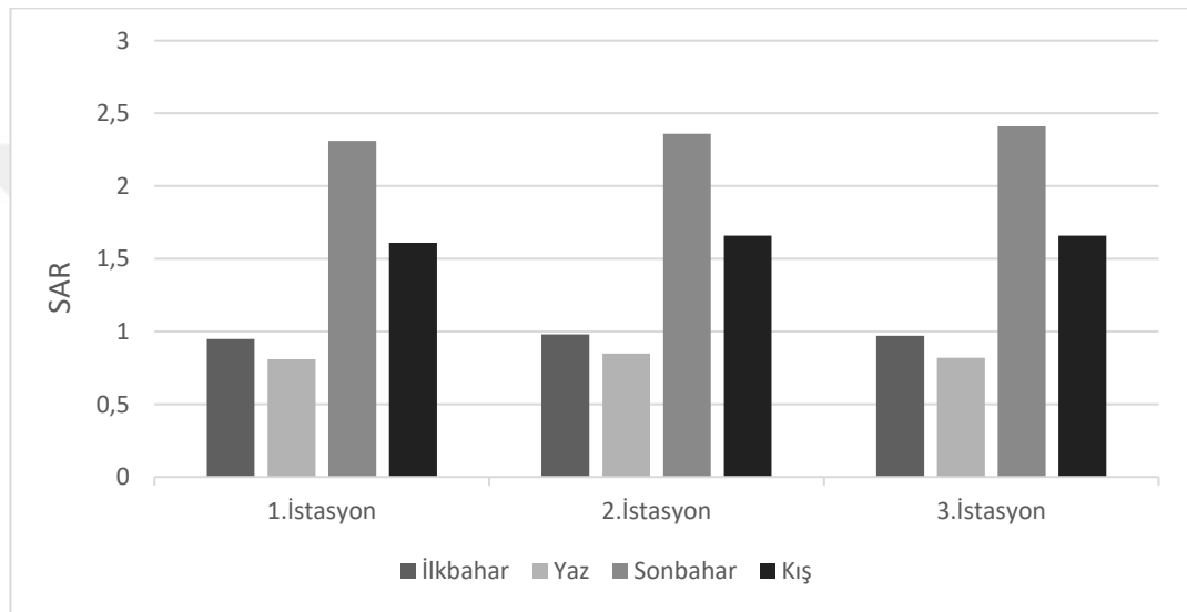
Şekil 4.14 Araştırmada ölçülen sodyum adsorbsiyon oranının mevsimsel grafiği
