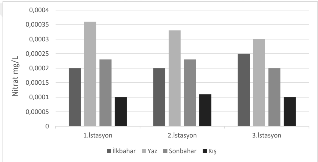
Şekil 4.19 Araştırmada ölçülen nitritin mevsimsel grafięi
