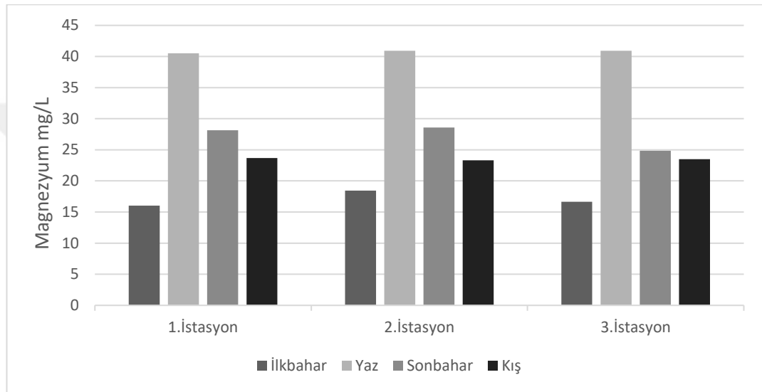
Şekil 4.15 Araştırmada ölçülen magnezyumun mevsimsel grafięi
