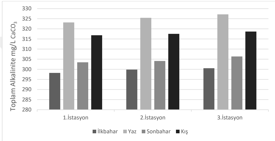
Şekil 4.16 Araştırmada ölçülen toplam alkalinitenin mevsimsel grafięi
