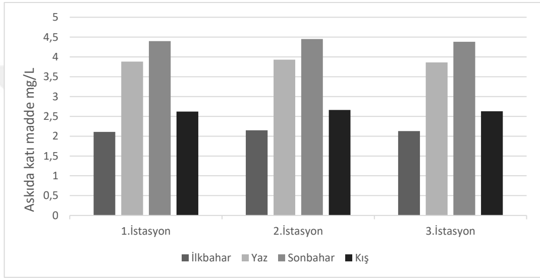
Şekil 4.17 Araştırmada ölçülen askıda katı maddenin mevsimsel grafiği
