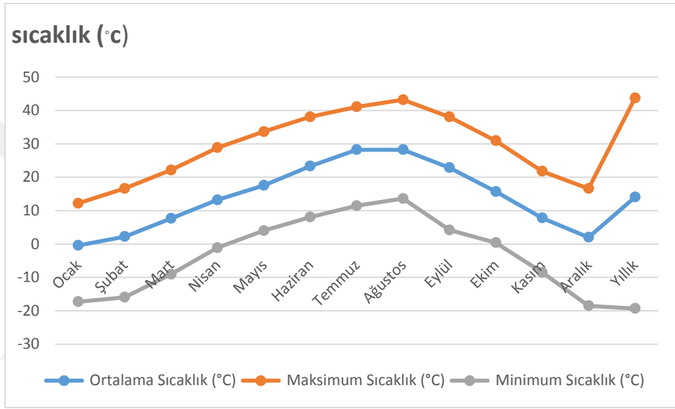
Şekil 1. Kovancılar Meteoroloji İstasyonu En Yüksek ve En Düşük Sıcaklıklar Ortalaması
