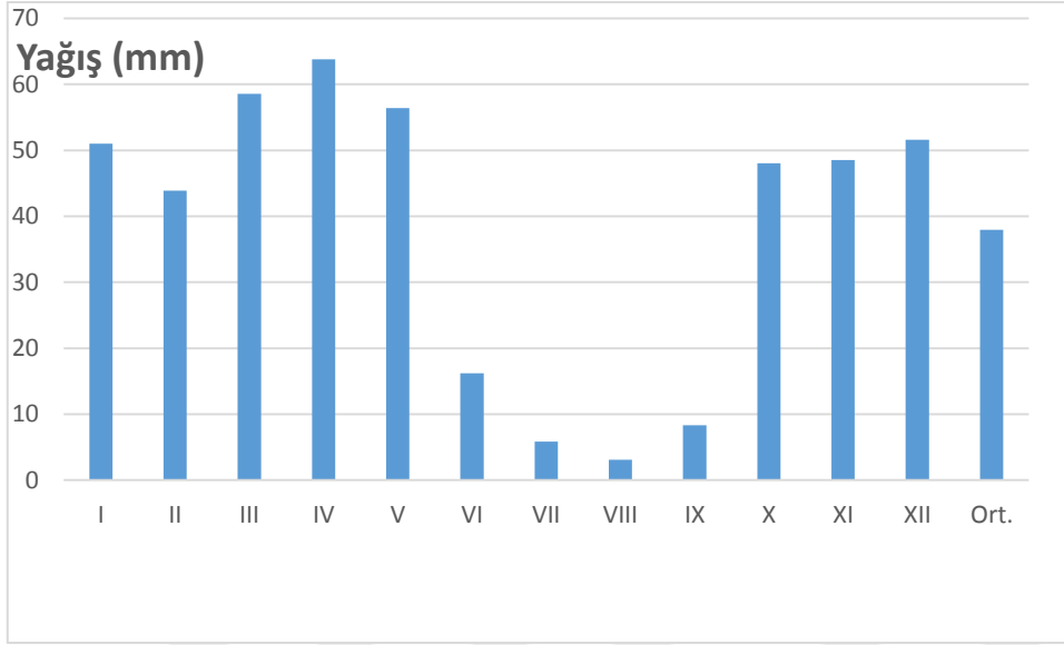
Şekil 2. Kovancılar Meteoroloji İstasyonuna Ait Yağış Grafiği
